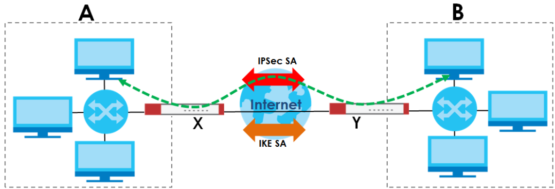
Figure 392 VPN: IKE SA and IPsec SA
