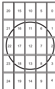
5 x 5
