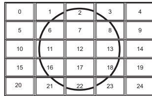
5 x 5
