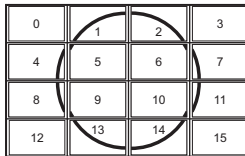
4 x 4
