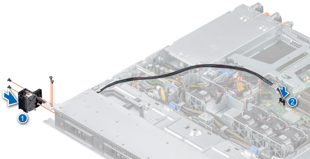
Figure 79. Installation du panneau de commande gauche
