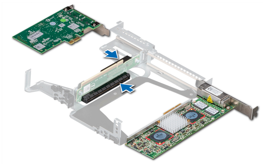
Figure 44. Installation d'une carte d'extension dans la carte de montage pour carte d'extension
