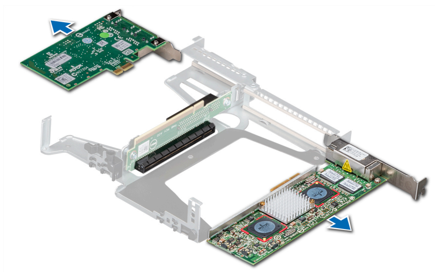
Figure 41. Retrait de la carte d'extension de la carte de montage pour carte d'extension
