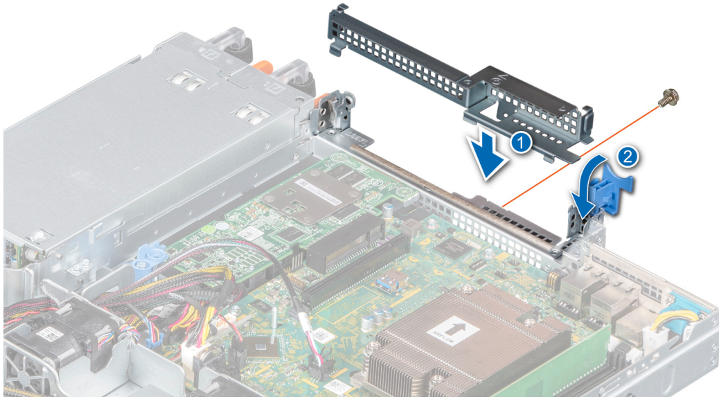
Figure 38. Installation de la plaque de recouvrement de la carte de montage pour carte d'extension
