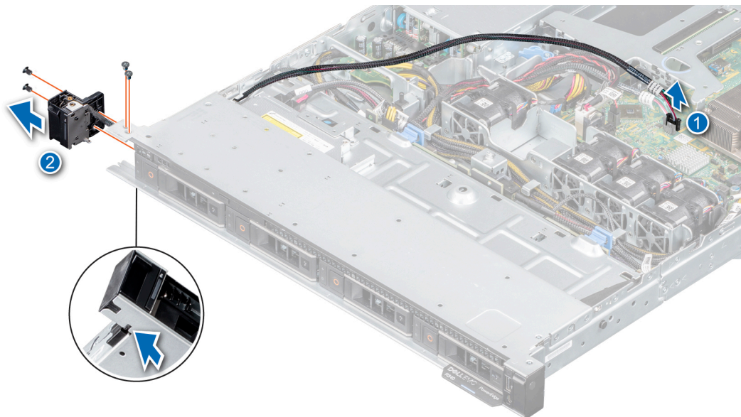
Figure 78. Retrait du panneau de commande gauche
