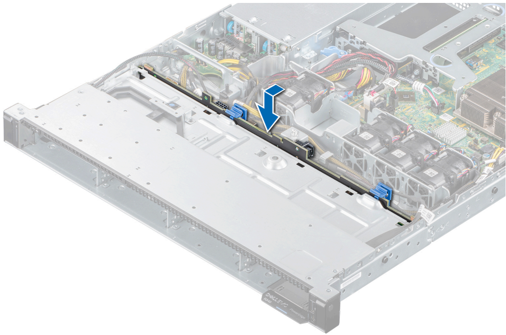
Figure 64. Installation du backplane de disque
