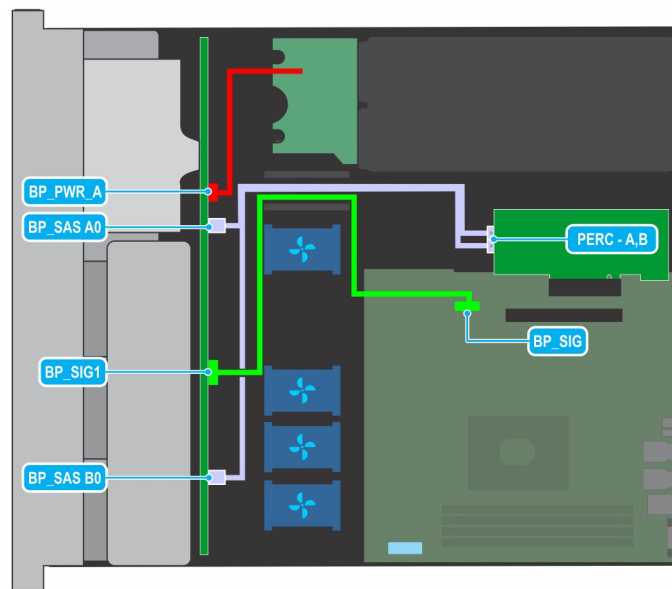
Figure 66. Acheminement des câbles : 8 fonds de panier SAS de 2,5 pouces avec carte PERC
