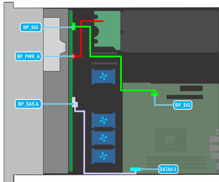
Figure 65. Acheminement des câbles - 4 fonds de panier SATA de 3,5 pouces
