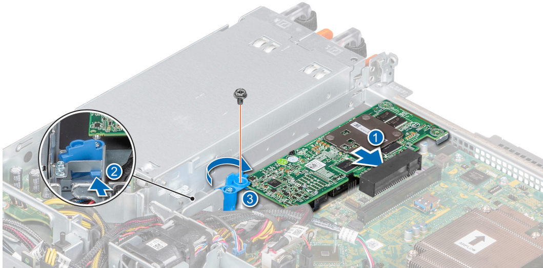
Figure 46. Installation de la carte PERC
