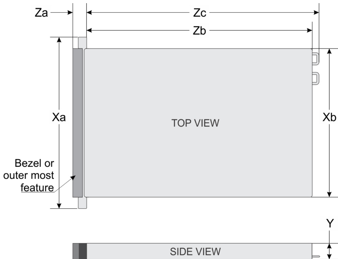
Figure 83. Dimensions du châssis
