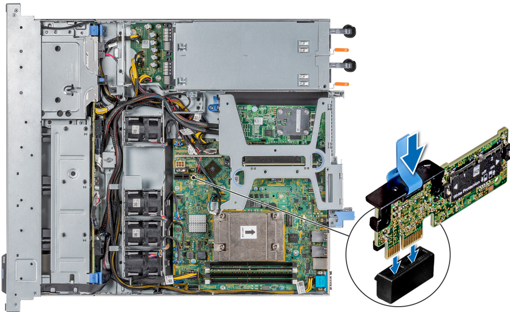
Figure 56. Installation de la carte IDSDM ou vFlash (en option)
