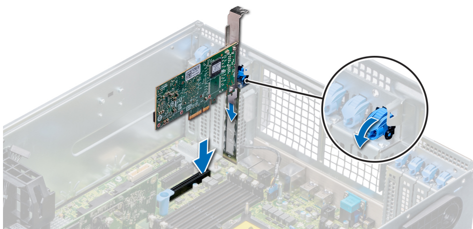
Figure 84. Installation d'une carte d'extension
