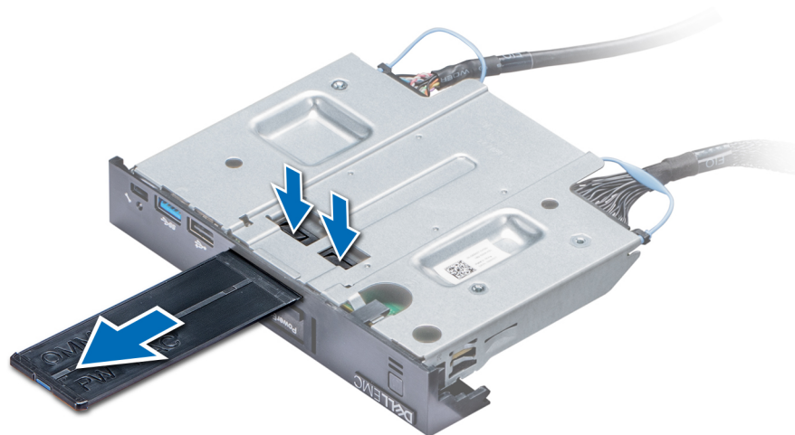
Figure 107. Retrait de la plaquette d'informations
