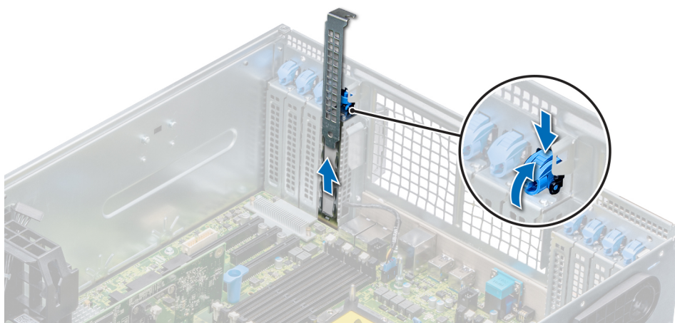
Figure 83. Retrait de la plaque de recouvrement
