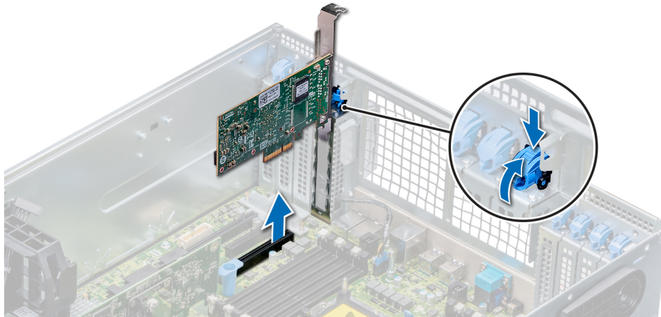
Figure 81. Retrait d'une carte d'extension
