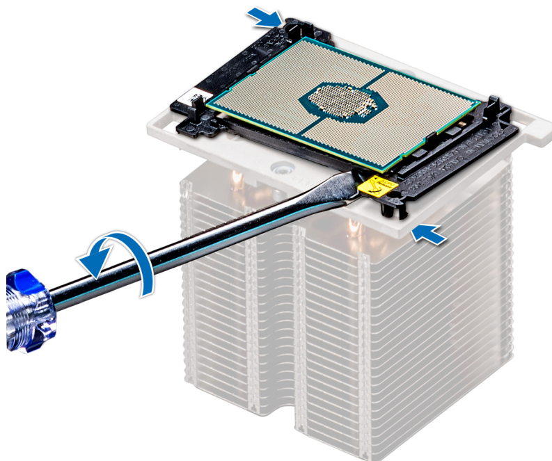
Figure 71. Pliage du support de processeur
