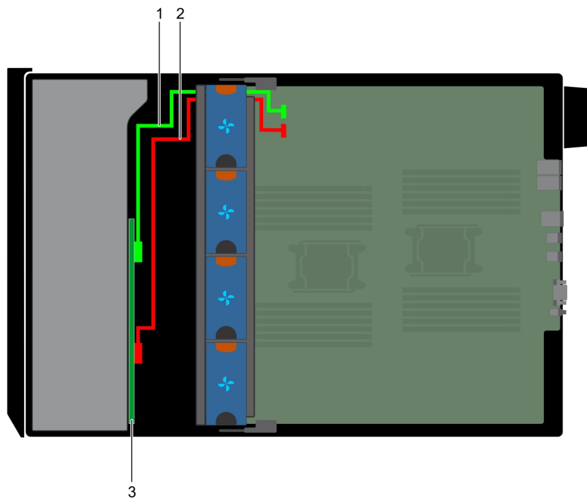
Figure 100. Contrôleur SAS intégré à 8 disques de 3,5 pouces
