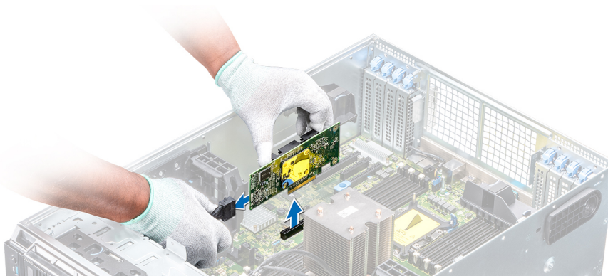
Figure 102. Retrait de la carte contrôleur de stockage intégrée
