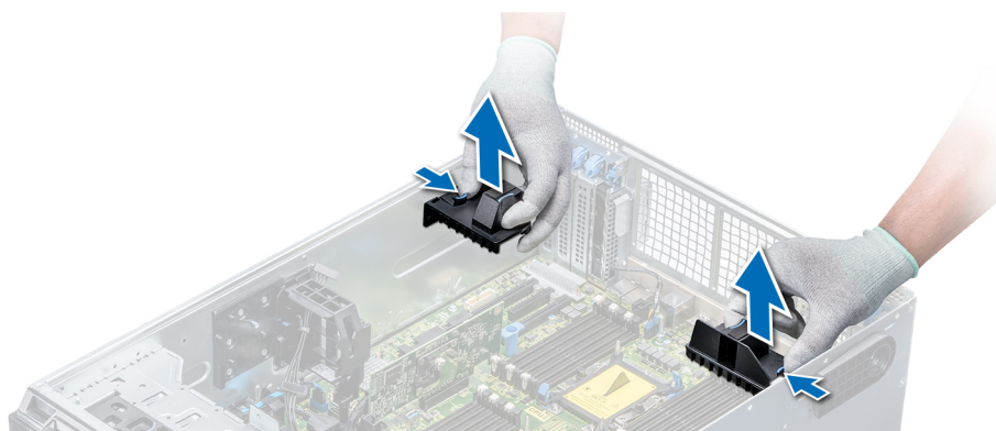
Figure 77. Retrait du support de carte d'extension
