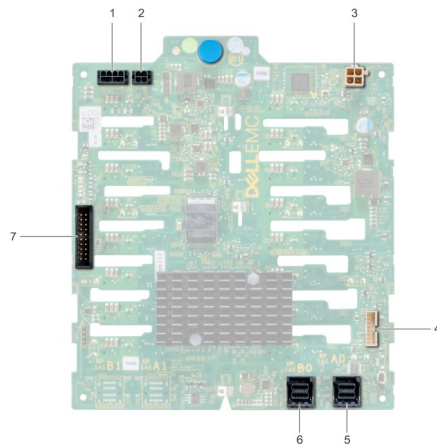
Figure 91. Backplane SAS/SATA à 16 disques de 2,5 pouces
