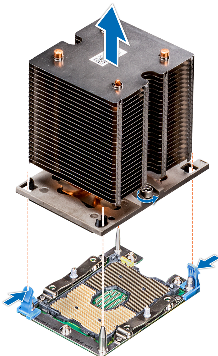
Figure 70. Retrait du module du processeur et du dissipateur de chaleur
