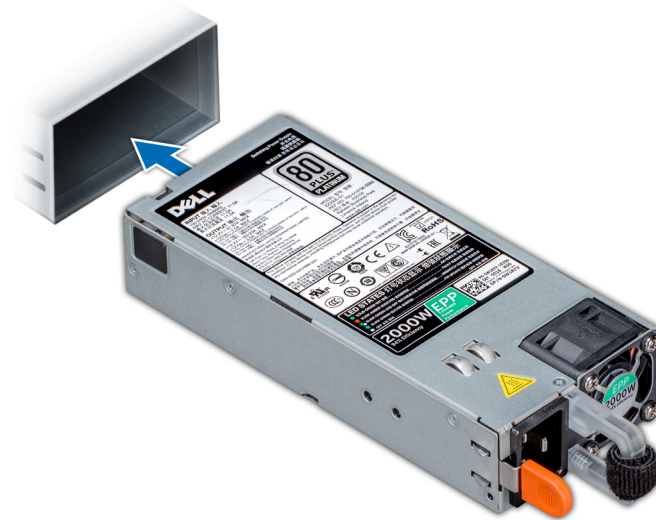
Figure 44. Installation d'une unité d'alimentation
