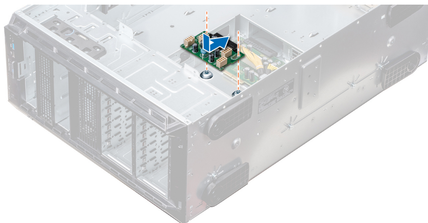
Figure 117. Installation de la carte intercalaire d'alimentation (PIB) GPU
