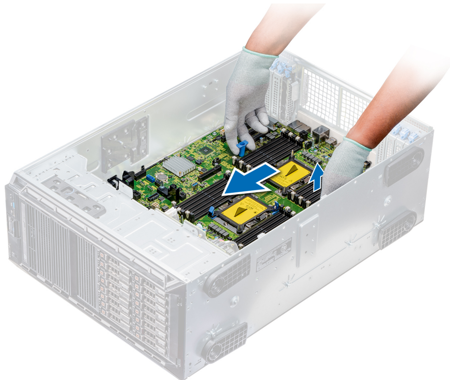
Figure 111. Retrait de la carte système
