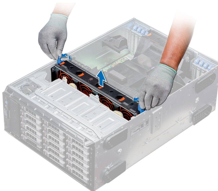
Figure 55. Retrait du module de ventilation central
