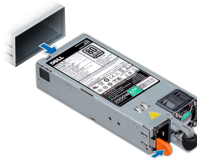
Figure 43. Retrait d'une unité d'alimentation
