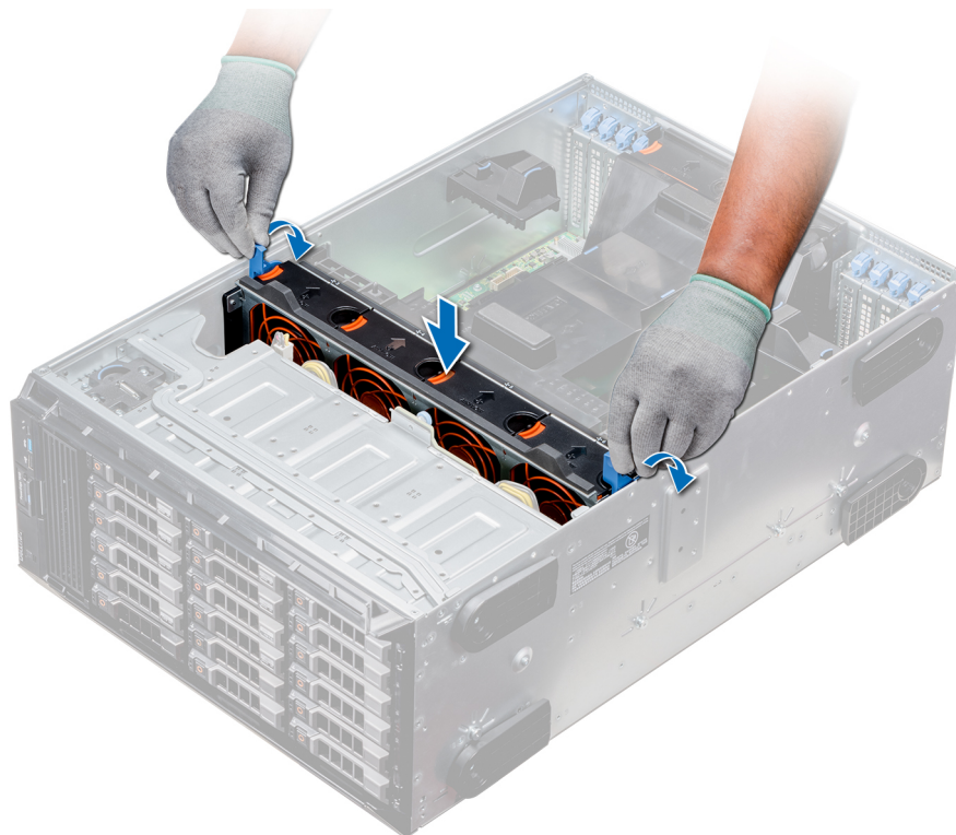
Figure 56. Installation du module de ventilation central
