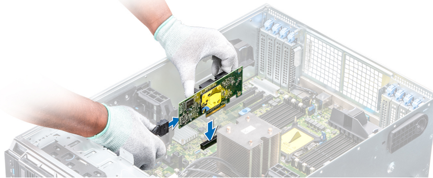
Figure 103. Installation de la carte contrôleur de stockage intégrée
