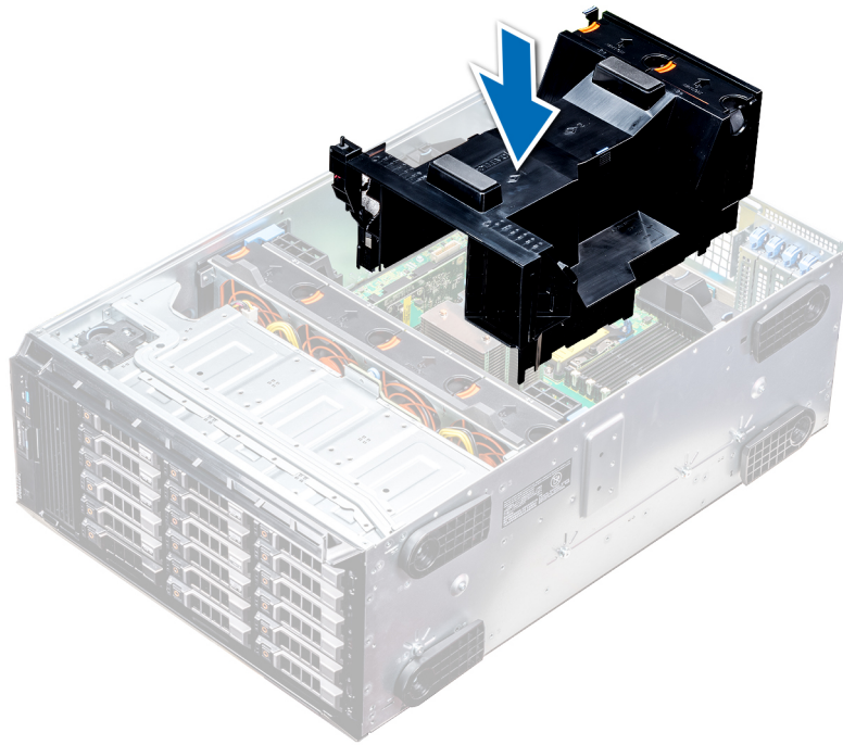
Figure 50. Installation du carénage d'aération
