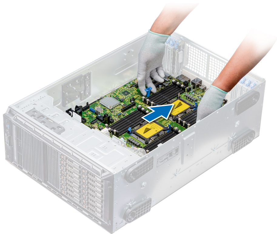
Figure 113. Installation de la carte système
