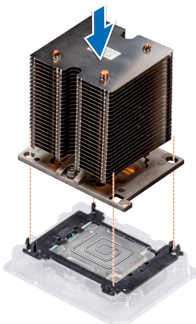
Figure 75. Installation du dissipateur de chaleur sur le processeur
