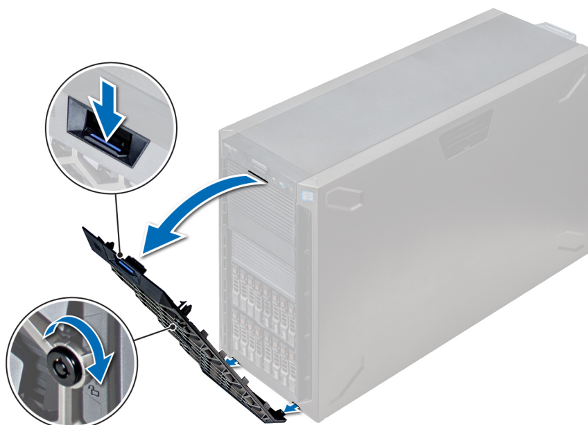
Figure 25. Retrait du cadre avant
