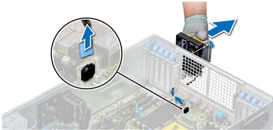
Figure 53. Retrait du ventilateur externe gauche
