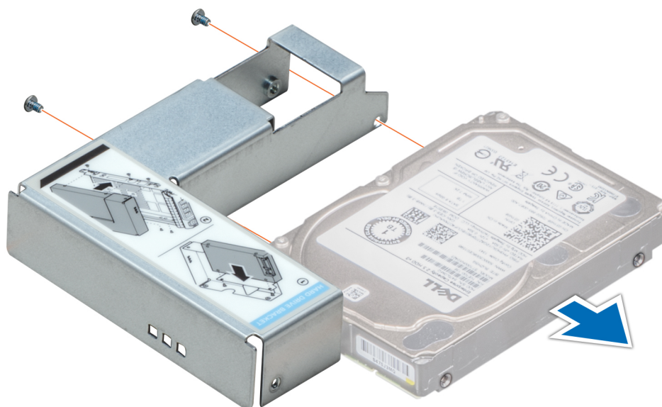
Figure 39. Retrait d'un lecteur de 2,5 pouces d'un adaptateur de lecteur de 3,5 pouces
