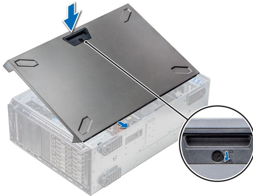
Figure 46. Installation du capot du système
