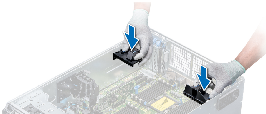
Figure 78. Installation du support de carte d'extension
