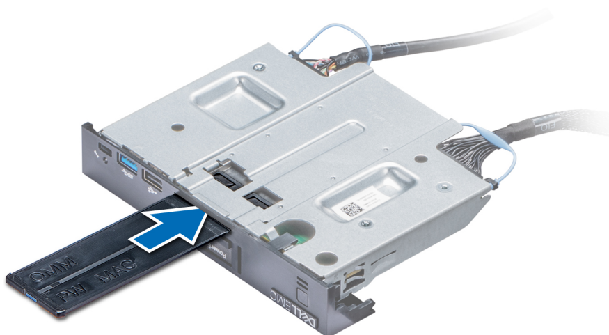
Figure 108. Installation de la plaquette d'informations
