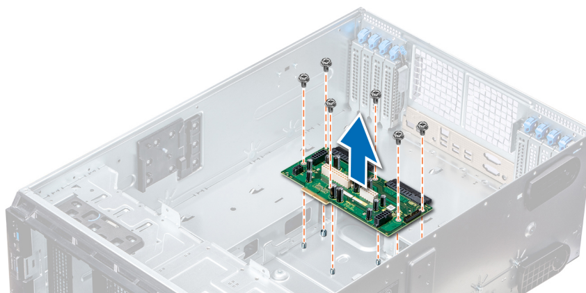
Figure 118. Retrait de la carte PIB principale
