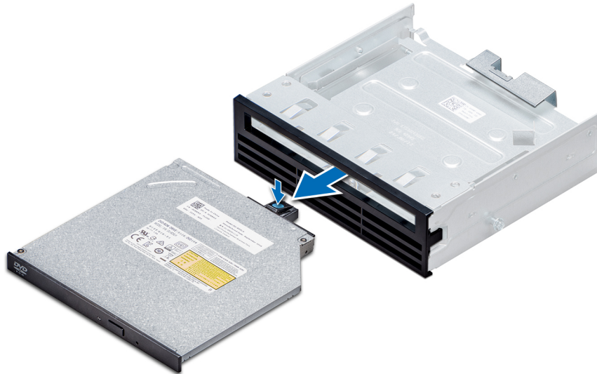
Figure 63. Retrait du cache du lecteur optique slim
