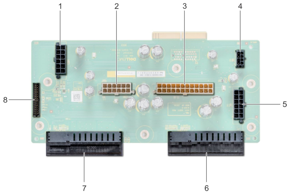
Figure 114. Principale carte intercalaire d'alimentation
