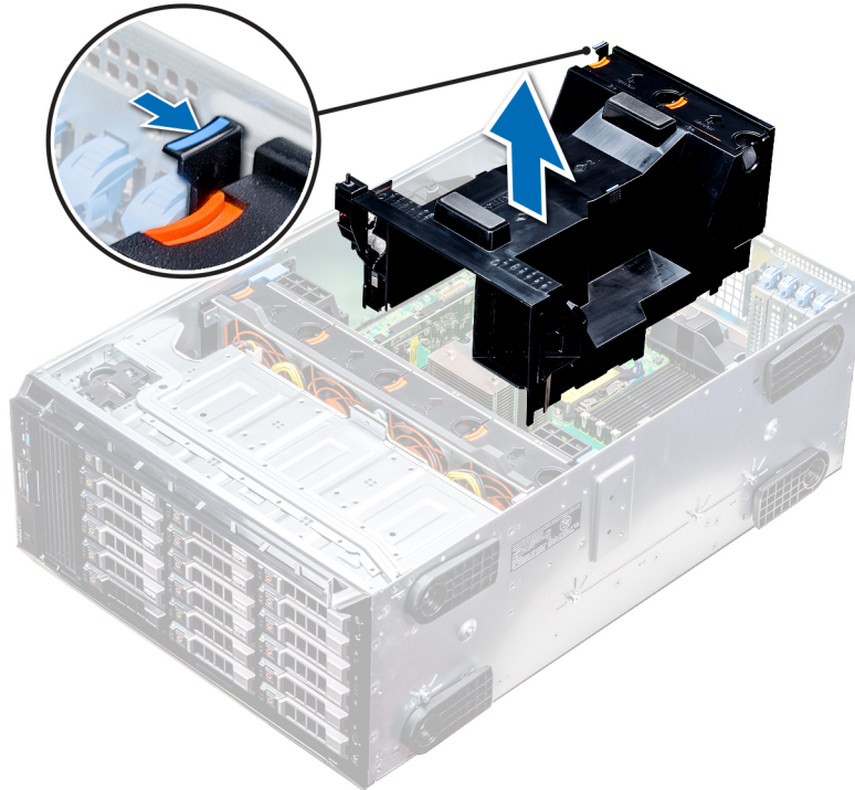
Figure 49. Retrait du carénage d'aération
