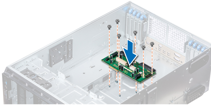
Figure 119. Installation de la principale carte intercalaire d'alimentation
