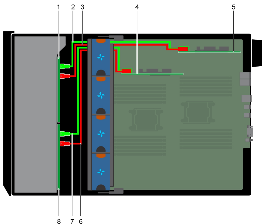
Figure 97. 32 disques SAS/SATA de 2,5 pouces vers PERC interne et adaptateur PERC
