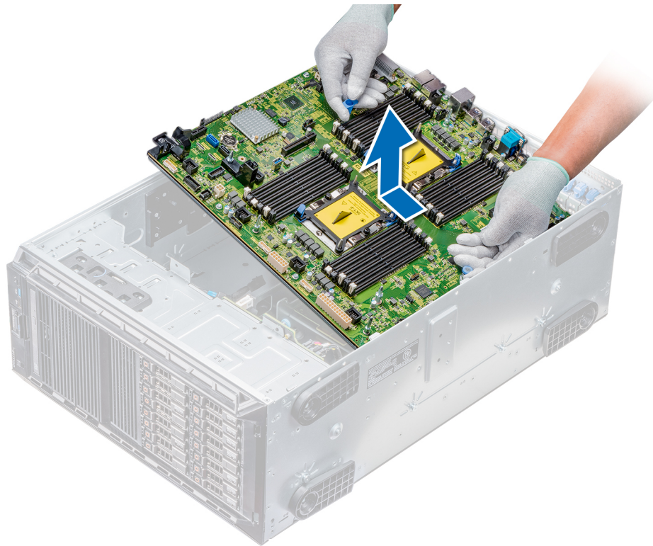
Figure 112. Retrait de la carte système
