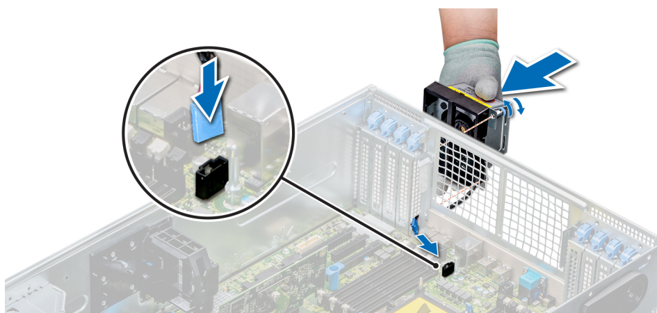
Figure 24. Installation du ventilateur externe droit
