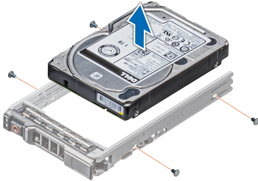
Figure 35. Retrait d'un lecteur installé dans un support
