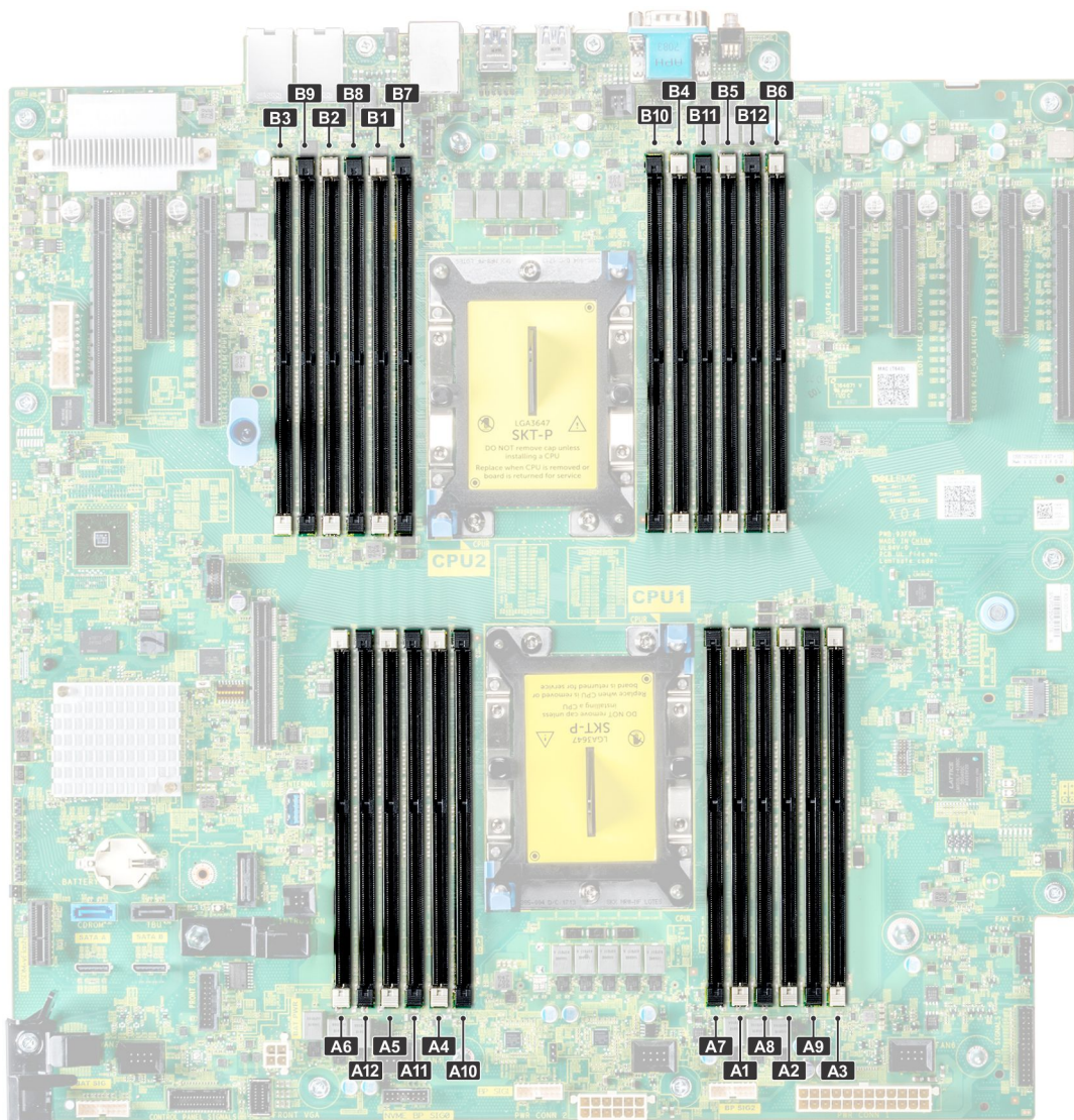
Figure 67. Vue du dessus du système
