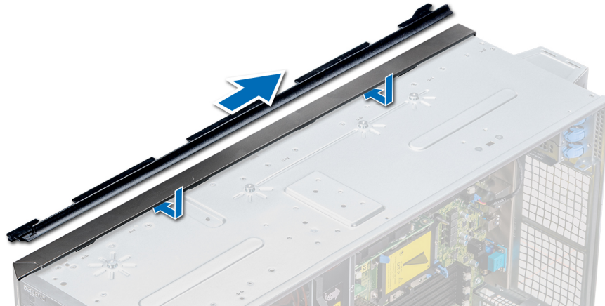
Figure 120. Installez le capot coulissant du rack
