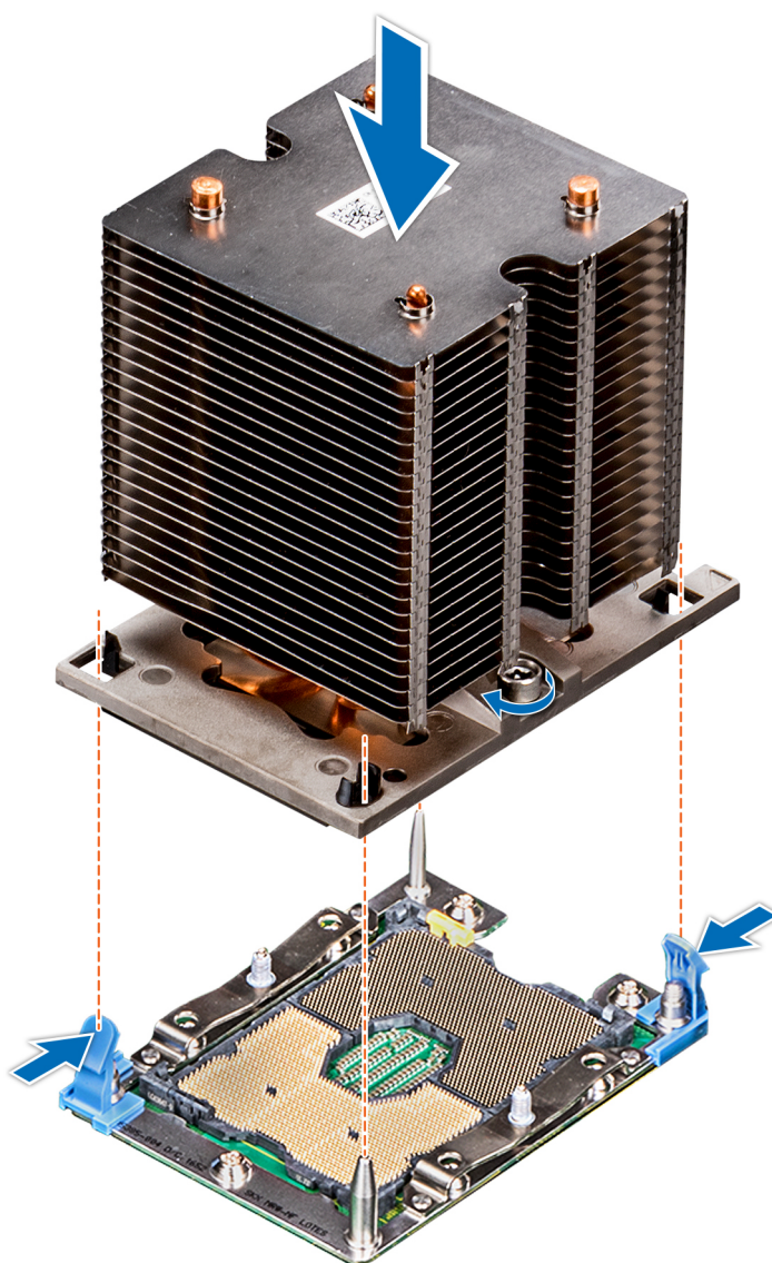
Figure 76. Installation du module processeur et dissipateur de chaleur
