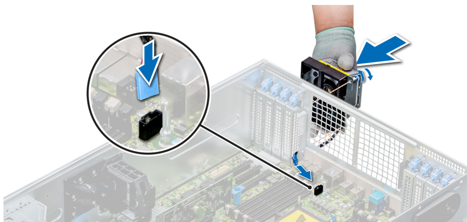
Figure 54. Installation du ventilateur externe droit
