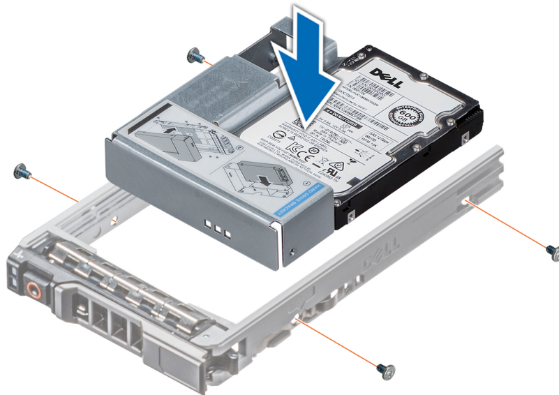
Figure 38. Installation d'un adaptateur de lecteur de 3,5 pouces dans un support de lecteur de 3,5 pouces
