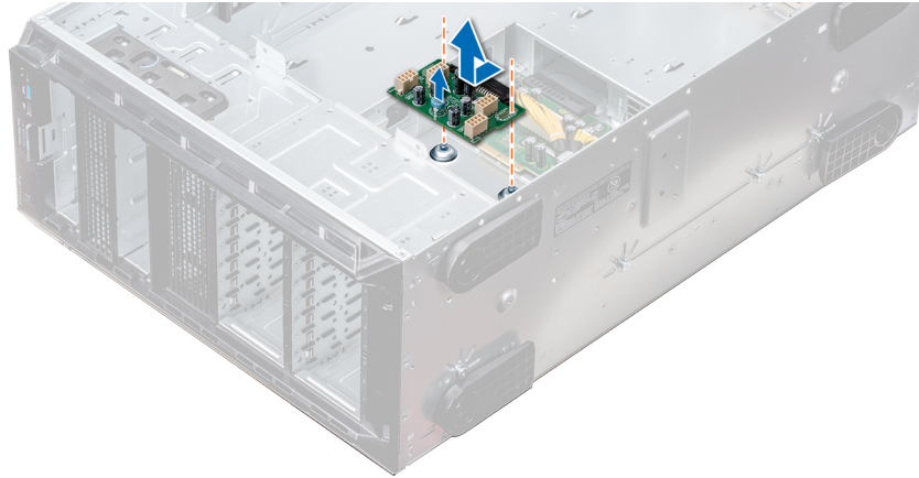
Figure 116. Retrait de la carte intercalaire d'alimentation (PIB) GPU
