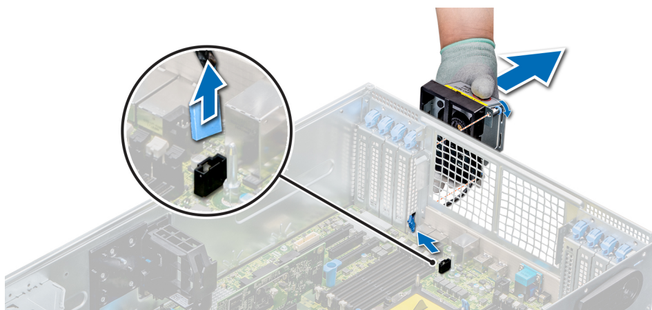
Figure 23. Retrait du ventilateur externe gauche
