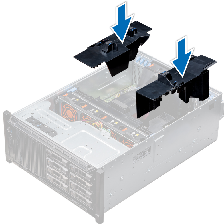
Figure 48. Installation des carénages d'aération optionnels du GPU
