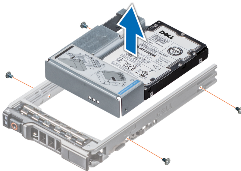
Figure 37. Retrait d'un adaptateur de lecteur de 3,5 pouces d'un support de lecteur de 3,5 pouces
