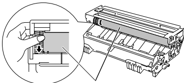
Lichtgevoelige drum
