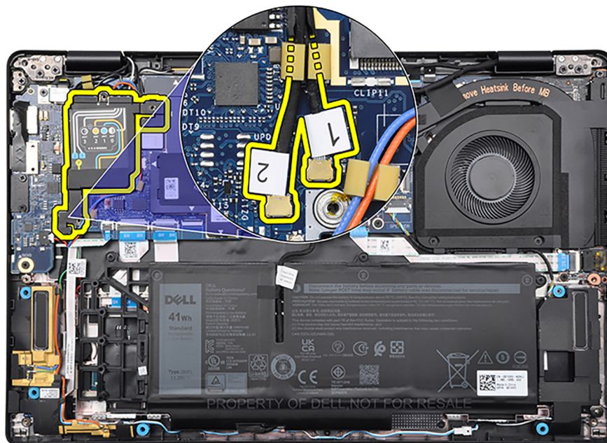
Afbeelding 5. 5G WWAN-configuratie
