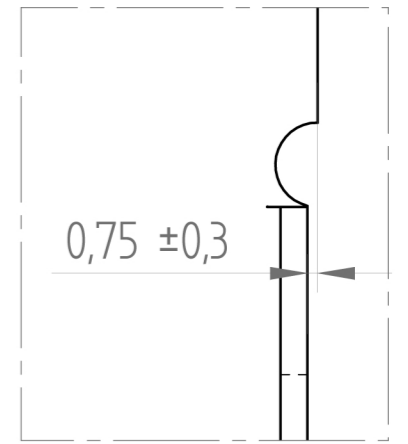
DETT. C
