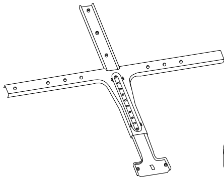
Držák pro upevnění na obrazovku
