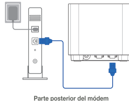
Parte posterior del módem
