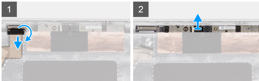
Ilustración 2. Extracción del módulo de la cámara infrarroja
