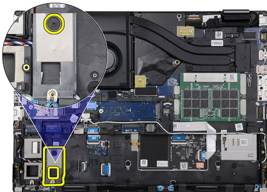
Figure 1. Retirez le cadre SSD du logement 4 de disque SSD.
