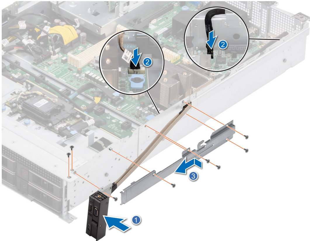
Ilustración 110. Instalación del panel de control derecho
