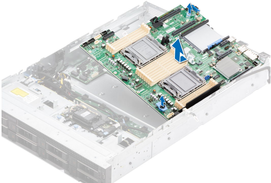
Ilustración 104. Extracción de la placa base
