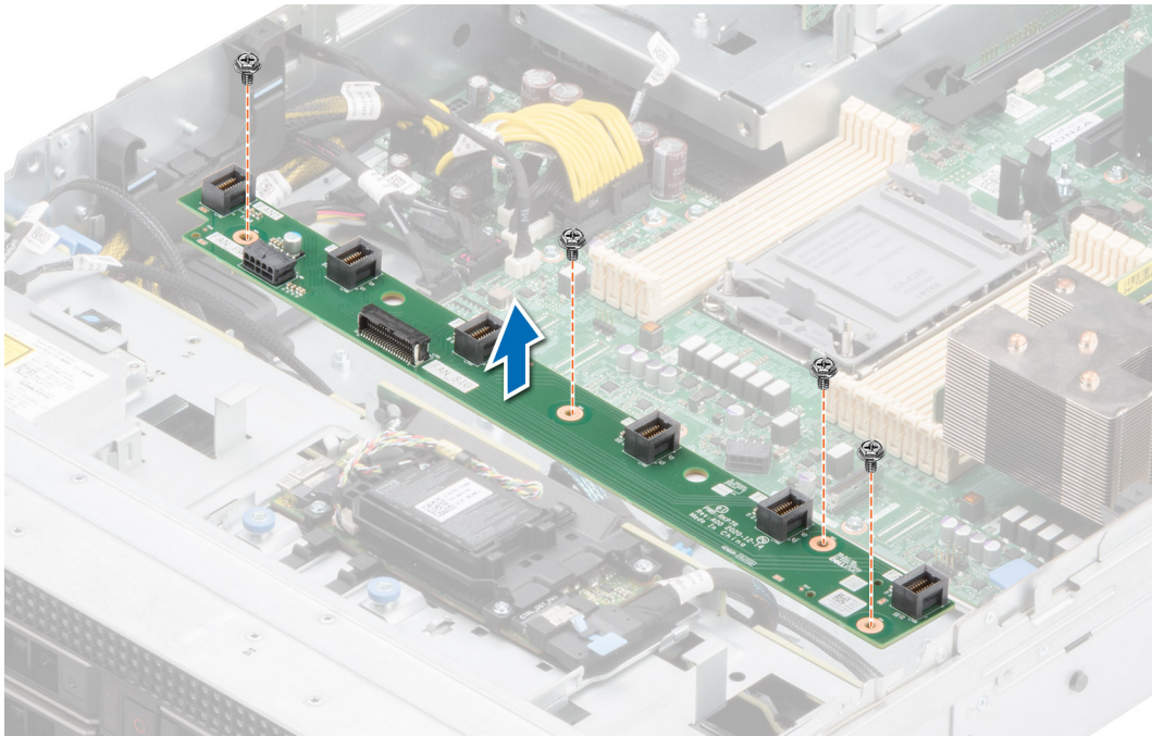
Ilustración 102. Extracción de la canastilla para el ventilador
