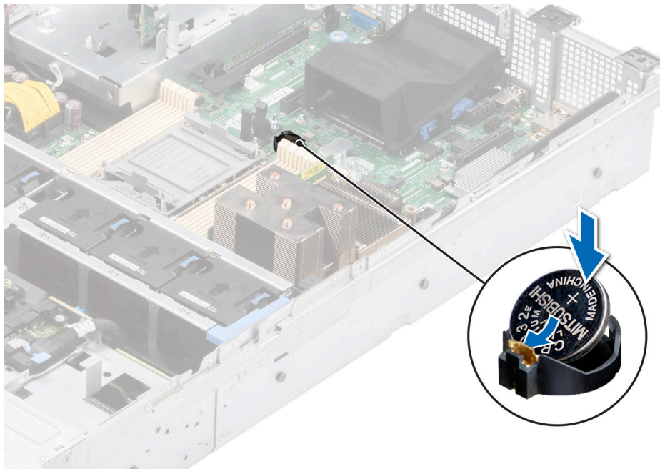
Ilustración 91. Instalación de la batería del sistema
