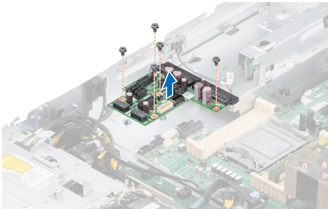
Ilustración 100. Extracción de la placa mediadora de alimentación
