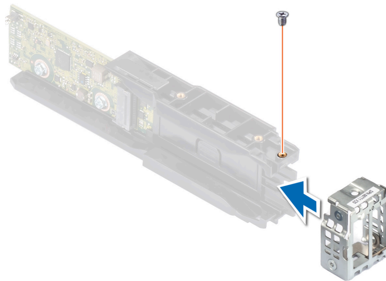
Ilustración 79. Instalación de la cubierta de Boot Optimized Storage Subsystem
