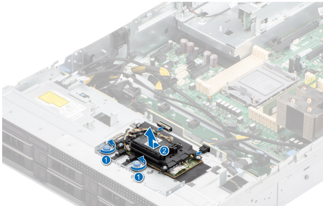
Ilustración 84. Extracción del módulo de PERC frontal de montaje frontal
