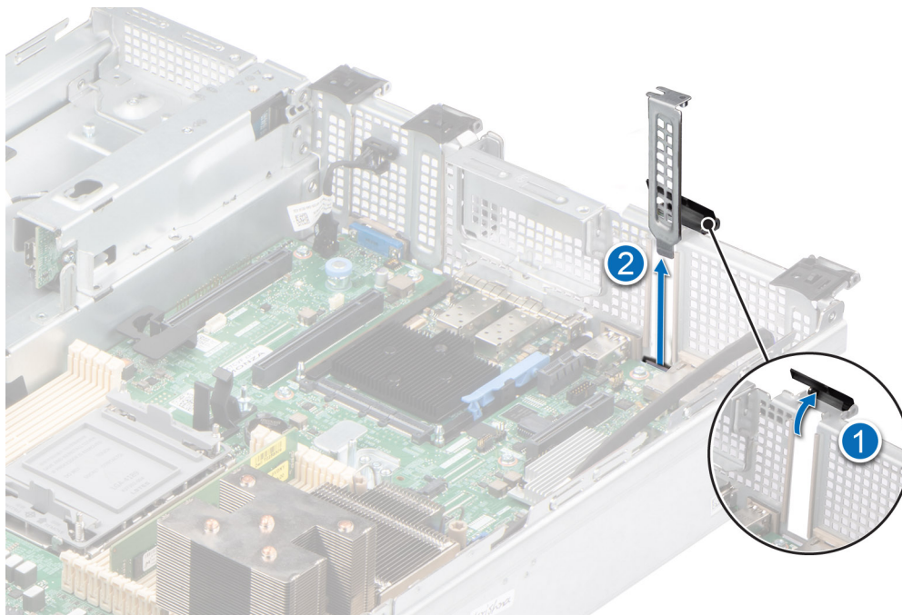
Ilustración 70. Extracción del soporte de relleno
