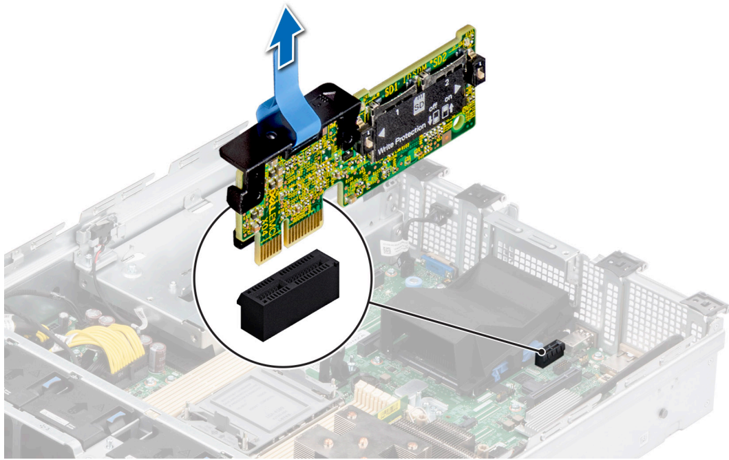
Ilustración 72. Extracción del módulo IDSDM
