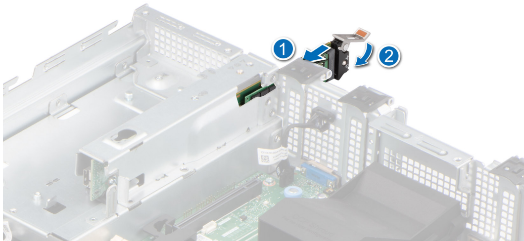
Ilustración 83. Instalación del portaunidades de tarjeta de Boot Optimized Storage Subsystem S2
