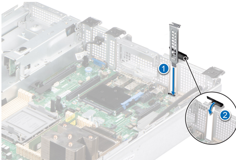
Ilustración 69. Instalación del soporte de relleno
