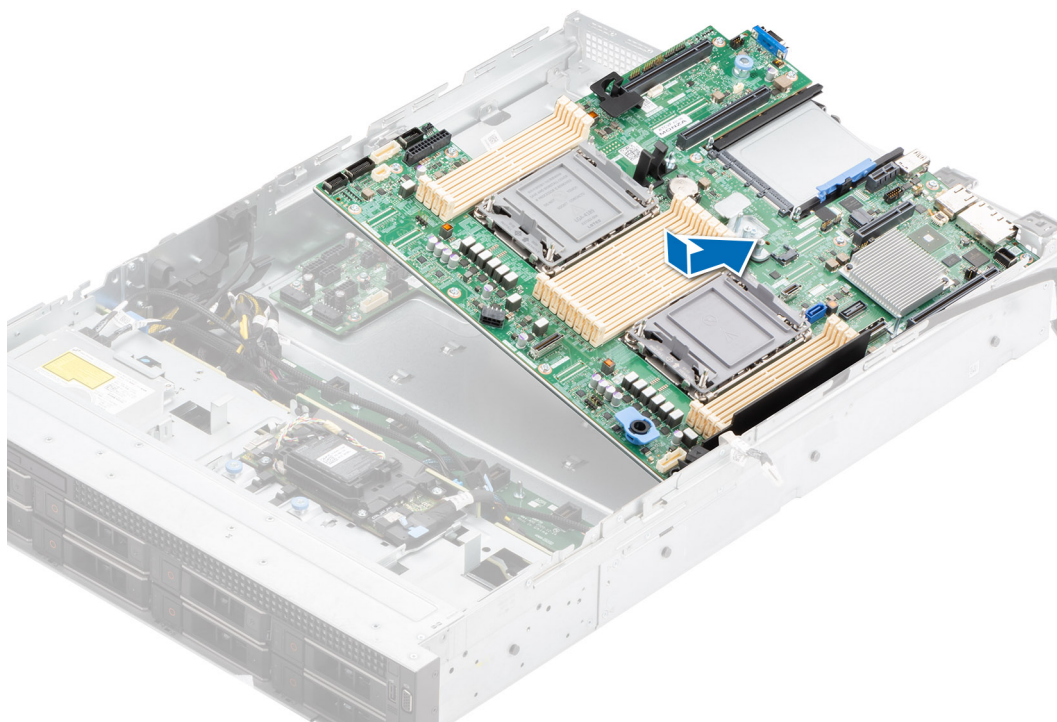
Ilustración 105. Instalación de la placa base
