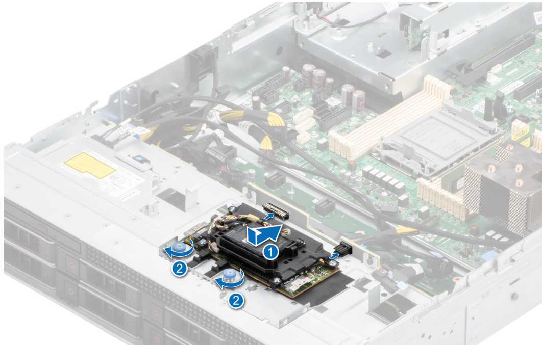
Ilustración 85. Instalación del módulo de PERC frontal de montaje frontal
