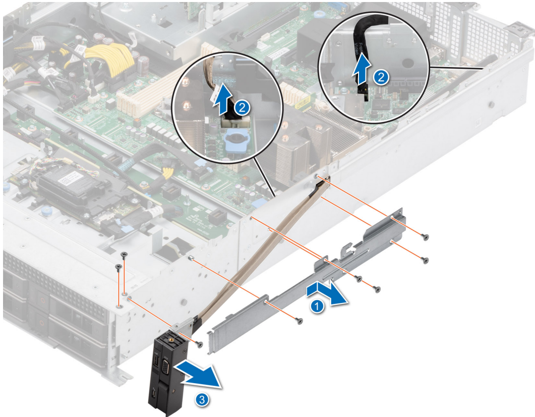
Ilustración 109. Extracción del panel de control derecho
