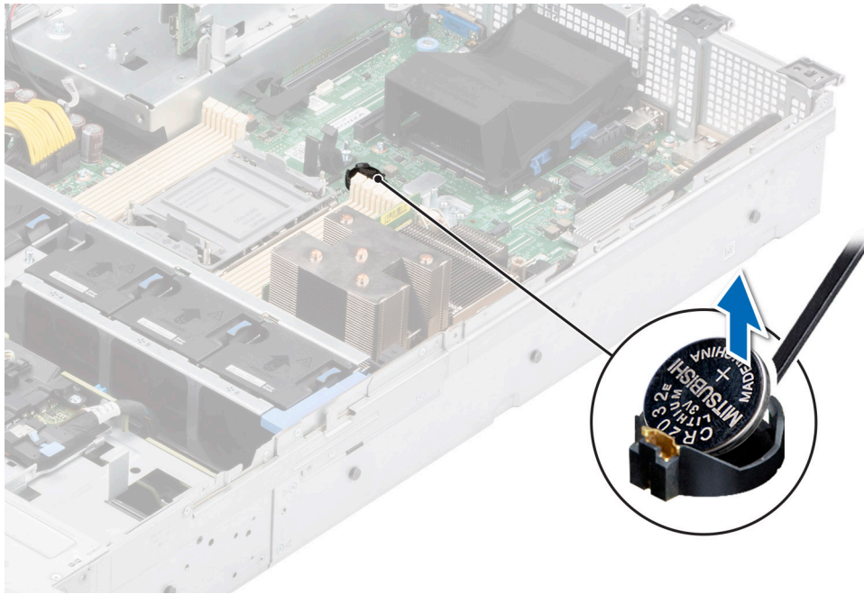
Ilustración 90. Extracción de la batería del sistema
