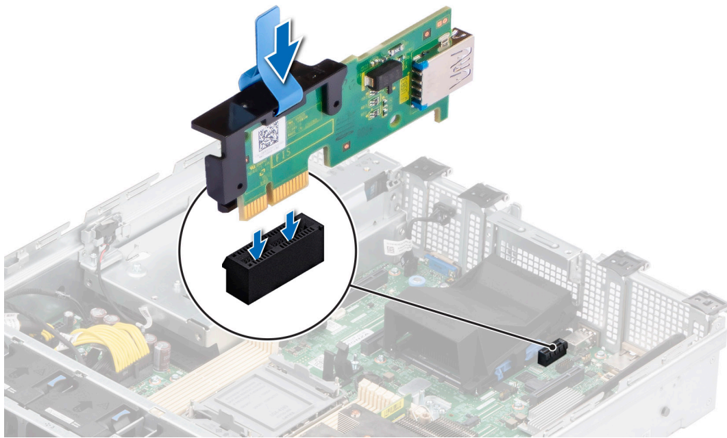
Ilustración 93. Instalación de la tarjeta USB interna
