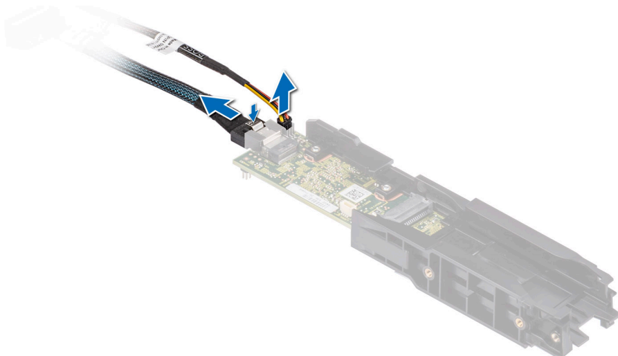
Ilustración 77. Extracción del cable de alimentación de BOSS y del cable de señal de BOSS
