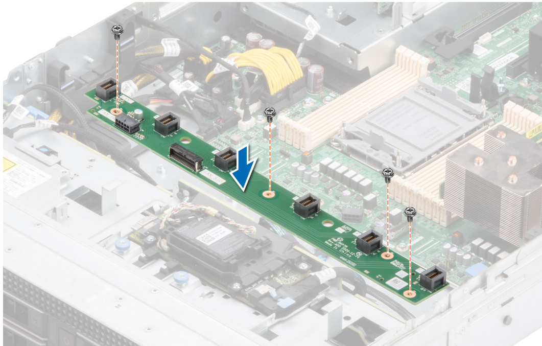
Ilustración 103. Instalación de la placa de la canastilla para el ventilador
