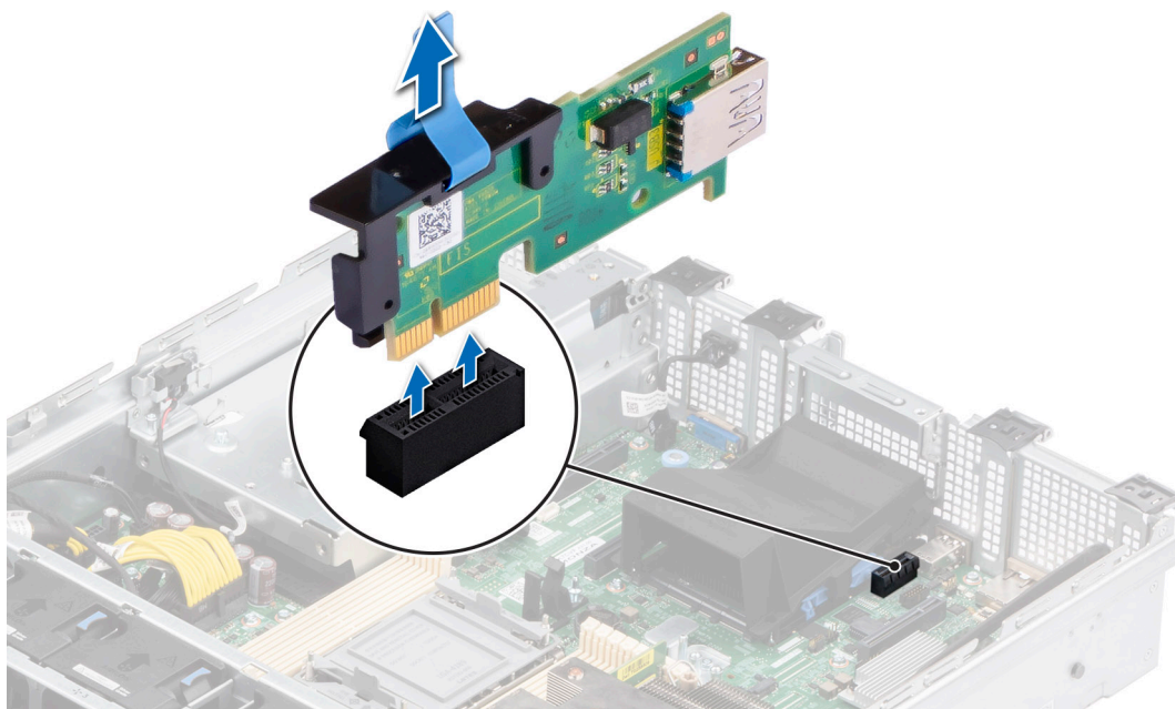
Ilustración 92. Extracción de la tarjeta USB interna
