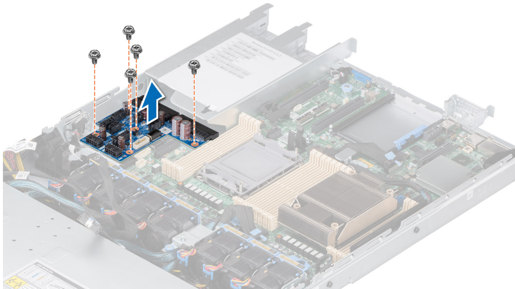
Abbildung 1. Stromzwischenplatte entfernen
