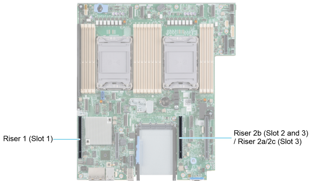
Abbildung 2. Erweiterungskarten-Steckplätze
