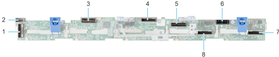
Figure 34. Fond de panier 10 disques NMVe de 2,5 pouces
