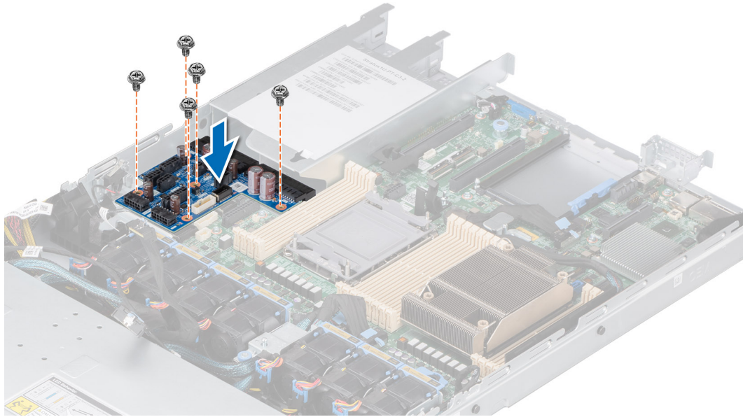
Figure 124. Installation de la carte intercalaire d'alimentation
