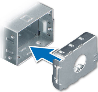
Figure 120. Installation du cache de bloc d'alimentation
