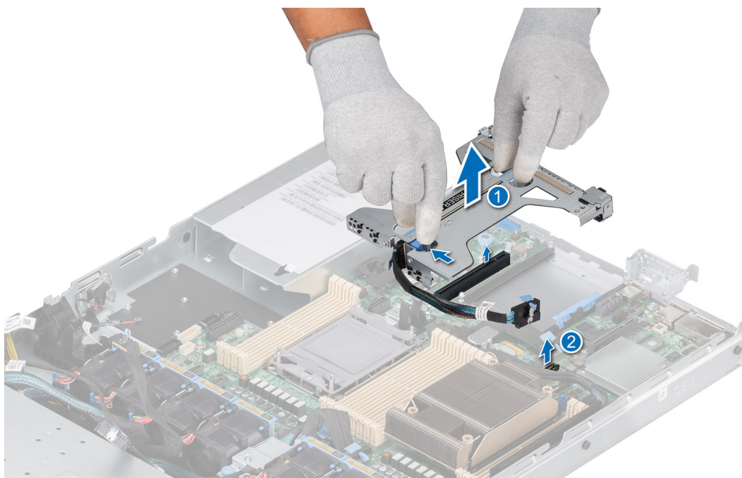
Figure 71. Retrait de la carte de montage 2b avec module SNAPI
