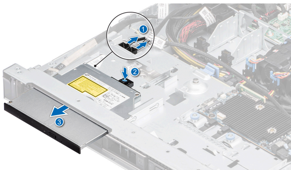
Figure 30. Retrait du lecteur optique
