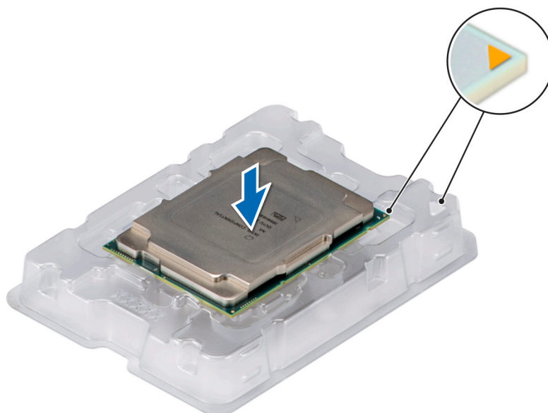
Figure 55. Alignement des repères de la broche 1 du processeur sur le plateau
