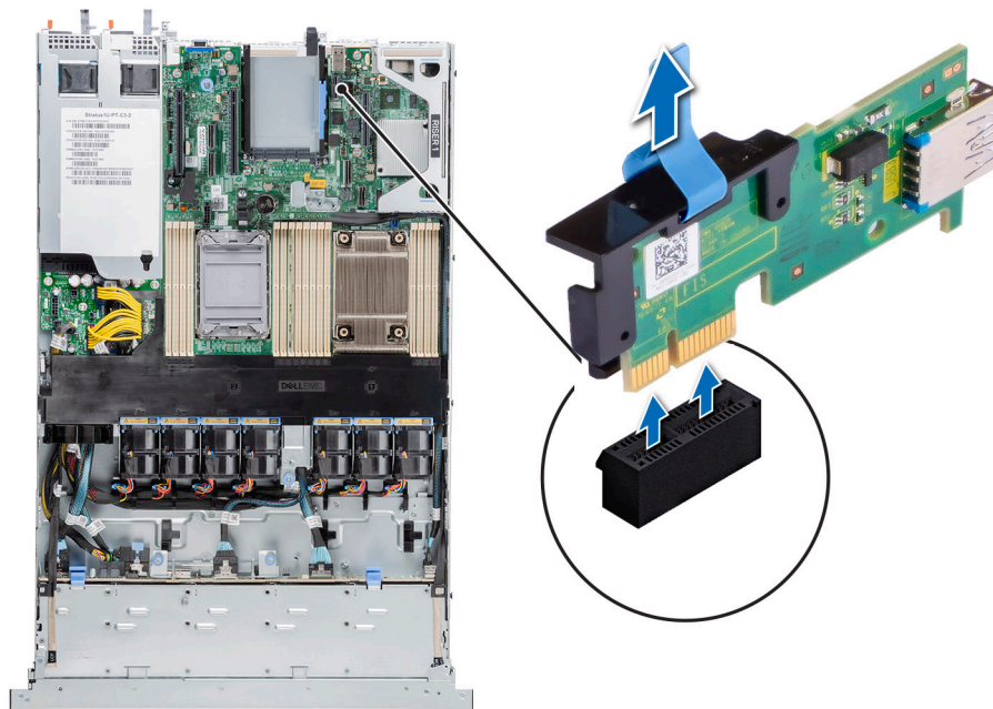
Figure 115. Retrait de la carte USB interne
