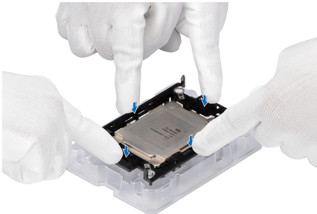
Ilustración 58. Presione el portaunidades en los cuatro lados
