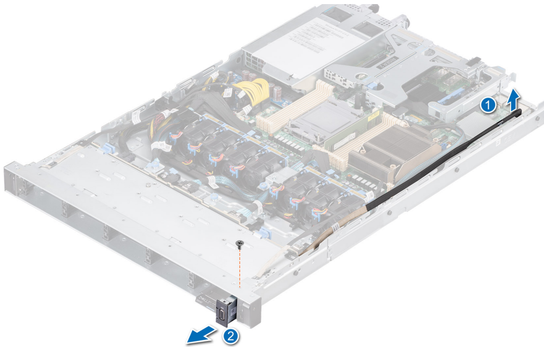
Ilustración 117. Extracción del módulo VGA
