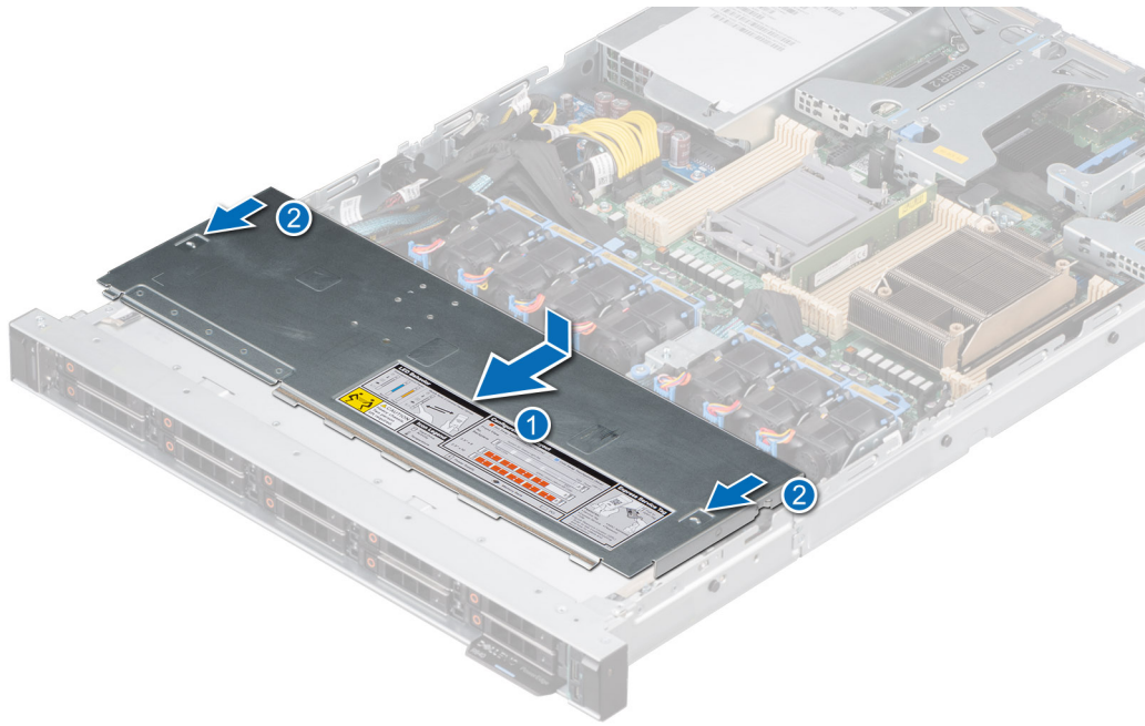
Ilustración 17. Instalación de la cubierta del backplane de la unidad
