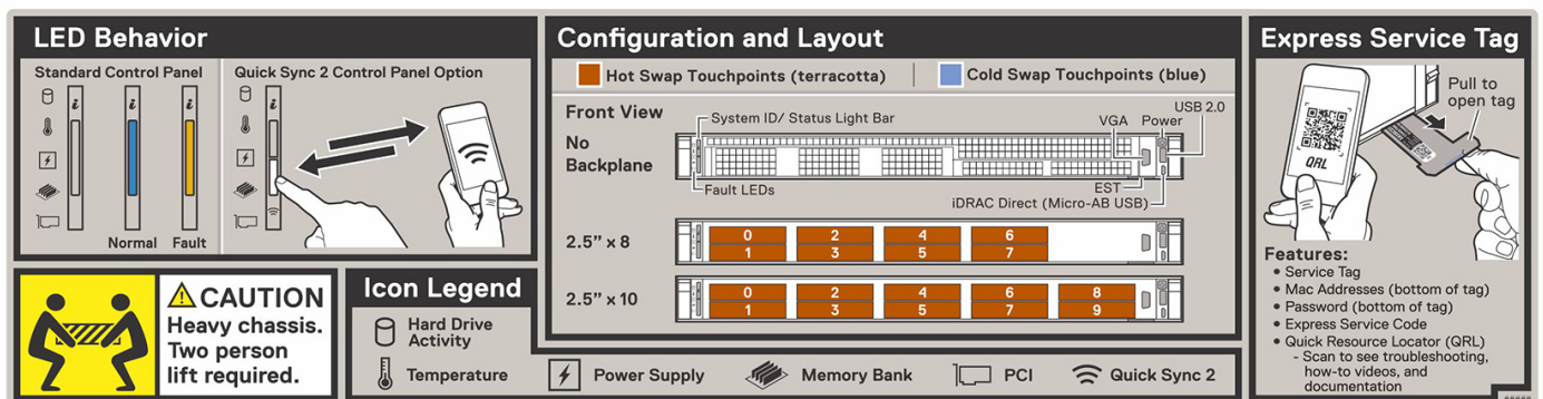
Ilustración 9. Comportamiento del LED, configuración y diseño, etiqueta de servicio exprés
