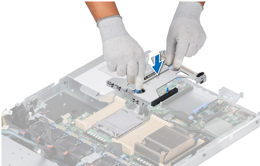
Ilustración 74. Instalación del soporte vertical 2a
