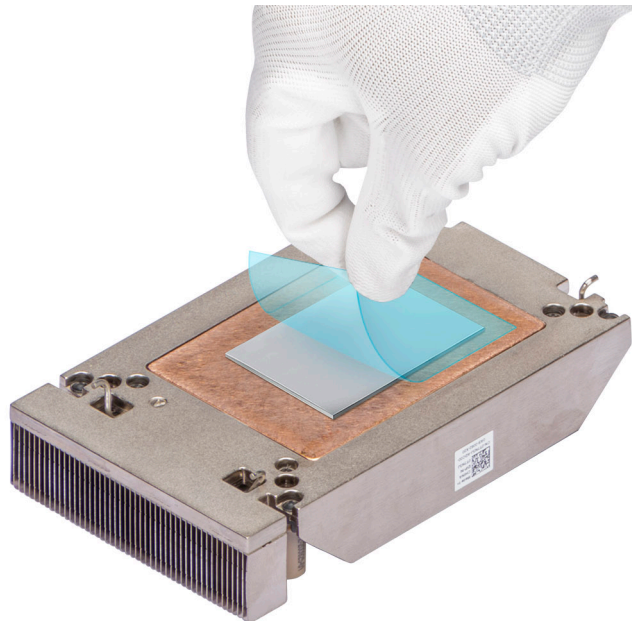
Ilustración 60. Extraiga la película de protección del material de interfaz térmica (TIM)
