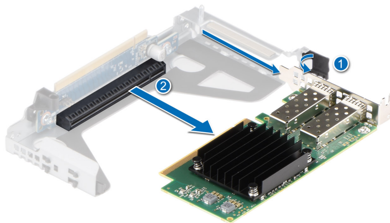
Ilustración 77. Extracción de una tarjeta de expansión del soporte vertical 1
