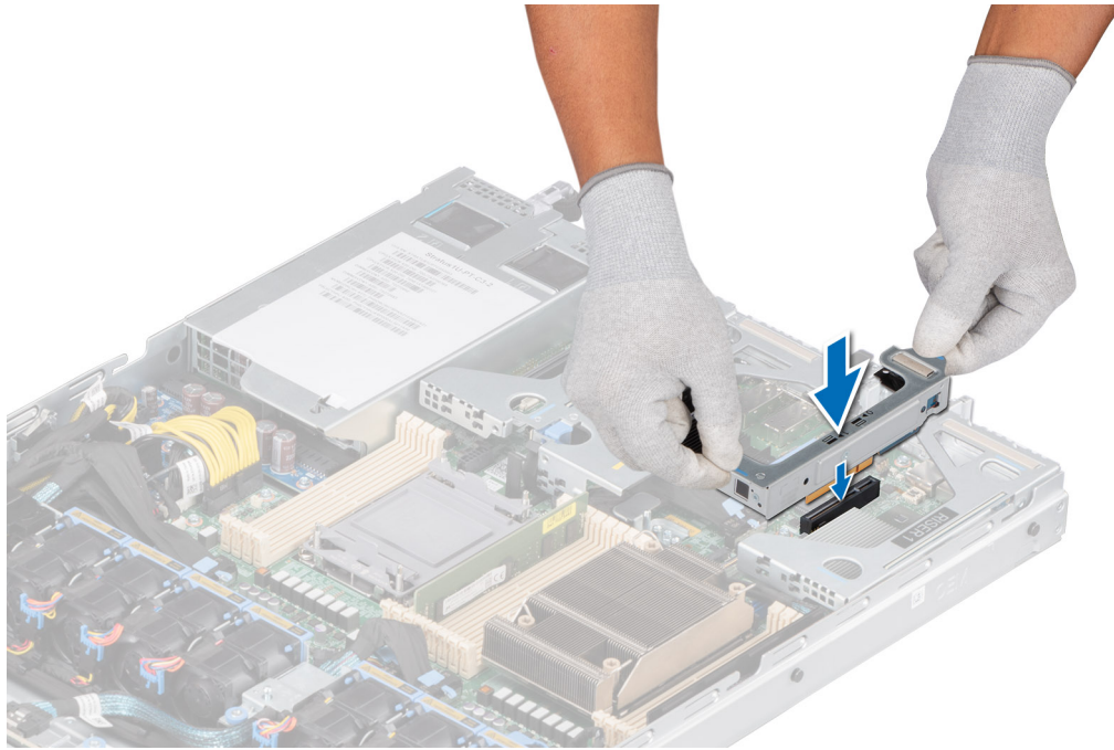
Ilustración 102. Instalación del soporte vertical BOSS M.2
