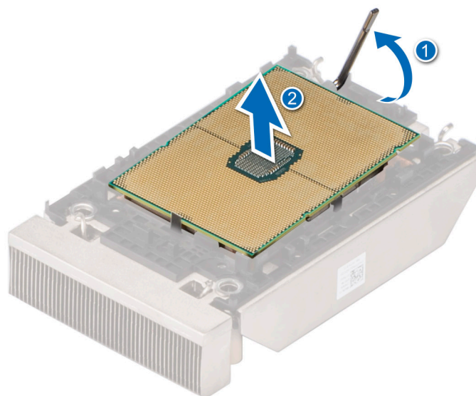
Ilustración 54. Levante la palanca de rotura del TIM
