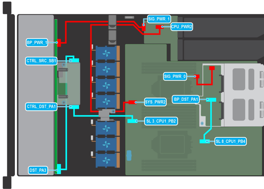
Ilustración 46. Colocación de cables: backplane de SAS/SATA de la unidad de 10 x 2,5 pulgadas con canastilla para unidades posteriores con backplane de SAS, soporte vertical de mariposa
