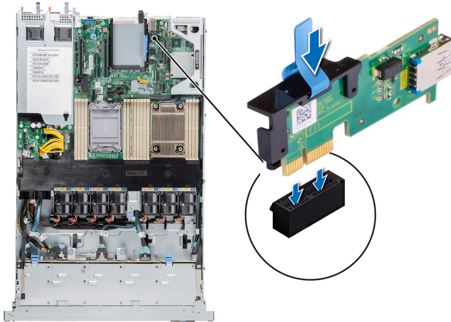
Ilustración 116. Instalación de la tarjeta USB interna
