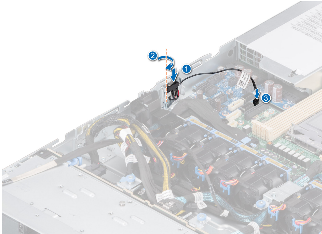
Ilustración 23. Instalación del interruptor de intrusiones
