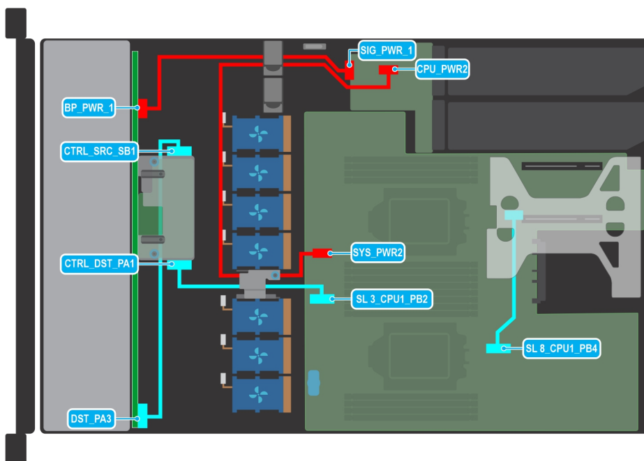
Ilustración 45. Colocación de los cables: backplane de SAS/SATA de unidad de 10 x 2,5 pulgadas con soporte vertical de mariposa
