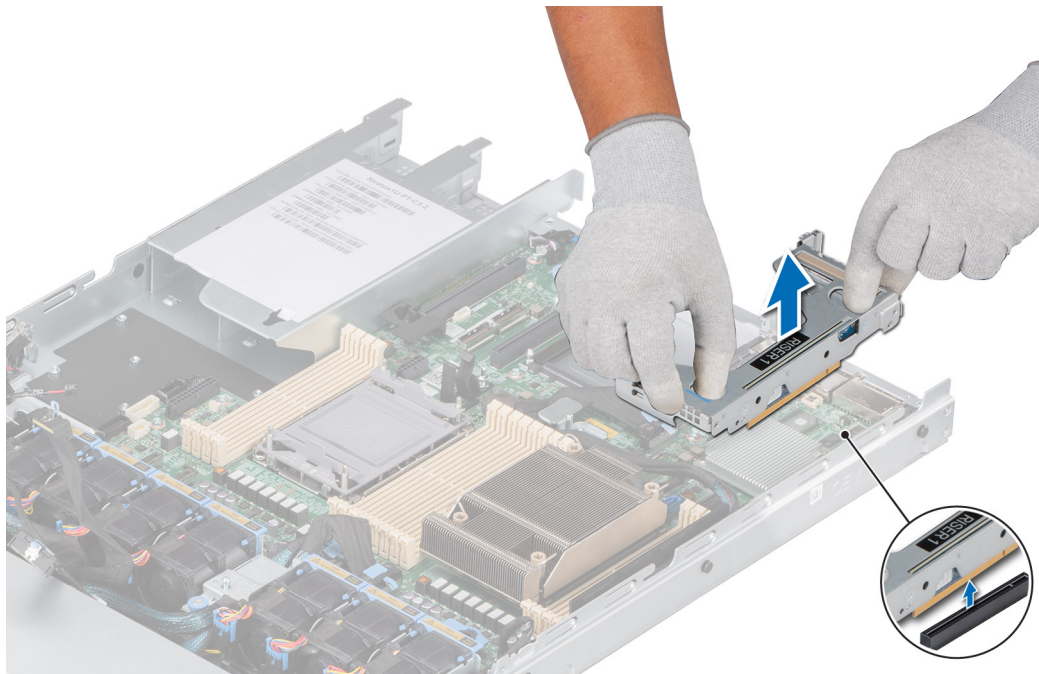
Ilustración 69. Extracción de la Tarjeta vertical 1
