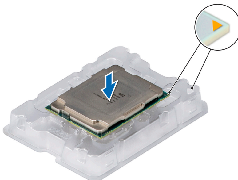
Ilustración 55. Alineación de las marcas de la pata 1 del procesador con la bandeja
