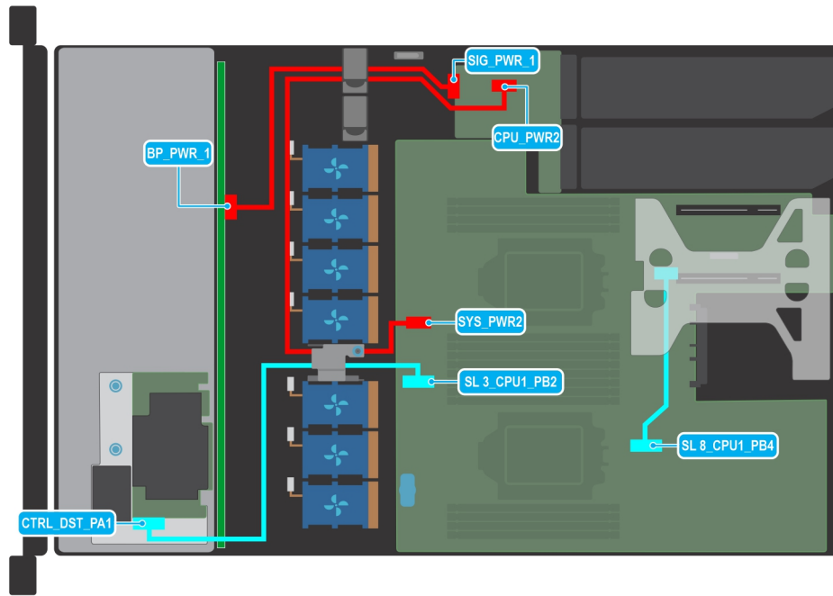
Ilustración 47. Colocación de los cables: backplane de SAS/SATA de unidad de 8 x 2,5 pulgadas con soporte vertical SNAP!
