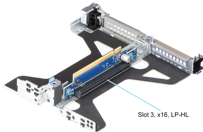
Ilustración 67. Soporte vertical 2b (SNAPI)
