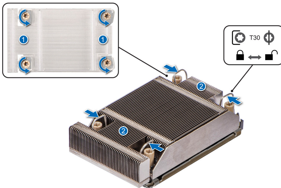
Ilustración 52. Aflojar las tuercas y establecer los cables antiinclinación en la posición de desbloqueo
