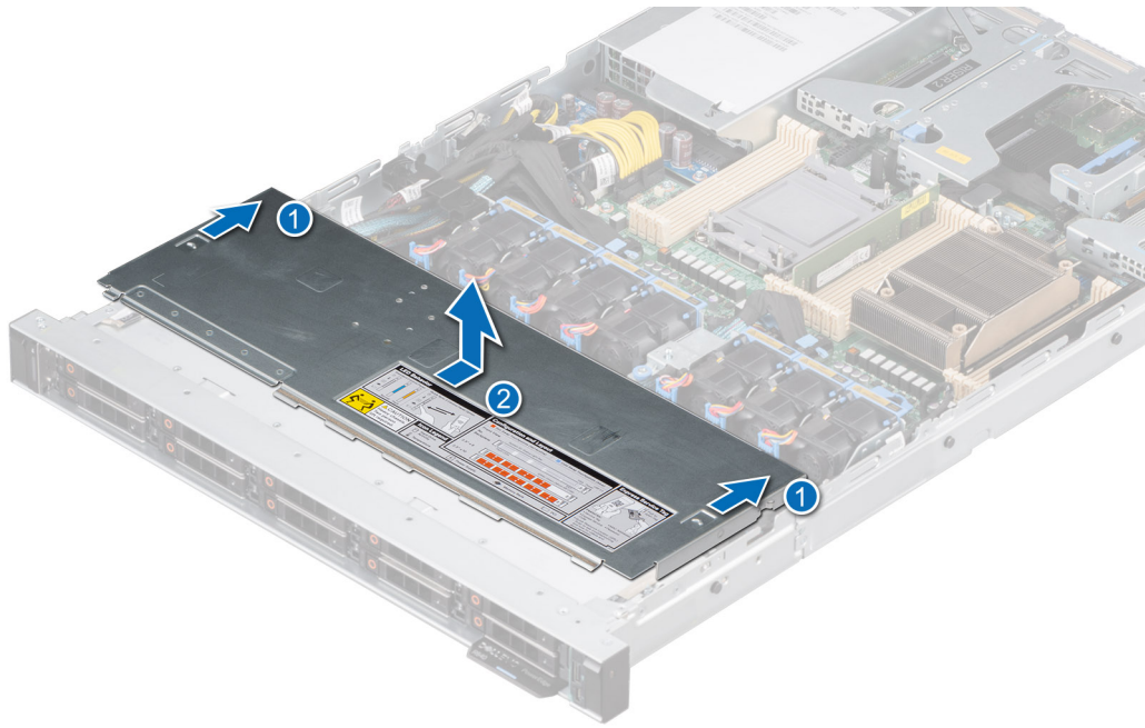
Ilustración 16. Extracción de la cubierta del backplane de la unidad
