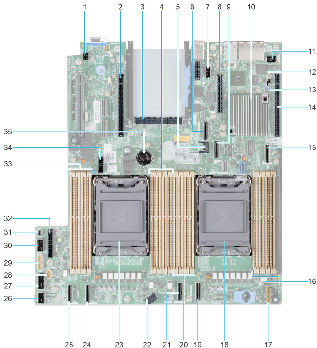
Ilustración 132. Puentes y conectores de la tarjeta madre
