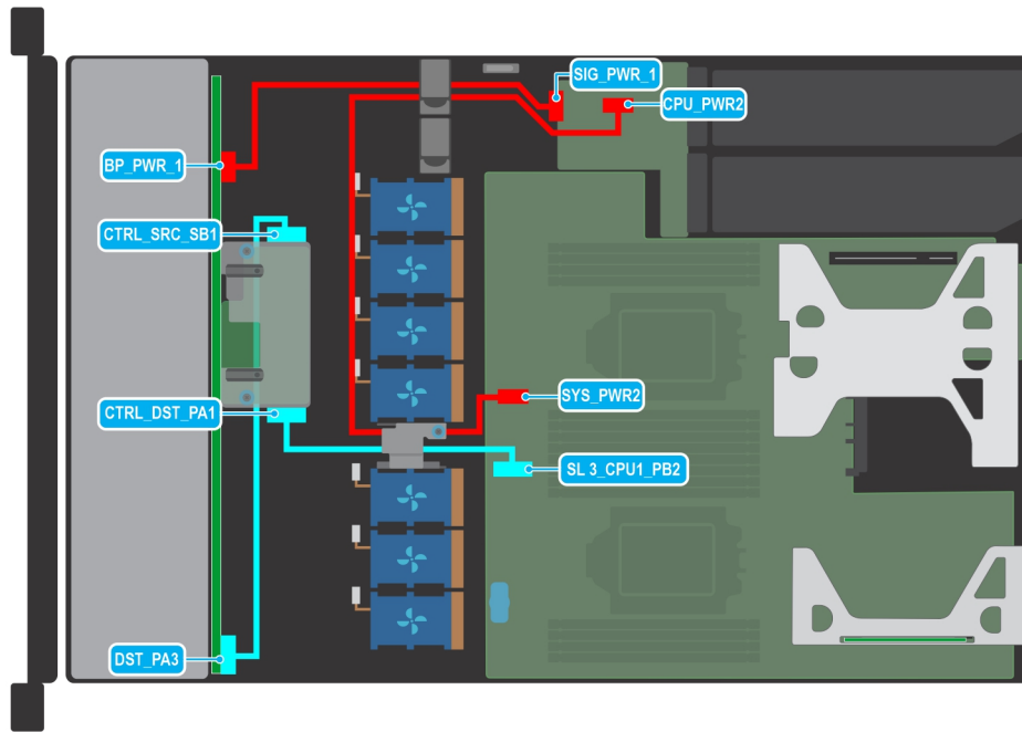
Ilustración 39. Enrutamiento de cables: backplane de unidad de 10 x 2,5 pulgadas con soporte vertical de mariposa y fPERC
