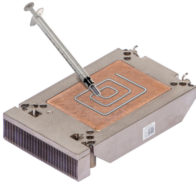
Ilustración 59. Aplicación de la grasa térmica
