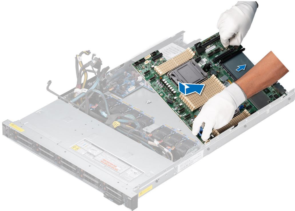
Ilustración 126. Instalación de la tarjeta madre
