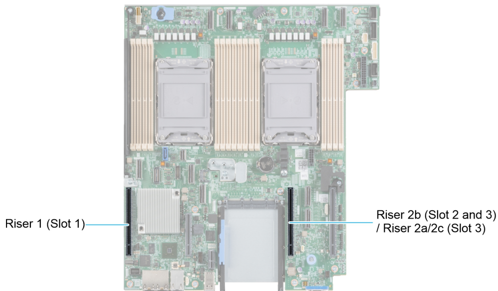
Ilustración 64. Conectores de la ranura de tarjetas de expansión
