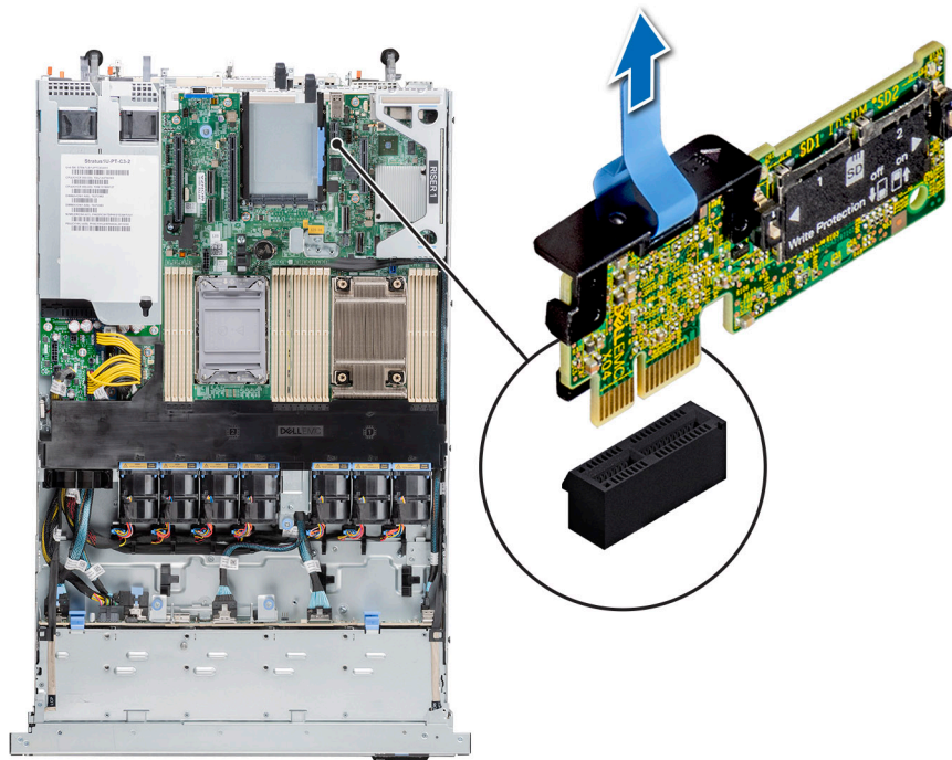
Ilustración 107. Extracción del módulo IDSDM
