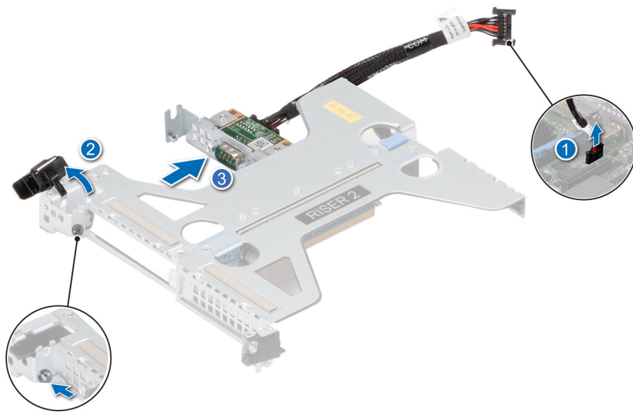
Ilustración 95. Extracción del puerto serial de COM
