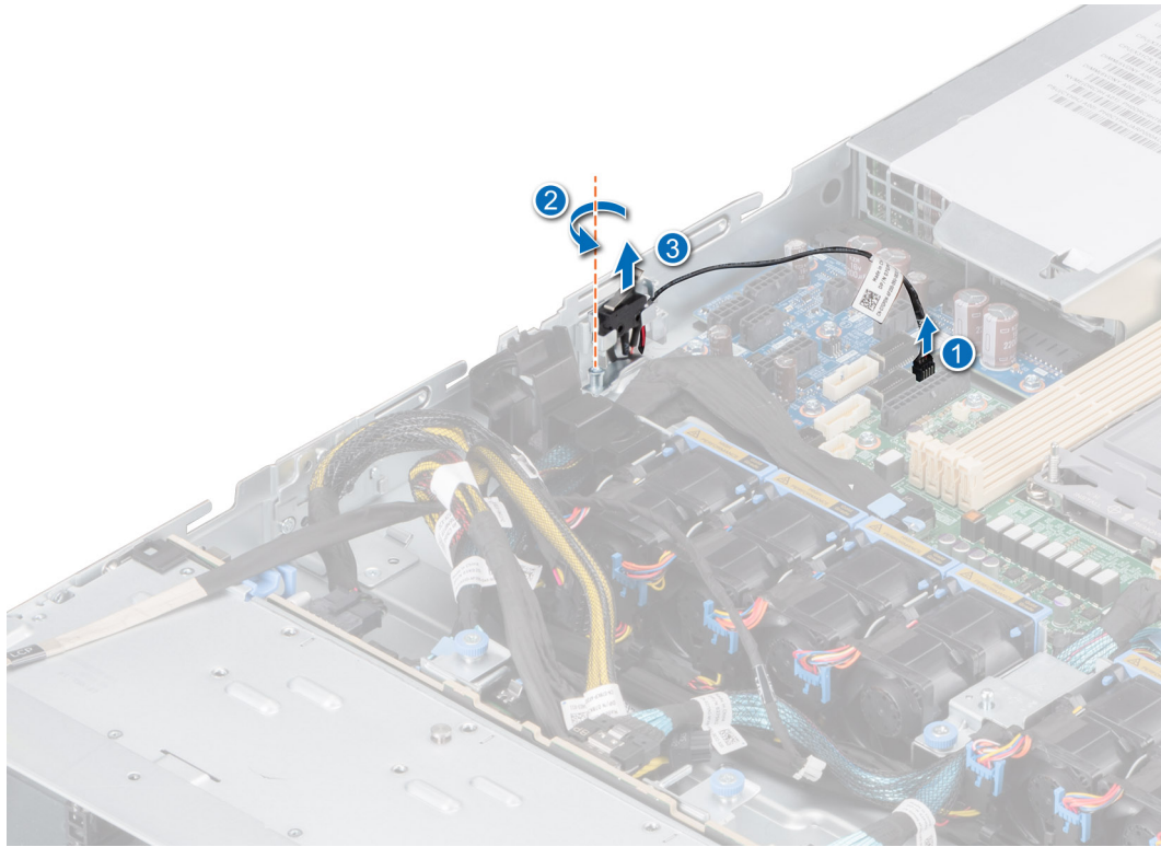
Ilustración 22. Extracción del módulo del interruptor de intrusiones
