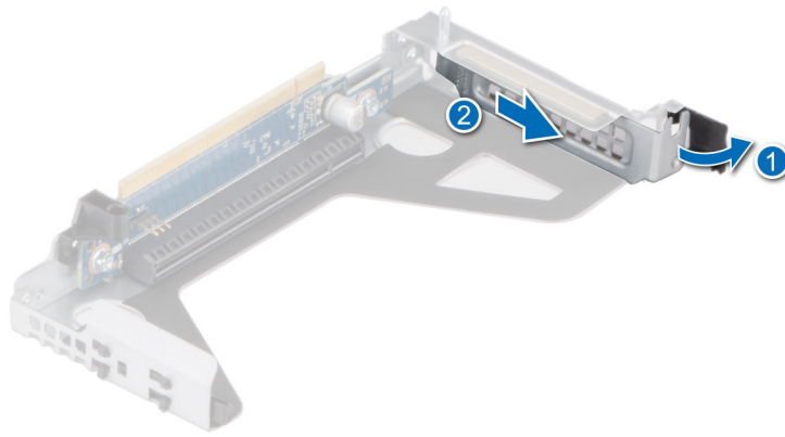
Ilustración 85. Extracción de un soporte de relleno del soporte vertical 1
