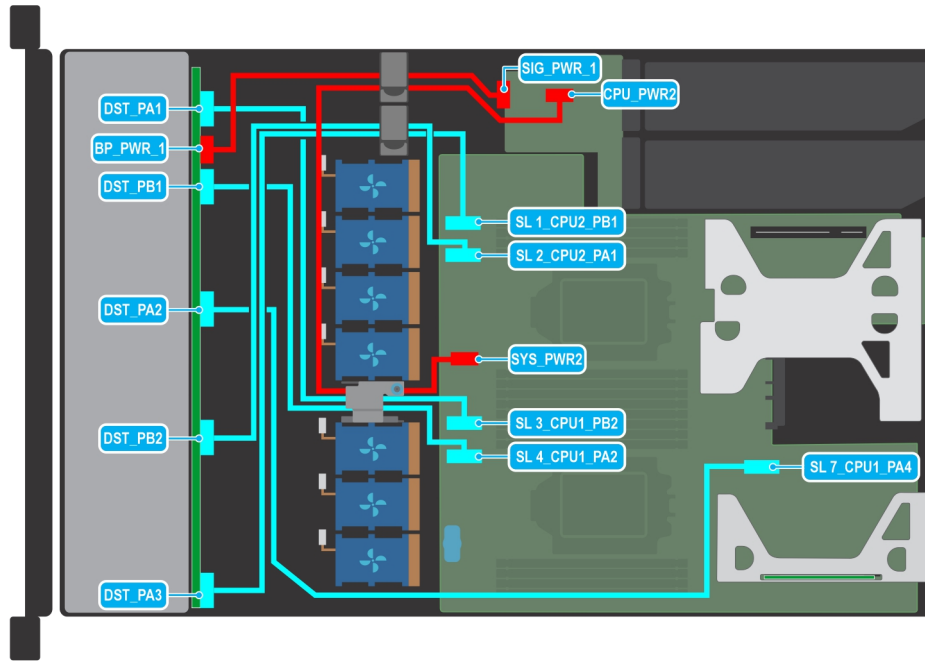
Ilustración 38. Enrutamiento de cables: backplane de unidad de 10 x 2,5 pulgadas a la controladora integrada (6:4 NVMe)
