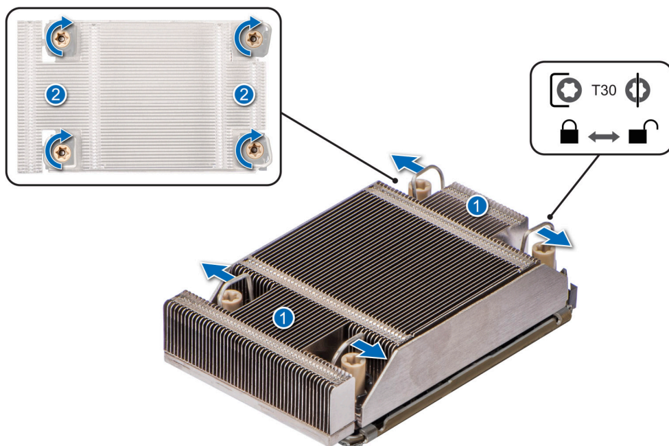
Ilustración 63. Establezca los cables de antiinclinación a la posición de bloqueo y ajuste las tuercas cautivas.
