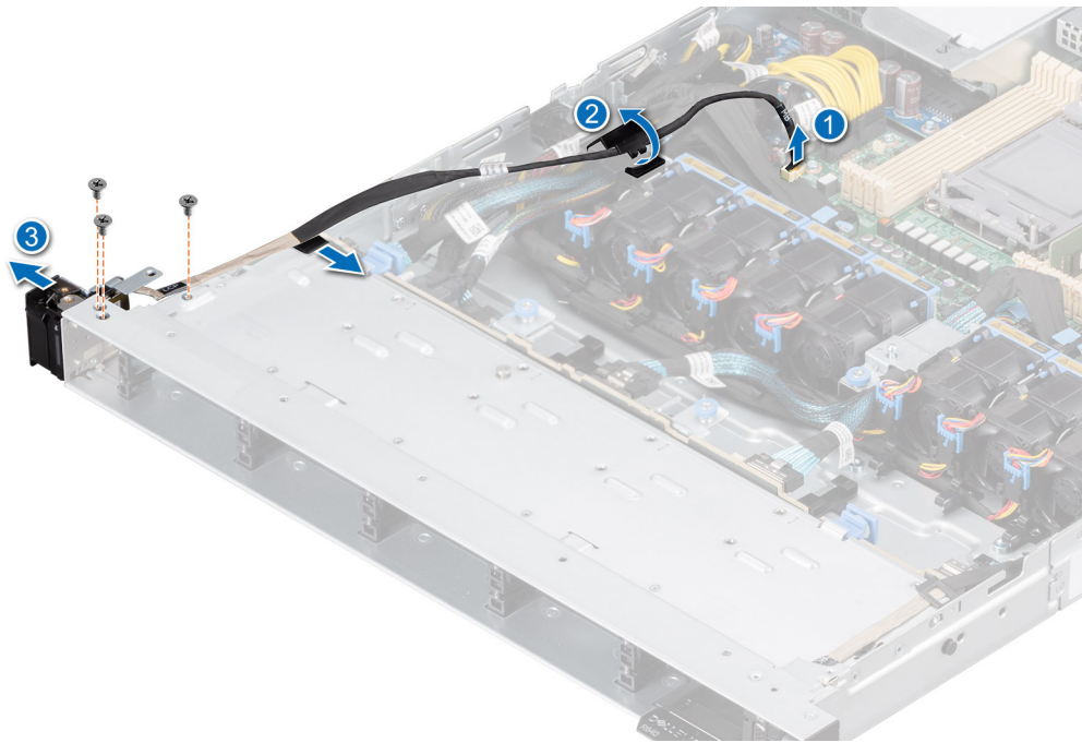
Ilustración 128. Extracción del panel de control izquierdo
