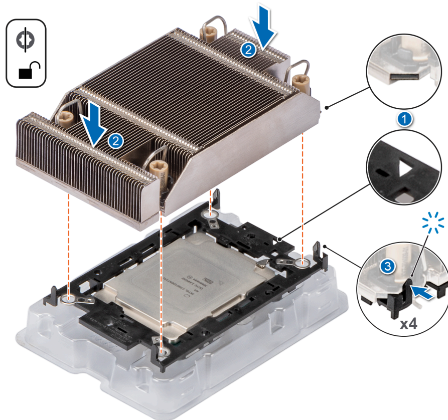
Ilustración 61. Instalación del disipador de calor en el procesador.
