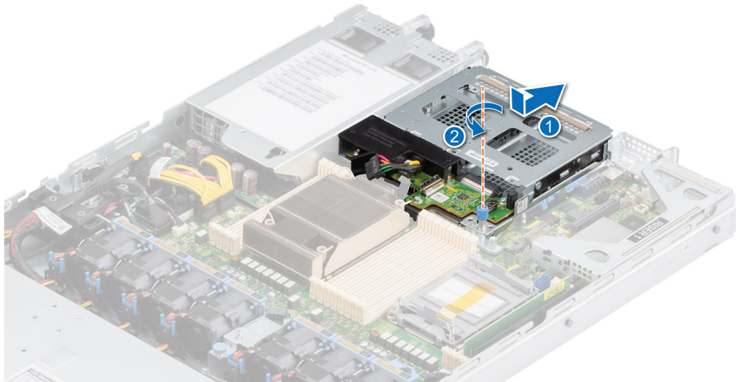
Ilustración 94. Instalación de la canastilla para unidades posteriores de 2,5 pulgadas
