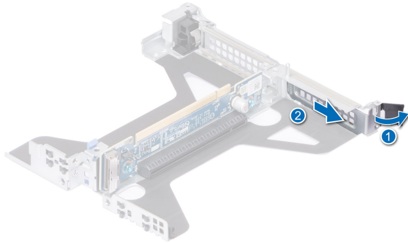
Ilustración 87. Extracción del soporte de relleno del soporte vertical 2b (SNAPI)
