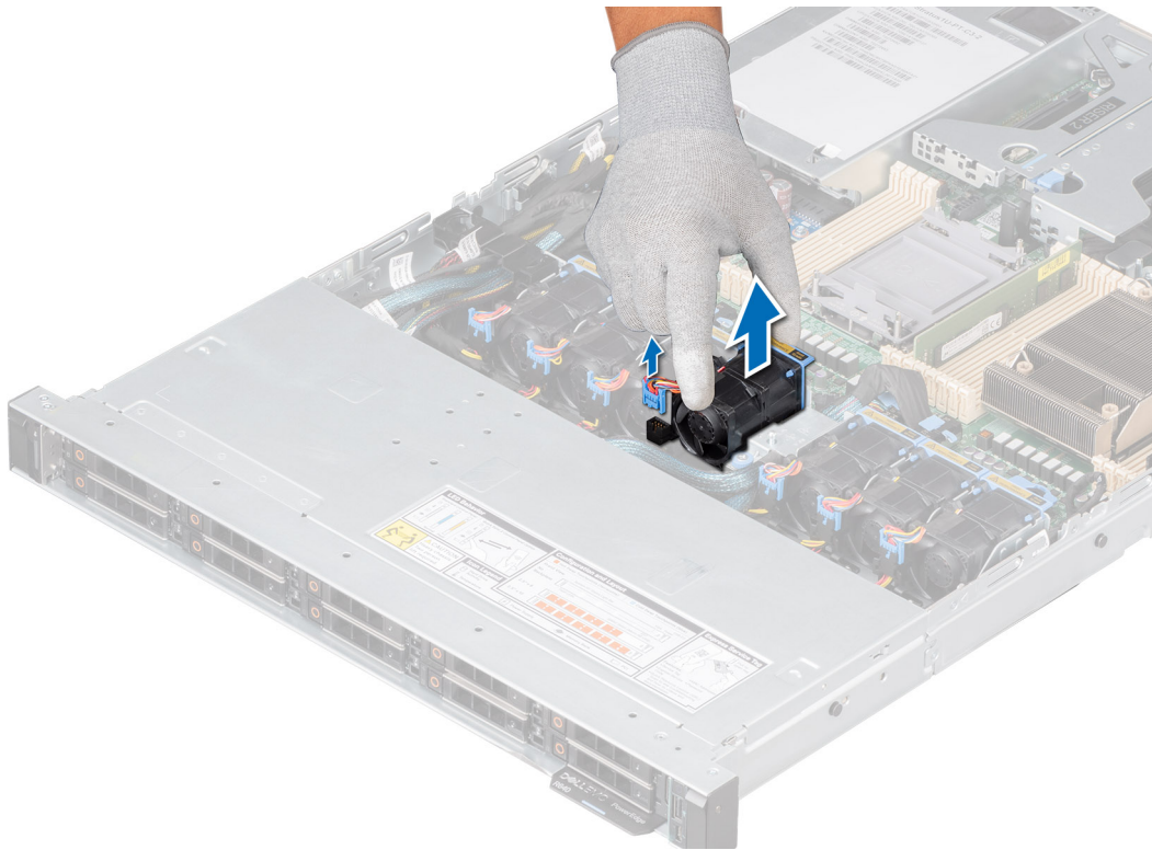
Ilustración 20. Extracción de un ventilador de refrigeración
