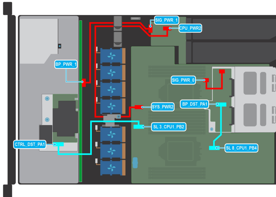
Ilustración 43. Enrutamiento de cables: backplane de SAS/SATA de unidad de 4 x 3,5 pulgadas con fPERC y canastilla para unidades posteriores con backplane NVMe
