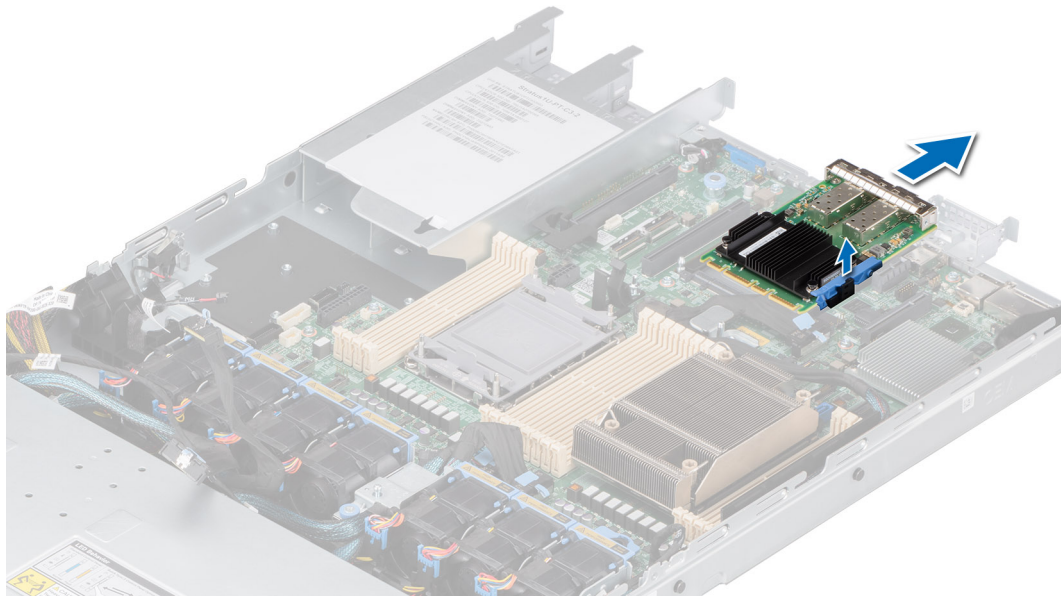
Ilustración 109. Extracción de la tarjeta OCP
