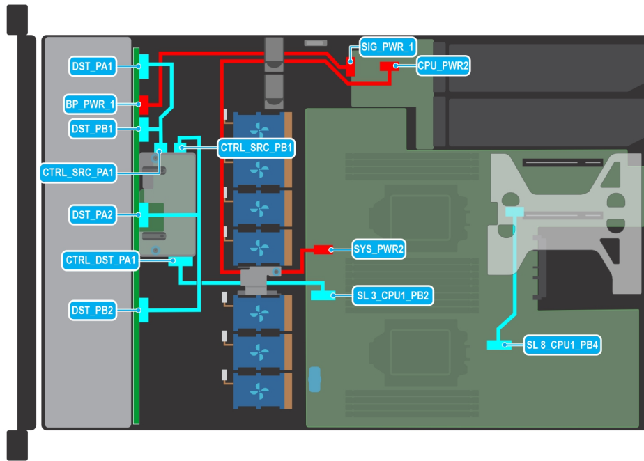
Ilustración 42. Colocación de cables: backplane NVMe de la unidad de 8 x 2,5 pulgadas con fPERC, soporte vertical de mariposa, soporte vertical de BOSS, SNAPI
