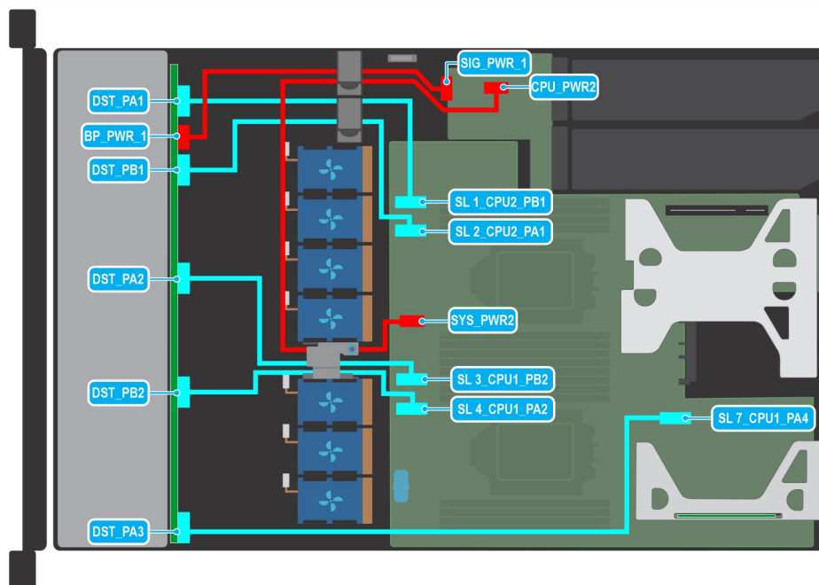
Ilustración 40. Enrutamiento de cables: backplane de unidad de 10 x 2,5 pulgadas en la controladora integrada (4:6 NVMe)
