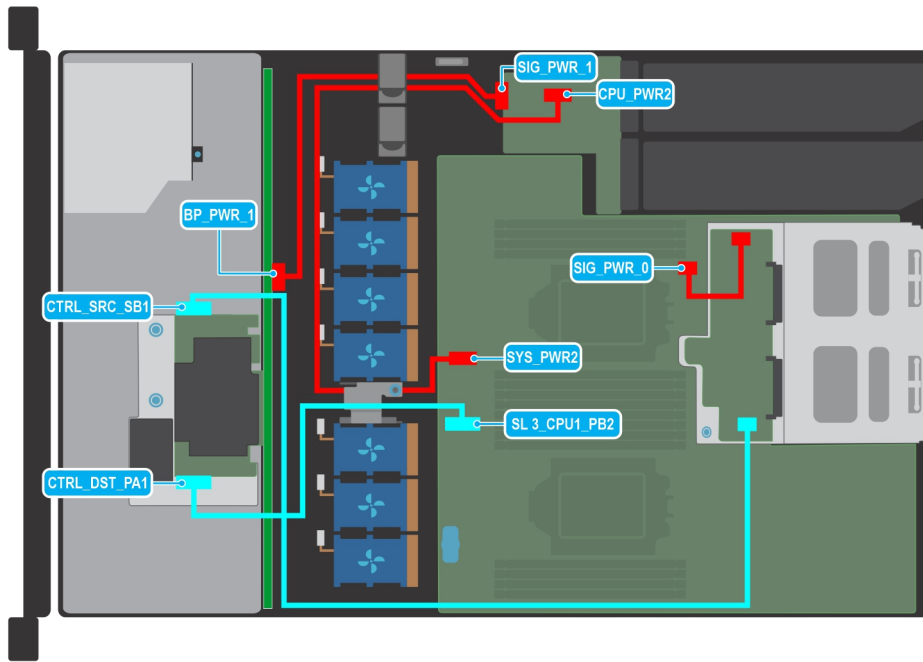
Ilustración 44. Colocación de cables: backplane de SAS/SATA de la unidad de 4 x 3,5 pulgadas con canastilla para unidades posteriores con backplane SAS, soporte vertical de mariposa
