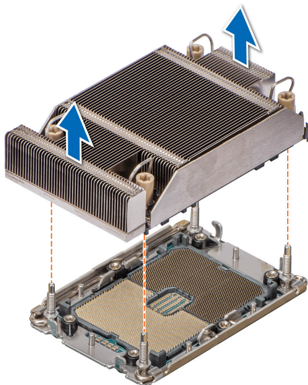
Ilustración 53. Extracción de un módulo del disipador de calor y procesador
