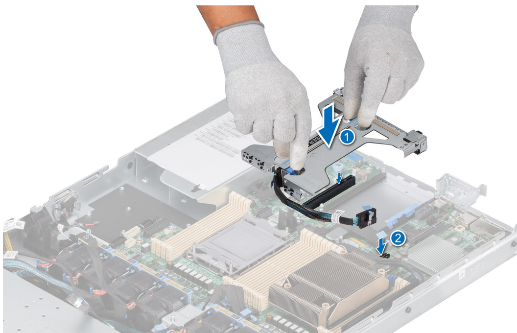
Ilustración 75. Instalación del soporte vertical 2b con el módulo SNAPi
