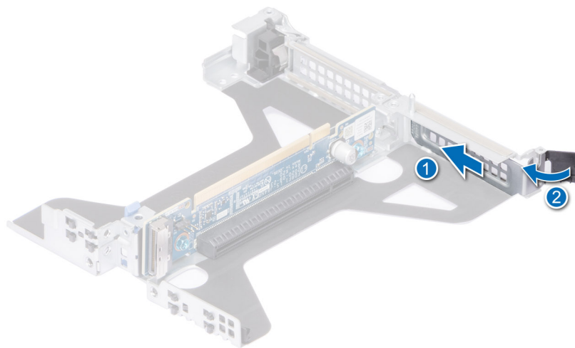
Ilustración 83. Instalación del soporte de relleno en el soporte vertical 2b (SNAPI)
