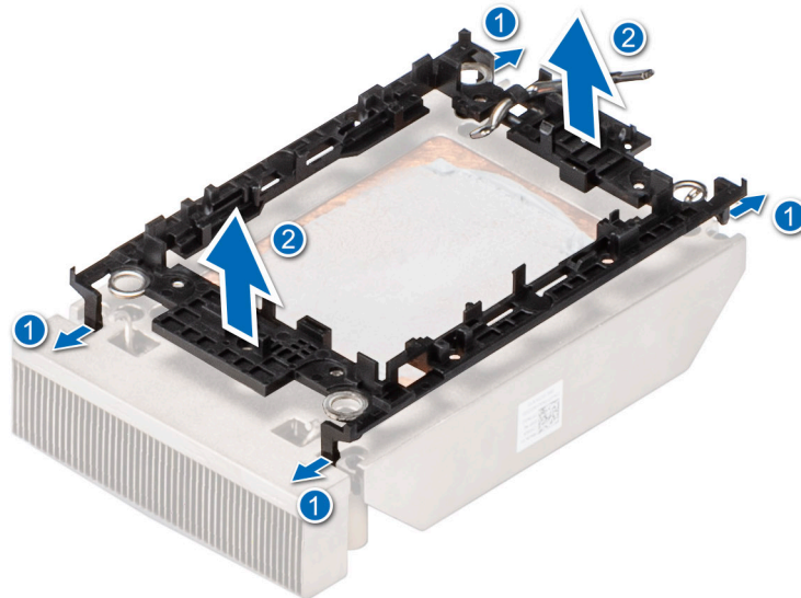
Ilustración 56. Extracción del portaunidades del procesador
