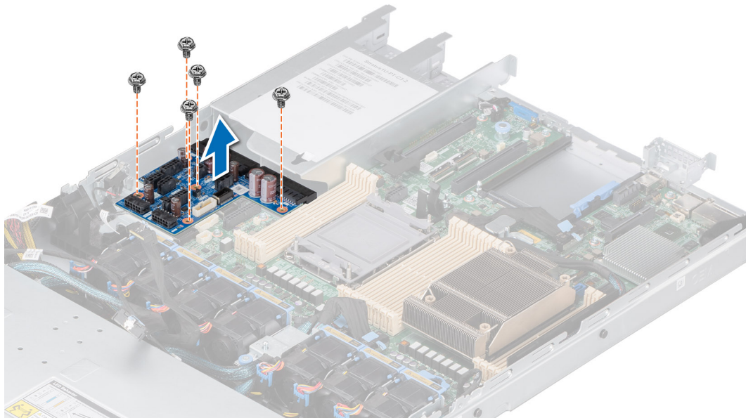
Ilustración 123. Extracción de la tarjeta mediadora de alimentación
