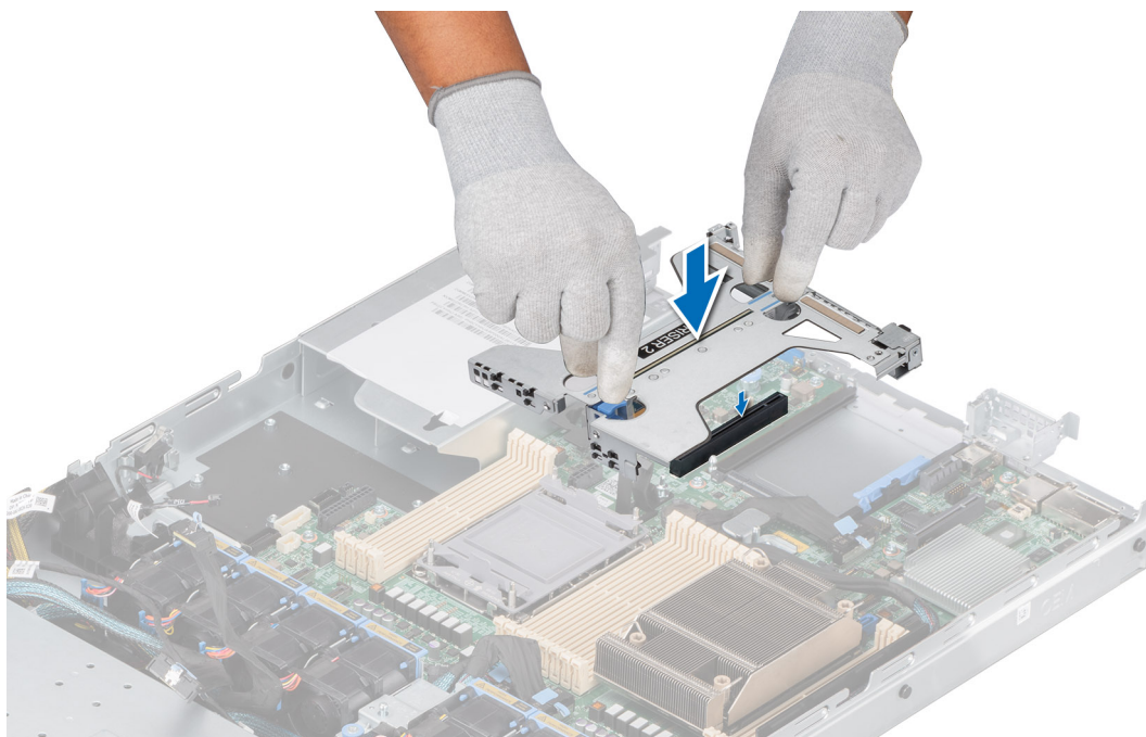
Ilustración 76. Instalación del soporte vertical 2c
