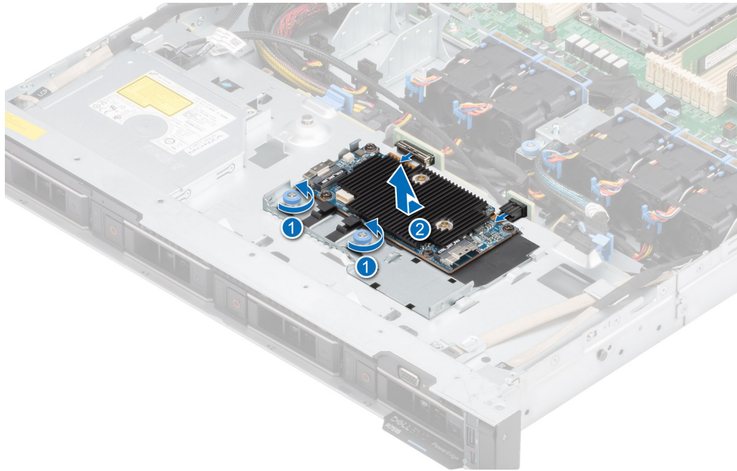
Ilustración 111. Extracción del módulo de PERC frontal de montaje frontal
