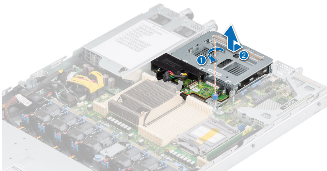
Ilustración 93. Extracción de la canastilla para unidades posteriores de 2,5 pulgadas
