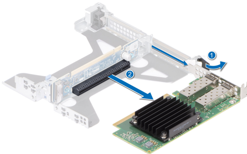
Ilustración 79. Extracción de una tarjeta de expansión del soporte vertical 2b (SNAPI)
