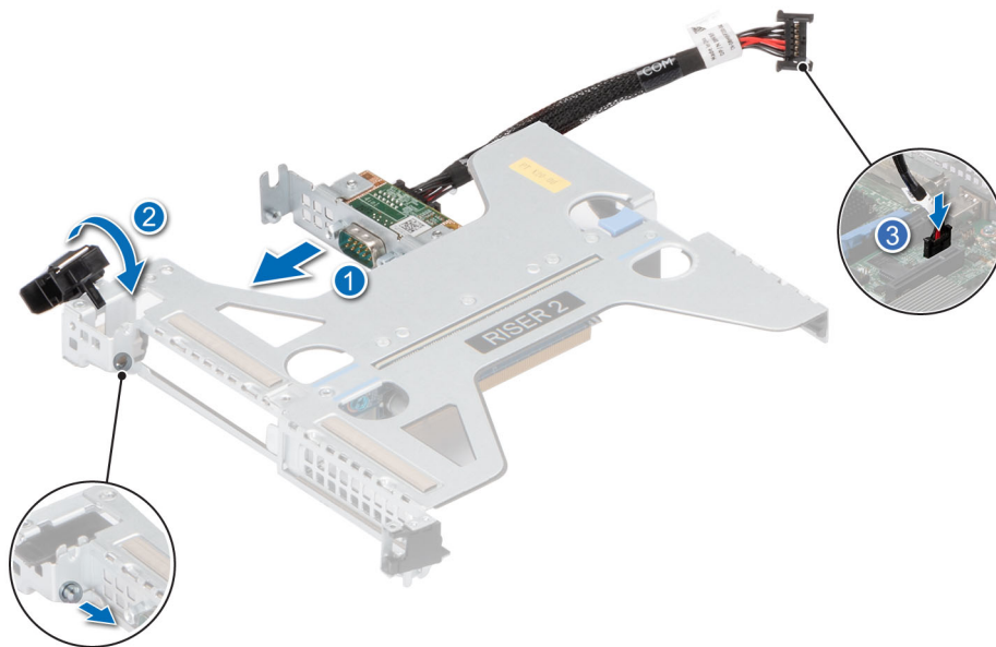
Ilustración 98. Instalación del puerto serie COM
