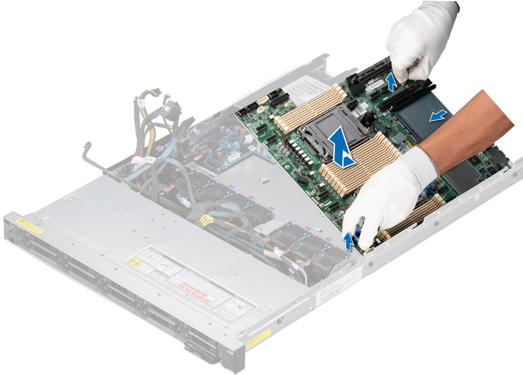
Ilustración 125. Extracción de la tarjeta madre
