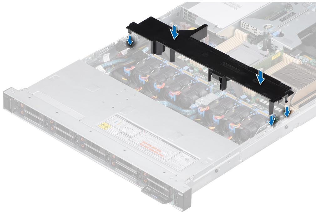
Ilustración 19. Instalación de la cubierta para flujo de aire
