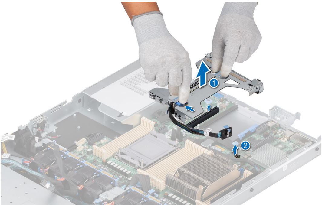
Ilustración 71. Extracción del soporte vertical 2B con el módulo SNAPi
