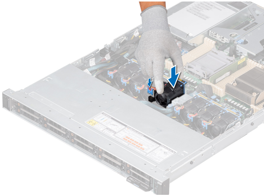
Ilustración 21. Instalación de un ventilador de refrigeración
