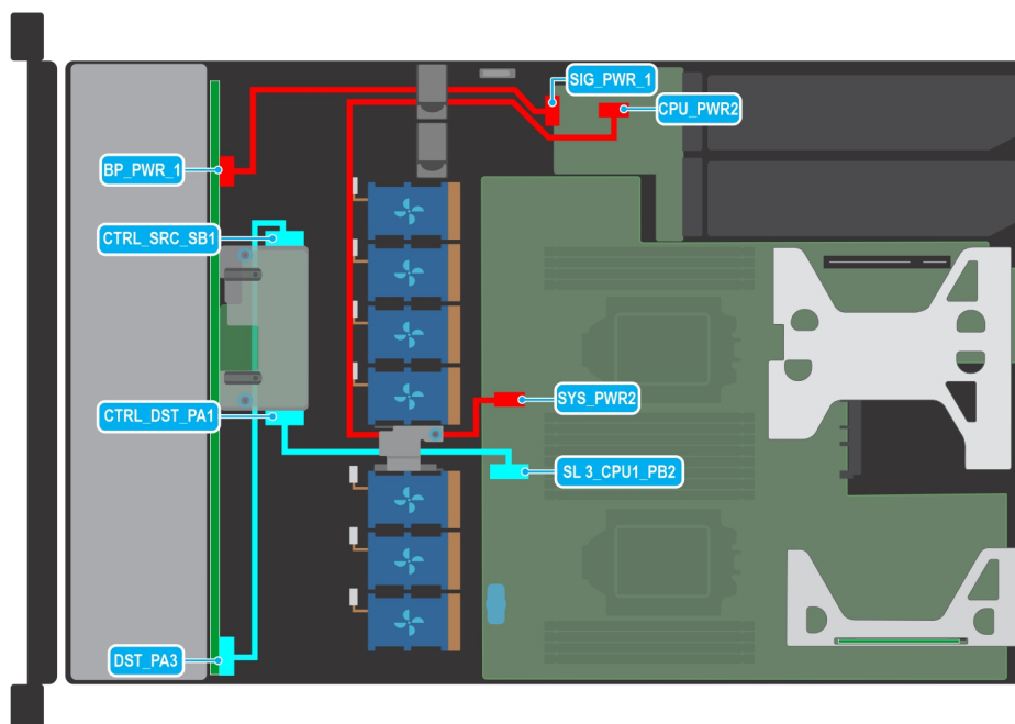
Ilustración 41. Colocación de los cables: backplane de SAS/SATA de unidad de 10 x 2,5 pulgadas con soporte vertical de mariposa y fPERC
