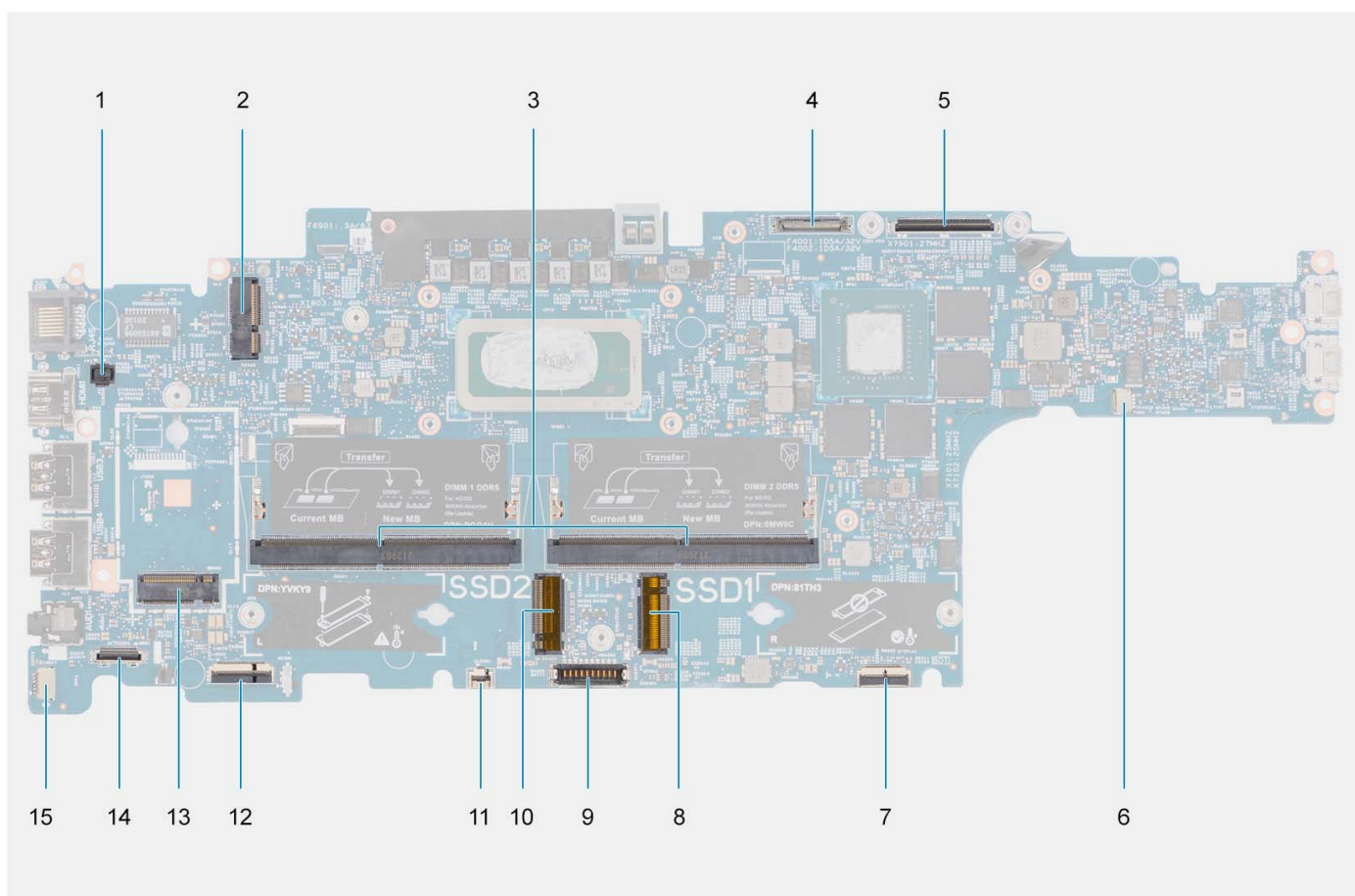
Afbeelding 1. Systeemkaartconnectoren
