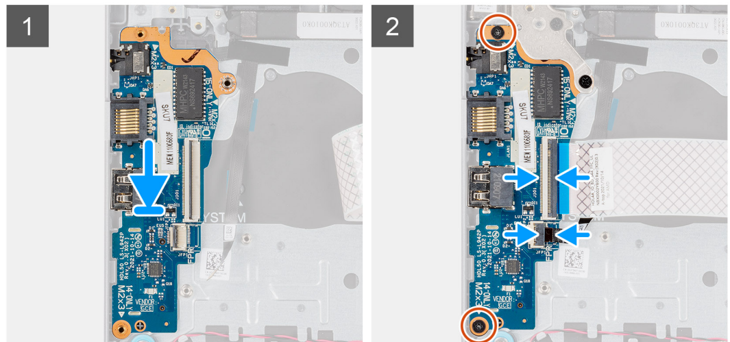
2x M2x3.5
