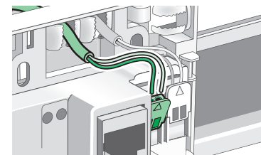
Câblage du demi-cordon ADSL sur le DTI
