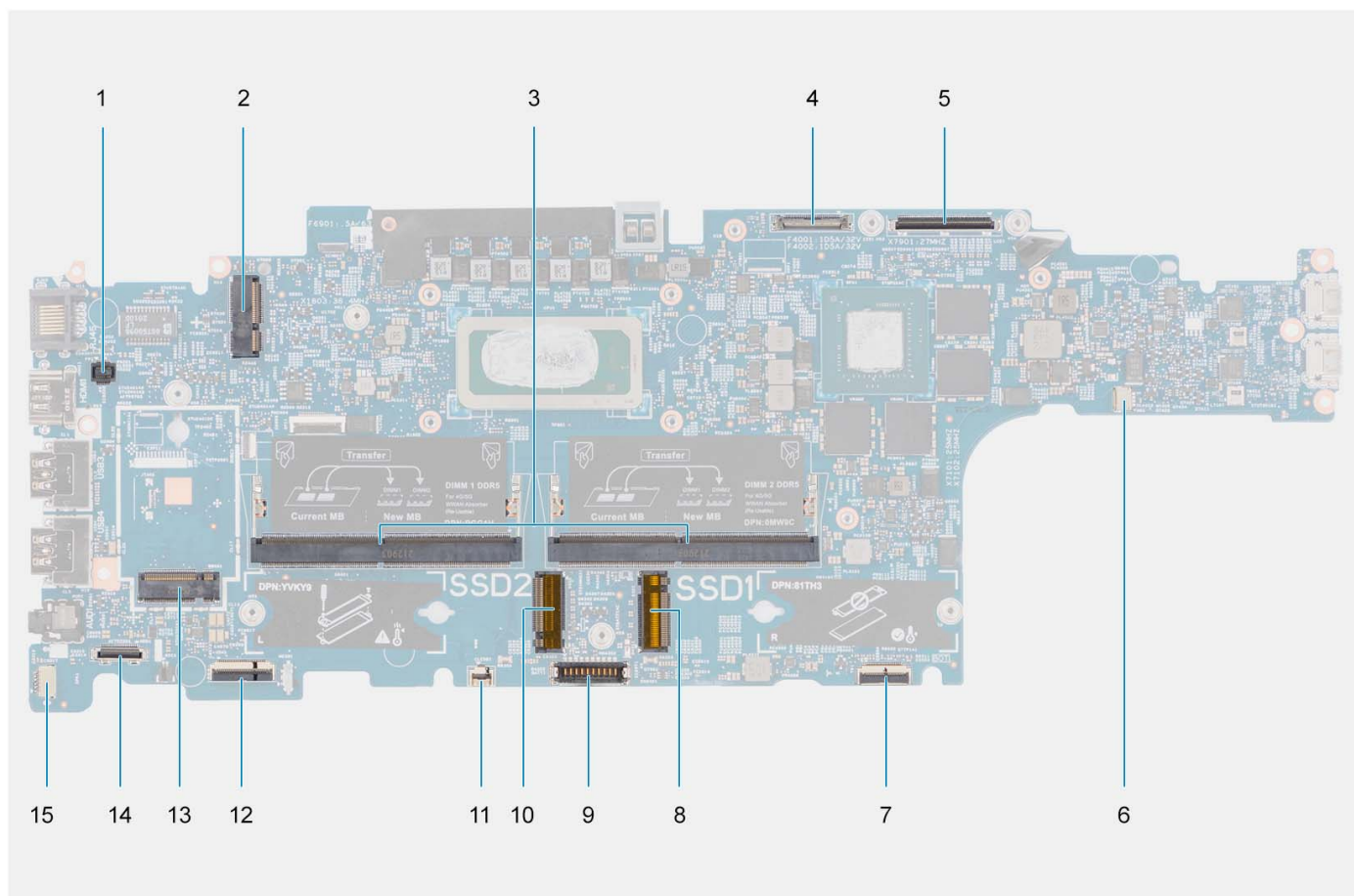
Figura 1. Connettori della scheda di sistema
