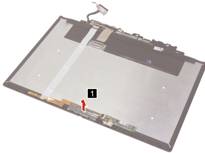
Figure 37. Remove the camera AI foil
