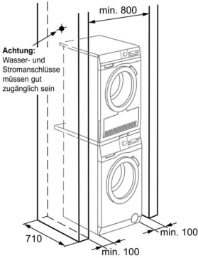
Belüftungsbeispiel für Wasch-Trockensäule, Nischeneinbau
