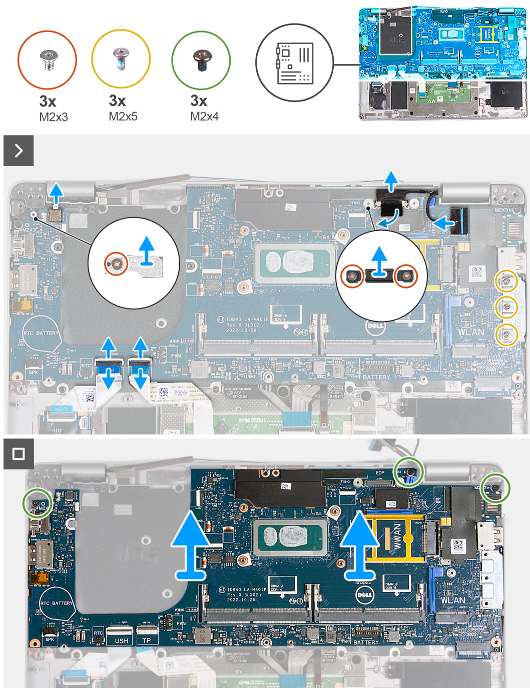
Ilustración 54. Extracción de la tarjeta madre
