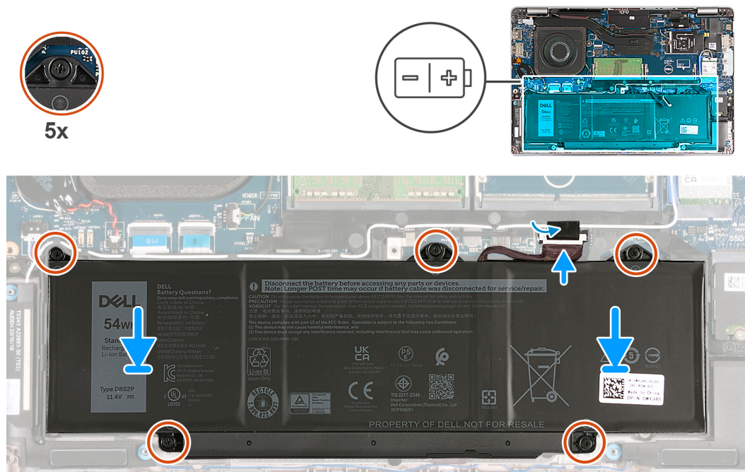
Figure 19. Installation de la batterie
