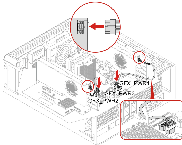
Figure 3. Cable connection for GTX RTX 4000 Ada /RTX 4500 Ada /RTX 5000 Ada /RTX 6000 Ada /RTX 5880 Ada
