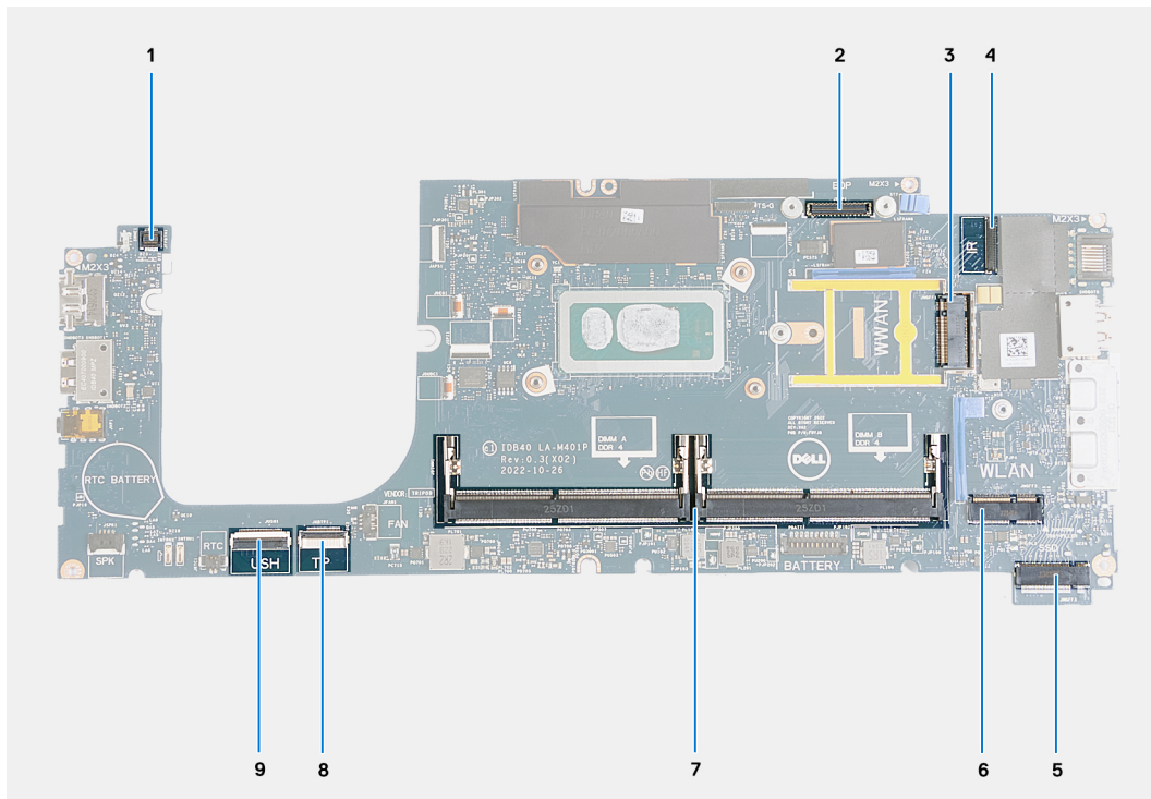
Abbildung 55. Systemplatinenanschlüsse
