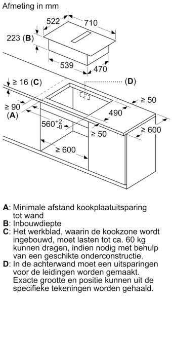
Afmeting in mm Vooraanzicht - Meubeluitsparing voor circulatielucht zonder kanaal
