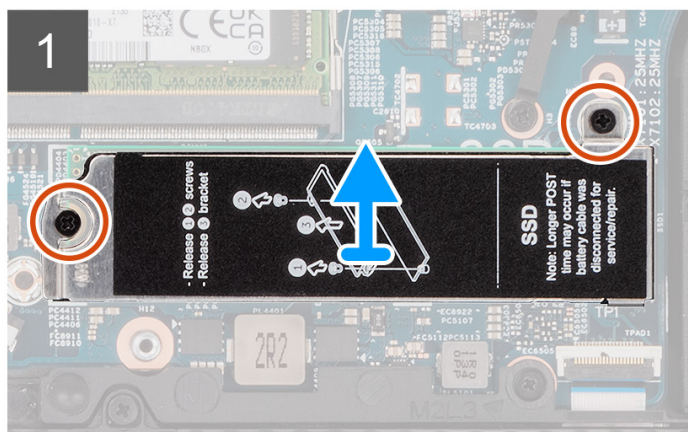
Abbildung 2. M.2-2280-Solid-State-Laufwerk mit Halterung
