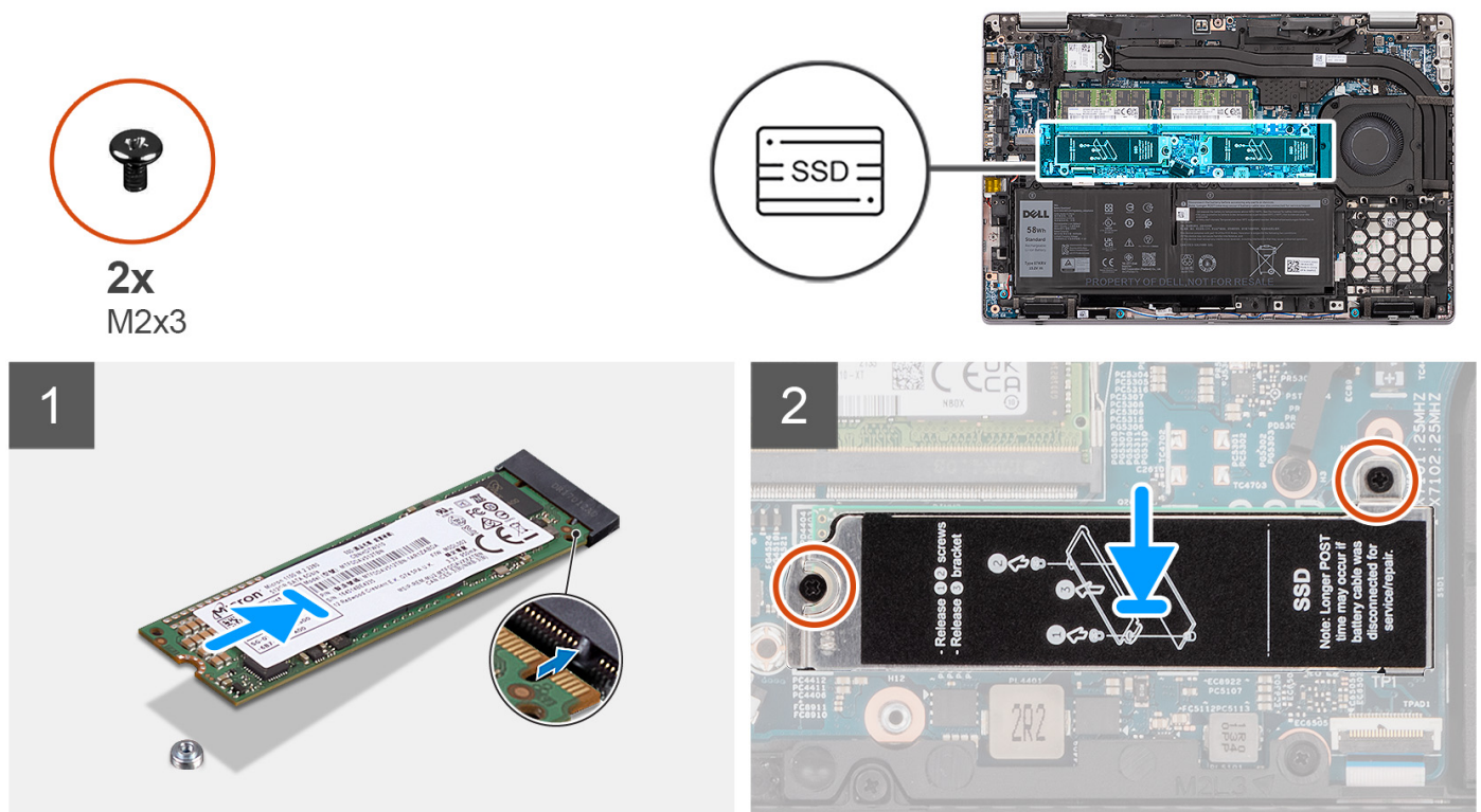
Abbildung 4. M.2-2280-Solid-State-Laufwerk mit Halterung
