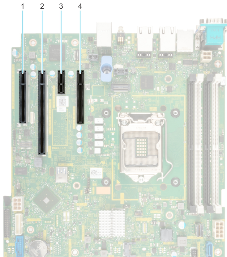
Abbildung 36. Erweiterungskarten-Steckplätze
