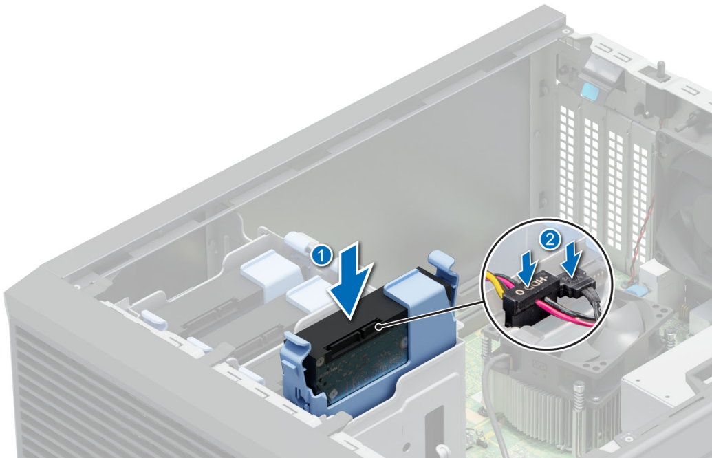
Abbildung 13. Installieren des Laufwerkträgers im Laufwerksschacht
