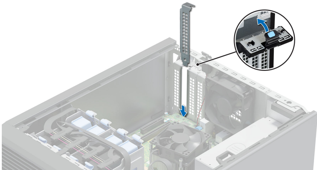
Abbildung 38. Einsetzen des Abdeckblechs
