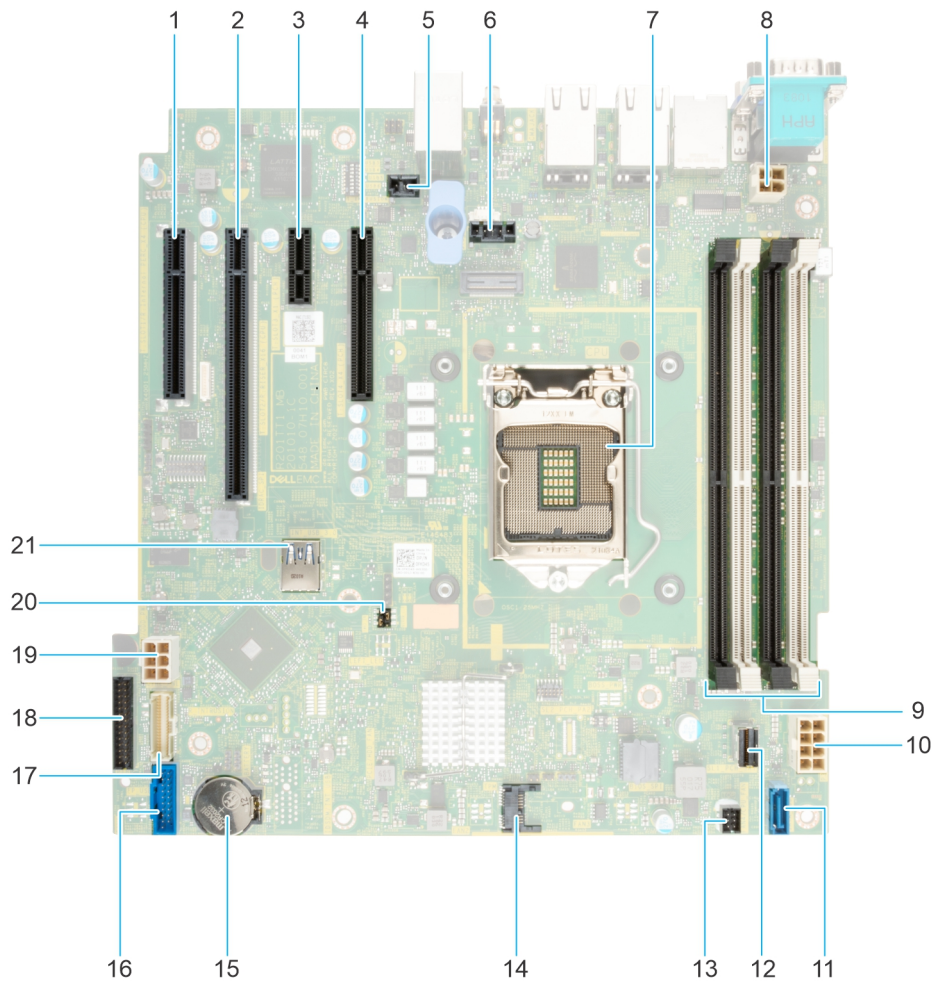
Abbildung 63. Jumper und Anschlüsse auf der Systemplatine
