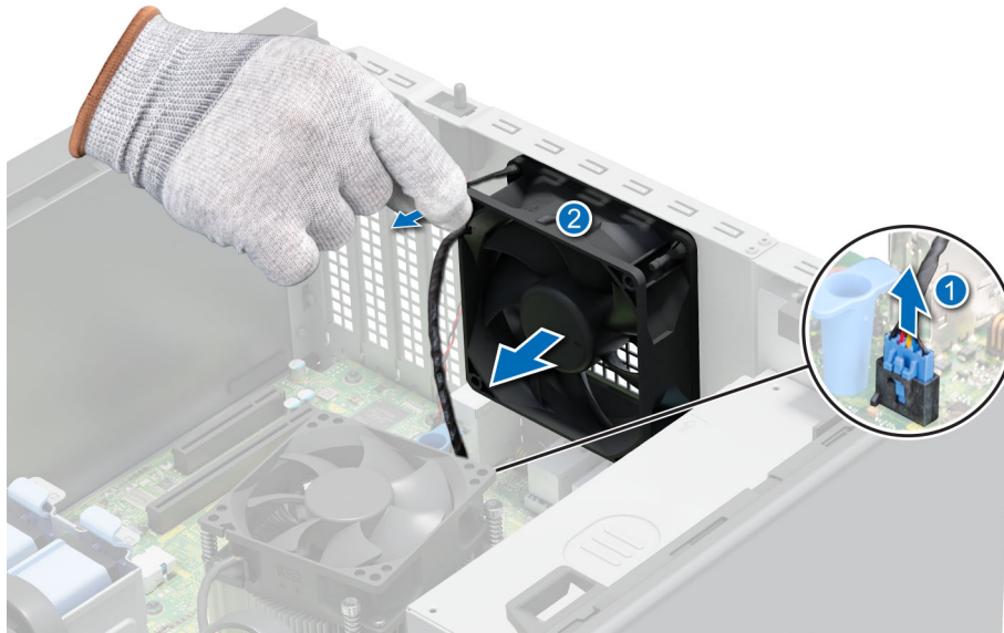
Abbildung 32. Kühlungs­lüfter entfernen
