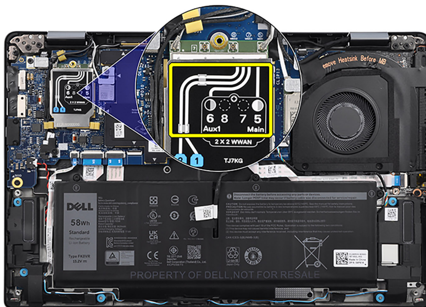
Figur 1. 4G WWAN-konfiguration
