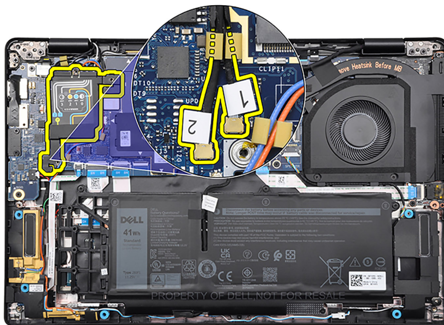
Figur 7. 5G WWAN-konfiguration
