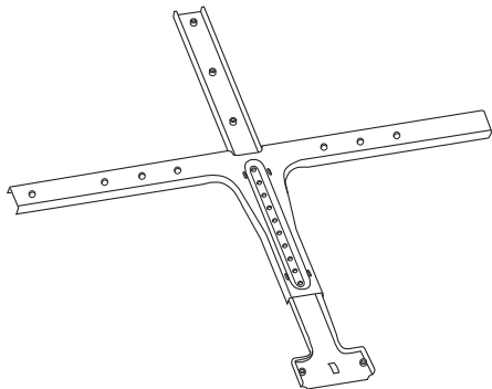
Držák na obrazovku
