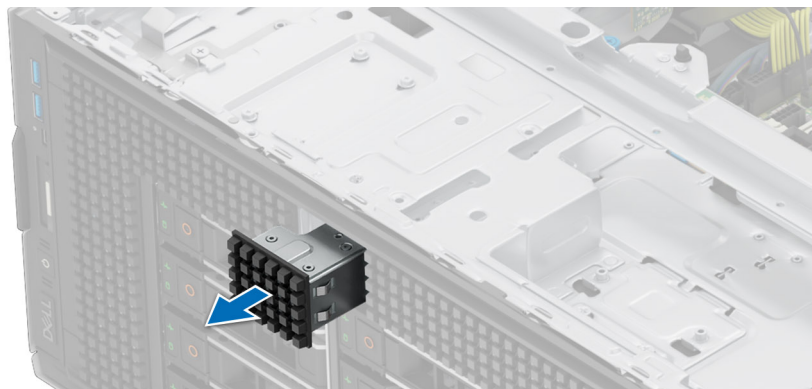
Abbildung 140. Entfernen des Platzhalters für das BOSS-N1-Modul
