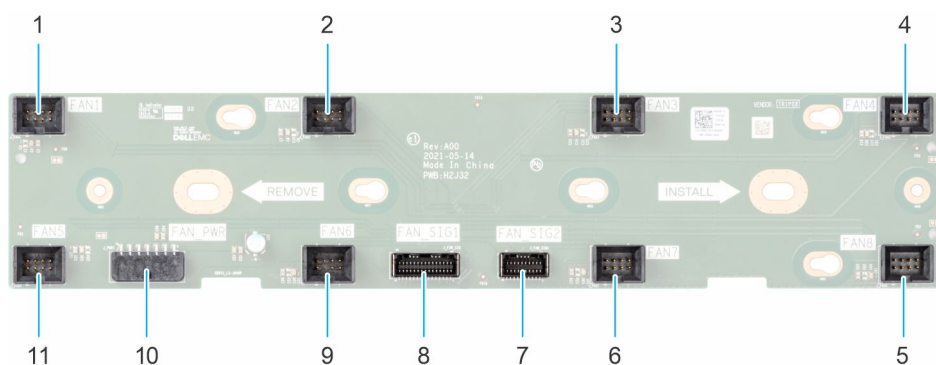
Abbildung 32. Anschlüsse auf der Lüfterplatine
