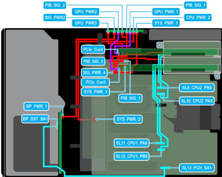
Abbildung 40. Konfiguration 2: 8 x 3,5" (Chipsatz-SATA) + 2 x GPU auf CPU 2
