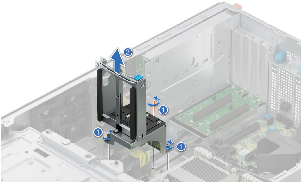
Abbildung 157. Entfernen der GPU-Karten-Halterung
