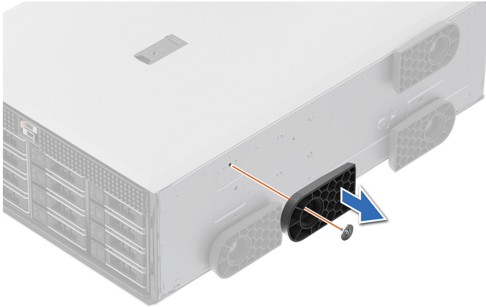
Abbildung 24. Entfernen der Systemstandfüße
