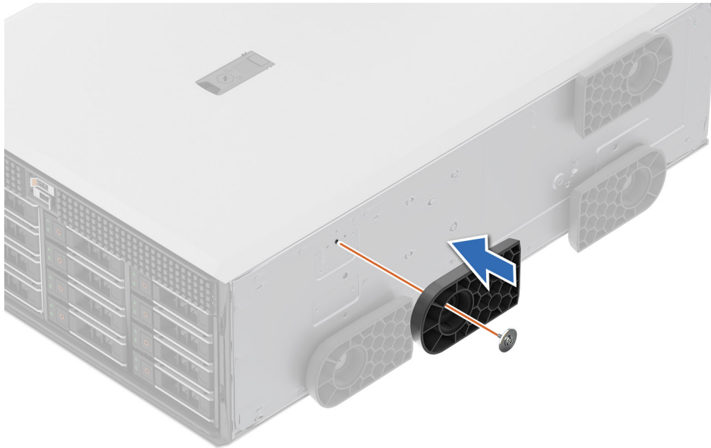
Abbildung 25. Installieren der Systemstandfüße
