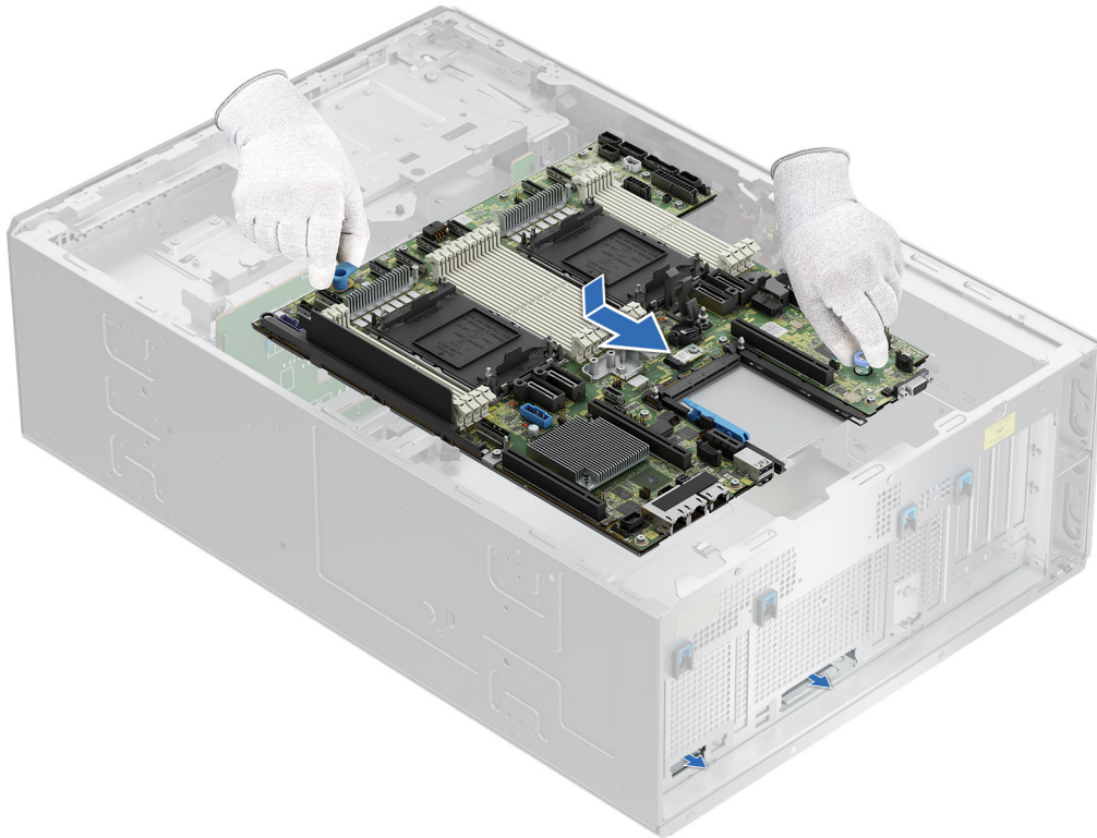
Abbildung 196. Einbauen der Systemplatine
