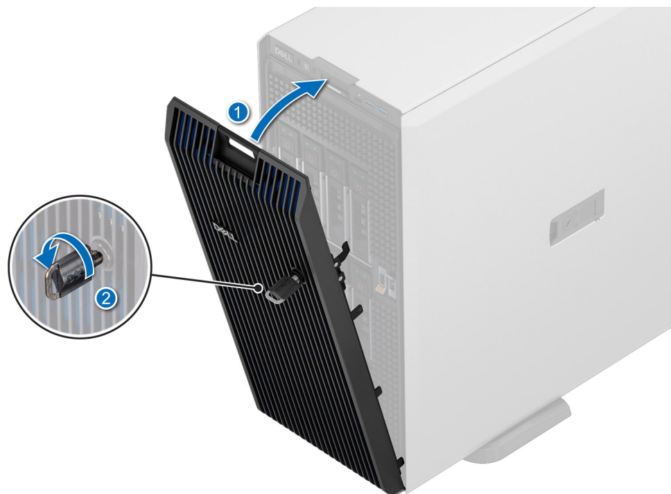
Abbildung 23. Installieren der Frontverkleidung
