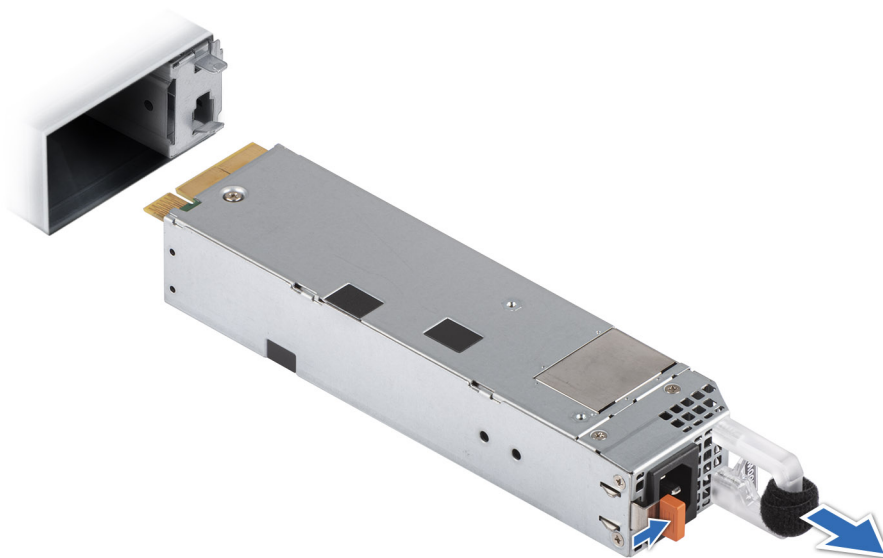
Abbildung 188. Entfernen eines 60-mm-Netzteils
