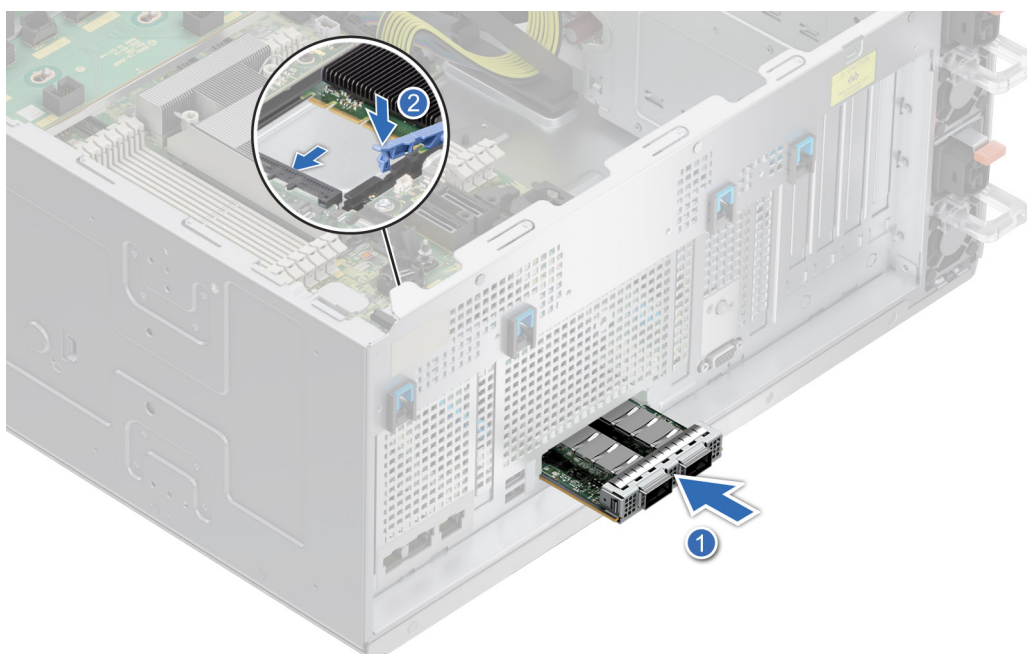
Abbildung 176. Installieren der OCP-Karte
