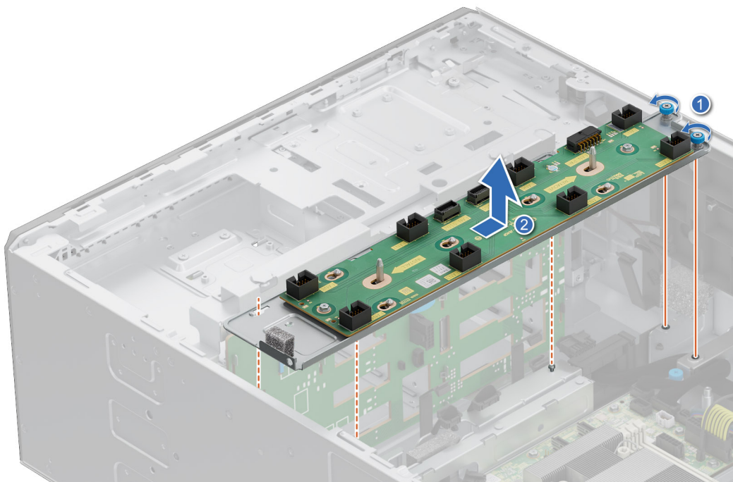
Abbildung 33. Lüfterplattenfach entfernen
