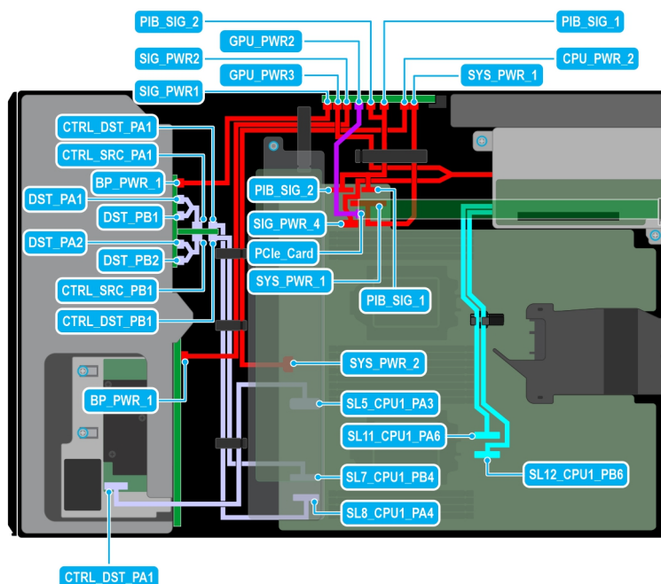
Abbildung 58. Konfiguration 20: 8 x 3,5" (SAS/SATA) + 8 x 2,5" (NVMe-RAID/fPERC12) + 1 x GPU auf CPU 2
