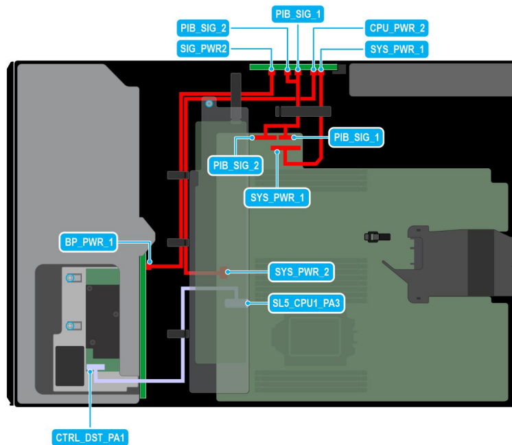
Abbildung 46. Konfiguration 8: 8 x 3,5" (SAS/SATA) auf CPU 1
