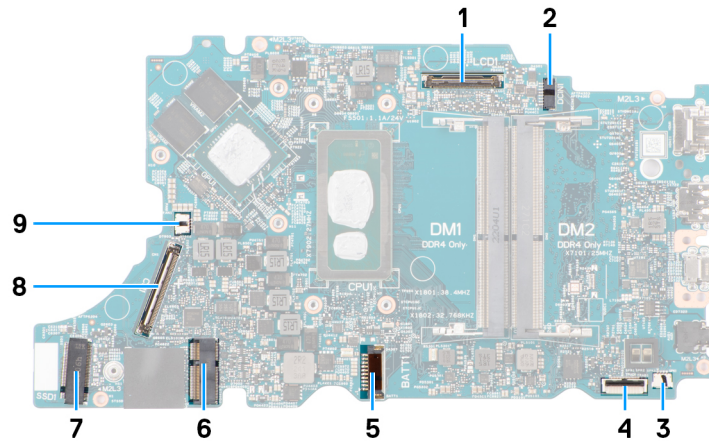
Figure 1. Connecteurs de la carte système
