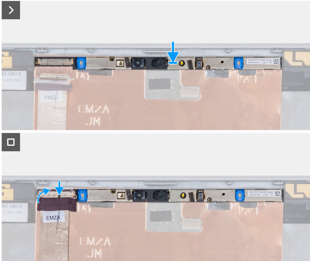
Ilustración 3. Instalación del módulo de la cámara
