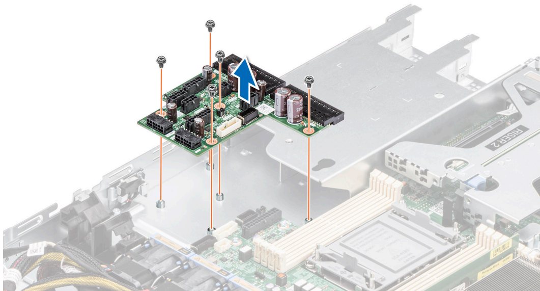
Ilustración 1. Extracción de la tarjeta mediadora de alimentación
