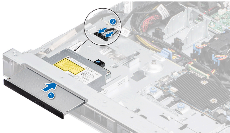
Abbildung 31. Installieren des optischen Laufwerks
