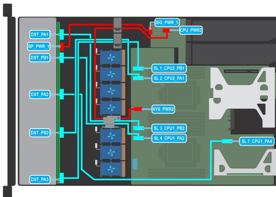
Abbildung 38. Kabelführung – 10 x 2,5-Zoll-Laufwerkrückwandplatine zum integrierten Controller (6:4 NVMe)
