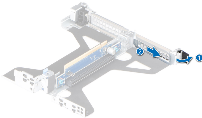
Abbildung 88. Entfernen des Abdeckblechs aus Riser 2c
