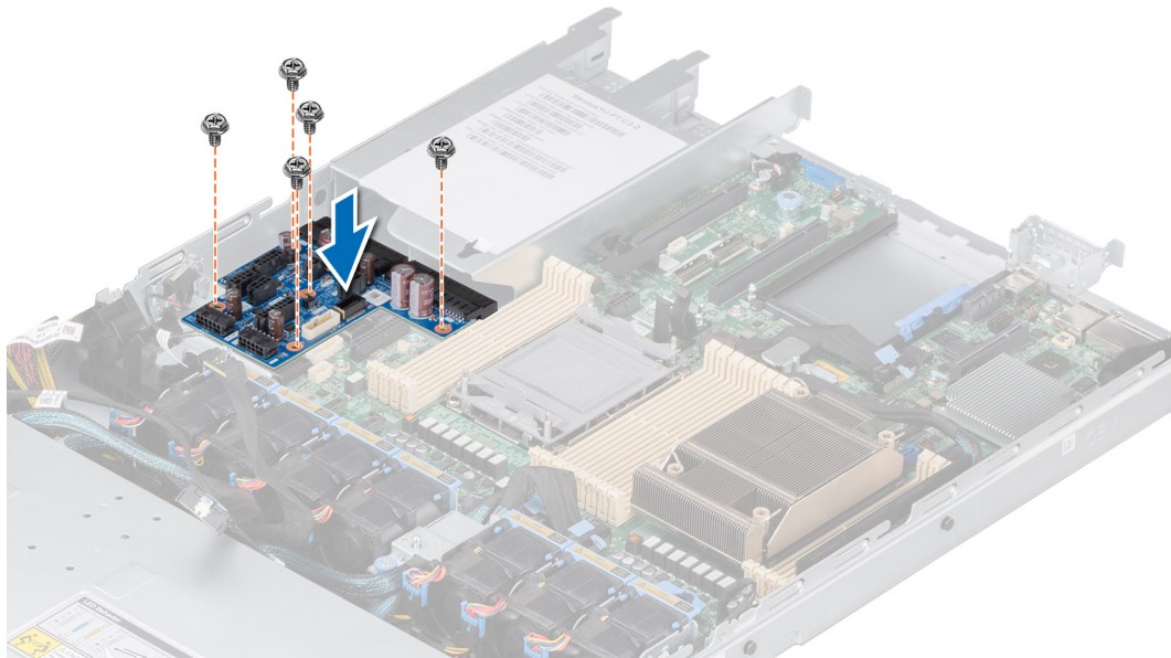
Abbildung 124. Installieren der Stromzwischenplatte
