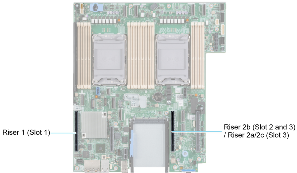
Abbildung 64. Erweiterungskarten-Steckplätze
