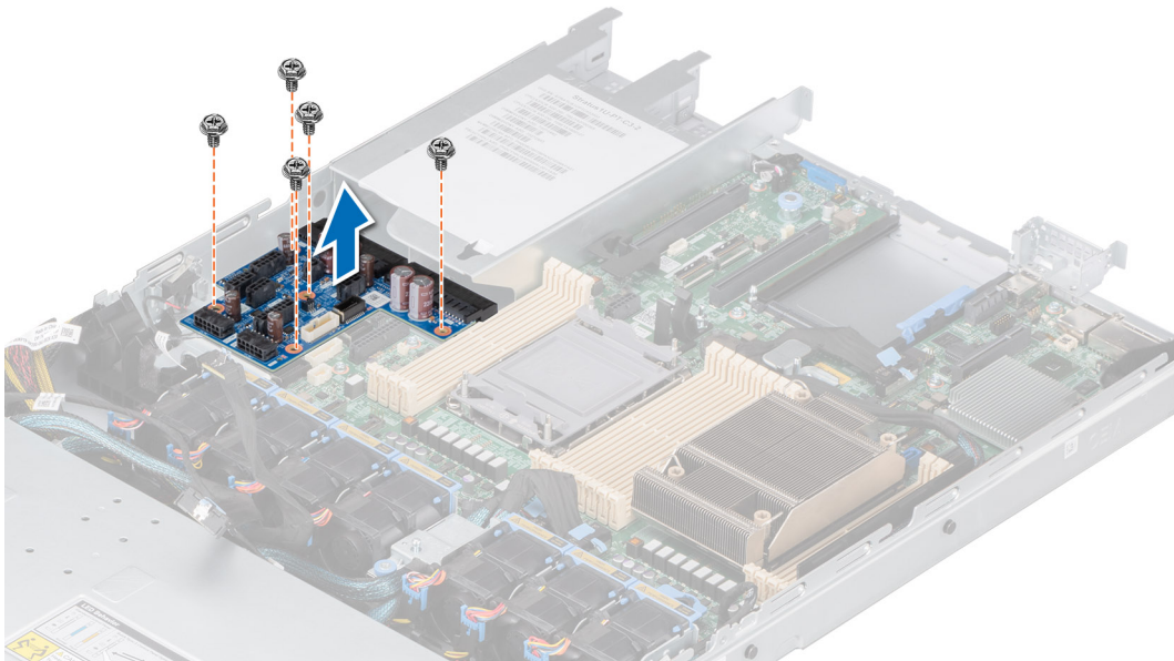
Abbildung 123. Stromzwischenplatine entfernen
