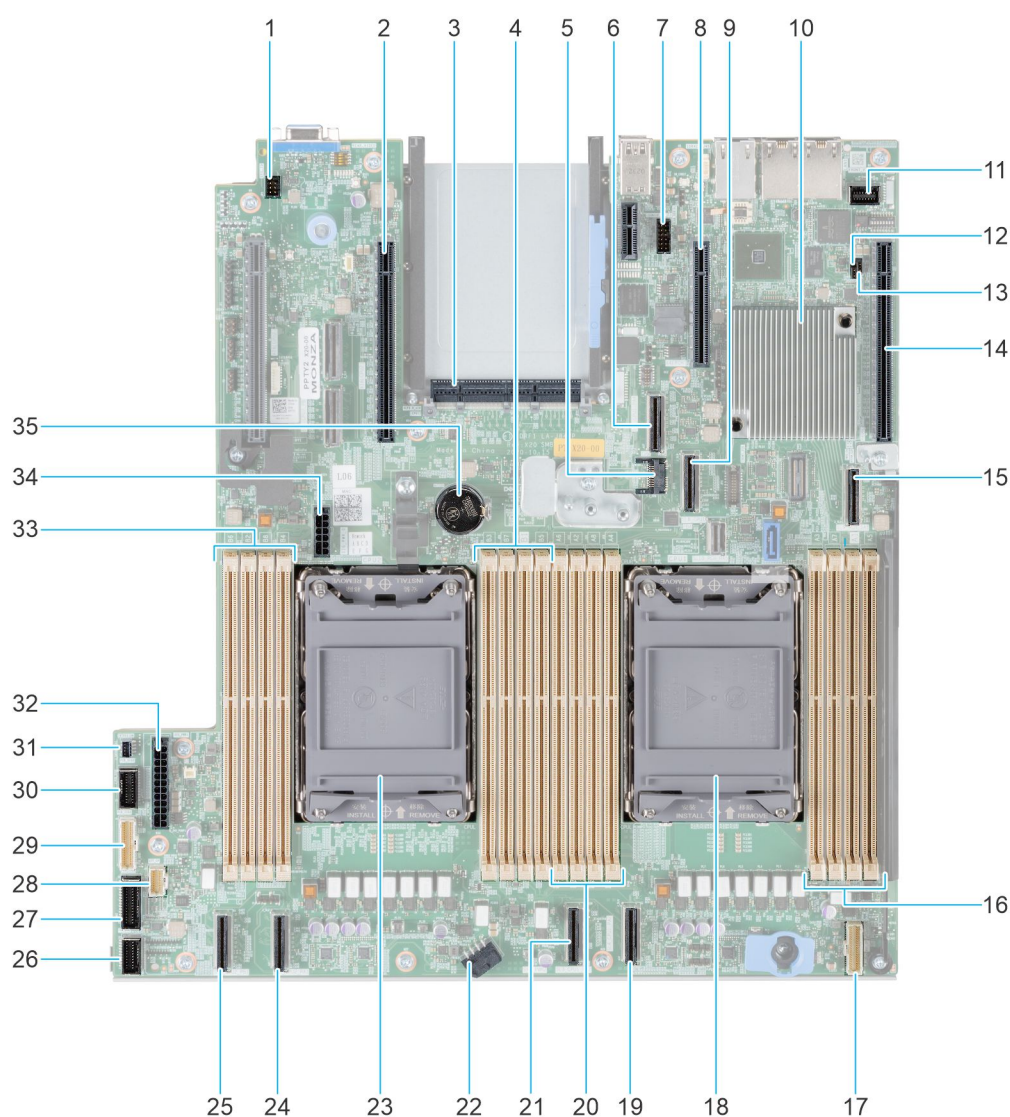
Ilustración 132. Puentes y conectores de la tarjeta madre del sistema
