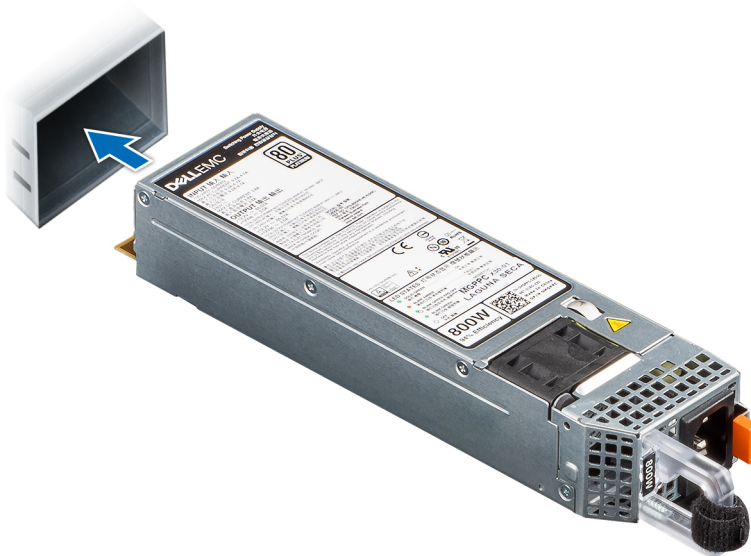
Ilustración 122. Instalación de una fuente de alimentación
