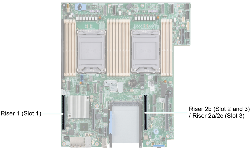
Ilustración 64. Conectores de la ranura de tarjetas de expansión
