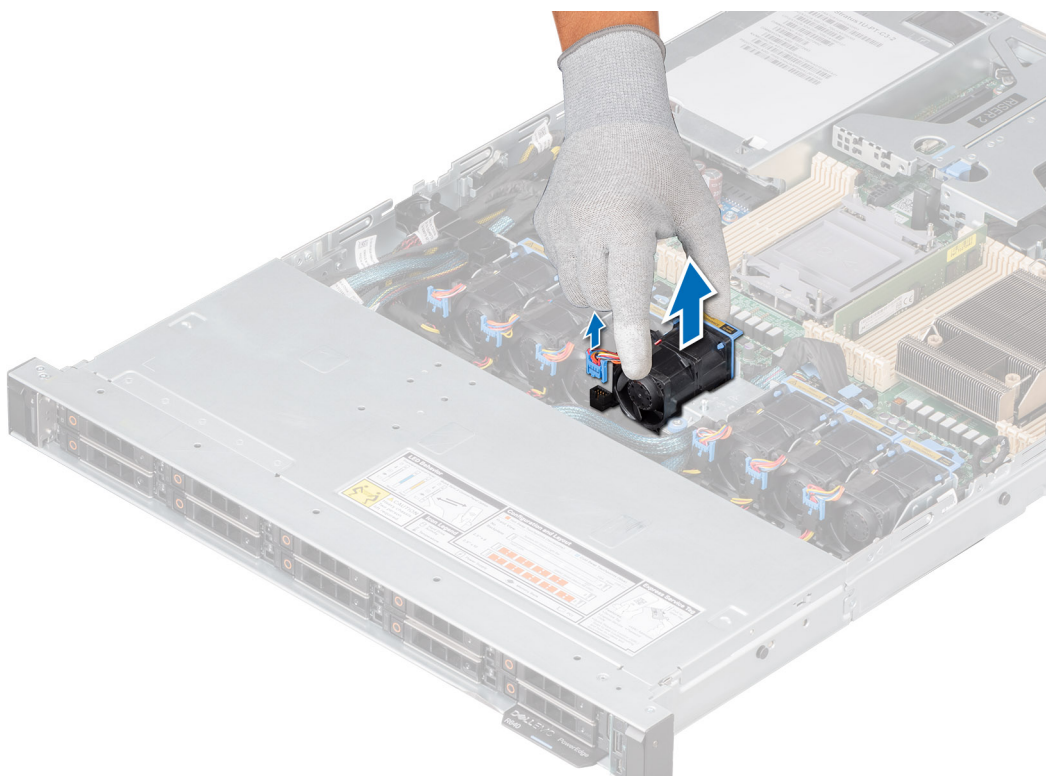
Ilustración 20. Extracción de un ventilador de refrigeración
