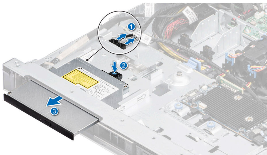
Ilustración 30. Extracción de la unidad óptica
