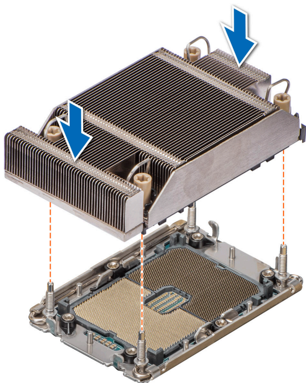
Ilustración 62. Instalación del procesador y del disipador de calor (PHM)
