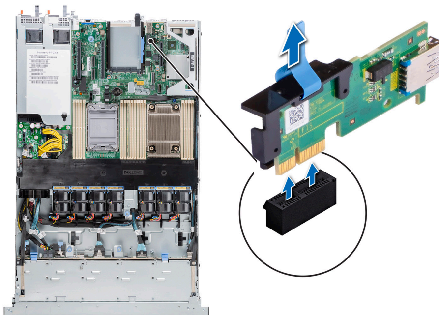
Ilustración 115. Extracción de la tarjeta USB interna
