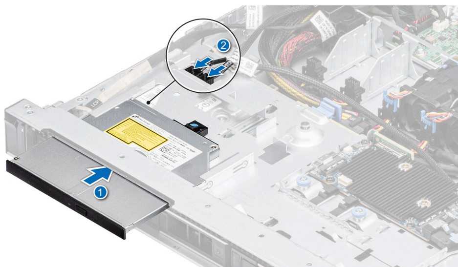
Ilustración 31. Instalación de la unidad óptica
