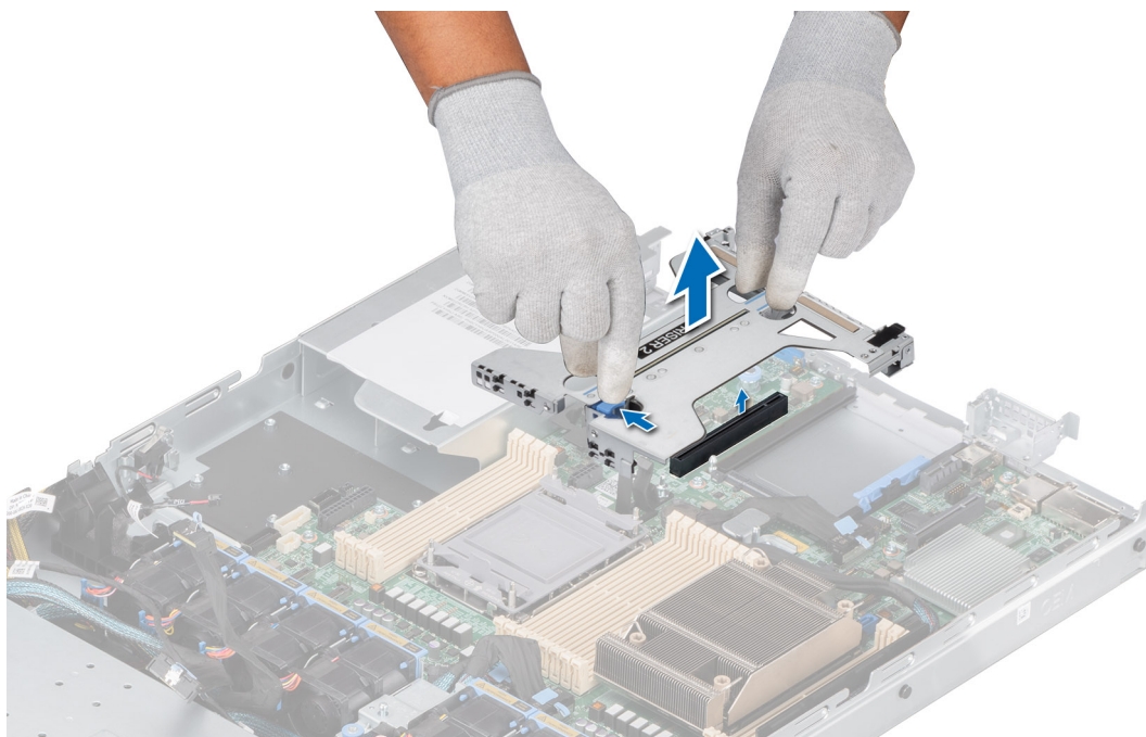
Ilustración 70. Extracción del Soporte vertical 2a
