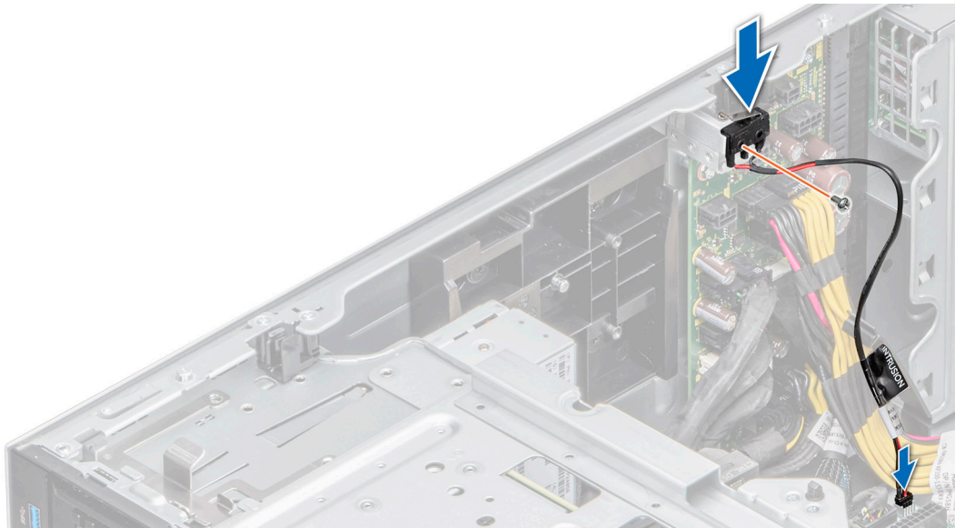
Figure 164. Installation du module du commutateur d'intrusion
