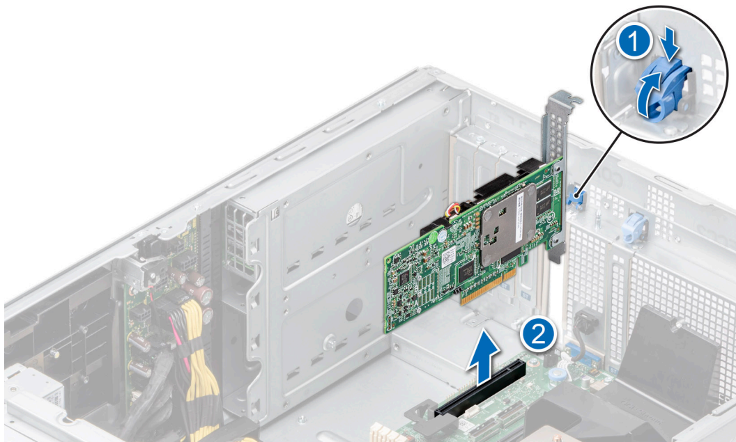
Figure 130. Retrait d'une carte d'extension
