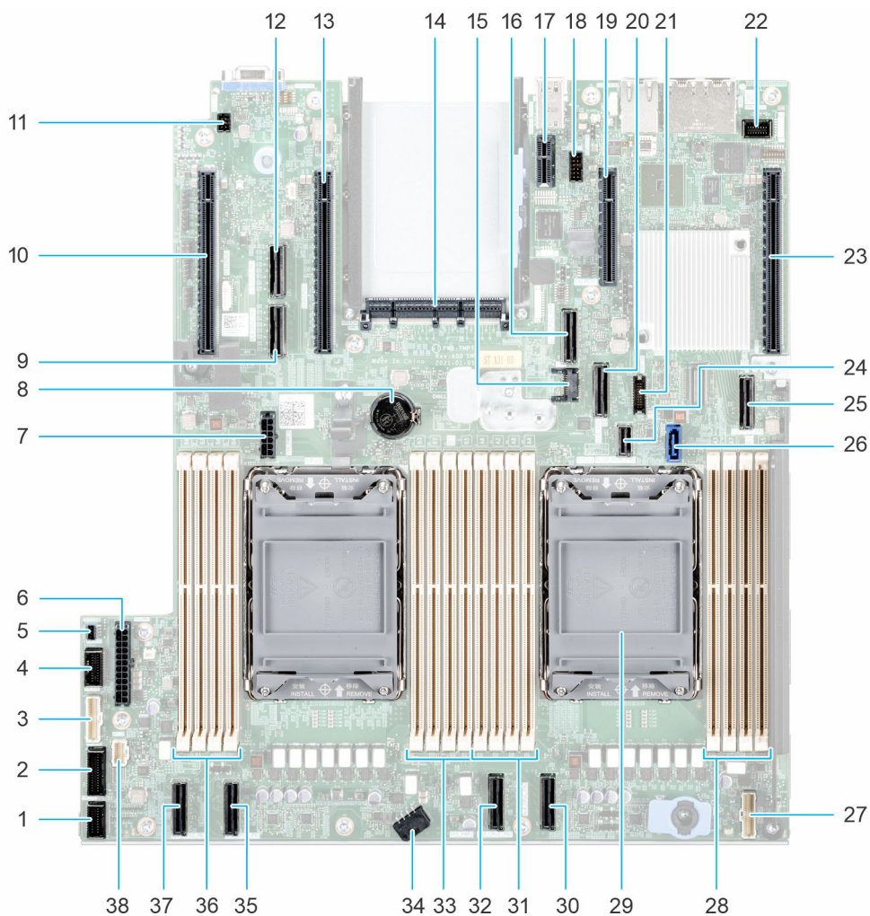
Figure 181. Connecteurs et cavaliers de la carte système
