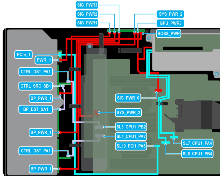
Figure 84. Acheminement des câbles : 24 disques SAS de 2,5 pouces avec carte de montage pour processeur graphique
