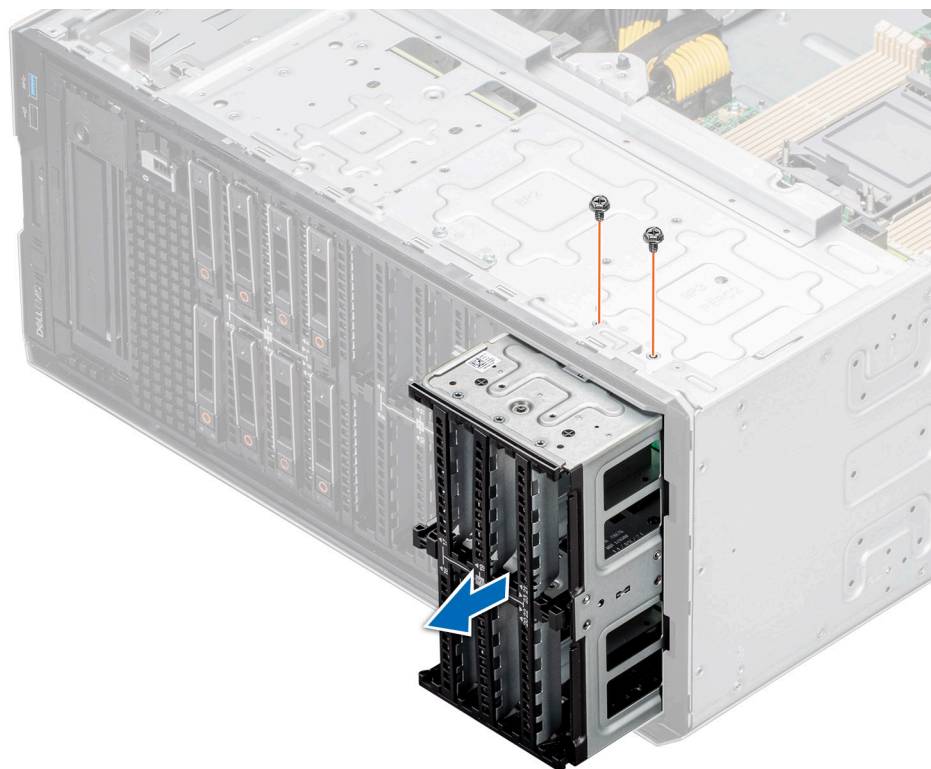
Figure 69. Retrait d'une baie de disques
