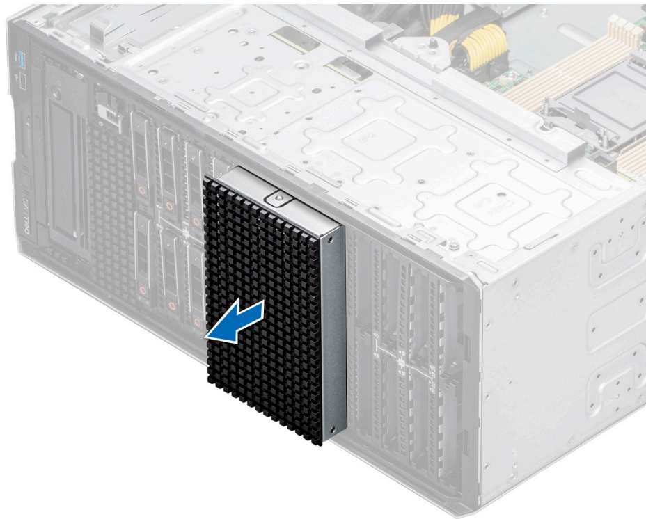
Figure 64. Retrait du cache du bâti de la baie de disques
