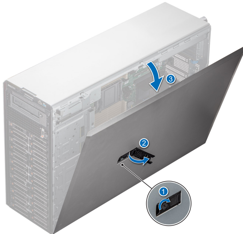
Figure 33. Retrait du capot du système
