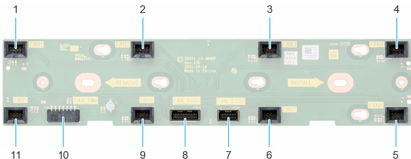
Figure 41. Connecteurs du ventilateur
