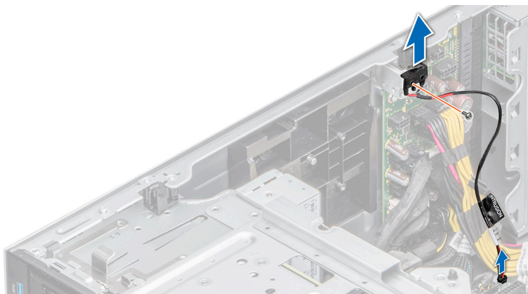
Figure 163. Retrait du module du commutateur d'intrusion
