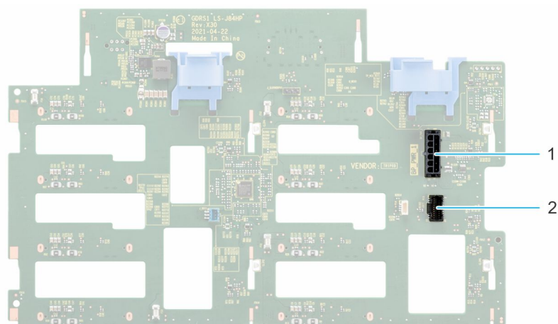
Figure 58. Fond de panier de disques de 3,5 pouces
