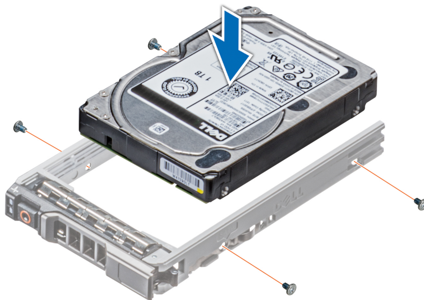
Figure 53. Installation d'un disque dans un support de disque
