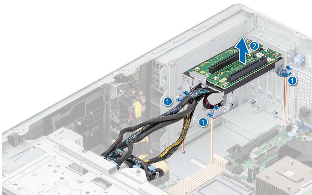
Figure 140. Retrait de la carte de montage de processeur graphique
