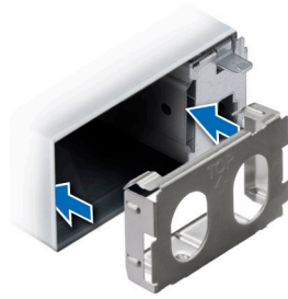
Figure 167. Installation du cache de bloc d'alimentation 60 mm
