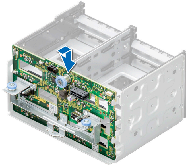
Figure 63. Installation le fond de panier de disque de 2,5 pouces
