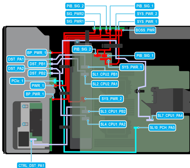
Figure 92. Acheminement des câbles : 8 disques de 3,5 pouces + 8 disques NVMe de 2,5 pouces avec module BOSS S2
