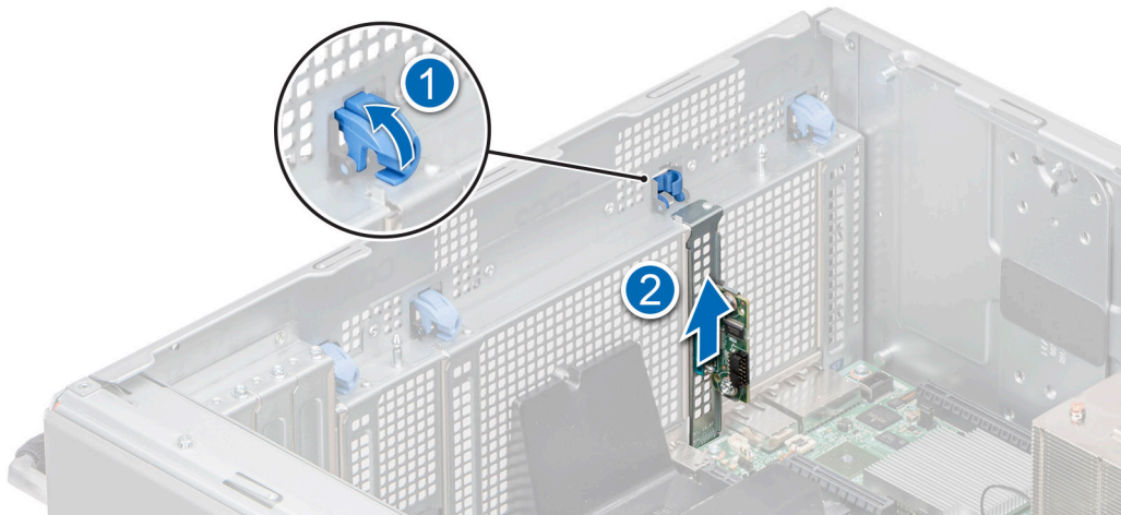
Figure 159. Retrait du port série COM
