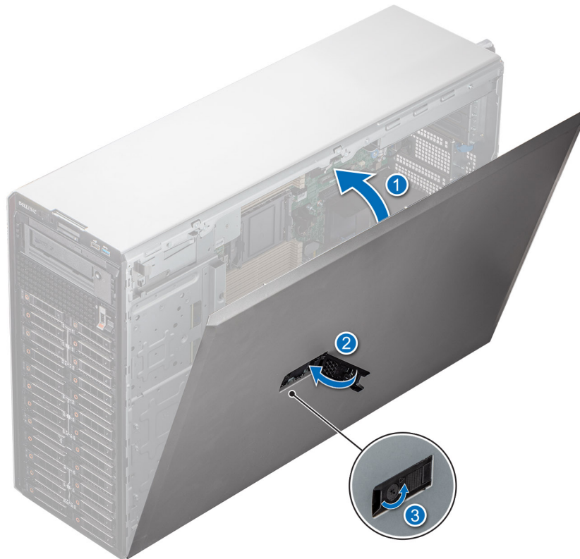
Figure 34. Installation du capot du système
