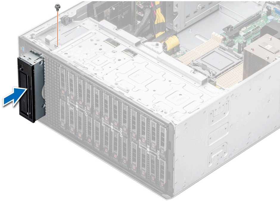
Figure 102. Installation de l'unité de sauvegarde sur bande
