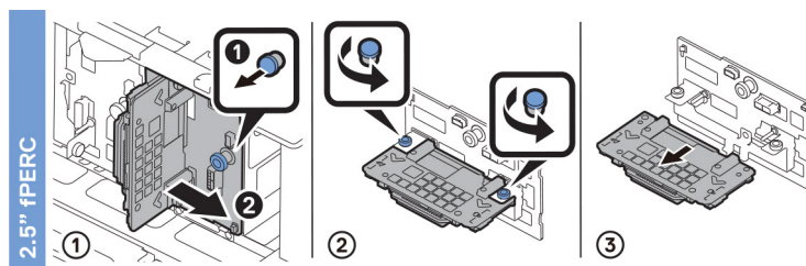
Figure 18. Disque PERC avant de 2,5 pouces
