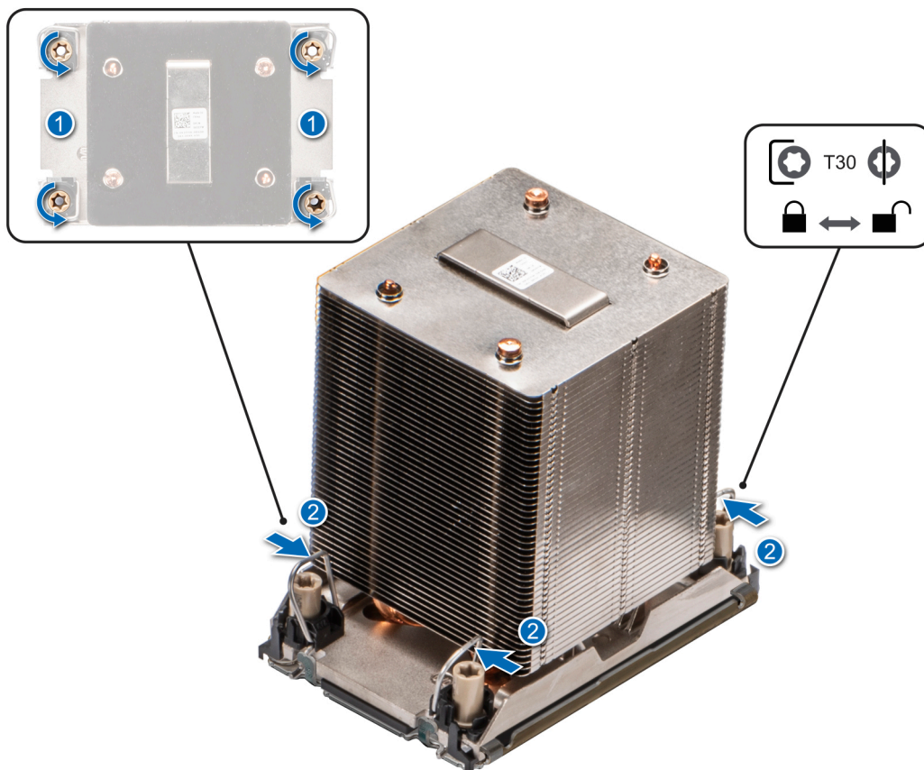
Figure 142. Retrait du module dissipateur de chaleur-processeur
