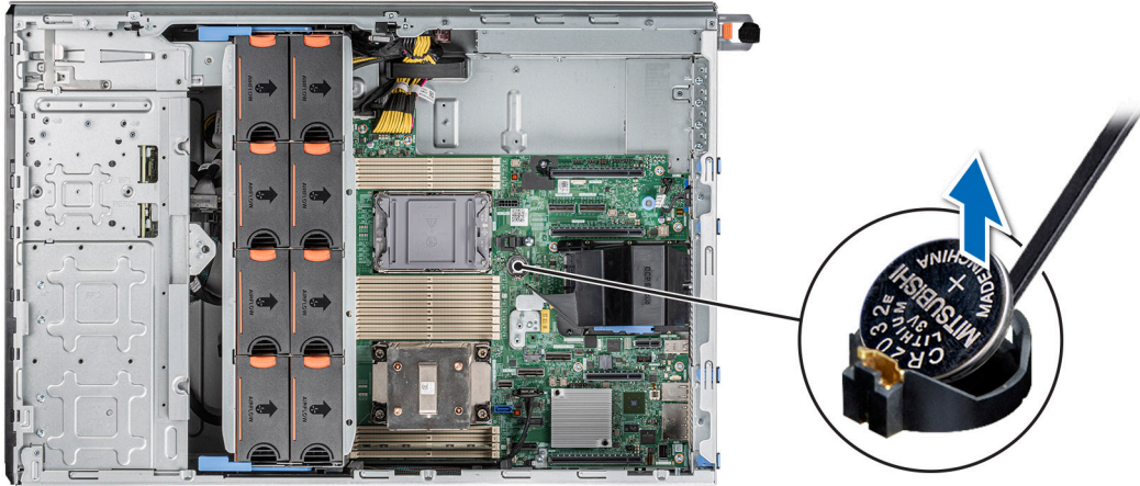
Figure 161. Retrait de la pile du système
