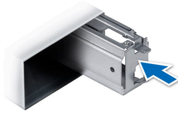
Figure 170. Installation d'un adaptateur de bloc d'alimentation
