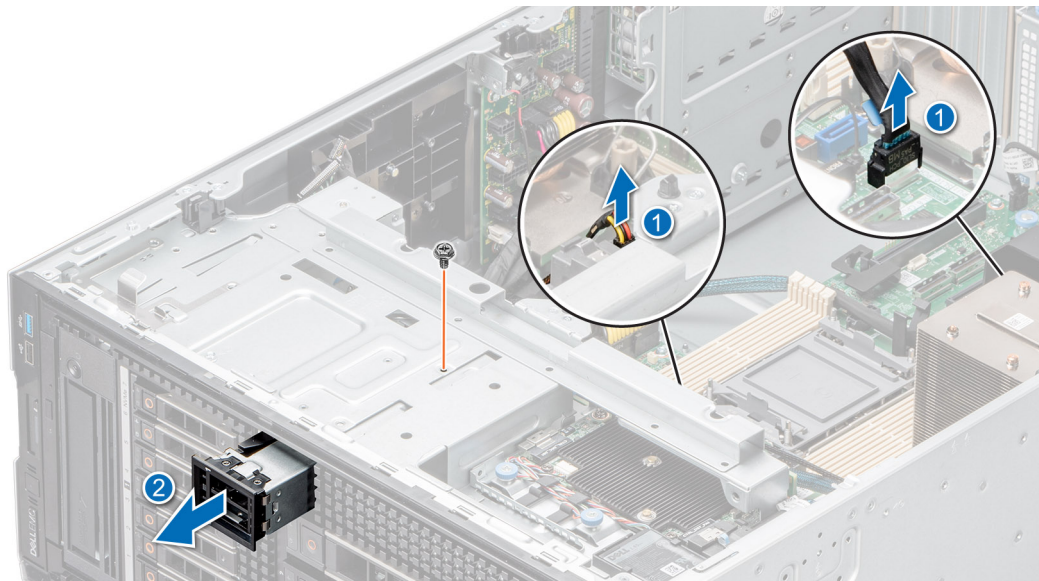
Figure 111. Retrait du module BOSS S2
