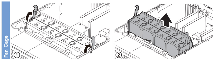
Figure 21. Plateau de la carte de ventilation
