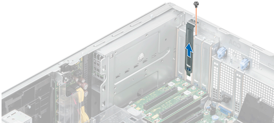
Figure 138. Retrait de la plaque de recouvrement
