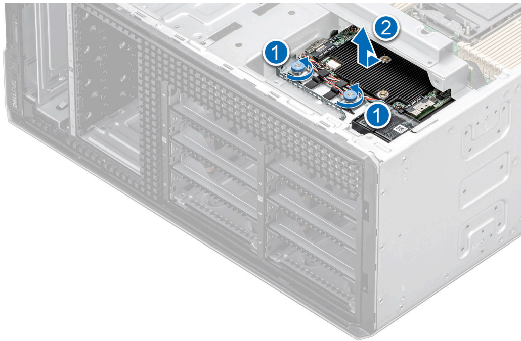
Figure 44. Retrait du module PERC avant pour fond de panier de disques de 3,5 pouces
