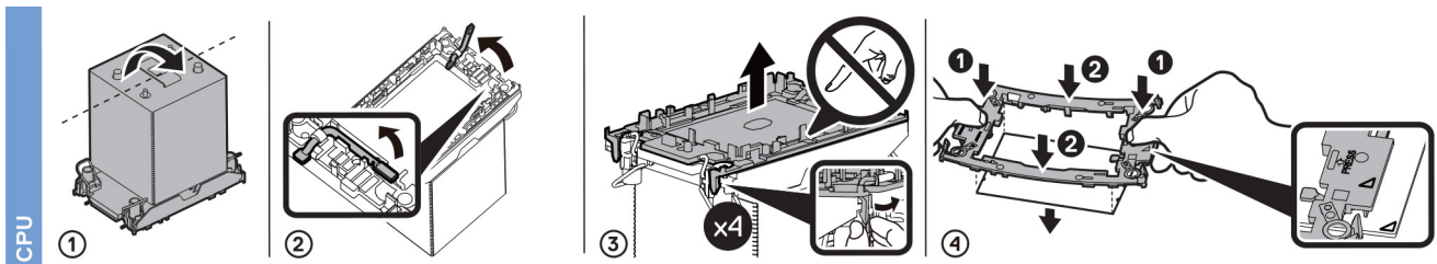
Figure 23. Processeur
