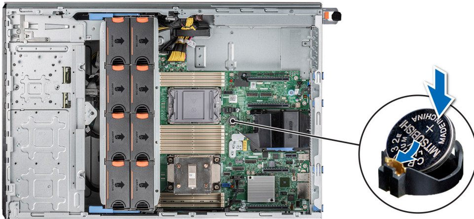
Figure 162. Installation de la pile du système
