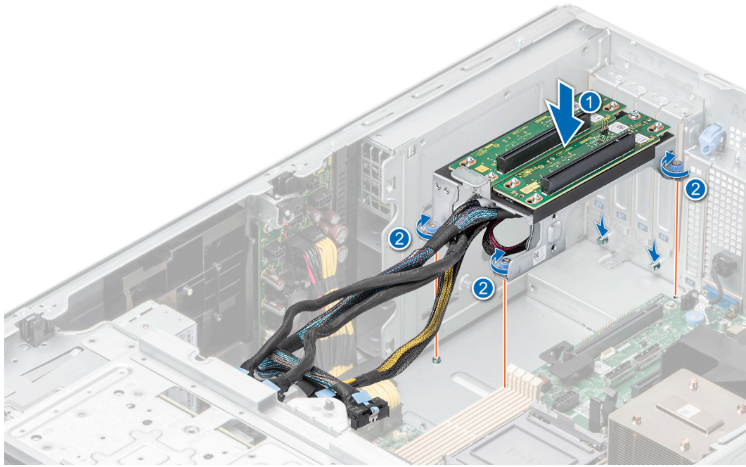
Figure 141. Installation de la carte de montage de processeur graphique
