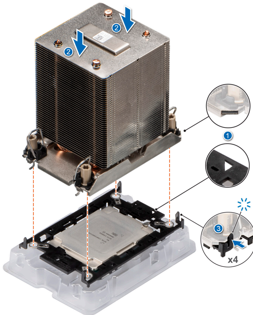
Figure 150. Installation du dissipateur de chaleur sur le processeur
