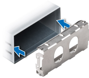
Figure 168. Installation du cache de bloc d'alimentation 86 mm
