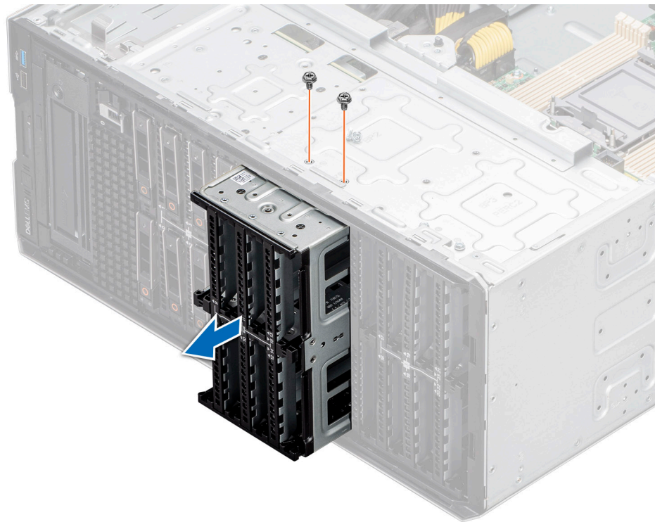
Figure 68. Retrait d'une baie de disques
