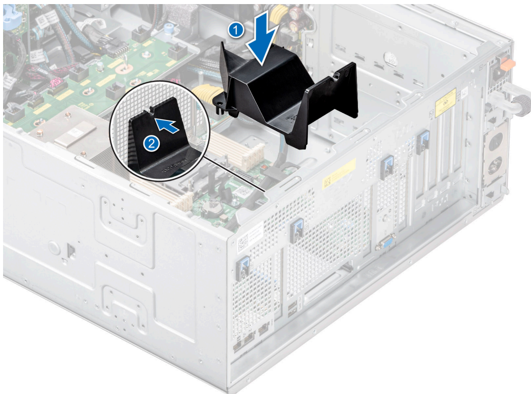
Figure 158. Installation du carénage d'aération OCP.
