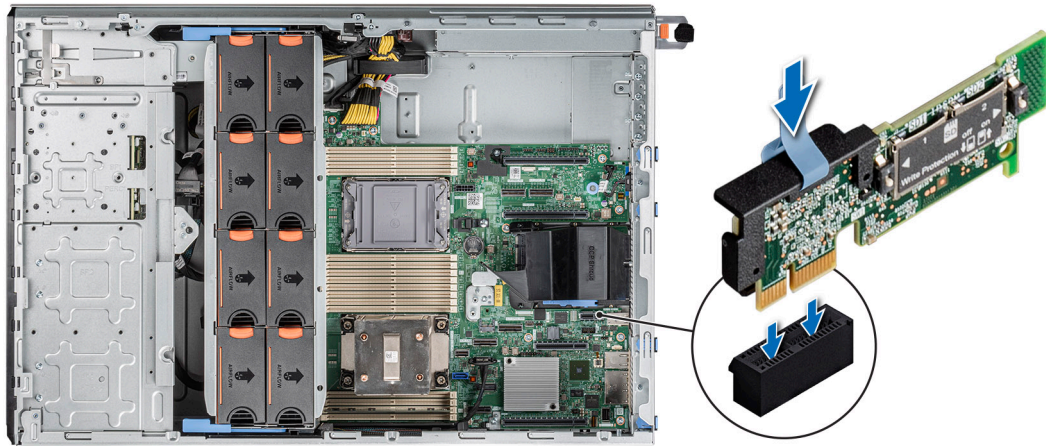
Figure 127. Installation du module IDSDM
