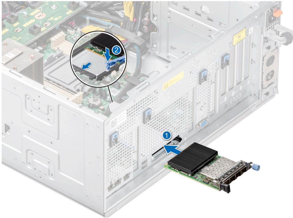
Figure 157. Installation de la carte OCP
