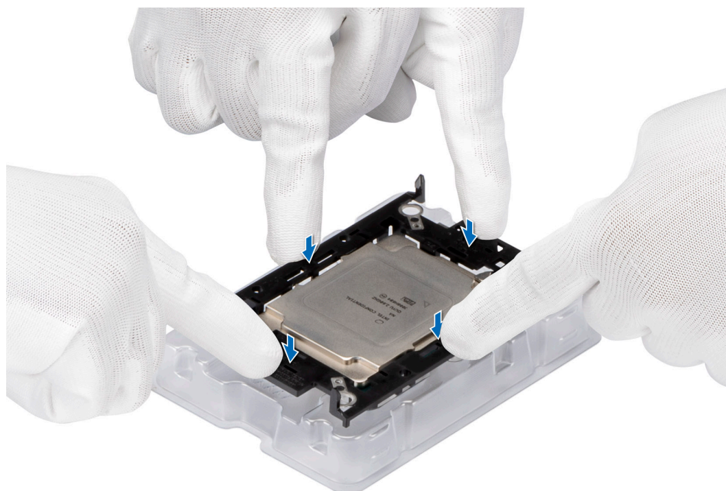
Figure 147. Pression sur le clip de fixation au niveau des quatre côtés
