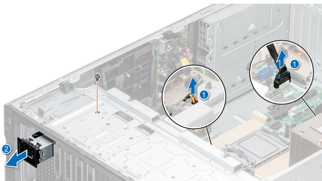
Figure 110. Retrait du module BOSS S2
