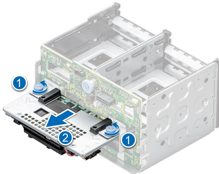
Figure 45. Retrait du module PERC avant pour fond de panier de disques de 2,5 pouces.
