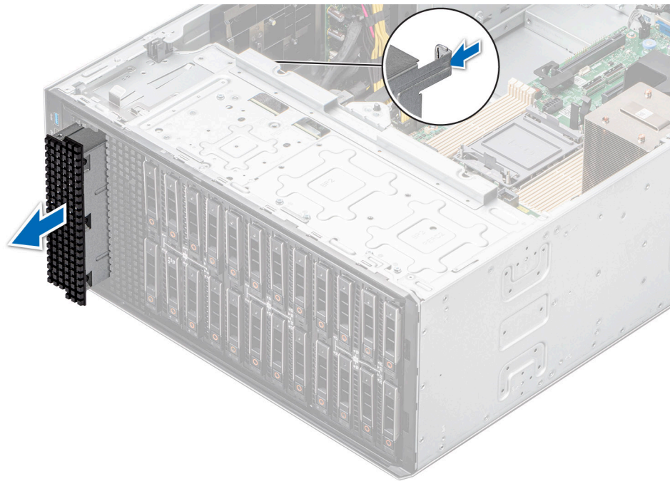
Figure 99. Retrait du cache de l'unité de sauvegarde sur bande
