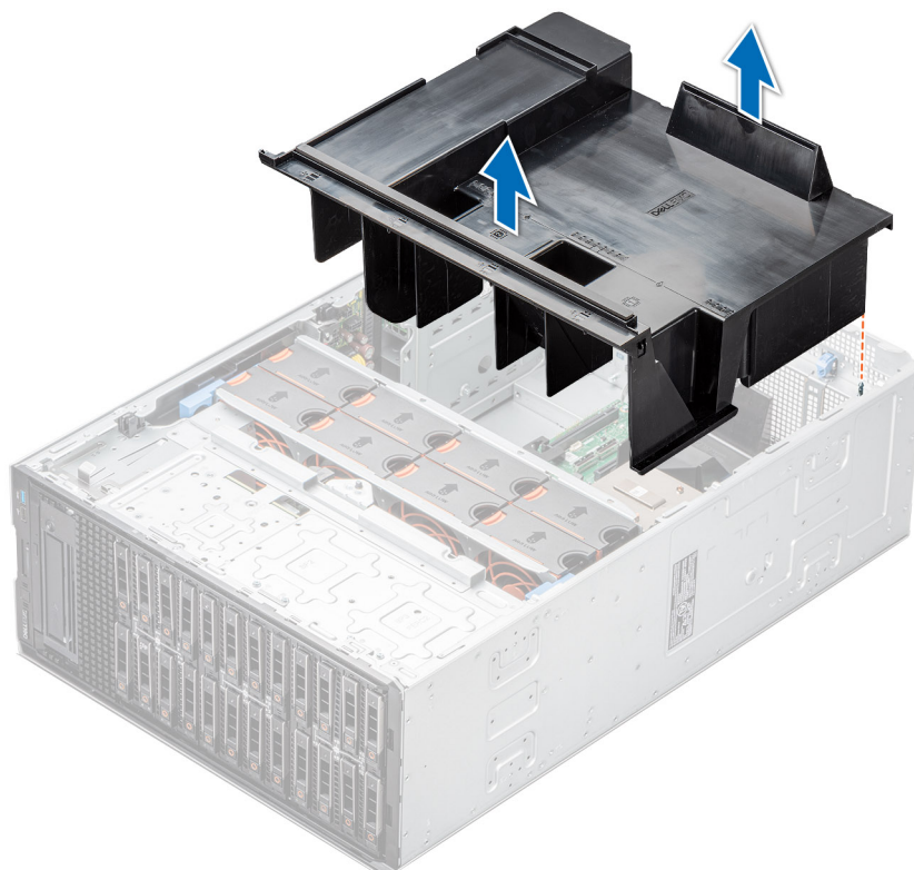
Figure 35. Retrait du carénage d'aération
