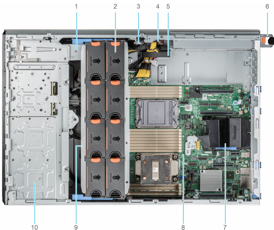
Figure 8. À l'intérieur du système pour une configuration de 24 disques de 2,5 pouces
