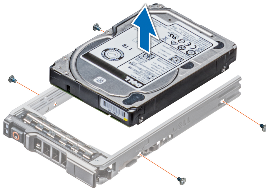
Figure 52. Retrait d'un disque dur installé de son support
