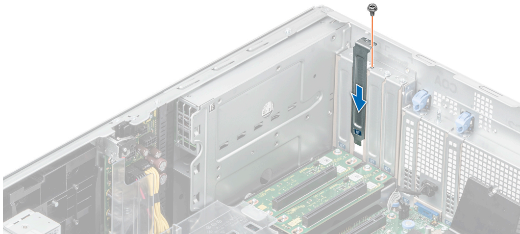
Figure 137. Installation d'une plaque de recouvrement
