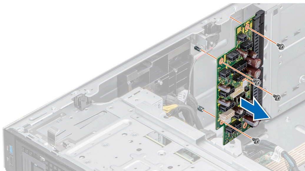
Figure 176. Retrait de la carte PIB
