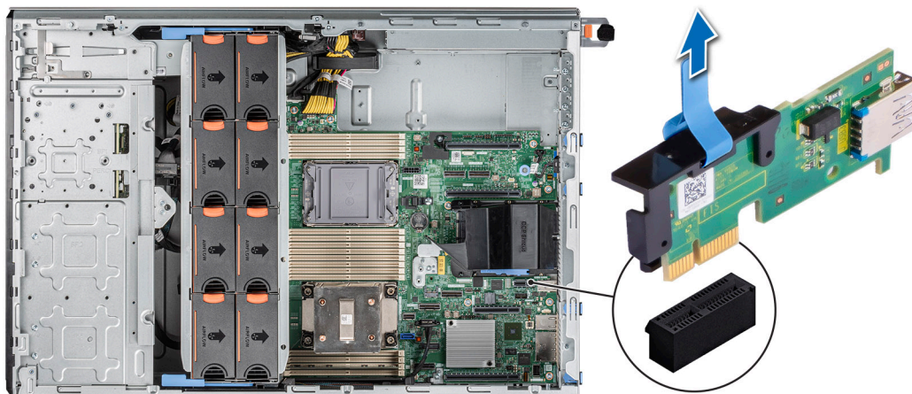
Figure 122. Retrait du module USB interne
