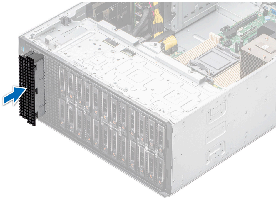
Figure 100. Installation du cache de l'unité de sauvegarde sur bande
