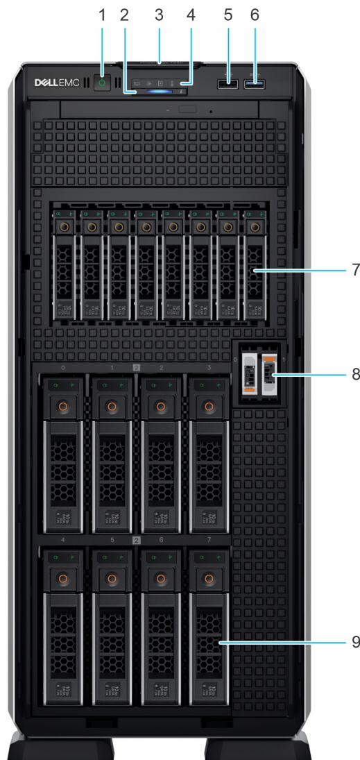
Figure 3. Vue avant du système de 8 disques de 3,5 pouces et de 8 disques de 2,5 pouces
