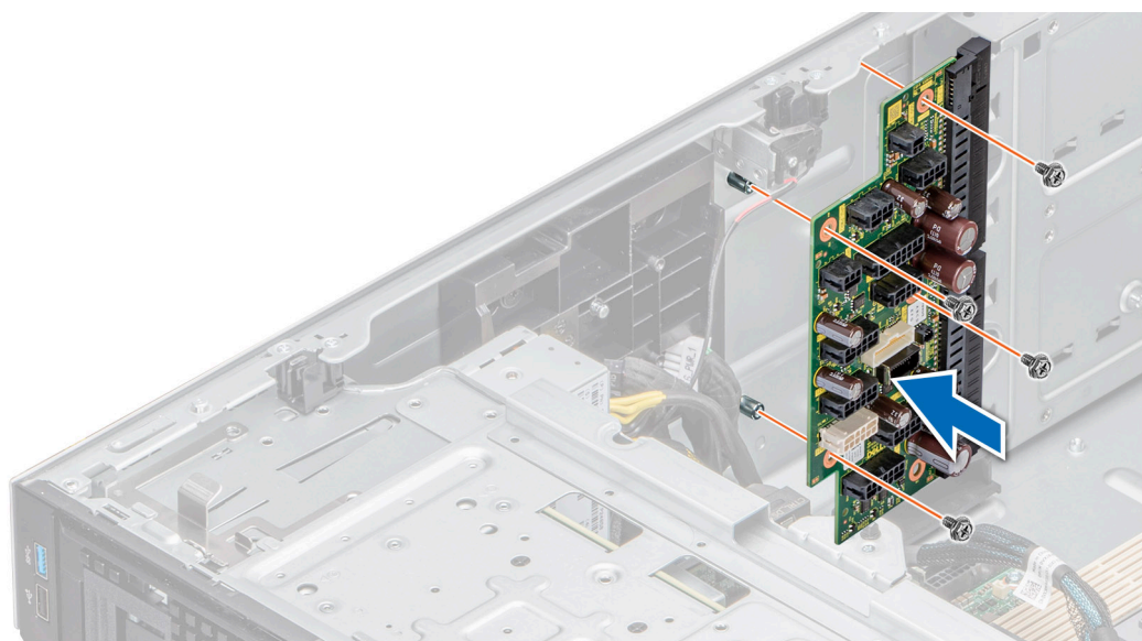
Figure 177. Installation de la carte intercalaire d'alimentation
