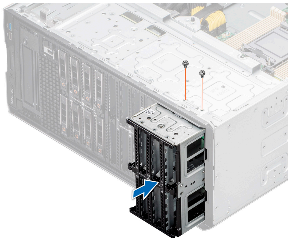
Figure 72. Installation d'une baie de disques
