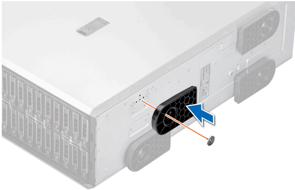
Figure 30. Installation des pieds du système
