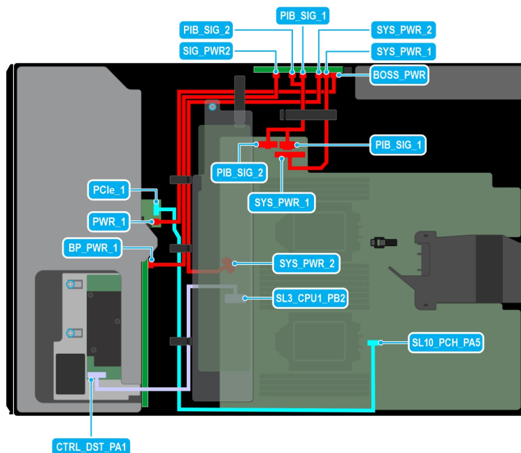
Figure 87. Acheminement des câbles : 8 disques SAS de 3,5 pouces avec module BOSS S2
