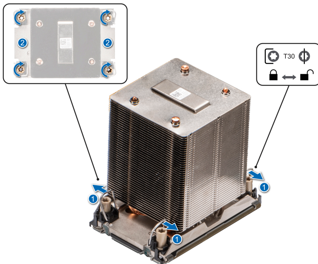
Figure 152. Placement des câbles anti-inclinaison en position verrouillée et serrage des écrous
