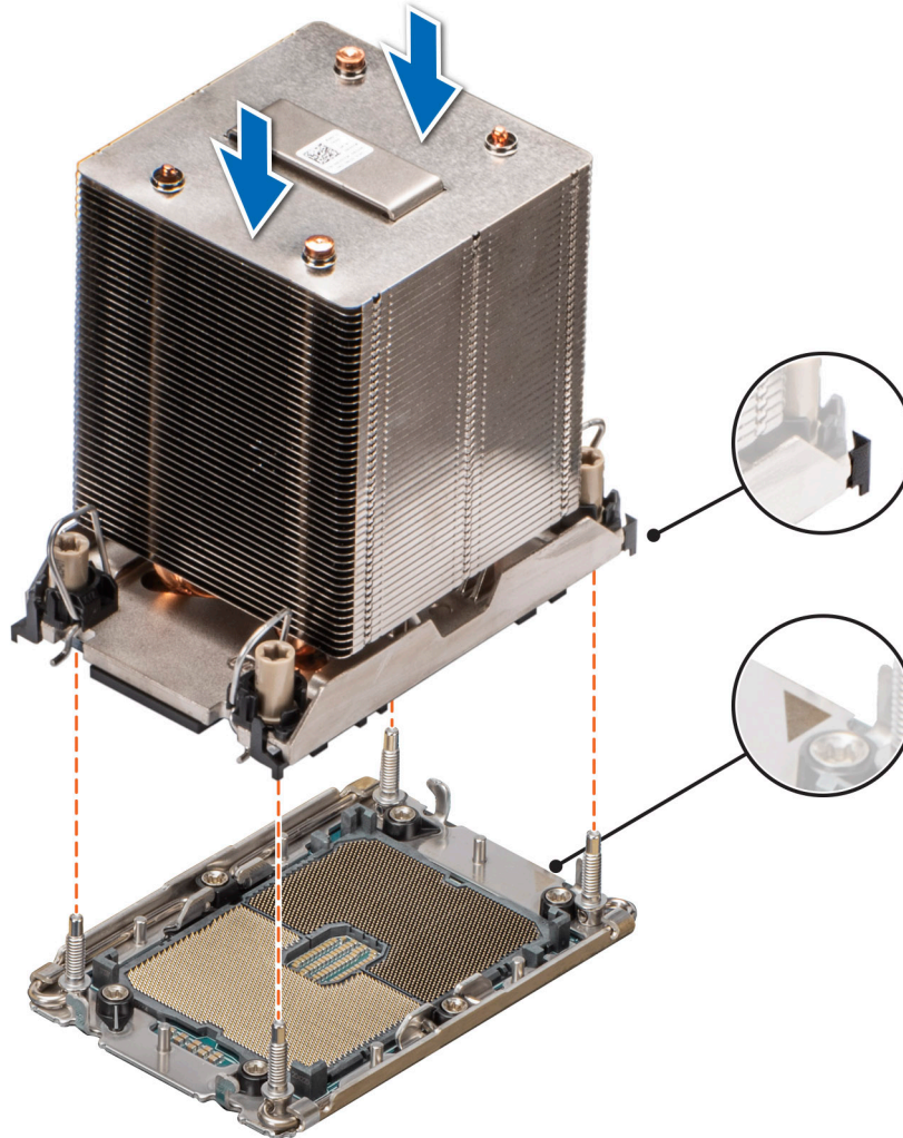
Figure 151. Installation du dissipateur de chaleur du processeur
