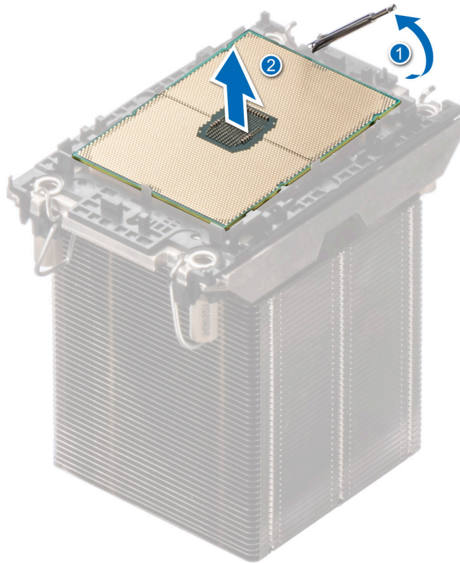
Figure 144. Levage du levier de dégagement du TIM
