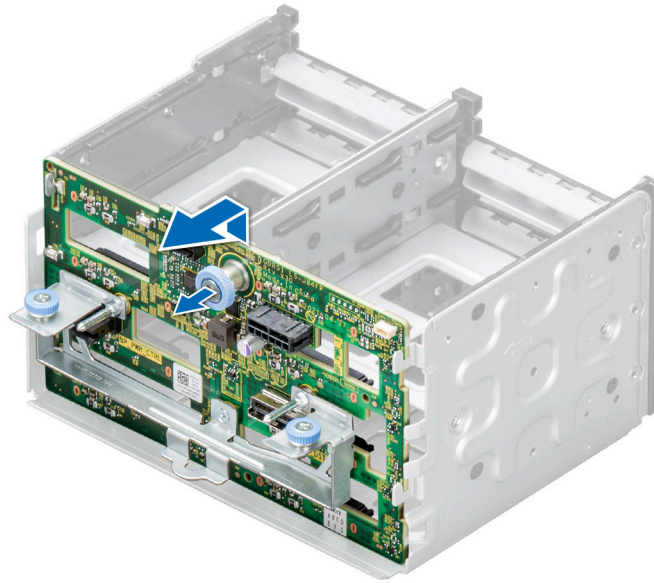
Figure 62. Retrait d'un fond de panier de disque de 2,5 pouces
