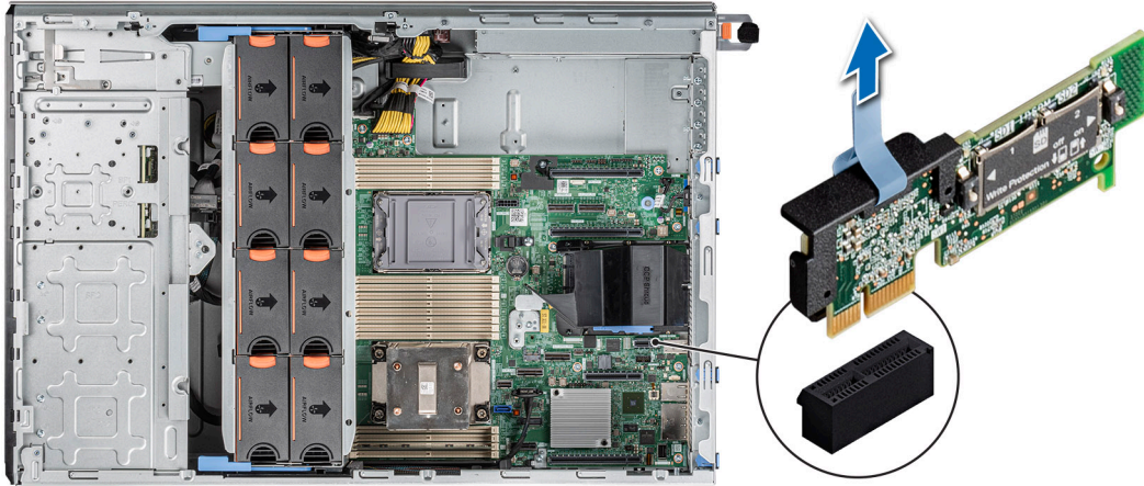
Figure 126. Retrait du module IDSDM
