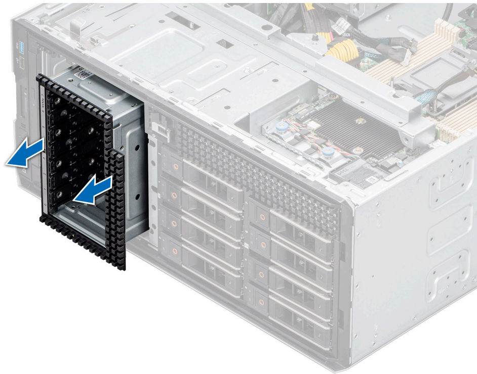
Figure 70. Retrait d'une baie de disques NVMe
