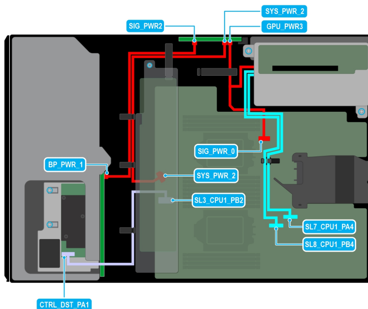
Figure 88. Acheminement des câbles : 8 disques SAS de 3,5 pouces avec carte de montage de processeur graphique
