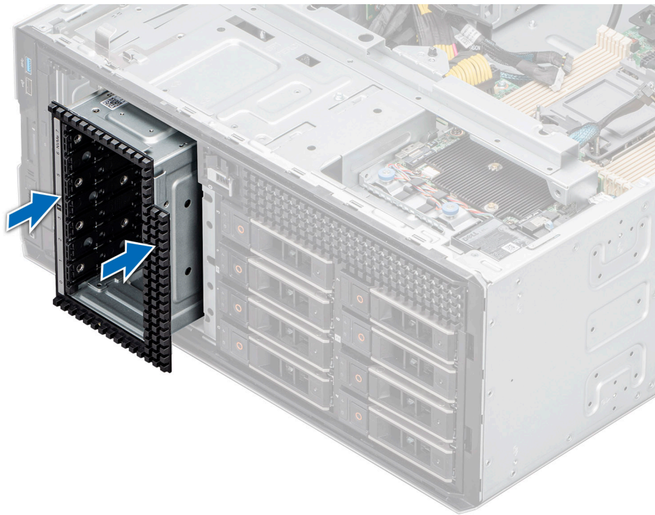
Figure 73. Installation d'une baie de disques NVMe
