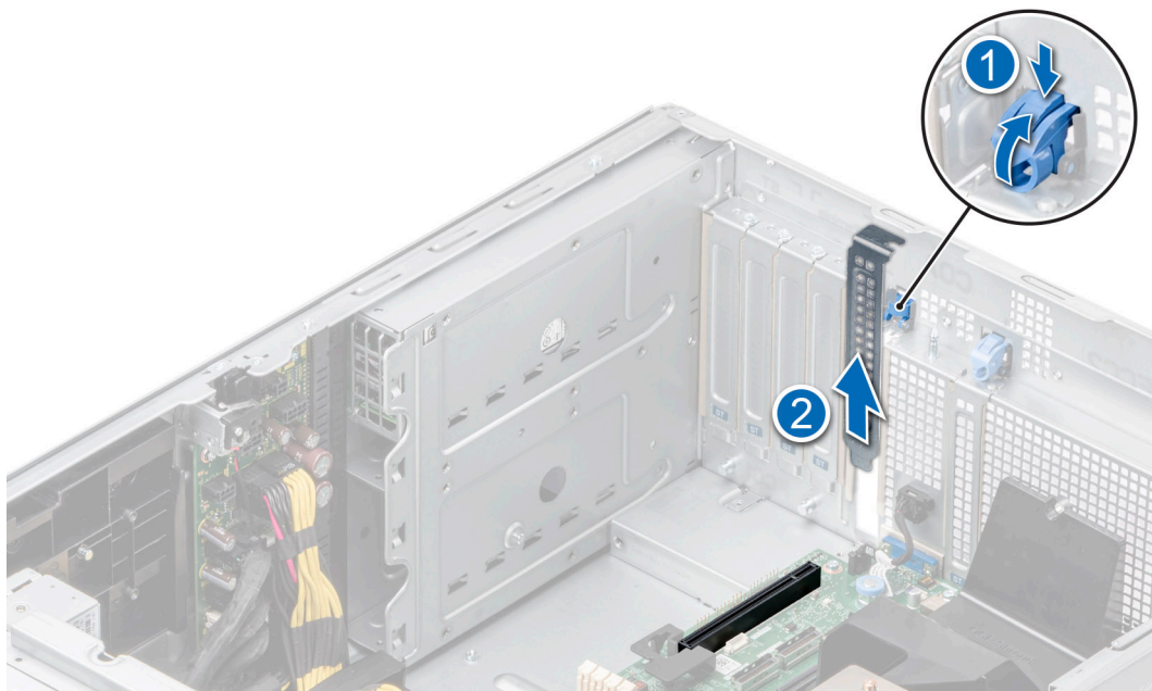
Figure 132. Retrait de la plaque de recouvrement
