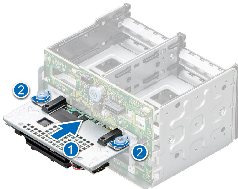
Figure 47. Installation du module PERC avant pour fond de panier de disque de 2,5 pouces.
