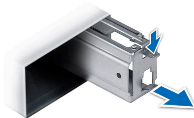
Figure 169. Retrait d'un adaptateur de bloc d'alimentation
