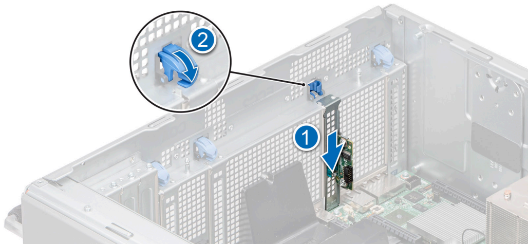
Figure 160. Installation du port série COM
