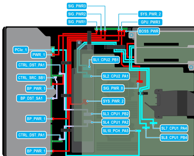
Figure 85. Acheminement des câbles : 24 disques SAS de 2,5 pouces avec deux cartes de montage de processeur graphique
