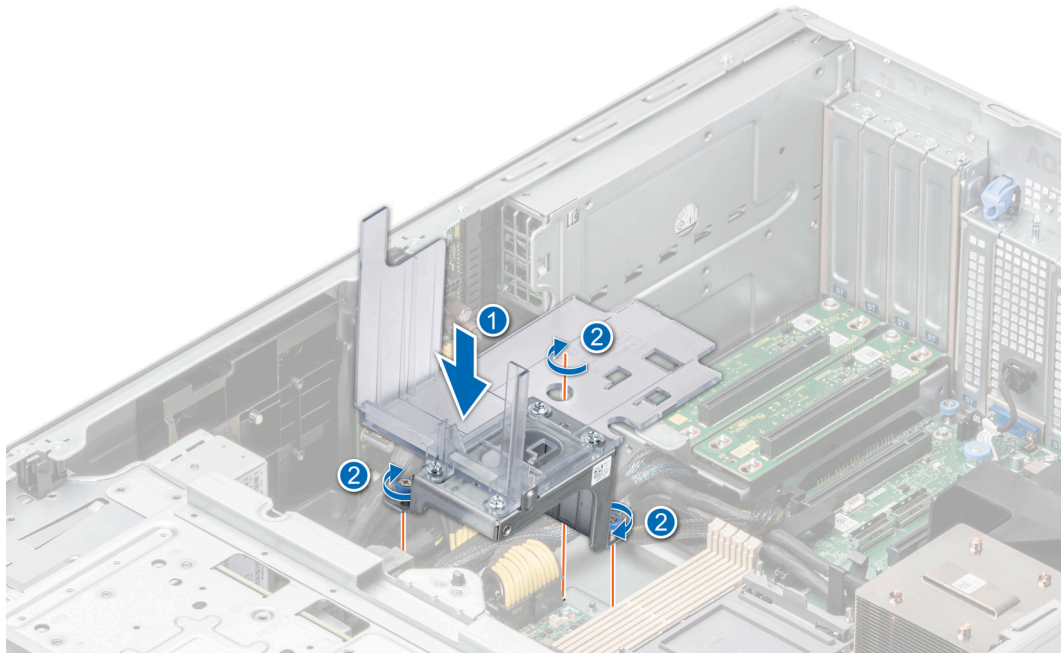
Figure 135. Installation du support de la carte de processeur graphique
