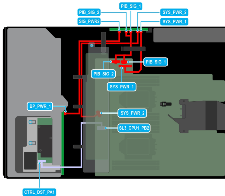
Figure 86. Acheminement des câbles : 8 disques SAS de 3,5 pouces
