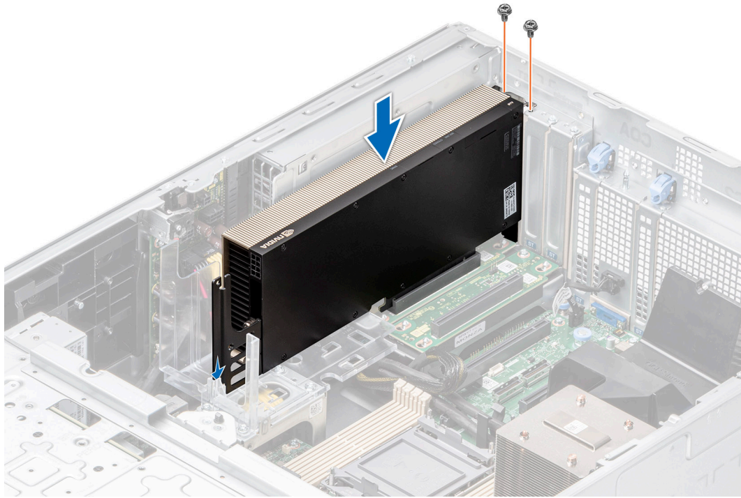
Figure 139. Installation de la carte de processeur graphique
