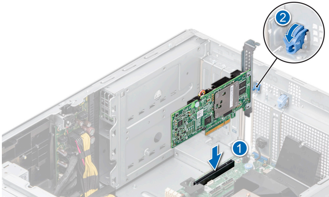
Figure 133. Installation d'une carte d'extension
