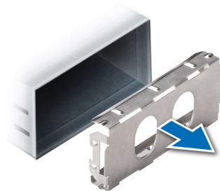
Figure 166. Retrait du cache du bloc d'alimentation 86 mm
