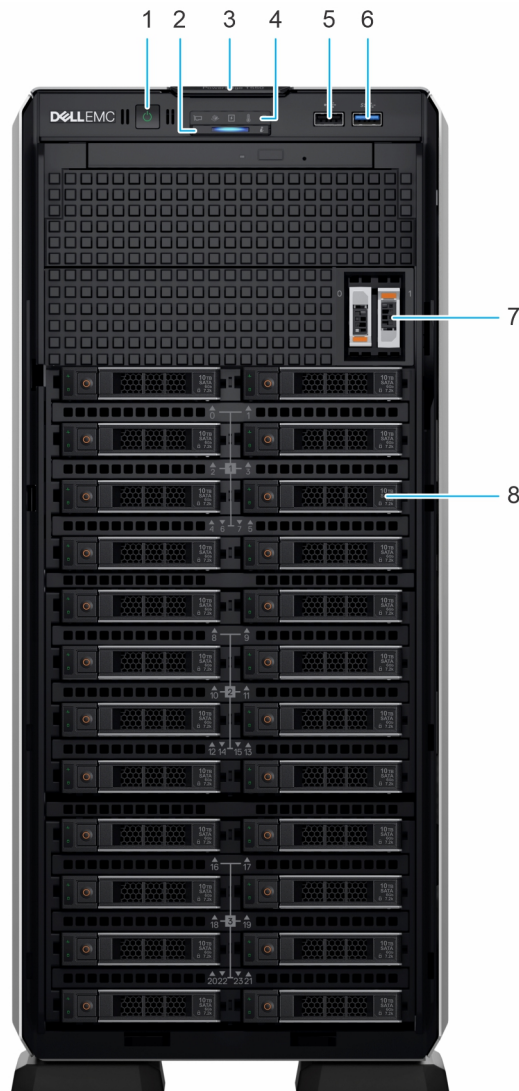
Figure 1. Vue avant du système de 24 disques de 2,5 pouces
