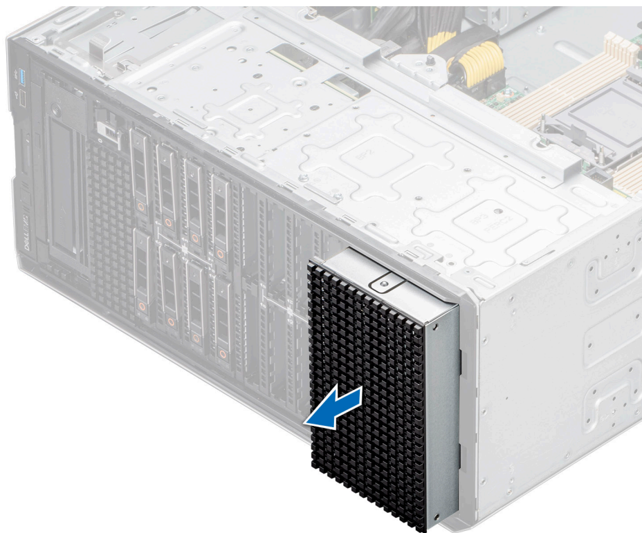
Figure 65. Retrait du cache du bâti de la baie de disques
