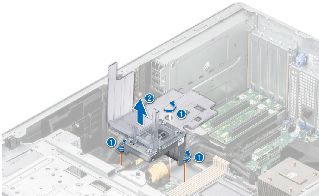
Figure 134. Retrait du support de carte de processeur graphique
