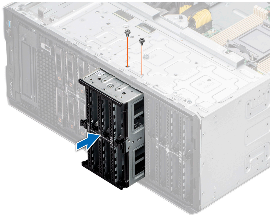
Figure 71. Installation d'une baie de disques
