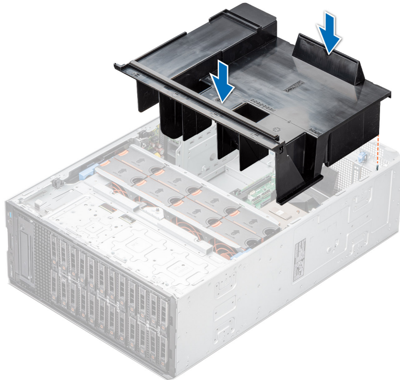
Figure 36. Installation du carénage d'aération
