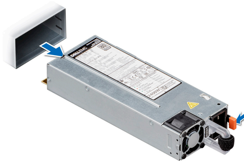
Figure 172. Retrait d'un bloc d'alimentation 86 mm
