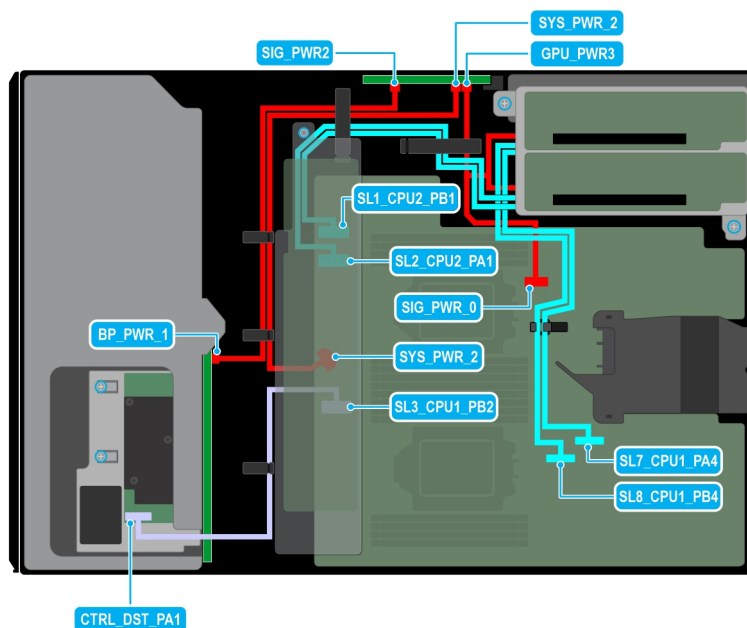
Figure 89. Acheminement des câbles : 8 disques SAS de 3,5 pouces avec deux cartes de montage du processeur graphique
