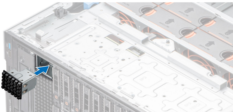
Figure 112. Installation du cache du module BOSS S2
