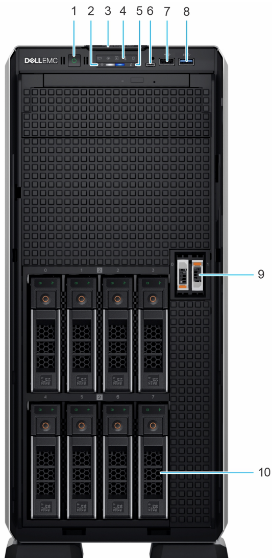
Figure 5. Vue avant d'un système de 8 disques de 3,5 pouces (configuration de vente incitative)
