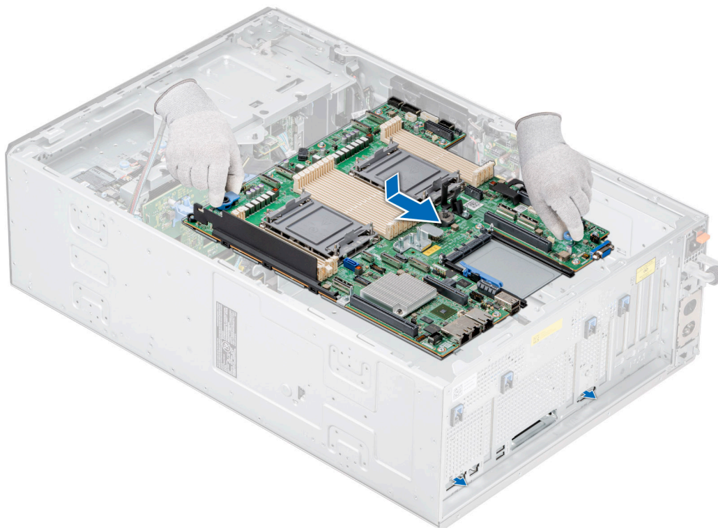
Figure 179. Installation de la carte système
