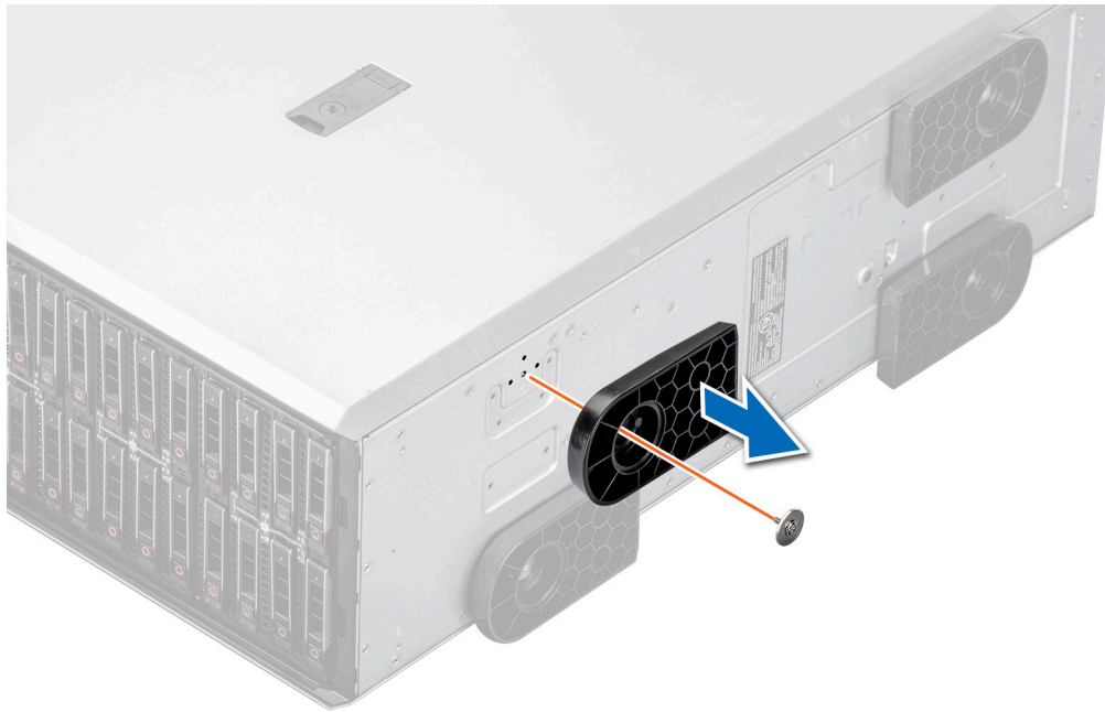
Figure 29. Retrait des pieds du système
