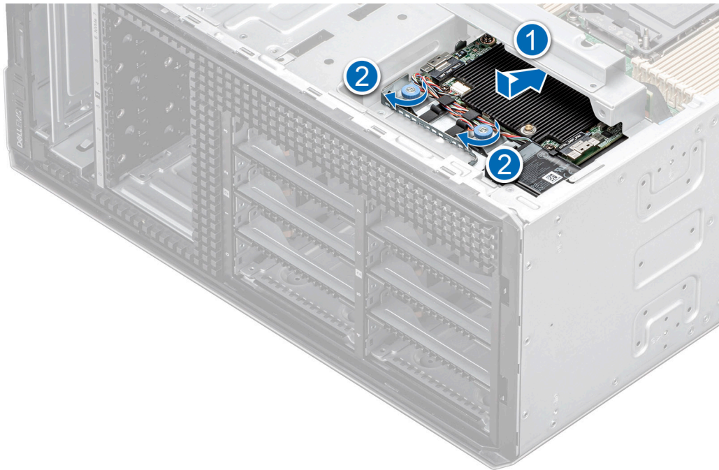
Figure 46. Installation du module PERC avant pour fond de panier de disque de 3,5 pouces.
