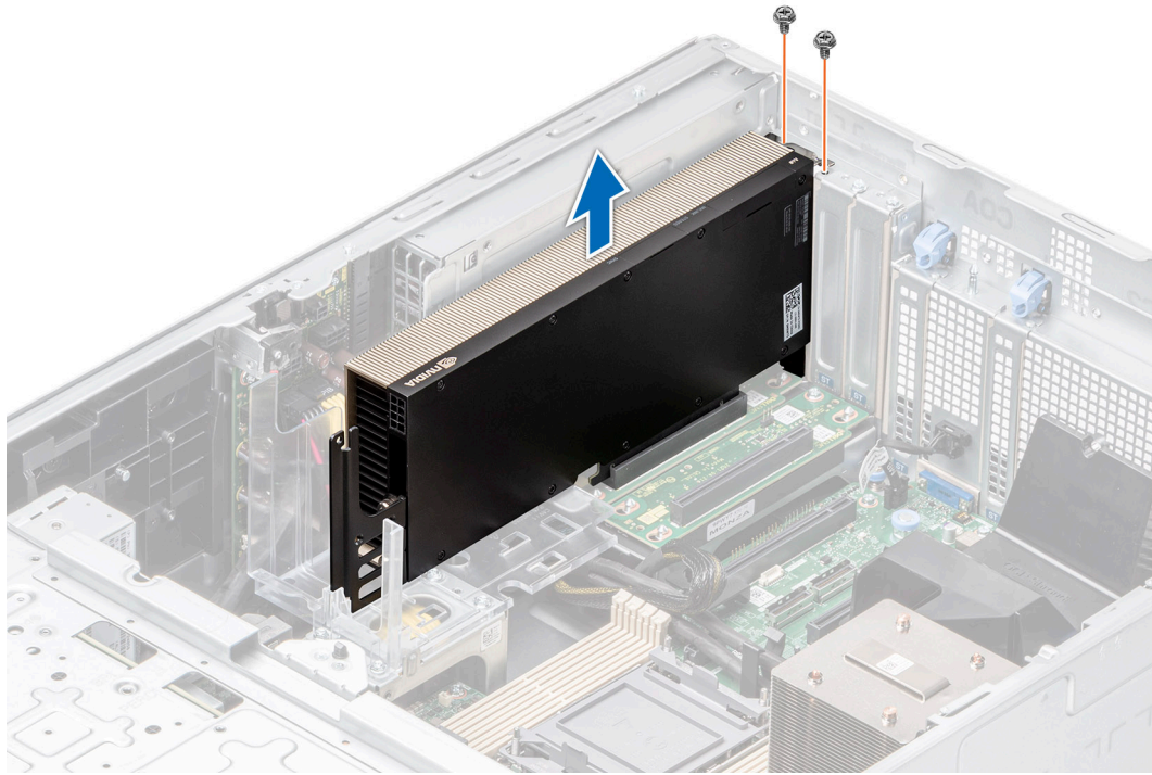
Figure 136. Retrait de la carte GPU
