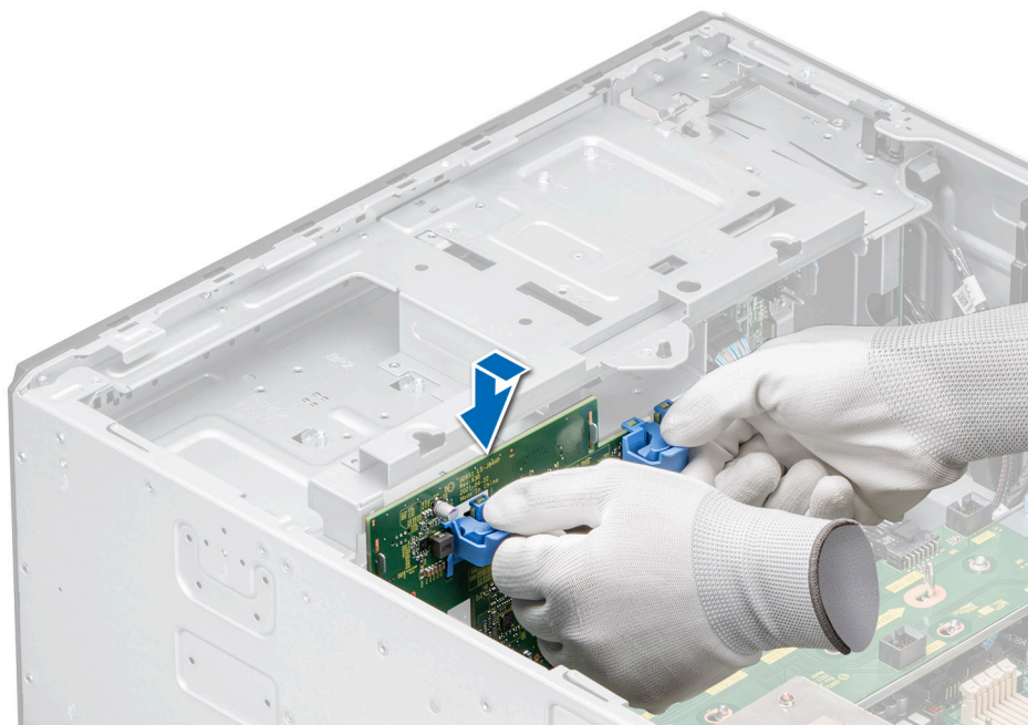
Figure 61. Installation du fond de panier du disque de 3,5 pouces
