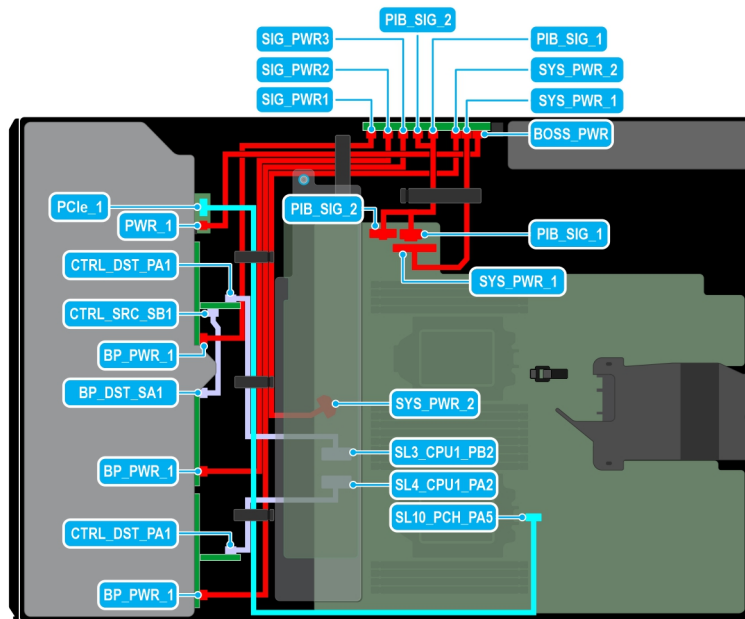
Figure 83. Acheminement des câbles : 24 disques SAS de 2,5 pouces avec module BOSS S2
