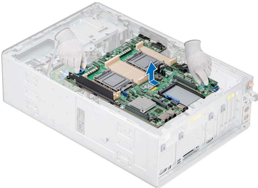
Figure 178. Retrait de la carte système
