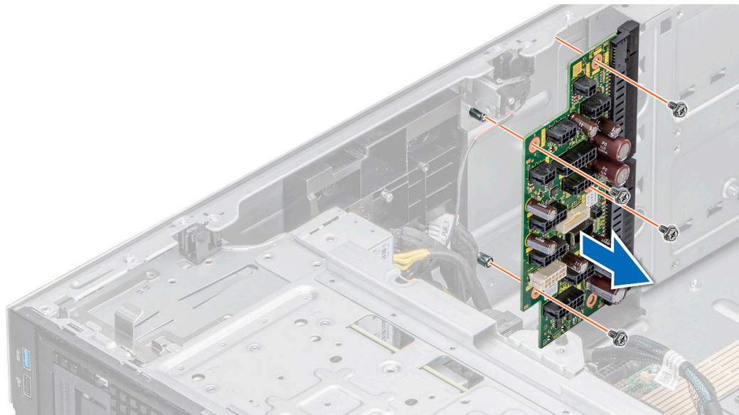
Abbildung 176. Entfernen der PIB
