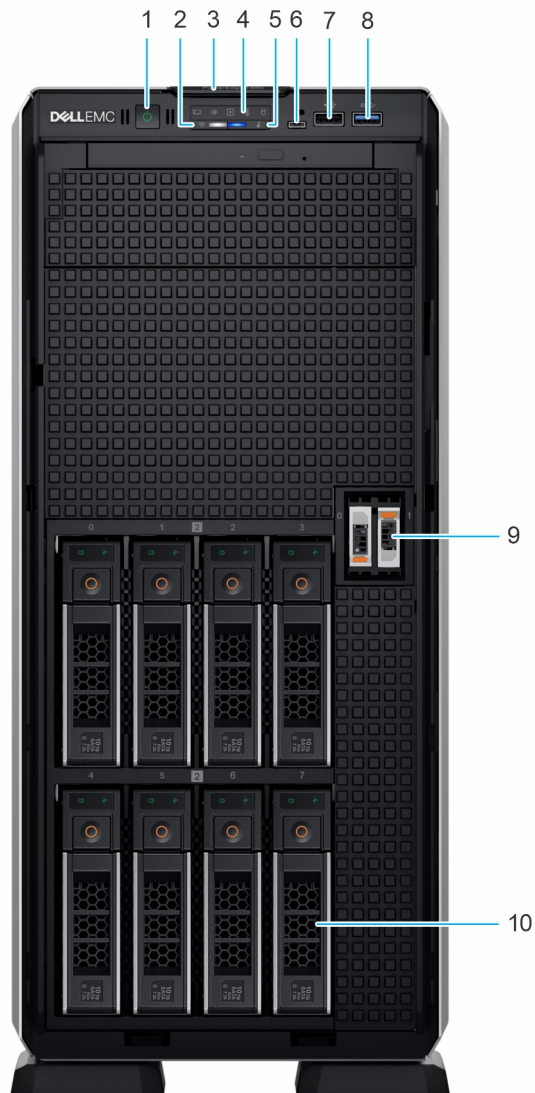
Abbildung 5. Vorderansicht eines Systems mit 8 x 3,5-Zoll-Laufwerken (Upsell-Konfiguration)
