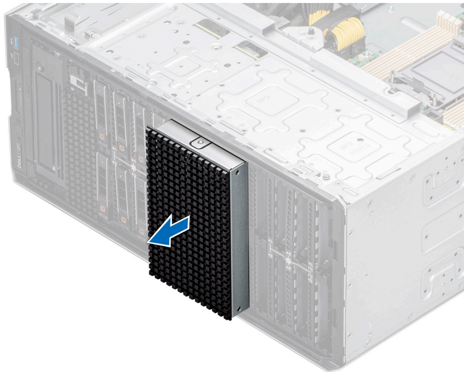
Abbildung 64. Entfernen des Platzhalters für das Laufwerkschachtgehäuse
