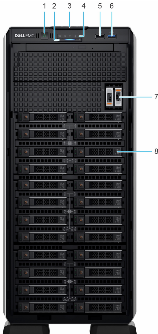
Abbildung 1. Vorderansicht eines Systems mit 24 x 2,5“-Laufwerken
