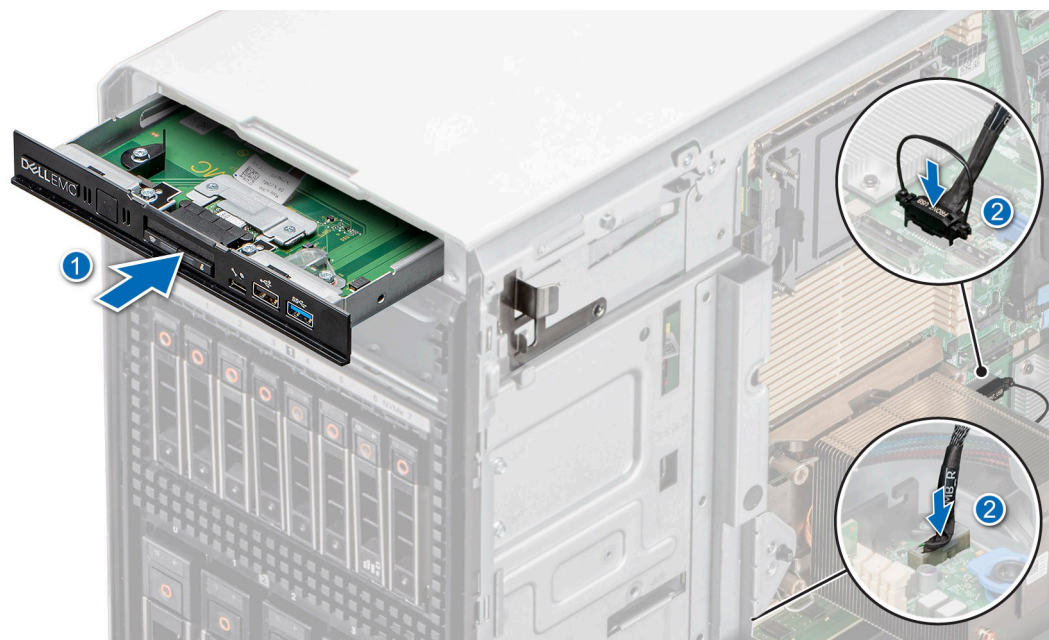
Abbildung 106. Installieren des vorderen E/A-Moduls für die Upsell-Konfiguration
