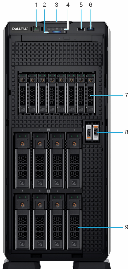
Abbildung 3. Vorderansicht eines Systems mit 8 x 3,5-Zoll- und 8 x 2,5-Zoll-Laufwerken
