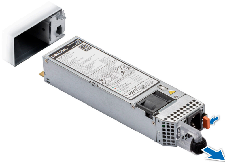
Abbildung 171. Entfernen eines 60-mm-Netzteils
