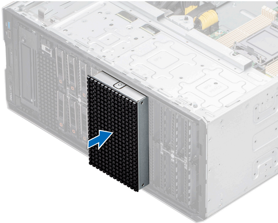
Abbildung 66. Installieren des Platzhalters für das Laufwerkschachtgehäuse
