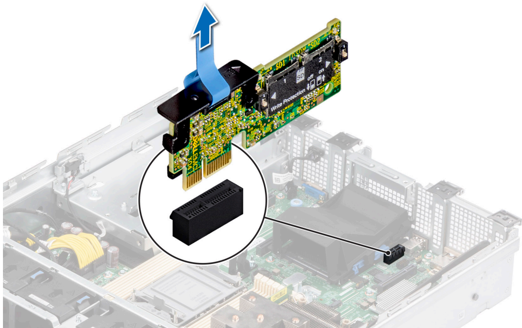
Figure 72. Retrait du module IDSDM
