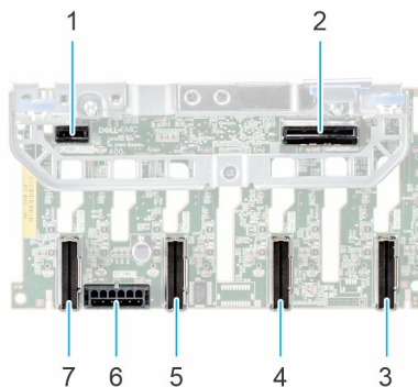
Figure 47. Fond de panier NVMe de 8 disques de 2,5 pouces
