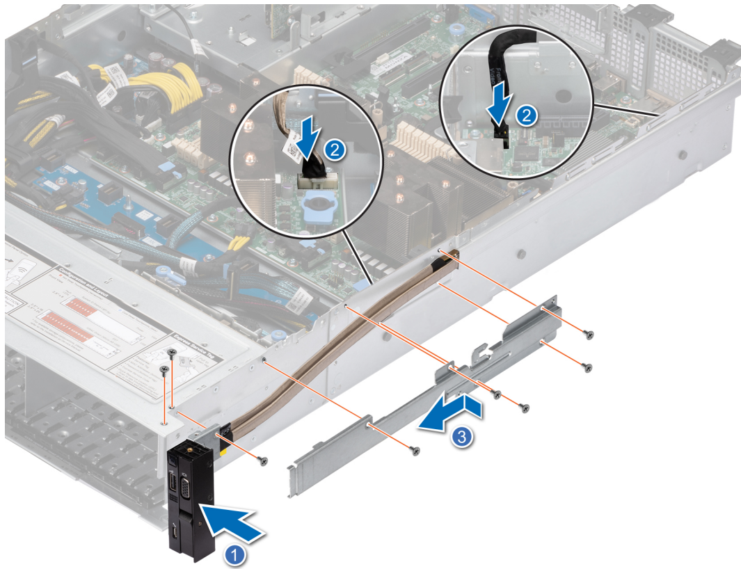
Figure 132. Installation du panneau de configuration droit
