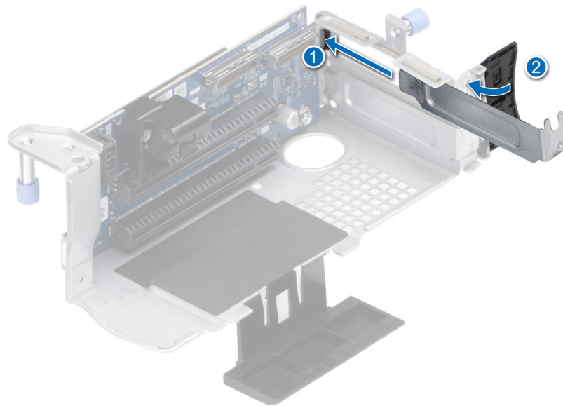
Figure 86. Installation de la plaque de recouvrement dans les cartes de montage 1A et 1B
