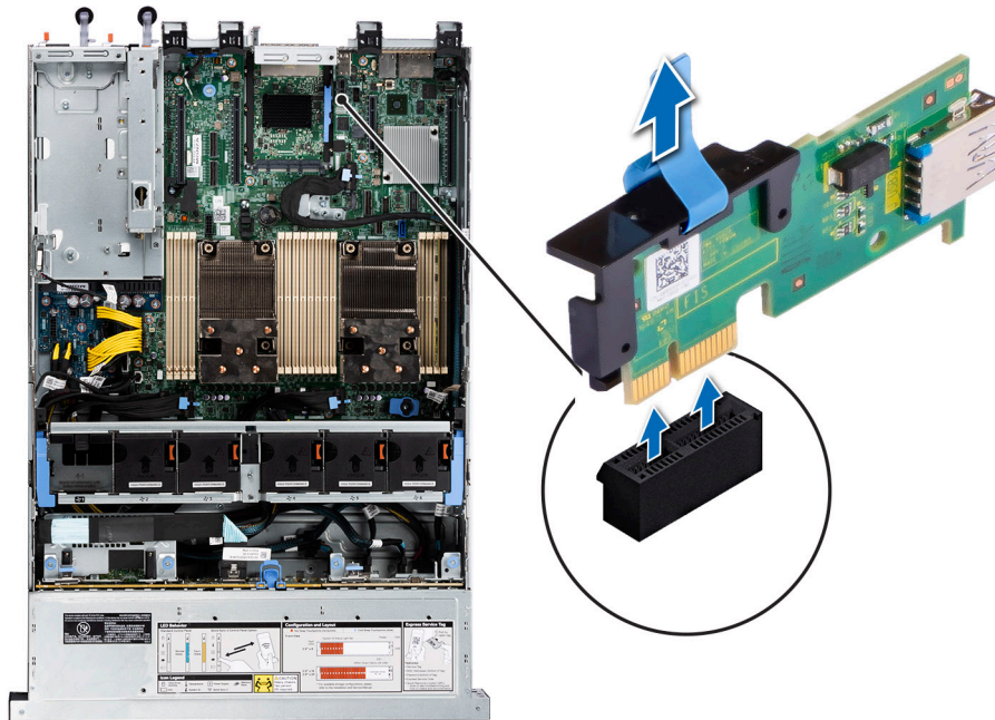
Figure 118. Retrait de la carte USB interne
