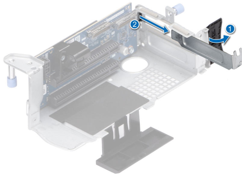
Figure 87. Retrait d'une plaque de recouvrement des cartes de montage 1A et 1B
