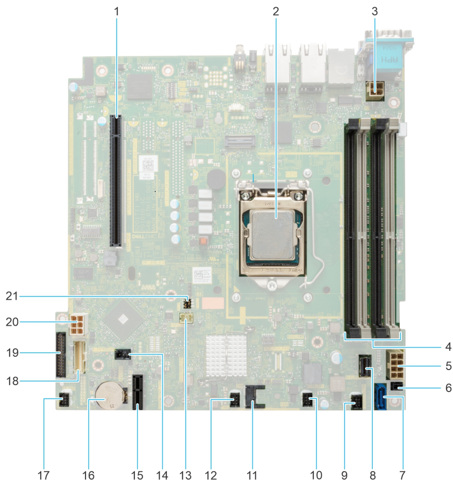
Abbildung 78. Jumper und Anschlüsse auf der Systemplatine
