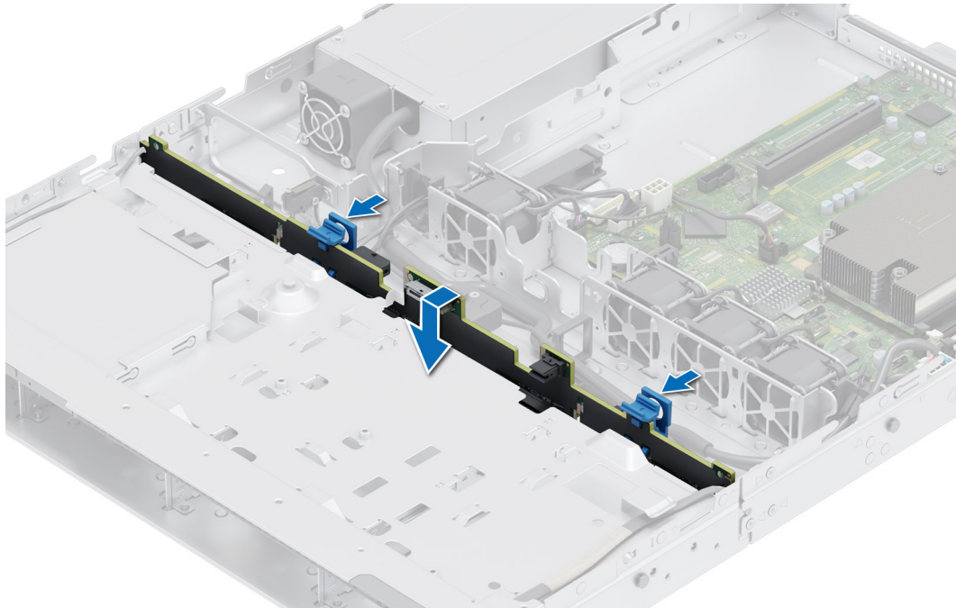
Abbildung 25. Laufwerkrückwandplatine installieren
