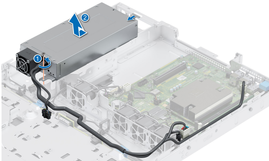
Abbildung 69. Entfernen des verkabelten Netzteils
