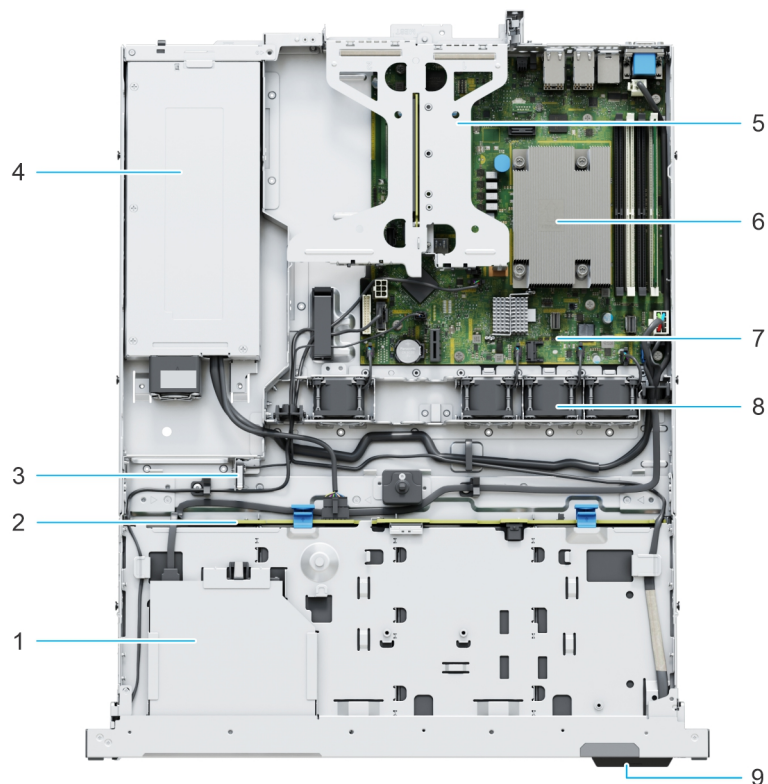
Abbildung 5. Innenansicht des Systems mit Rückwandplatine
