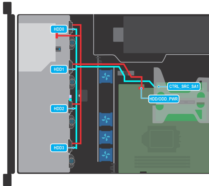
Abbildung 37. Kabelführung – Konfiguration mit 4 verkabelten 3,5-Zoll-Laufwerken mit PERC
