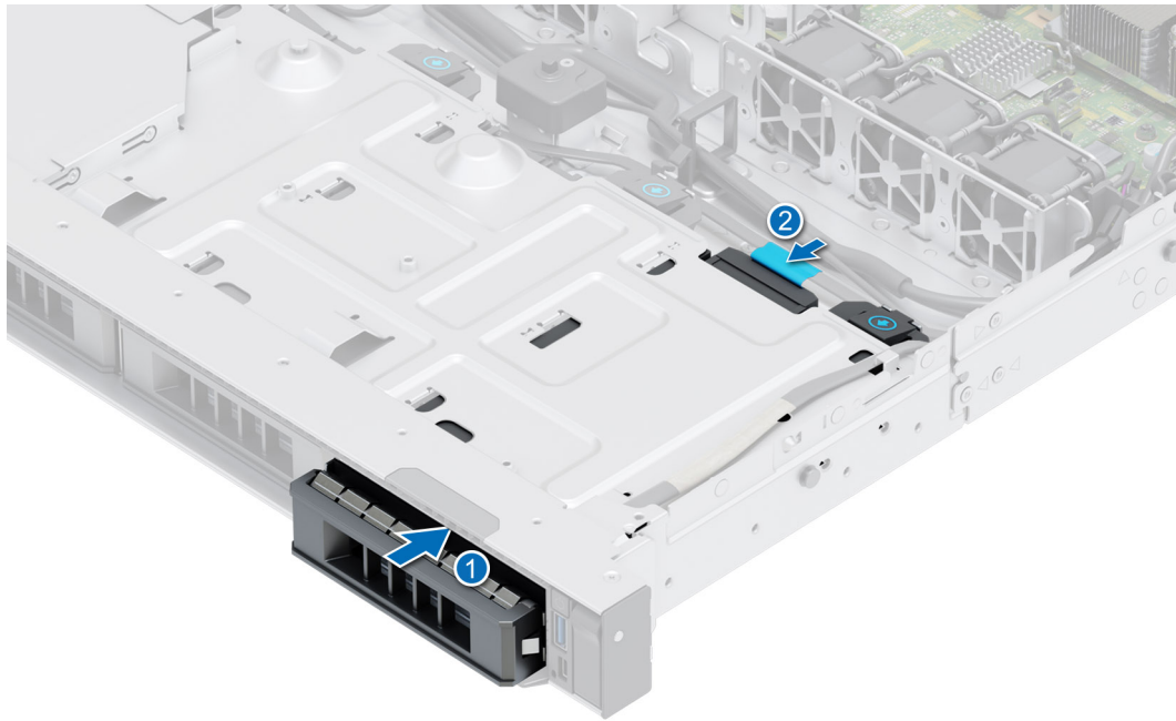
Abbildung 29. Einbauen des verkabelten Laufwerks
