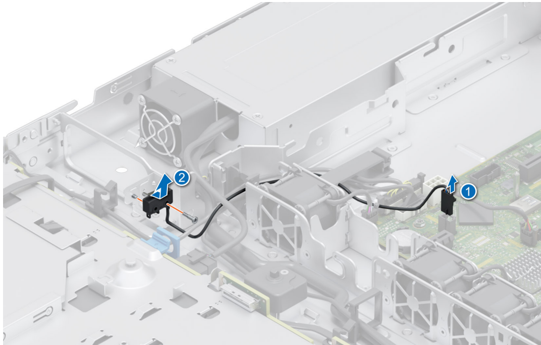
Abbildung 21. Entfernen des Eingriffsschaltermoduls
