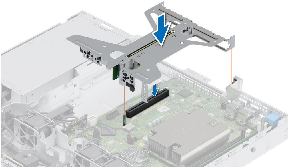
Abbildung 52. Installieren des Risers
