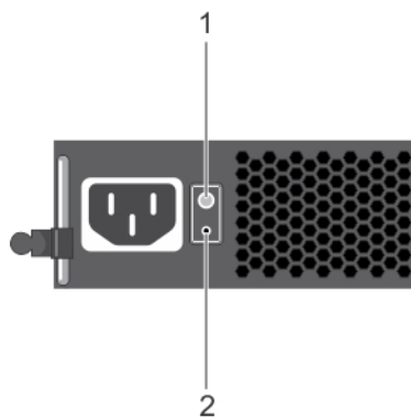
Abbildung 79. Statusanzeige und Selbstdiagnosetaste eines nicht redundanten verkabelten Wechselstrom-Netzteils
