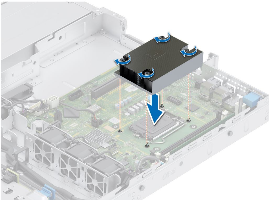
Abbildung 47. Einsetzen des Kühlkörpers
