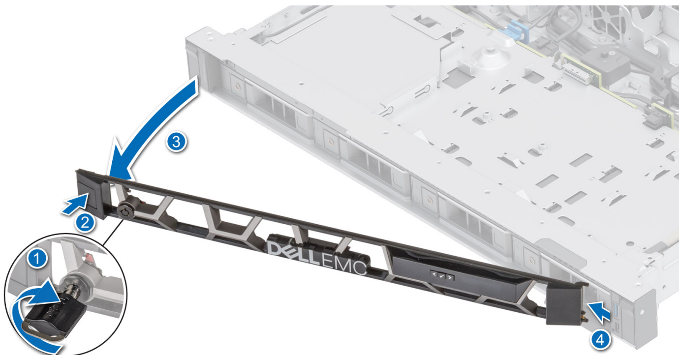
Abbildung 11. Entfernen der Frontblende mit LCD-Display
