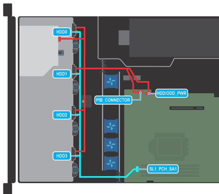
Abbildung 36. Kabelführung – Konfiguration mit 4 verkabelten 3,5-Zoll-Laufwerken
