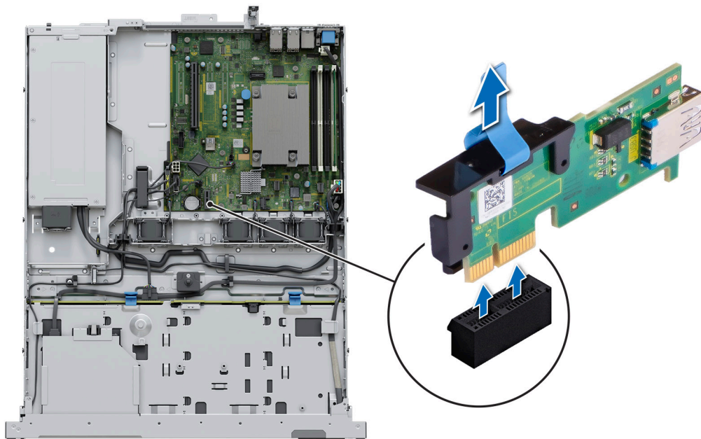
Abbildung 67. Entfernen der internen USB-Karte
