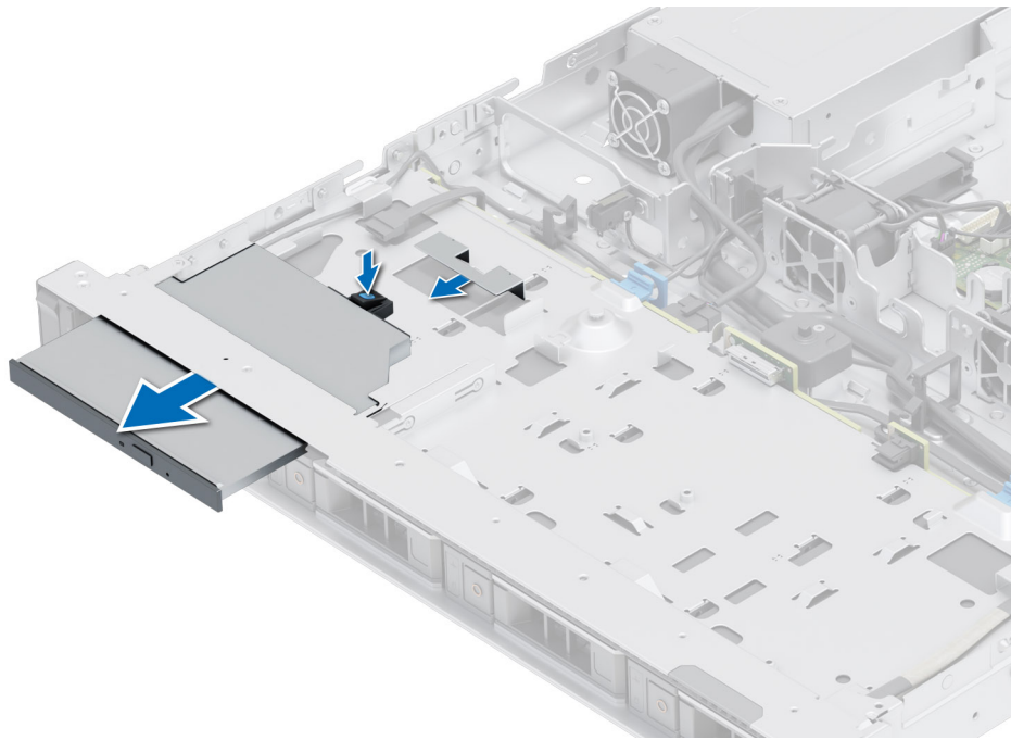
Abbildung 15. Entfernen des optischen Laufwerks
