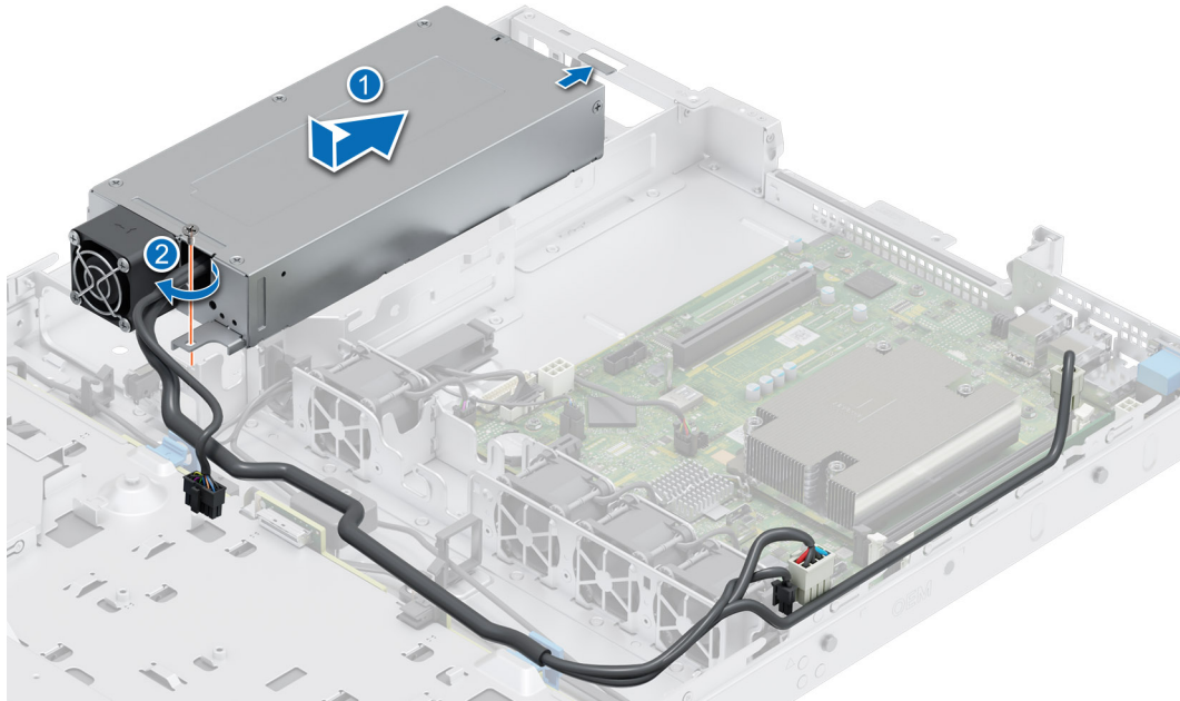
Abbildung 70. Installieren des verkabelten Netzteils
