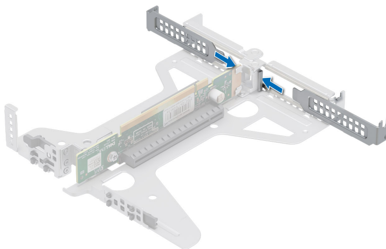
Abbildung 51. Einsetzen des Abdeckblechs
