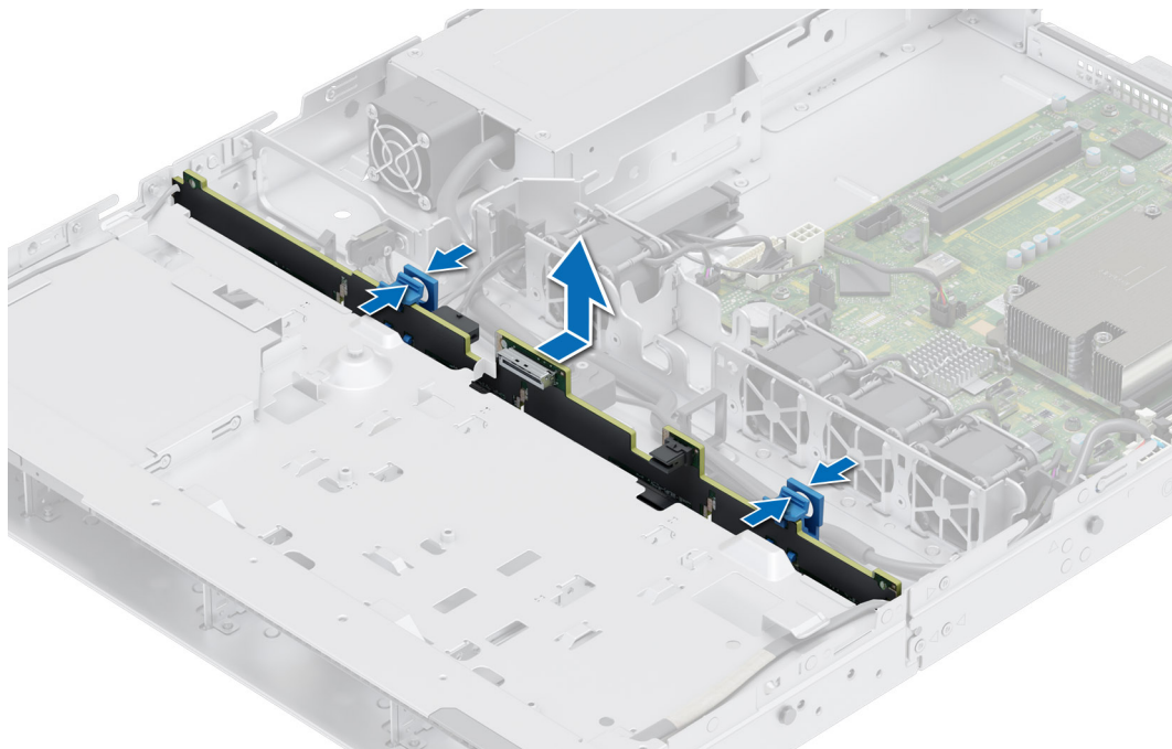
Abbildung 24. Entfernen der Rückwandplatine
