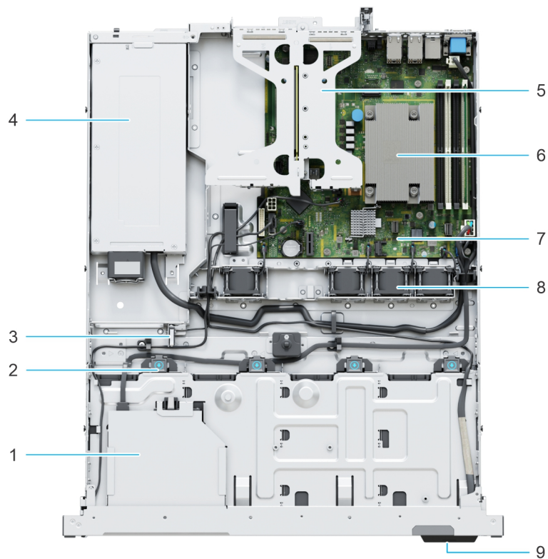
Abbildung 6. Innenansicht des verkabelten Laufwerksystems
