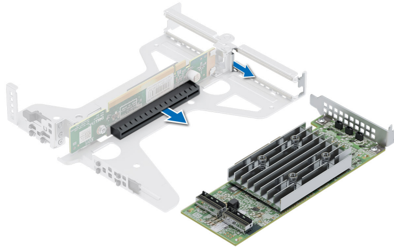
Abbildung 64. Installieren des Adapter-PERC
