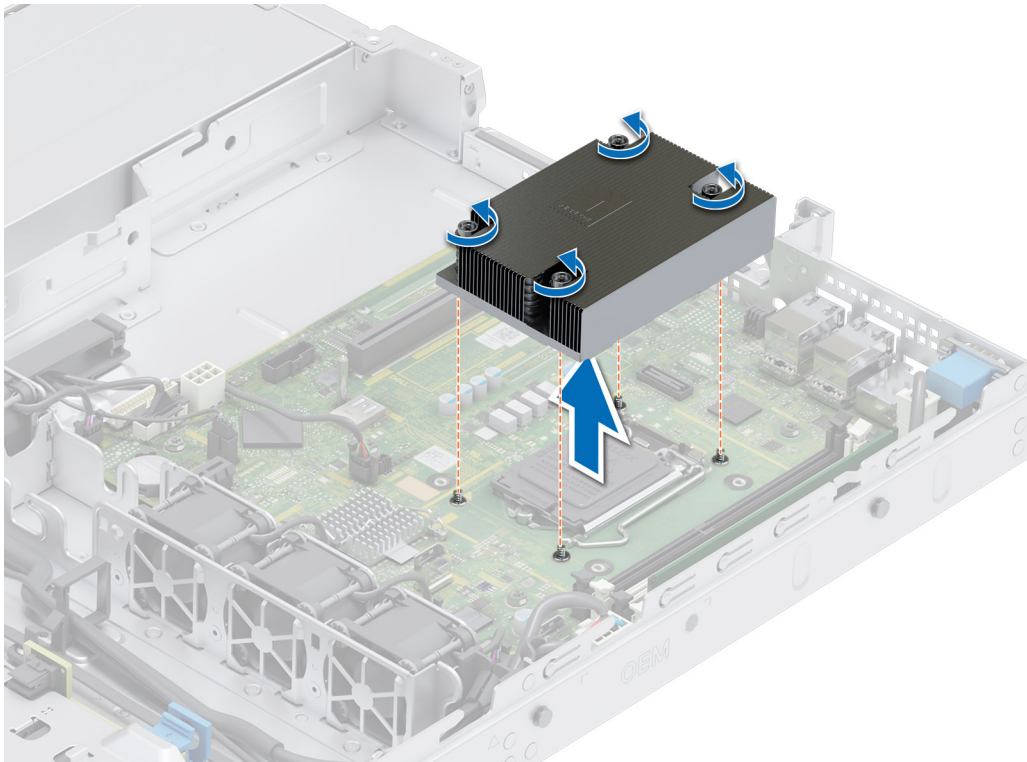
Abbildung 43. Entfernen eines Kühlkörpers
