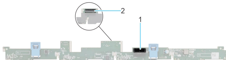
Abbildung 23. 4 x 3,5-Zoll-Laufwerkrückwandplatine
