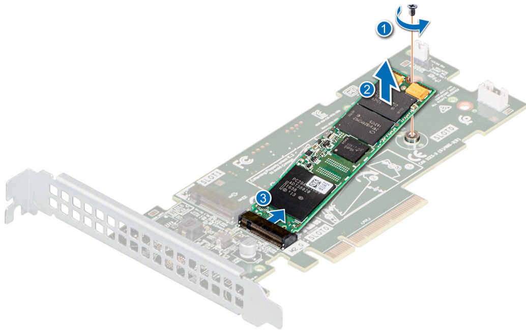
Abbildung 61. Entfernen der M.2-SSD aus dem BOSS-S1-Kartenträger
