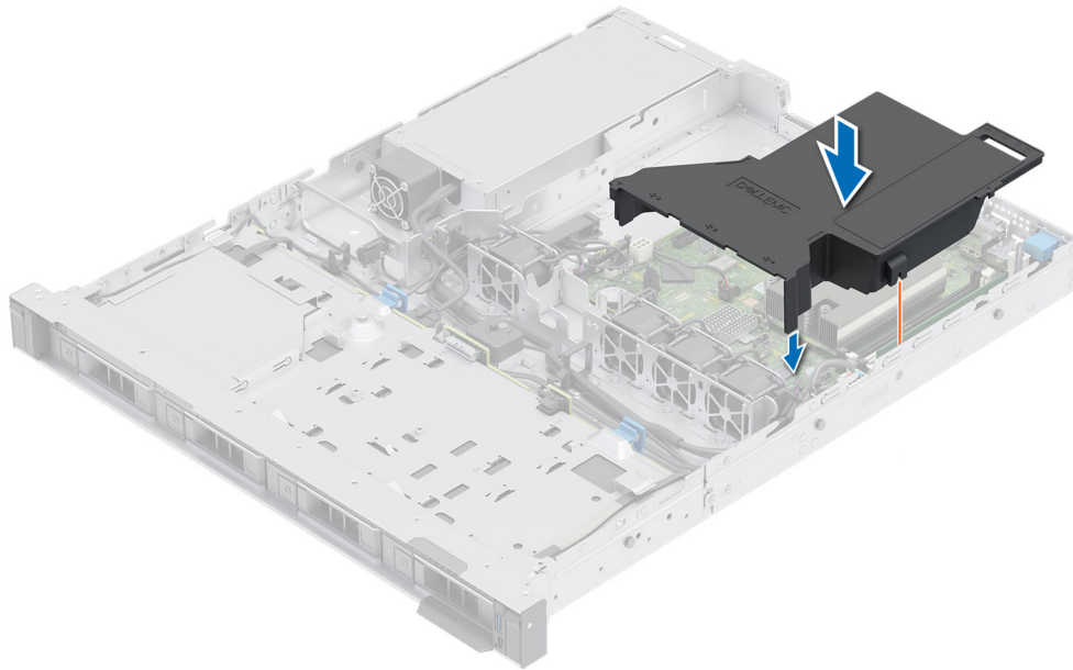
Abbildung 18. Luftstromverkleidung einbauen
