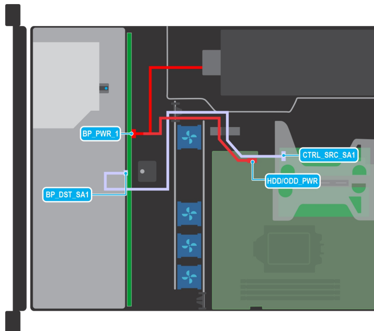
Abbildung 34. Kabelführung – 4 x 3,5-Zoll-Rückwandplattenkonfiguration mit PERC-Adapter
