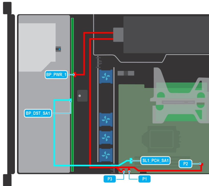
Abbildung 35. Kabelführung für 4 x 3,5-Zoll-Rückwandplattenkonfiguration mit integriertem SATA und Netzteil (Bronze)
