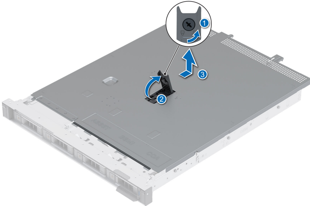
Abbildung 13. Systemabdeckung entfernen
