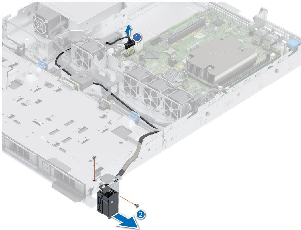
Abbildung 76. Entfernen des rechten Bedienfelds
