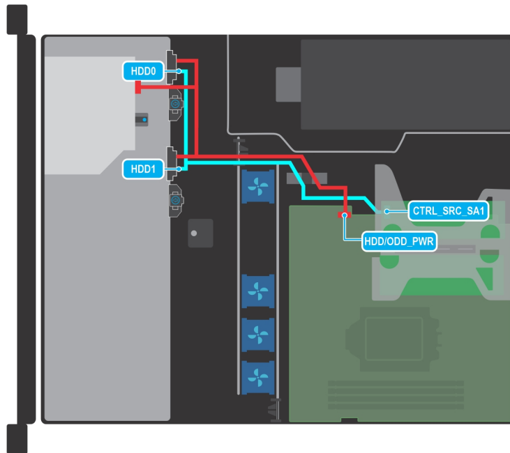
Abbildung 38. Kabelführung – Konfiguration mit 2 verkabelten 3,5-Zoll-Laufwerken mit PERC
