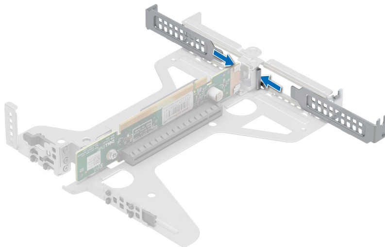
Abbildung 54. Einsetzen des Abdeckblechs in den Riser
