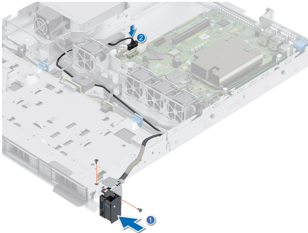
Abbildung 77. Installieren des rechten Bedienfelds
