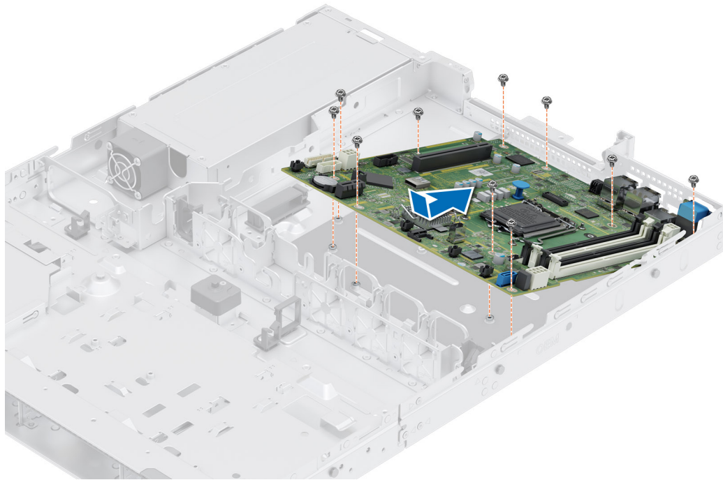
Abbildung 72. Einbauen der Systemplatine
