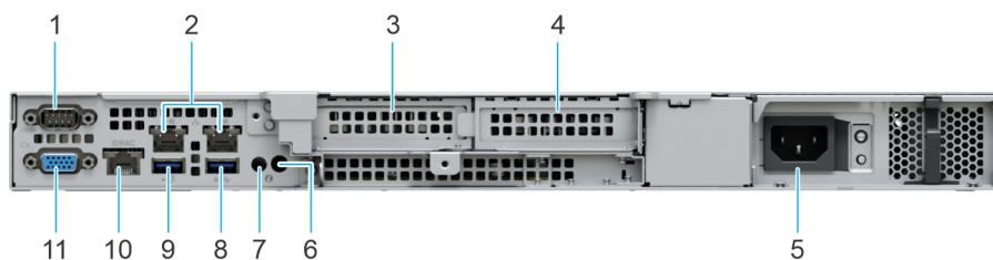
Abbildung 4. Rückansicht des Systems
