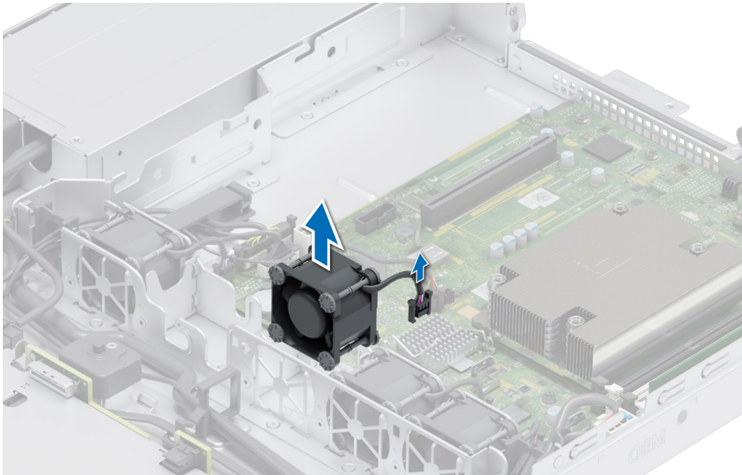
Abbildung 19. Entfernen eines Kühlungslüfters
