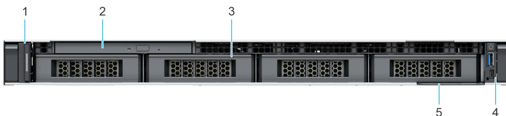
Abbildung 2. Vorderansicht eines Systems mit 4 x 3,5-Zoll-SAS/SATA-Laufwerk (Hot-Swap-fähig)
