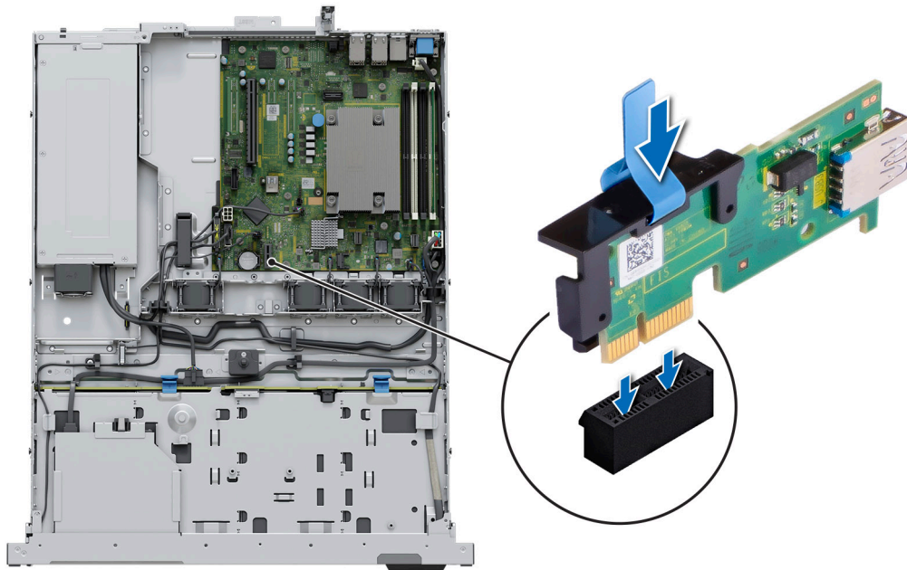
Abbildung 68. Installieren des internen USB-Sticks
