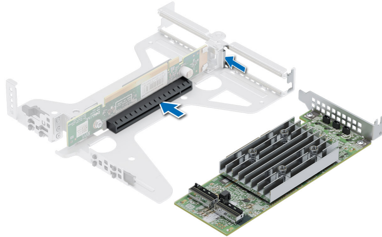
Abbildung 63. Entfernen des Adapter-PERC
