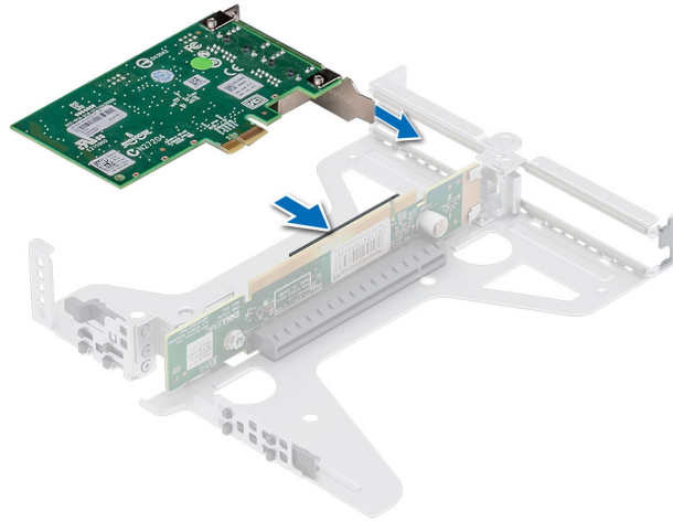
Abbildung 56. Installieren der Erweiterungskarte
