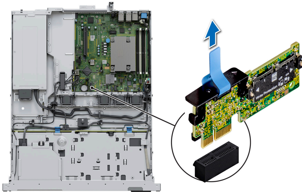
Abbildung 57. Entfernen des IDSDM-Moduls
