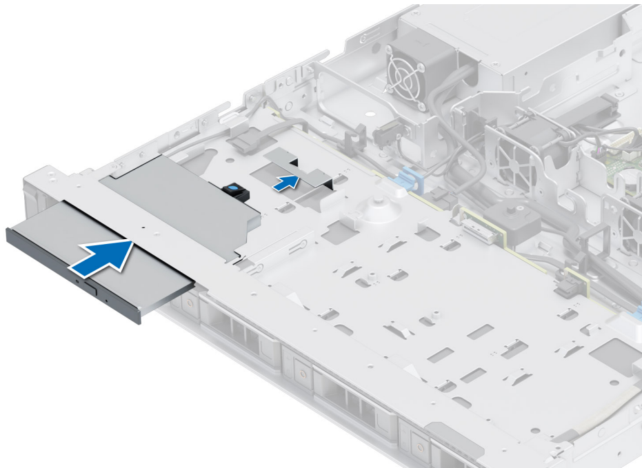
Abbildung 16. Installieren des optischen Laufwerks
