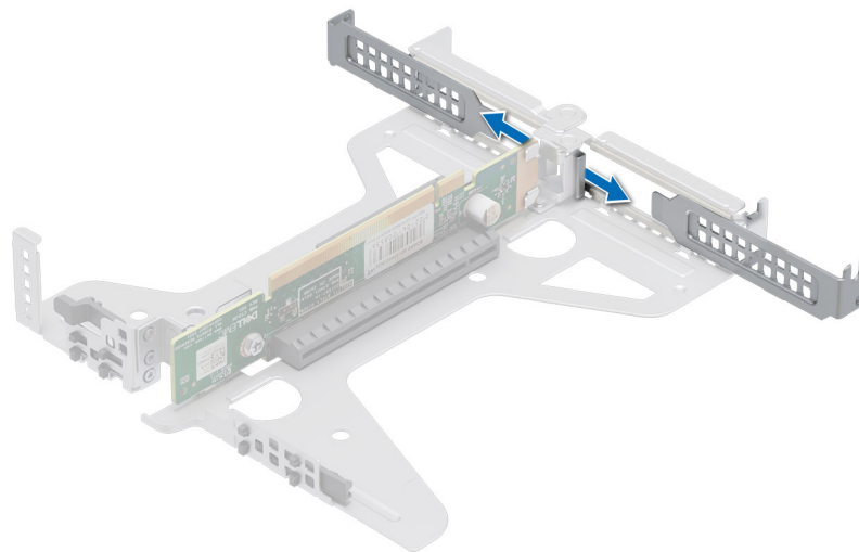
Abbildung 55. Entfernen des Abdeckblechs
