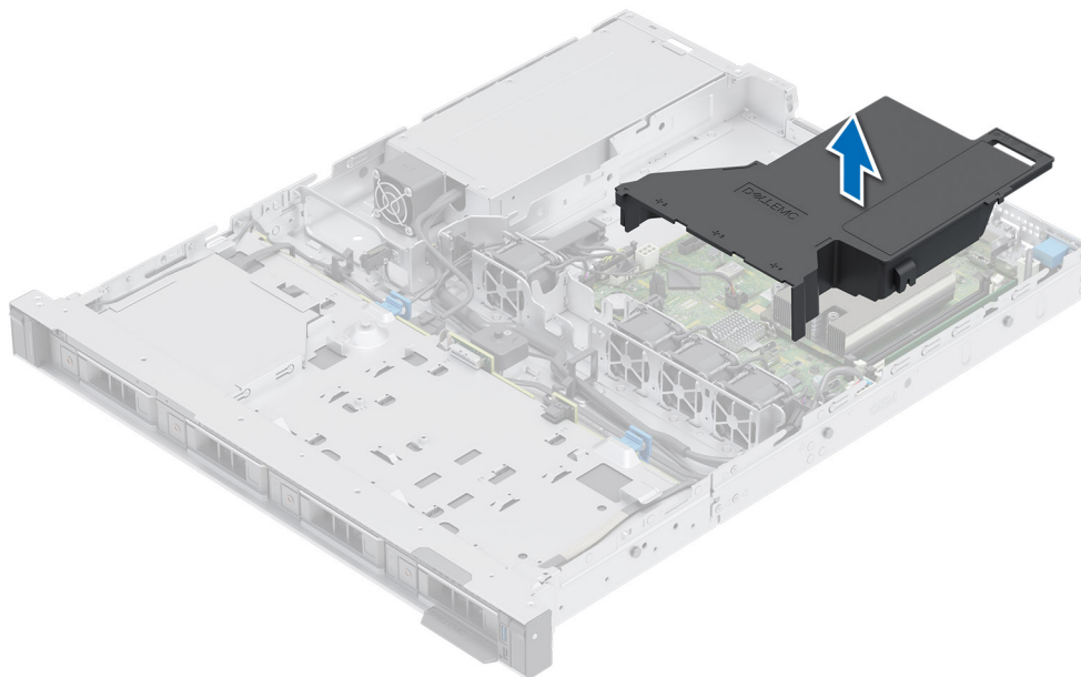
Abbildung 17. Entfernen des Kühlgehäuses
