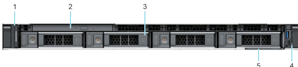
Abbildung 3. Vorderansicht eines Systems mit 2 x 3,5-Zoll-SAS/SATA-Laufwerken (kabelgebunden)
