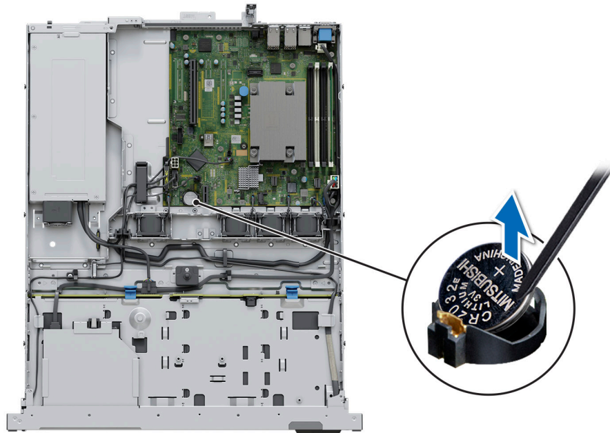
Abbildung 65. Entfernen der Systembatterie
