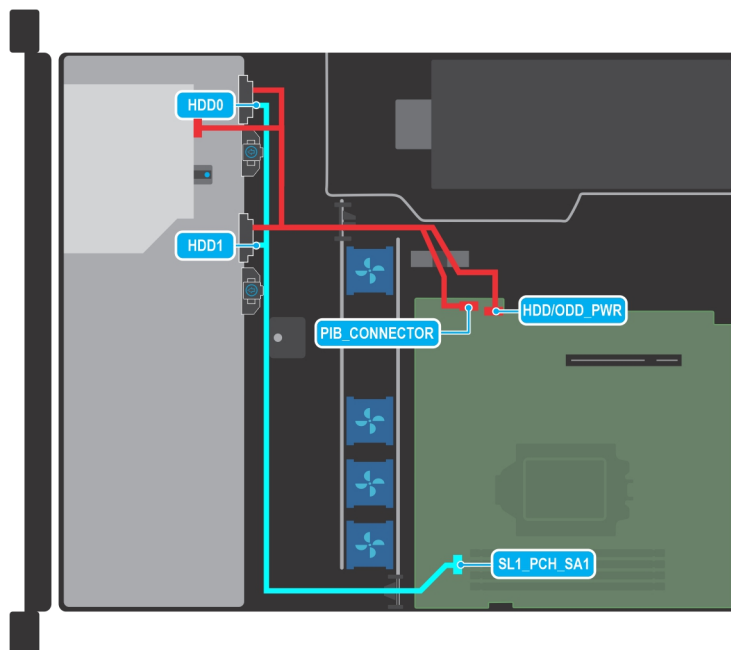
Abbildung 39. Kabelführung – Konfiguration mit 2 verkabelten 3,5-Zoll-Laufwerken mit SATA-Anschluss
