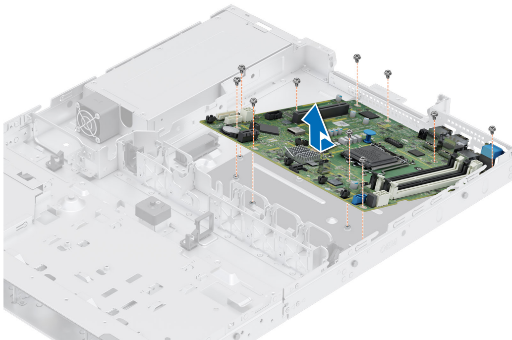
Abbildung 71. Entfernen der Hauptplatine
