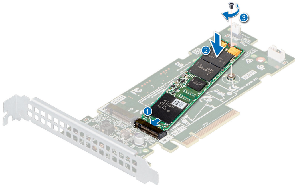
Abbildung 62. Einbauen des M.2-SSD-Moduls
