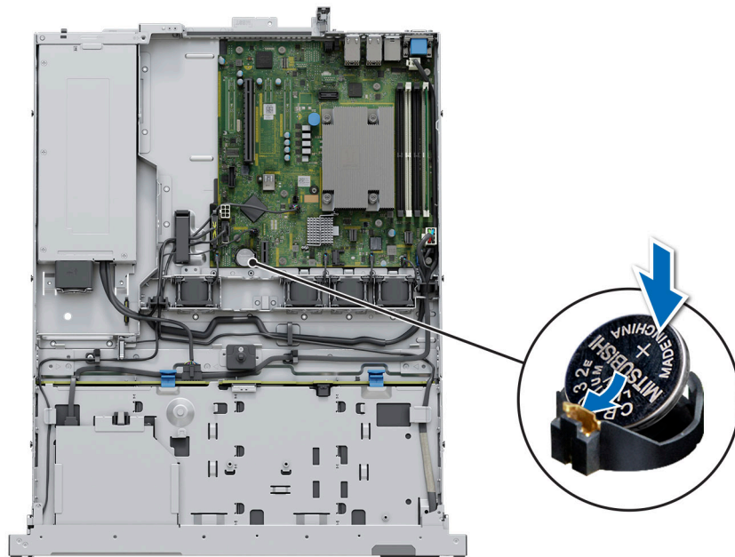
Abbildung 66. Installieren der Systembatterie
