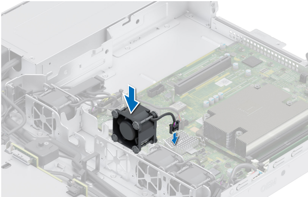
Abbildung 20. Einsetzen eines Kühlungslüfters
