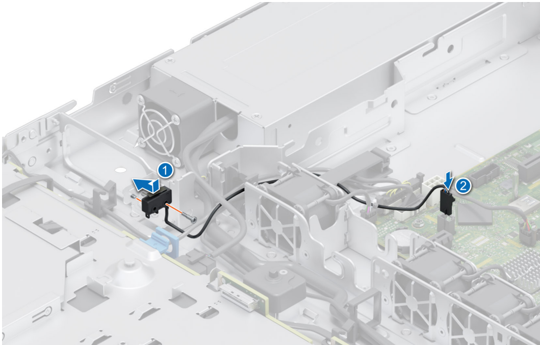
Abbildung 22. Installieren des Eingriffsschalters
