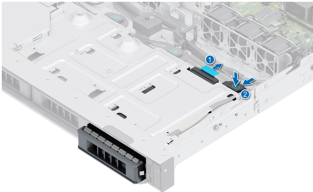
Abbildung 28. Entfernen des verkabelten Laufwerks
