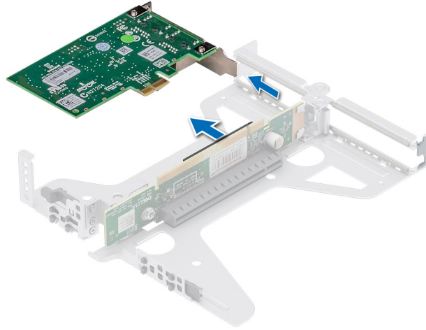
Abbildung 53. Entfernen einer Erweiterungskarte aus dem Riser
