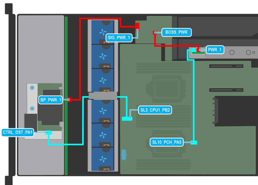
Abbildung 48. 8 x 3,5-Zoll-SAS/SATA
