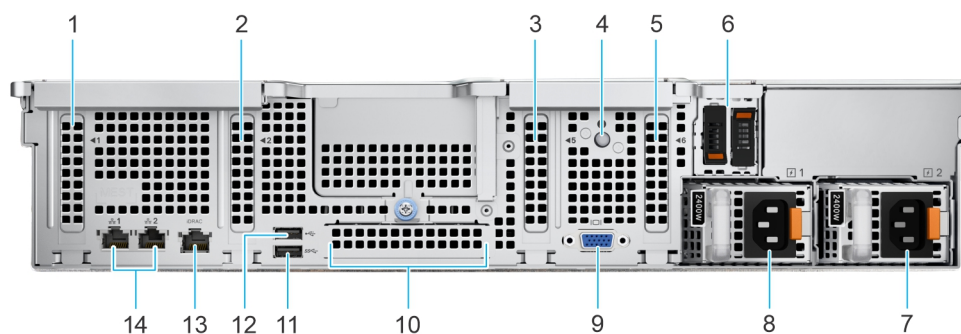
Abbildung 7. Rückansicht des Systems
