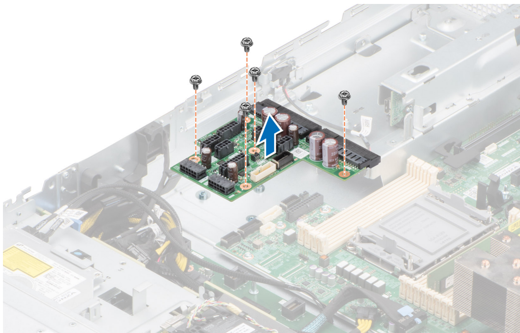
Abbildung 102. Stromzwischenplatine entfernen
