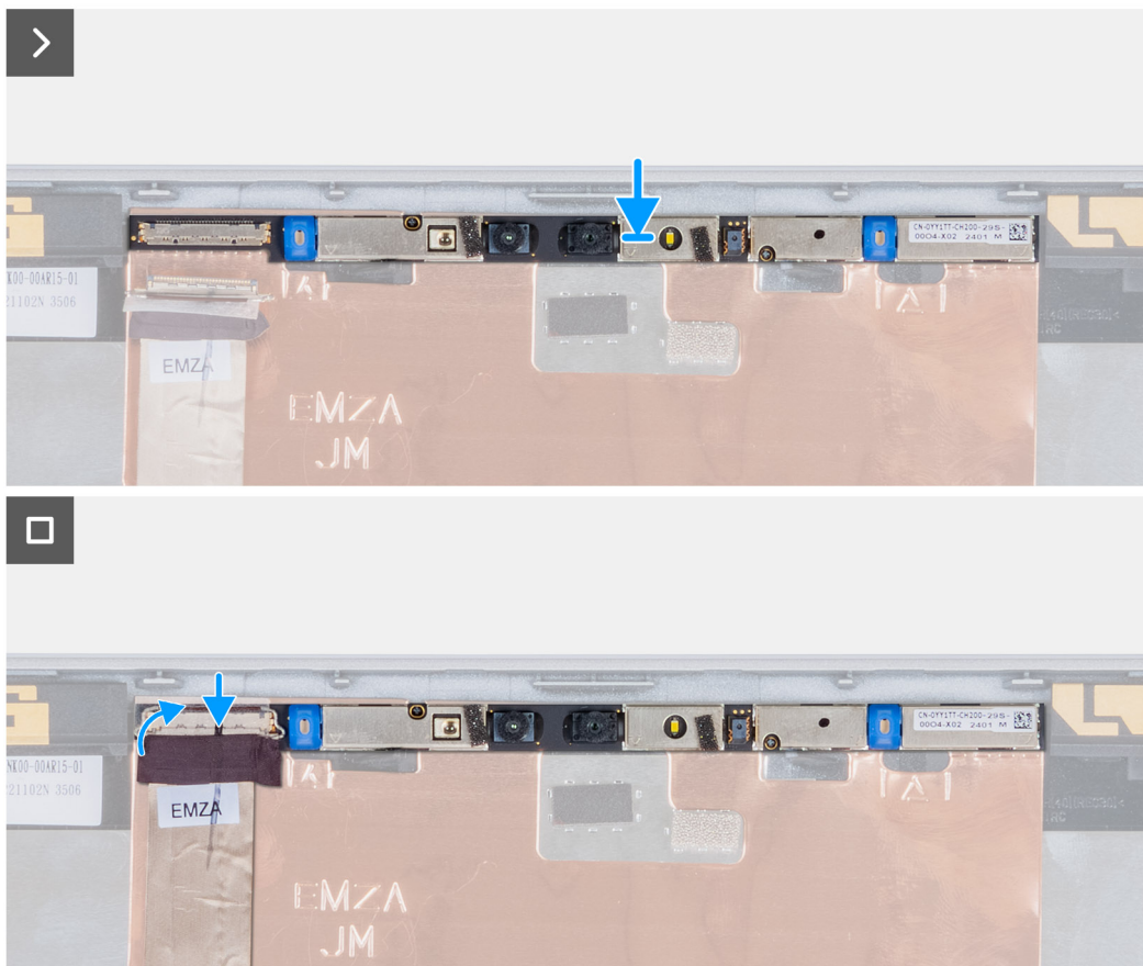
איור 5. התקנת מודול המצלמה
