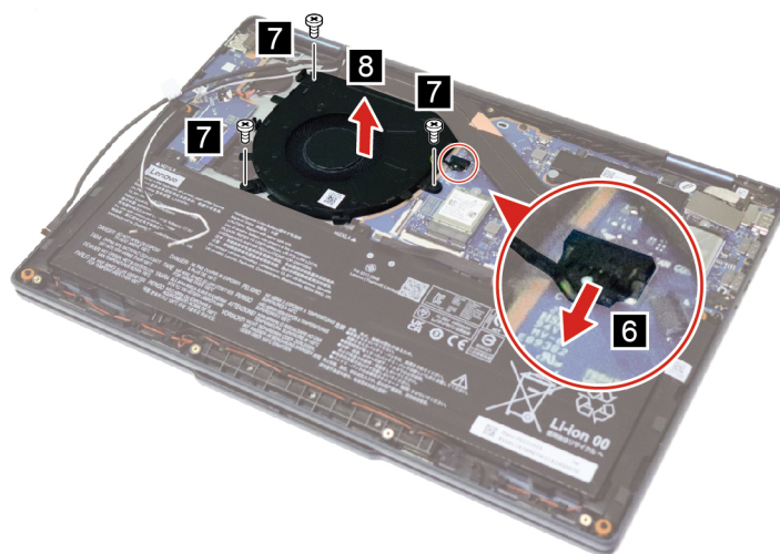
Figure 15. Disconnect the fan cable and remove the fan
