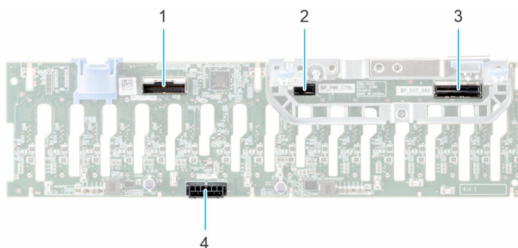
Ilustración 61. Backplane de 16 unidades de 2,5 pulgadas
