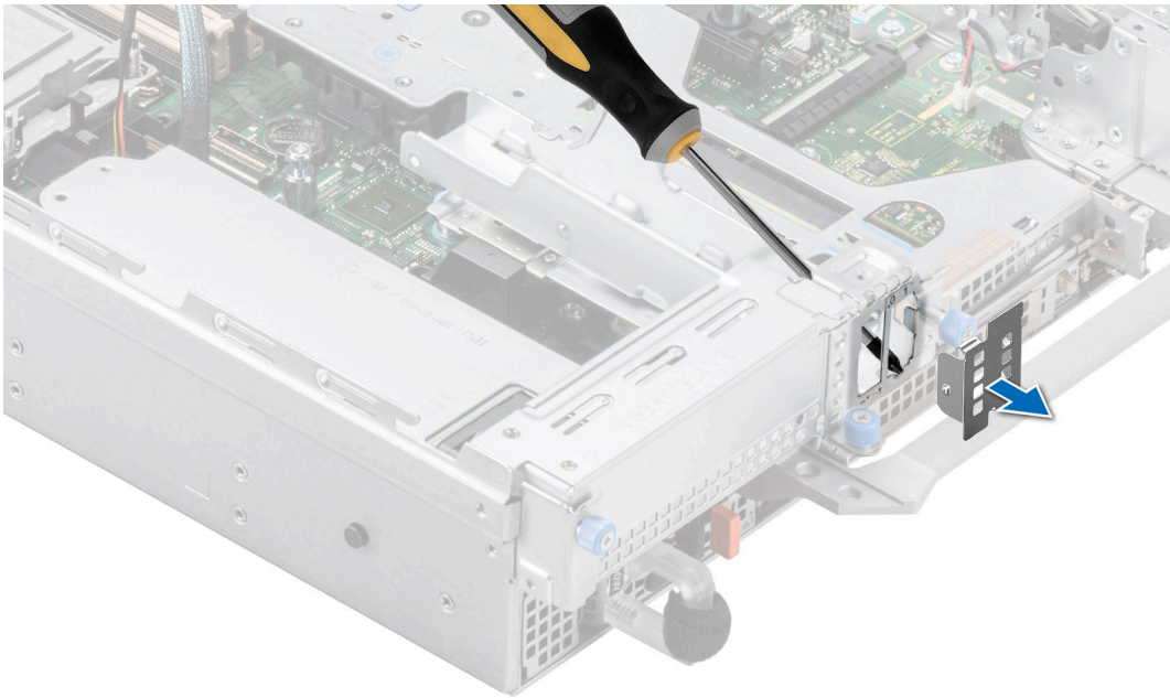
Ilustración 228. Extracción del módulo de Boot Optimized Storage Subsystem S2 de relleno
