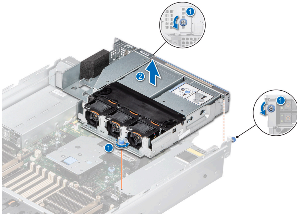
Ilustración 55. Extracción del módulo de 4 unidades posteriores de 2,5 pulgadas
