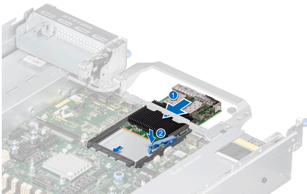
Ilustración 205. Instalación de la tarjeta OCP
