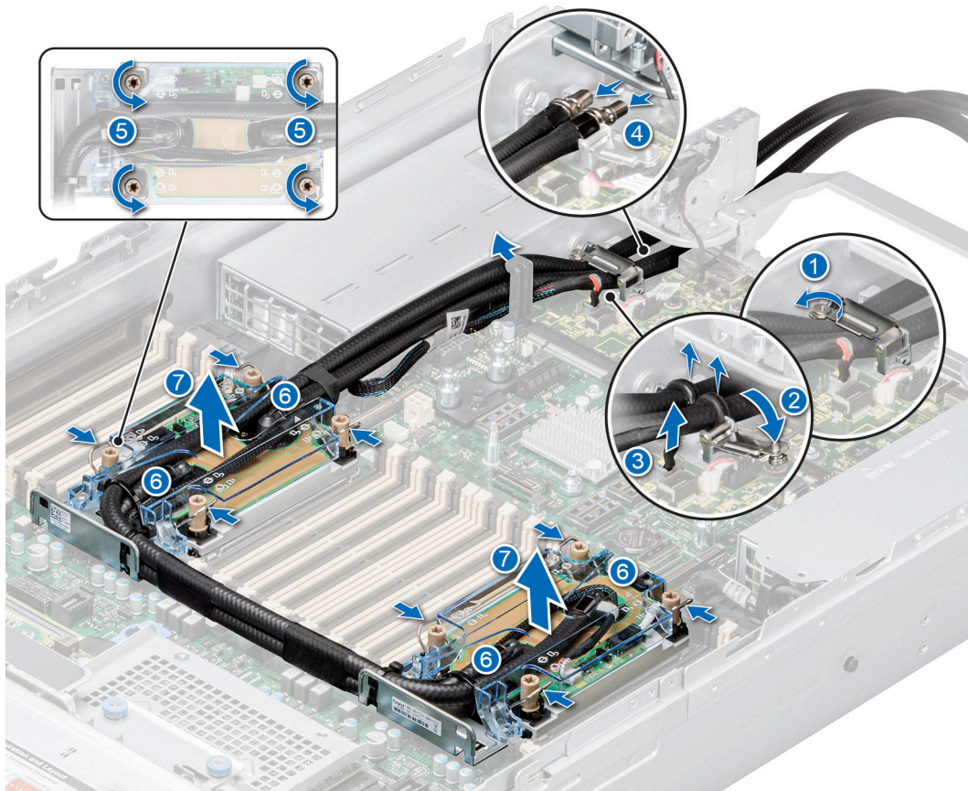
Ilustración 116. Extracción del módulo de enfriamiento líquido
