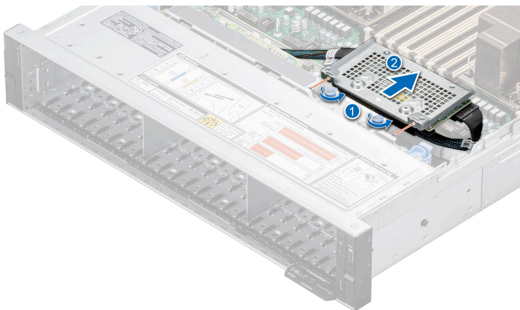
Ilustración 96. Extracción del módulo de PERC frontal de montaje posterior
