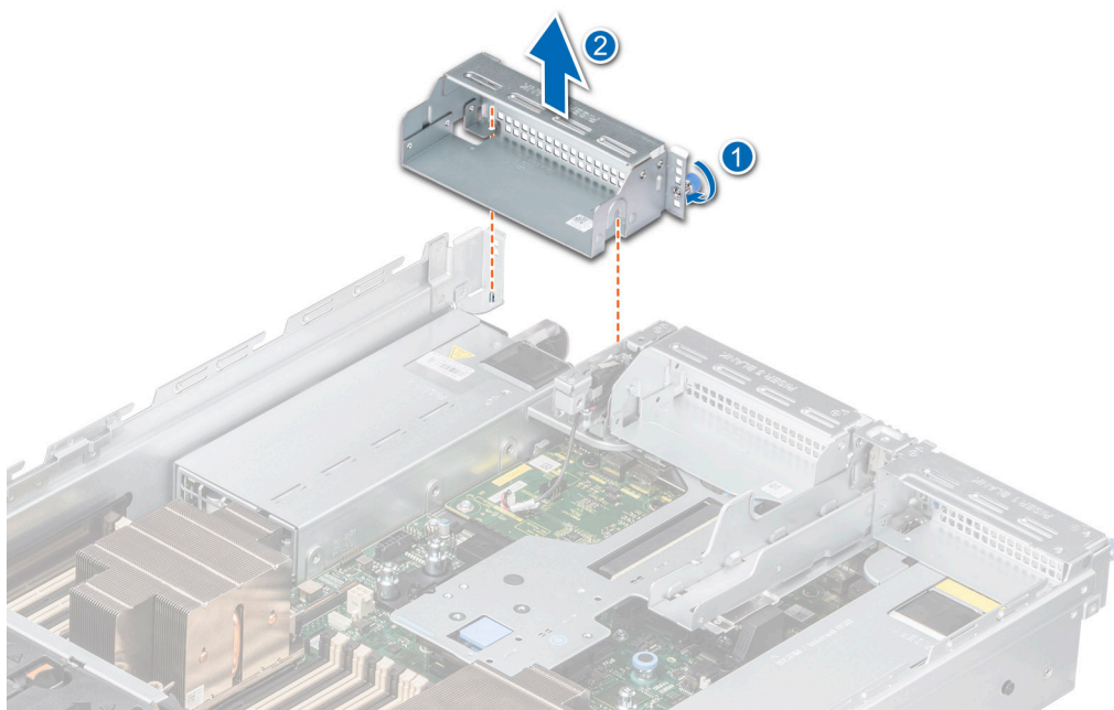
Ilustración 157. Extracción del soporte vertical de relleno 4
