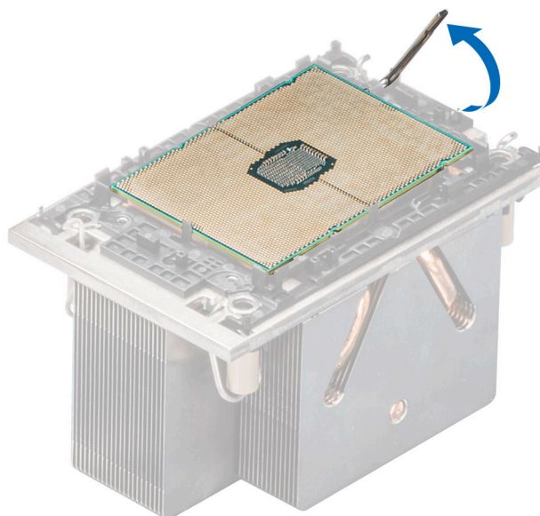
Ilustración 107. Levante la palanca de liberación del TIM
