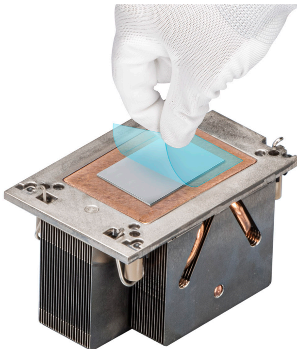
Ilustración 112. Extracción de la película de protección del material de interfaz térmica (TIM)
