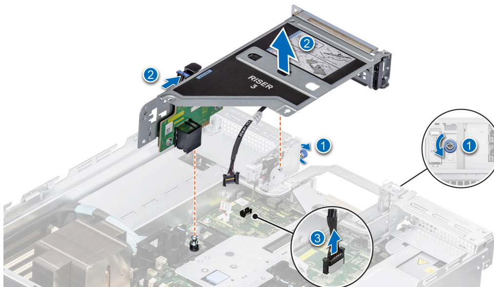
Ilustración 172. Desconexión del puerto serial COM
