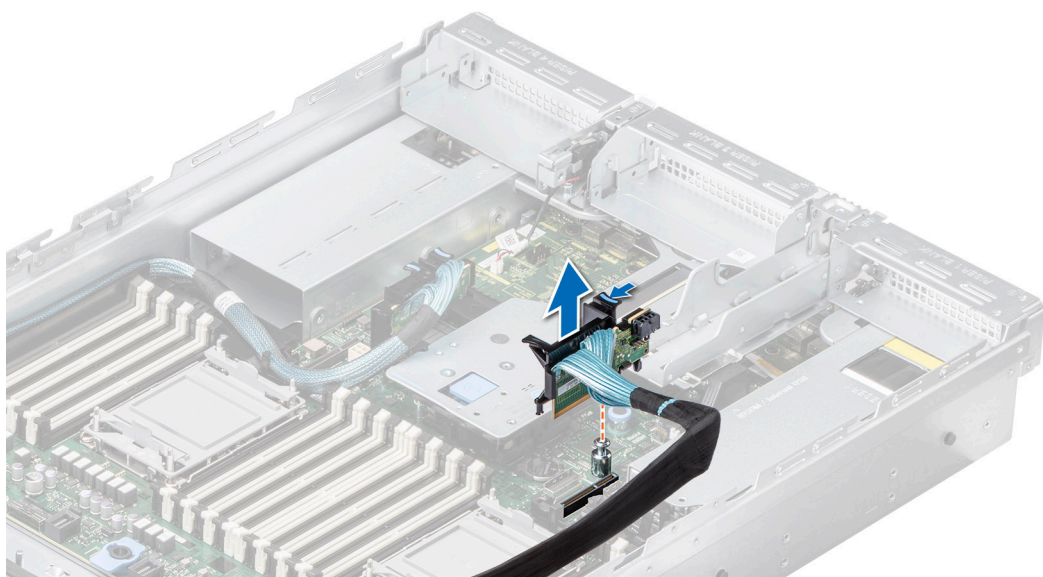
Ilustración 166. Extracción de la tarjeta de paleta R1
