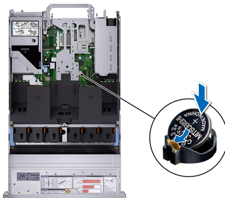
Ilustración 197. Instalación de la batería del sistema
