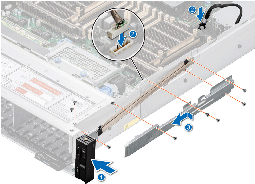
Ilustración 224. Instalación del panel de control derecho
