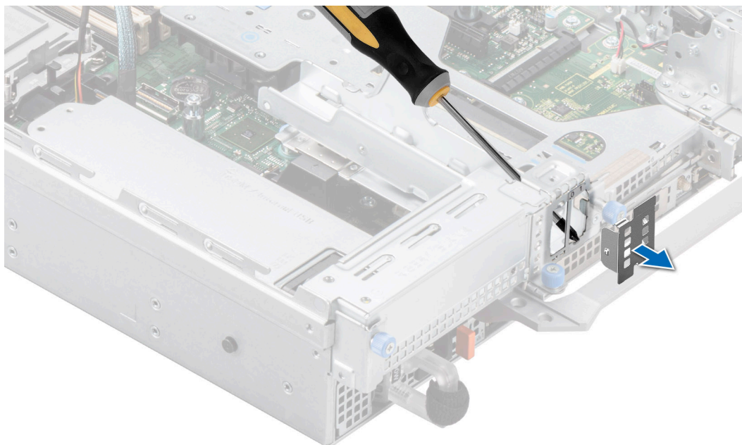
Ilustración 184. Extracción del módulo de Boot Optimized Storage Subsystem S2 de relleno
