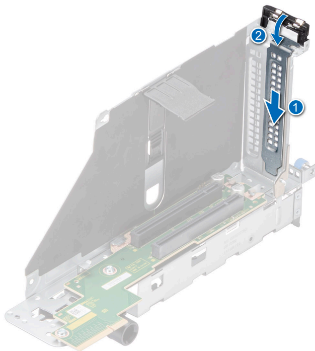
Ilustración 148. Instalación del soporte de relleno
