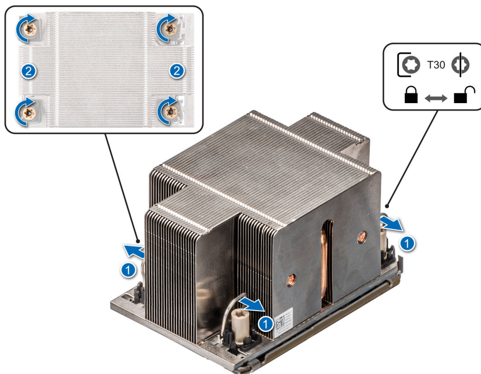
Ilustración 115. Coloque los cables antiinclinación en la posición de bloqueo y ajuste las tuercas
