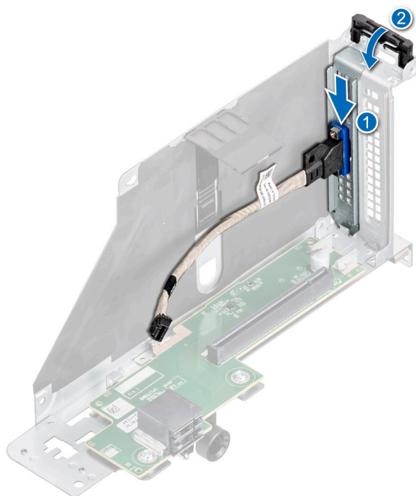
Ilustración 178. Instalación del puerto de VGA
