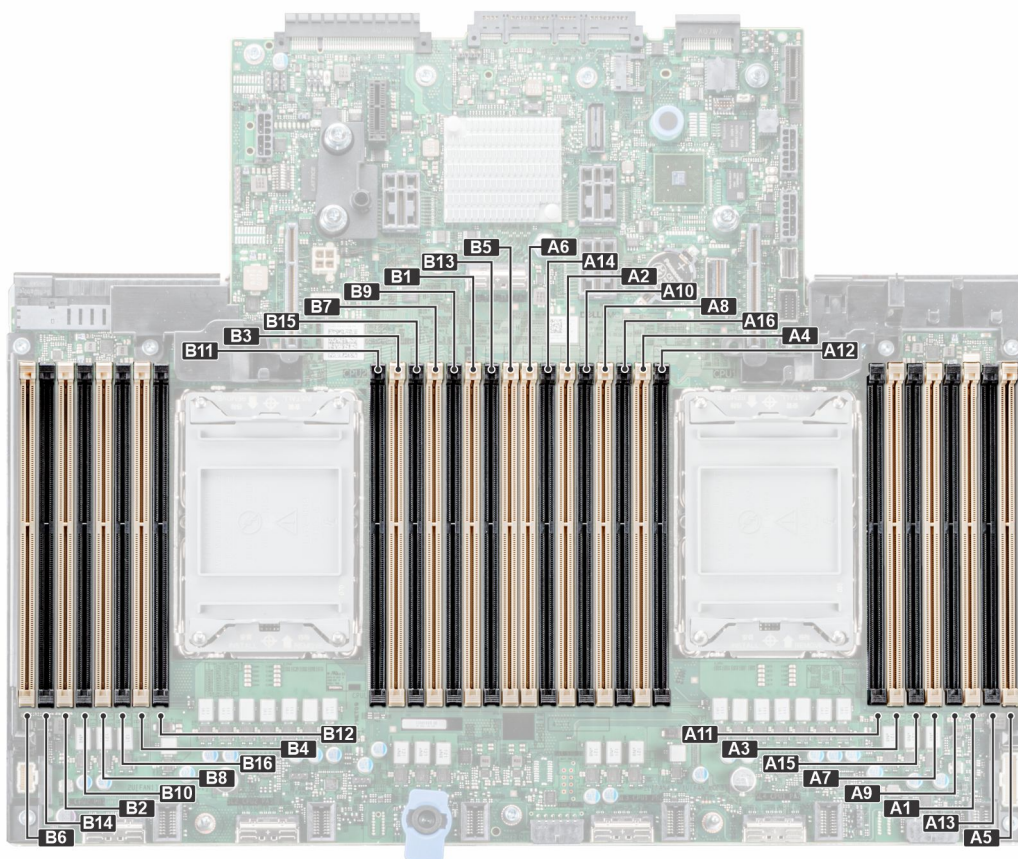
Ilustración 102. Canales de la memoria
