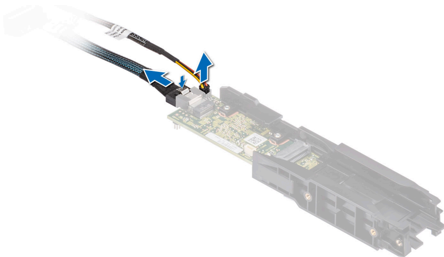
Ilustración 191. Extracción de los cables de alimentación y de señal de Boot Optimized Storage Subsystem S2 del módulo de Boot Optimized Storage Subsystem S2
