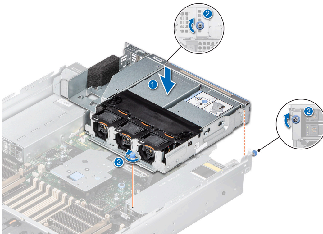
Ilustración 56. Instalación del módulo de unidades posterior de 4 x 2,5 pulgadas
