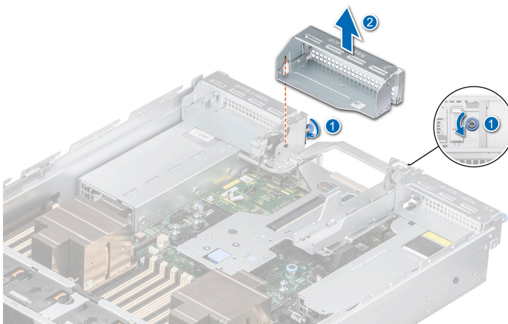
Ilustración 141. Extracción del soporte vertical de relleno 3
