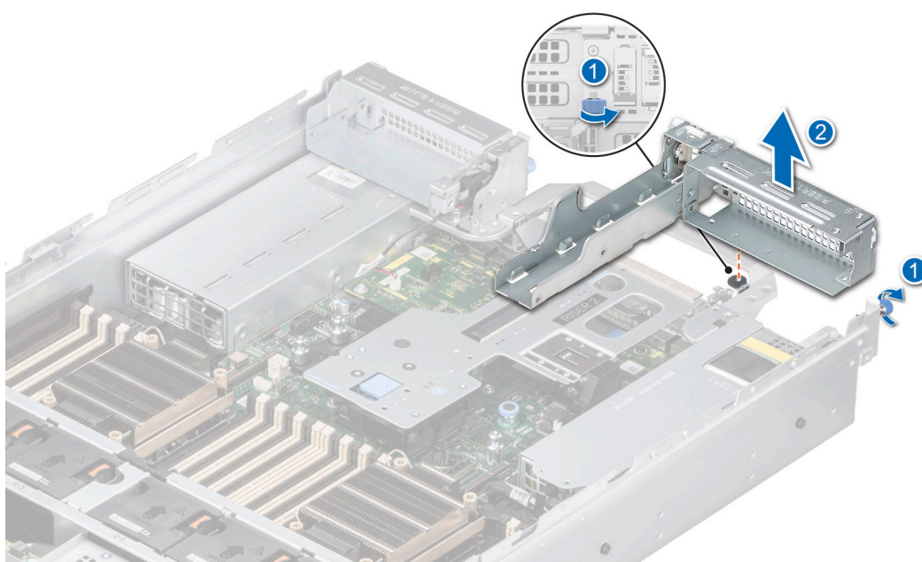
Ilustración 140. Extracción del soporte vertical de relleno 1
