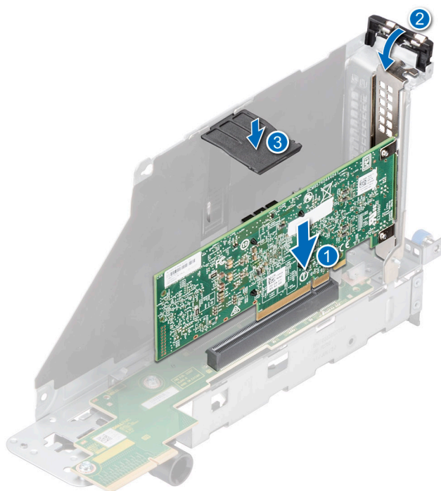
Ilustración 150. Instalación de una tarjeta de expansión en el soporte vertical para tarjetas de expansión
