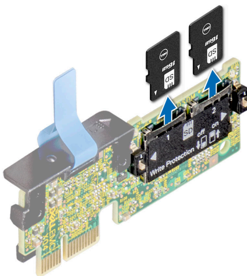
Ilustración 182. Extracción de la tarjeta microSD
