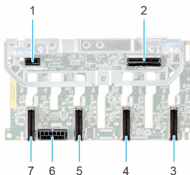
Ilustración 59. Backplane de 8 unidades de 2,5 pulgadas
