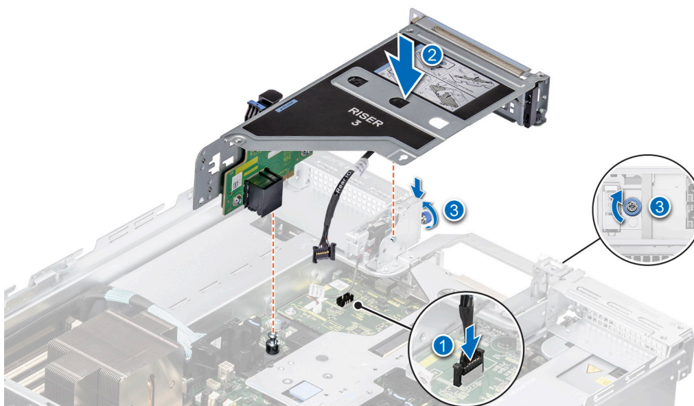
Ilustración 175. Conexión del puerto serial de COM
