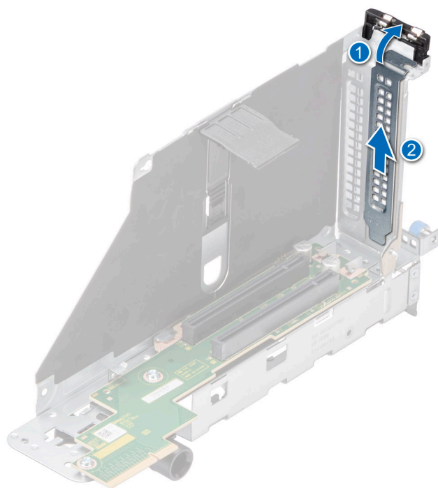
Ilustración 149. Extracción del soporte de relleno
