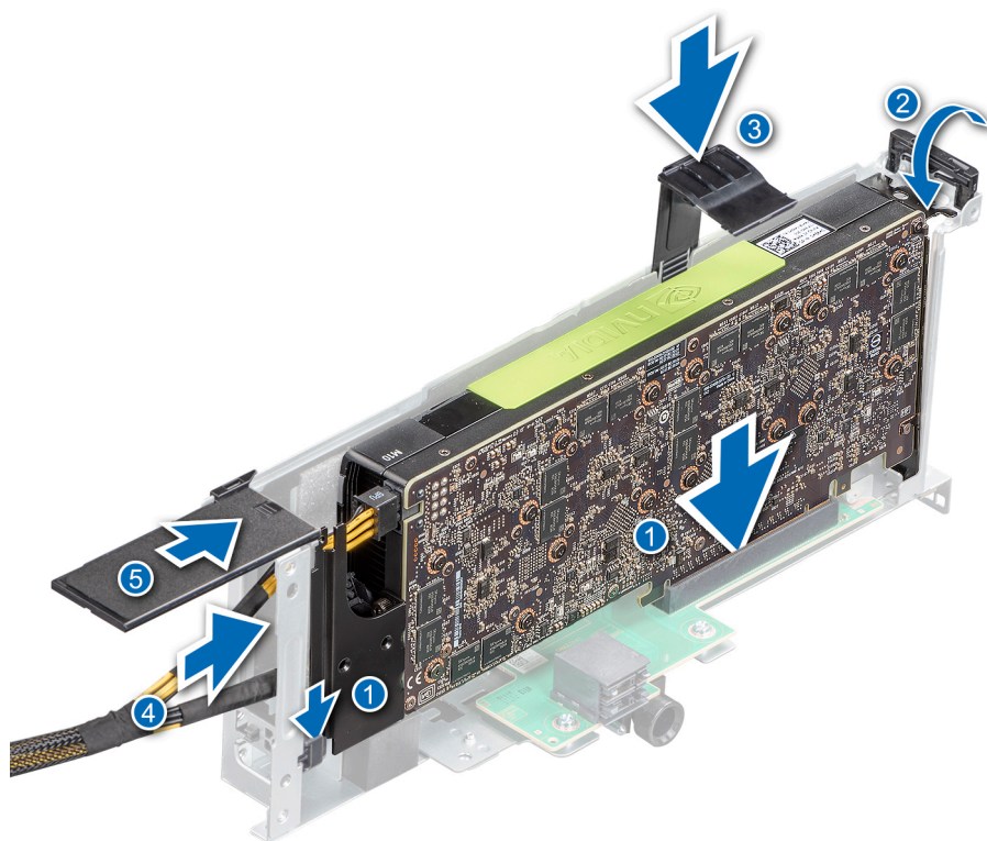
Ilustración 165. Instalación de la GPU en el soporte vertical 4
