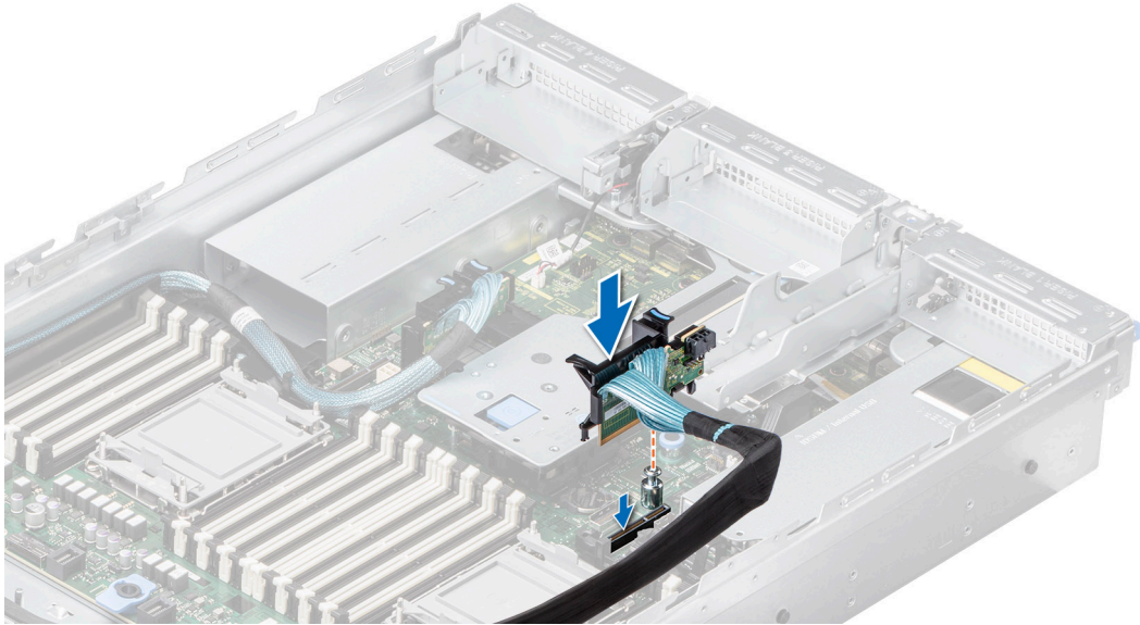
Ilustración 168. Instalación de la tarjeta de paleta R1
