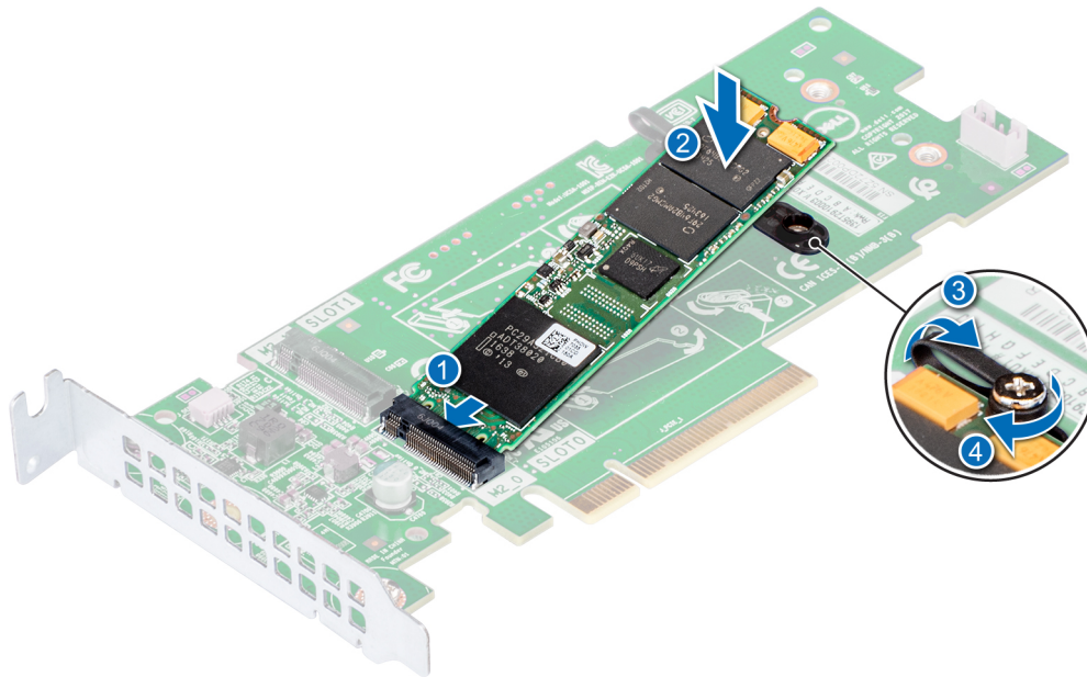
Ilustración 171. Instalación del módulo de SSD M.2
