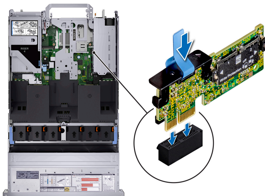
Ilustración 181. Instalación del módulo IDSDM
