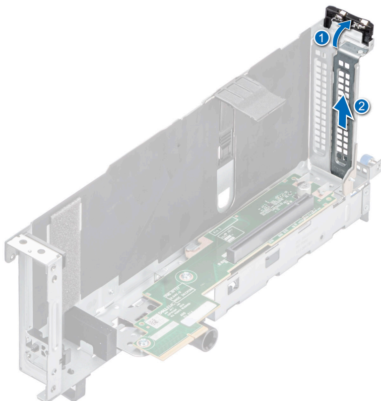
Ilustración 163. Extracción del soporte de relleno
