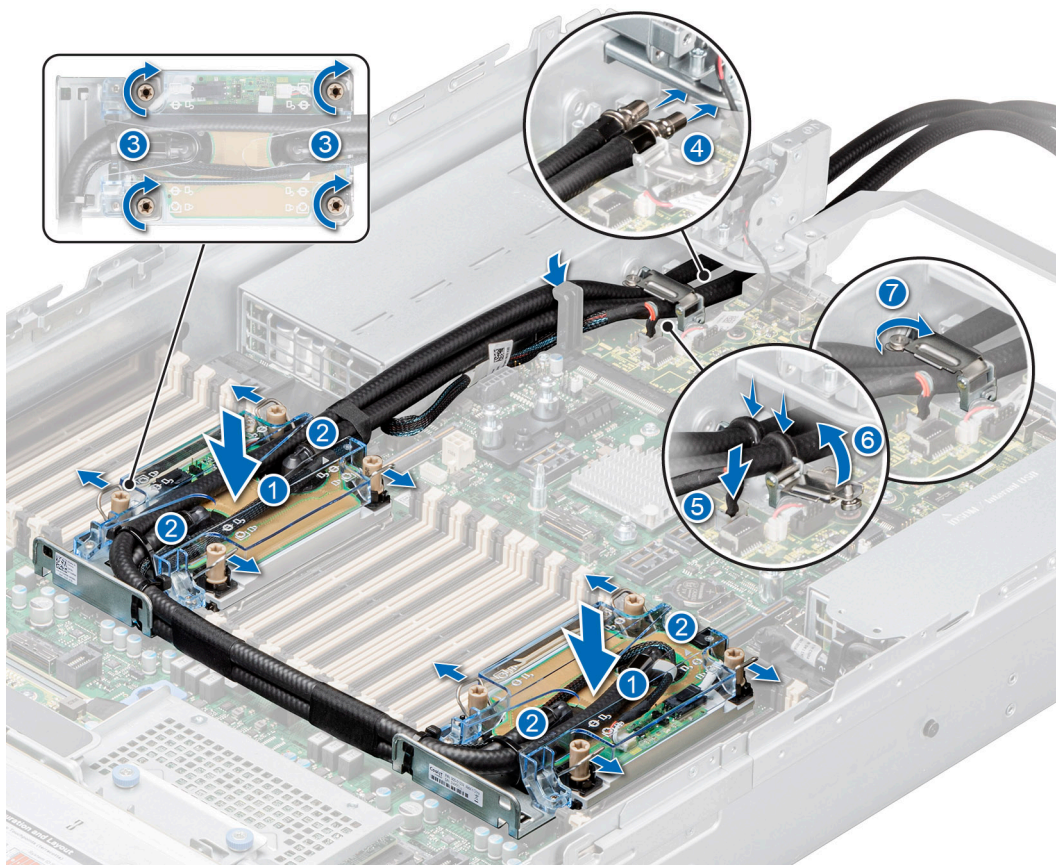
Ilustración 117. Instalación del módulo de enfriamiento con líquido
