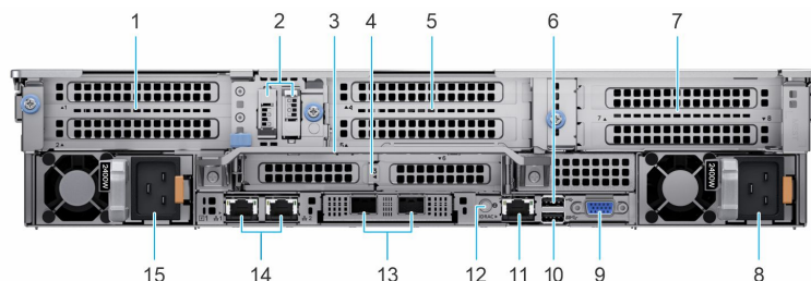
Ilustración 8. Vista posterior del sistema
