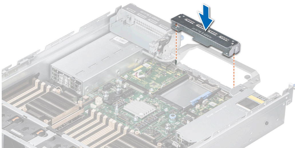
Ilustración 136. Instalación de la tarjeta elevadora de relleno 2
