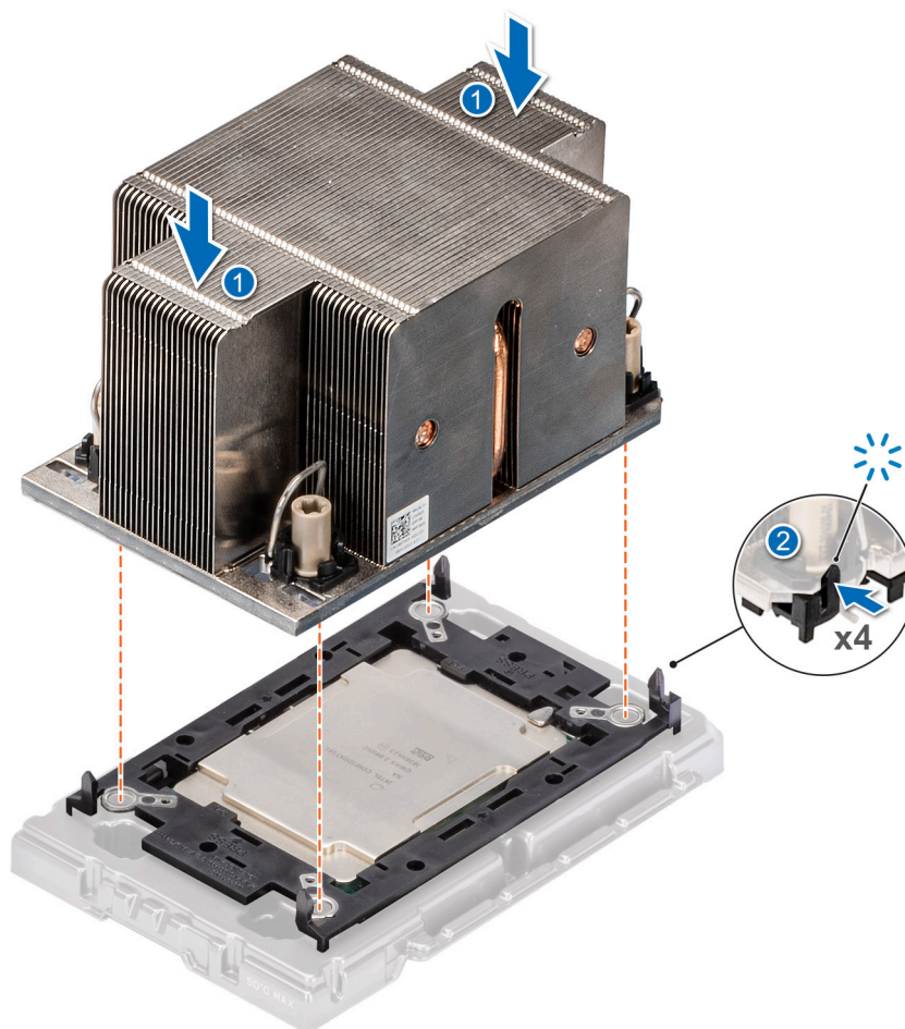
Ilustración 113. Instalación del dissipador de calor en el procesador.
