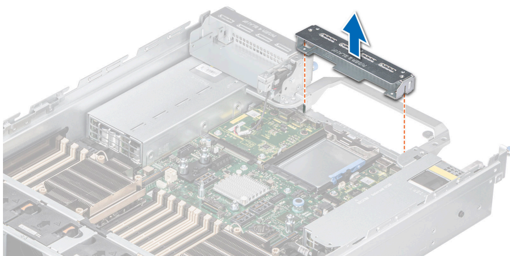
Ilustración 139. Extracción del soporte vertical de relleno 2
