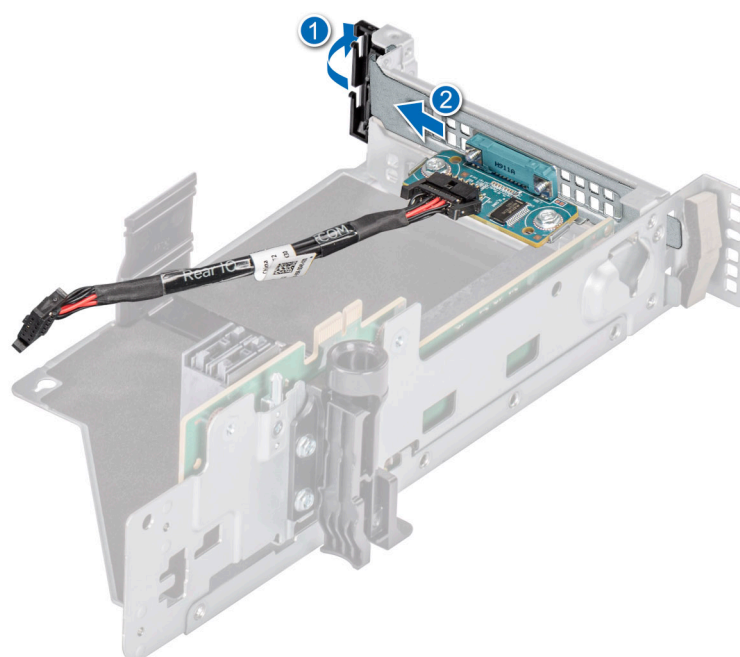
Ilustración 173. Extracción del puerto serial de COM
