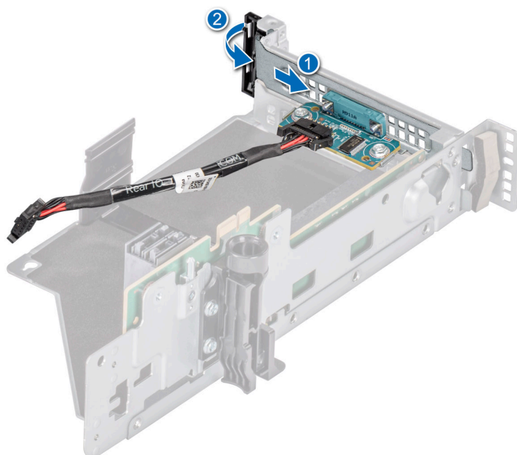
Ilustración 174. Instalación del puerto serie COM
