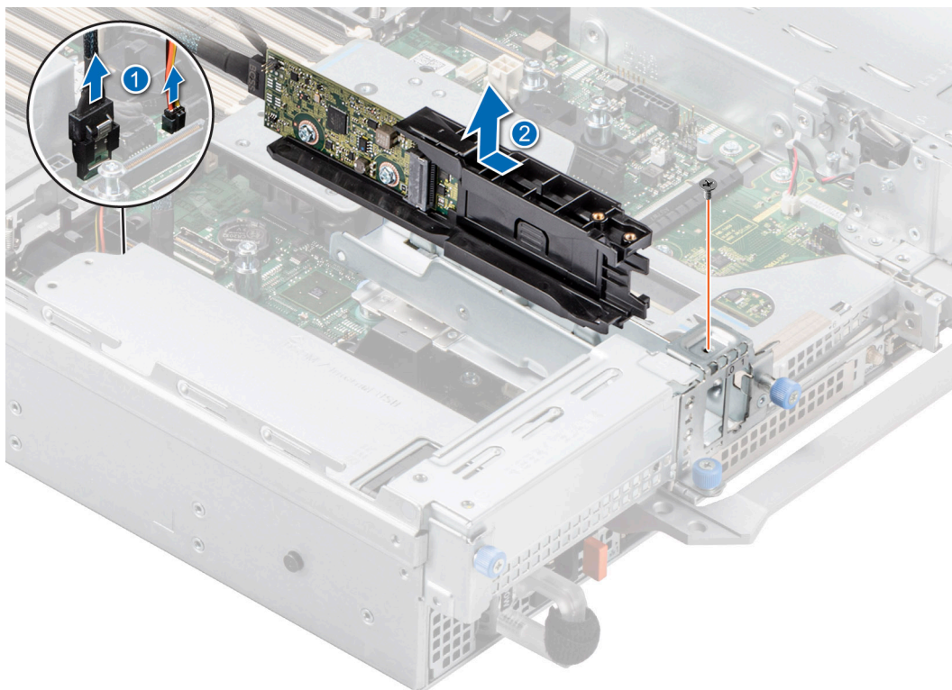
Ilustración 190. Extracción del módulo de Boot Optimized Storage Subsystem S2
