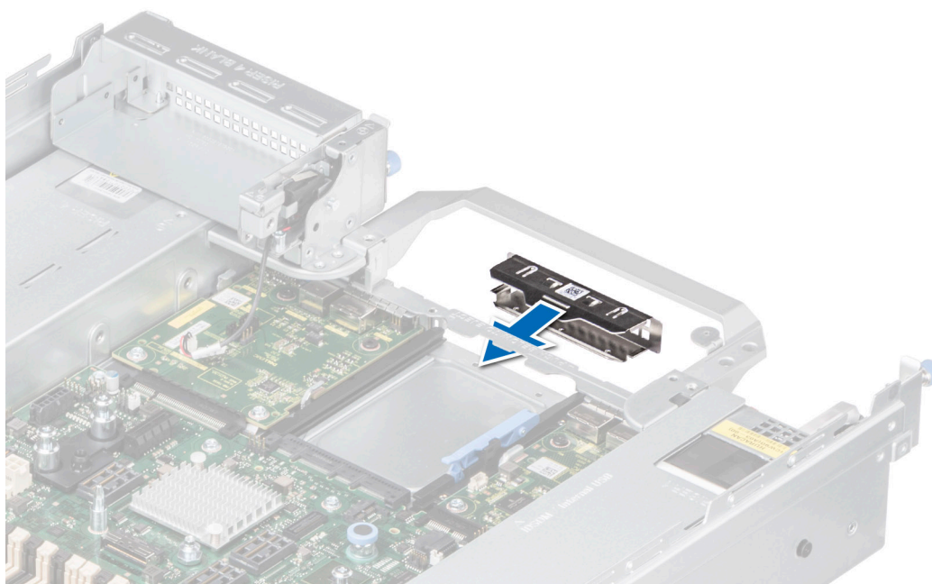
Ilustración 203. Instalación del soporte de relleno
