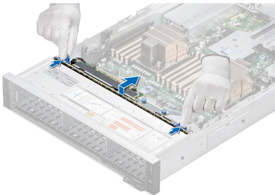
Ilustración 65. Extracción del backplane de la unidad
