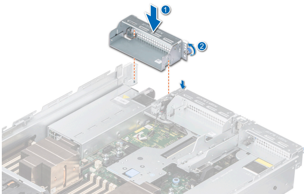
Ilustración 138. Instalación de la tarjeta elevadora de relleno 4
