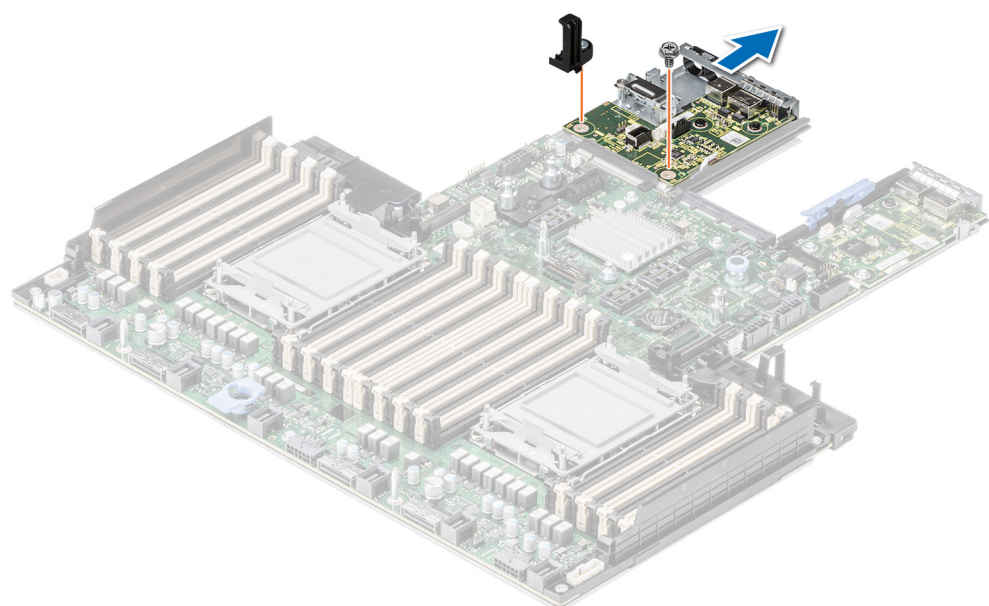
Ilustración 220. Extracción de la placa de I/O posterior de enfriamiento con líquido
