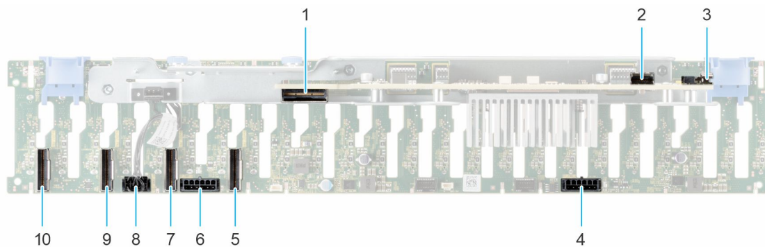
Ilustración 62. Backplane de 24 unidades de 2,5 pulgadas
