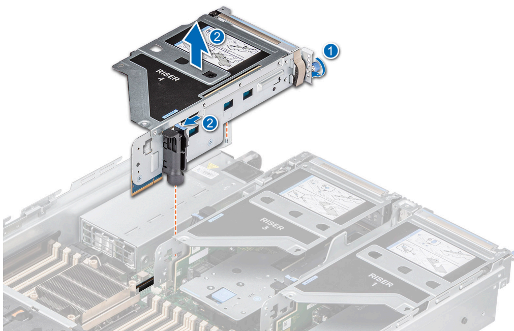
Ilustración 134. Extracción de la tarjeta elevadora para tarjetas de expansión (tarjeta elevadora 4)
