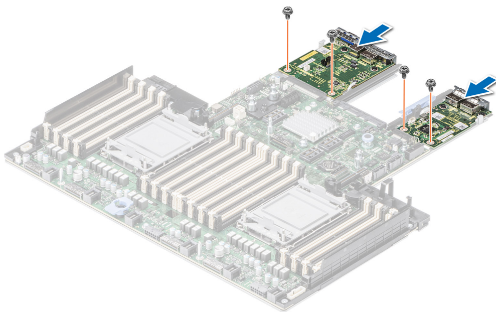
Ilustración 221. Instalación de la tarjeta LOM y la placa de I/O posterior
