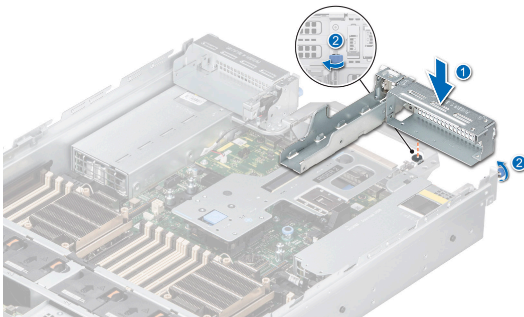
Ilustración 135. Instalación de la tarjeta elevadora de relleno 1
