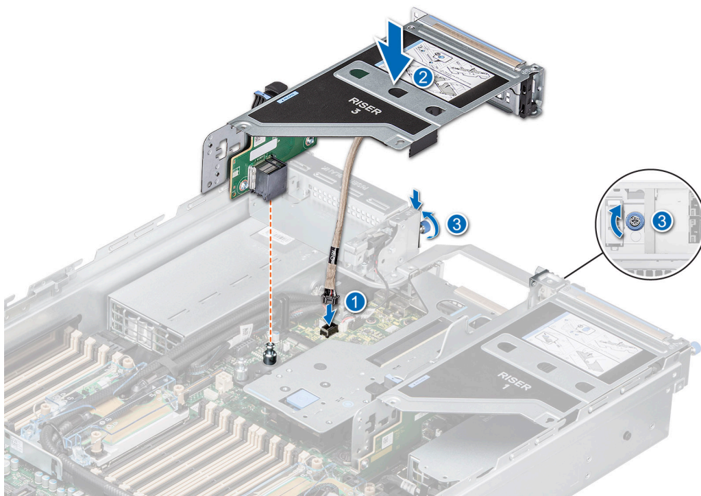
Ilustración 179. Conexión del cable del puerto de VGA.
