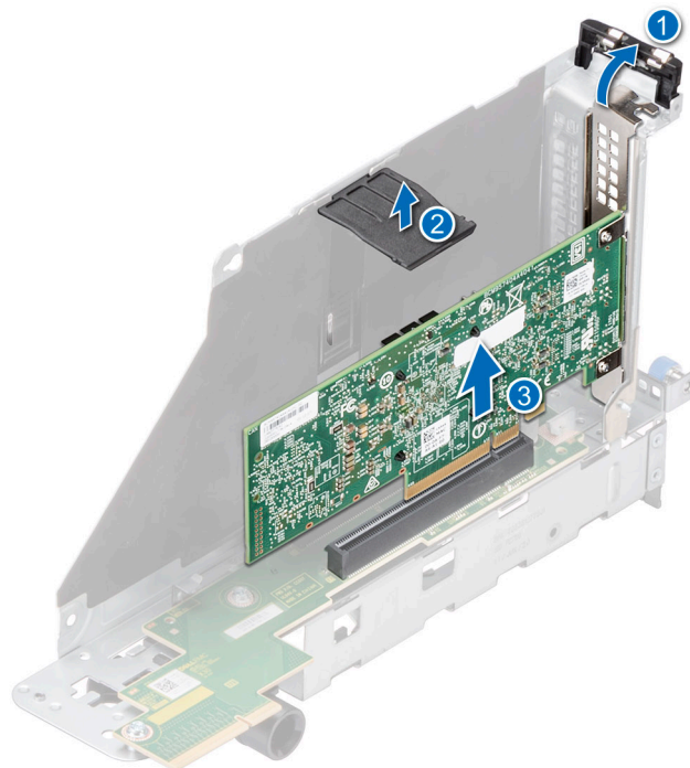
Ilustración 147. Extracción de una tarjeta de expansión del soporte vertical para tarjetas de expansión
