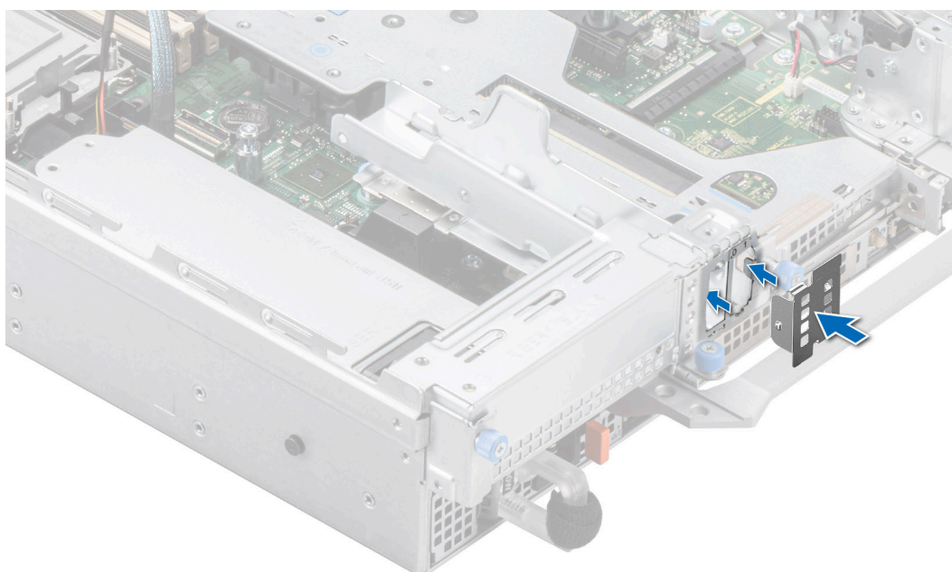
Ilustración 185. Instalación del módulo de Boot Optimized Storage Subsystem S2 de relleno
