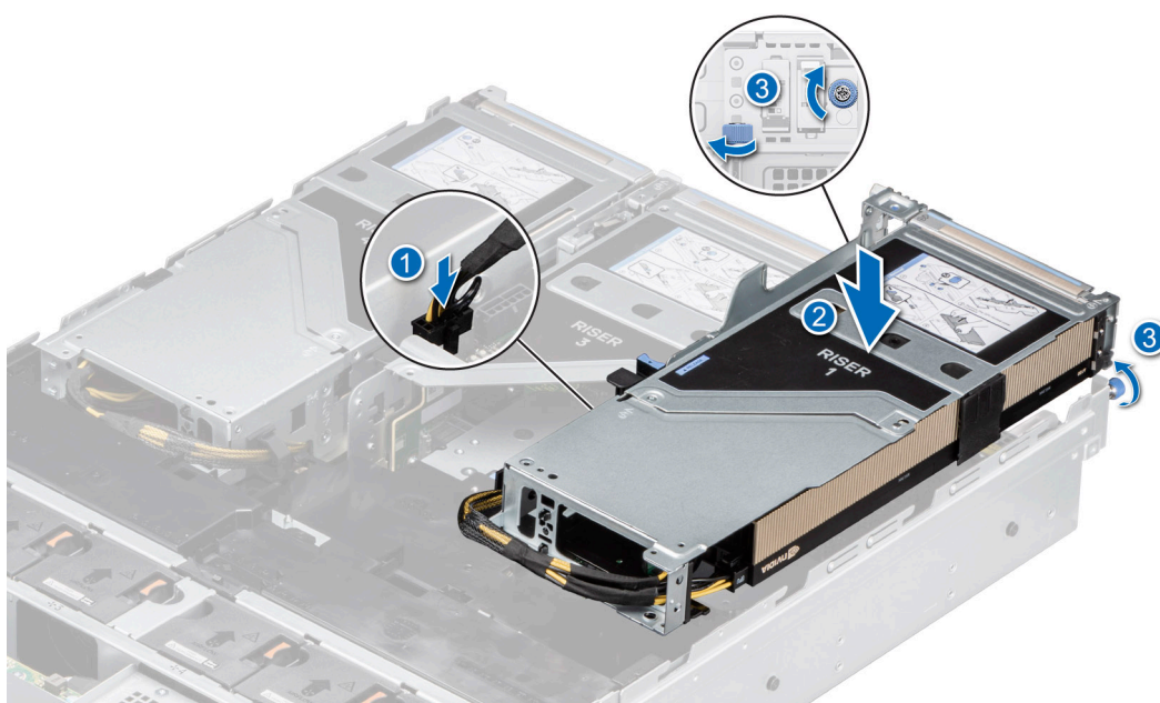
Ilustración 158. Instalación del soporte vertical para tarjetas de expansión (soporte vertical 1)
