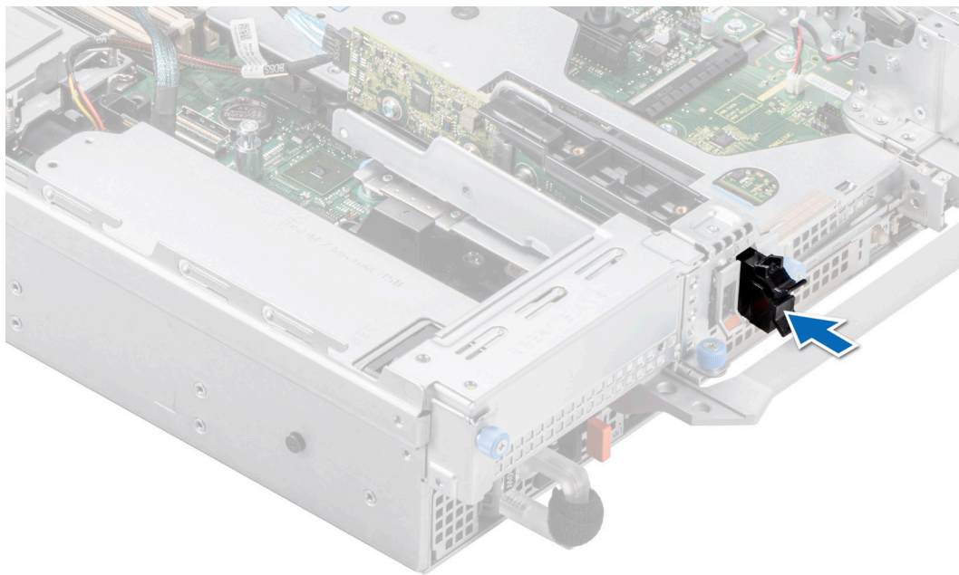
Ilustración 187. Instalación del soporte de tarjetas de relleno de Boot Optimized Storage Subsystem S2
