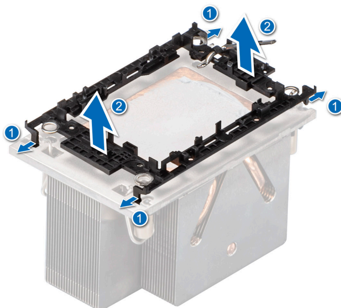
Ilustración 108. Extracción del gancho de retención
