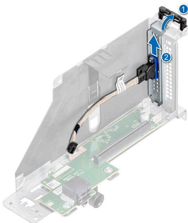
Ilustración 177. Extracción del puerto de VGA
