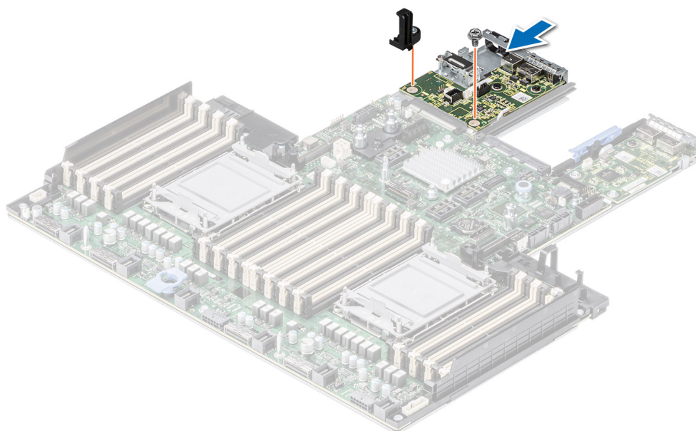
Ilustración 222. Instalación de la placa de I/O posterior de enfriamiento con líquido
