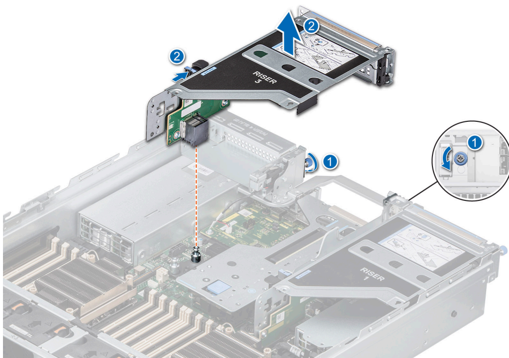
Ilustración 132. Extracción de la tarjeta elevadora para tarjetas de expansión (tarjeta elevadora 3)
