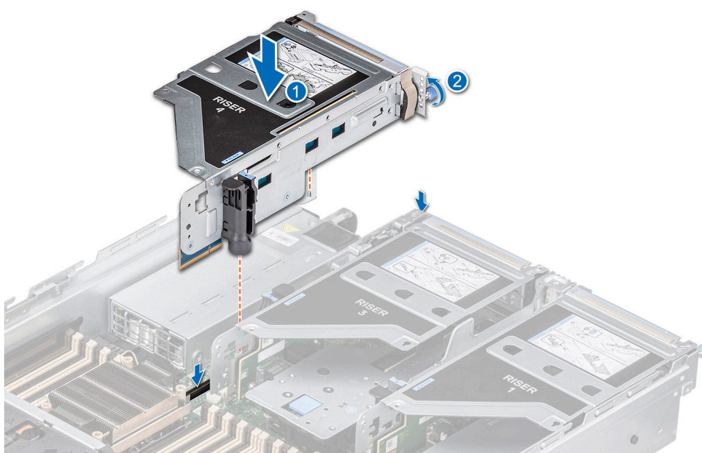
Ilustración 146. Instalación del soporte vertical para tarjetas de expansión (soporte vertical 4)
