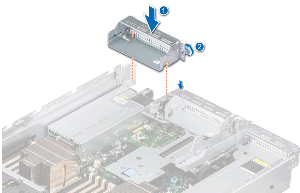
Ilustración 155. Instalación del soporte vertical de relleno 4
