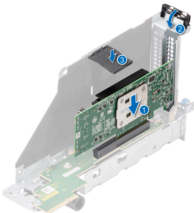
Ilustración 101. Instalación del módulo de APERC
