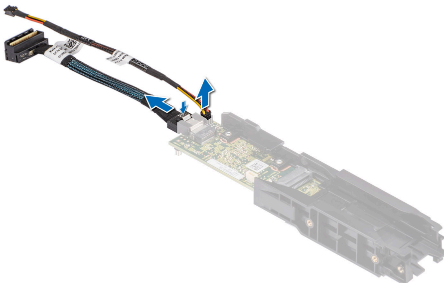
Ilustración 151. Extracción del cable de alimentación de Boot Optimized Storage Subsystem y el cable de señal de Boot Optimized Storage Subsystem del módulo de la tarjeta controladora de Boot Optimized Storage Subsystem S2
