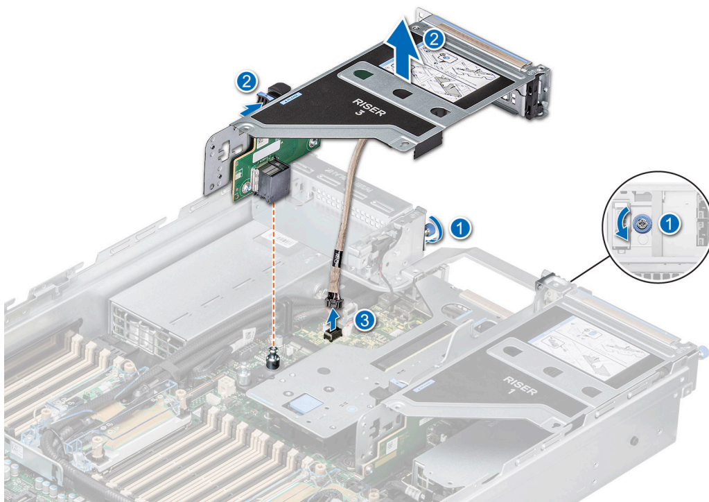
Ilustración 176. Desconexión del cable del puerto de VGA
