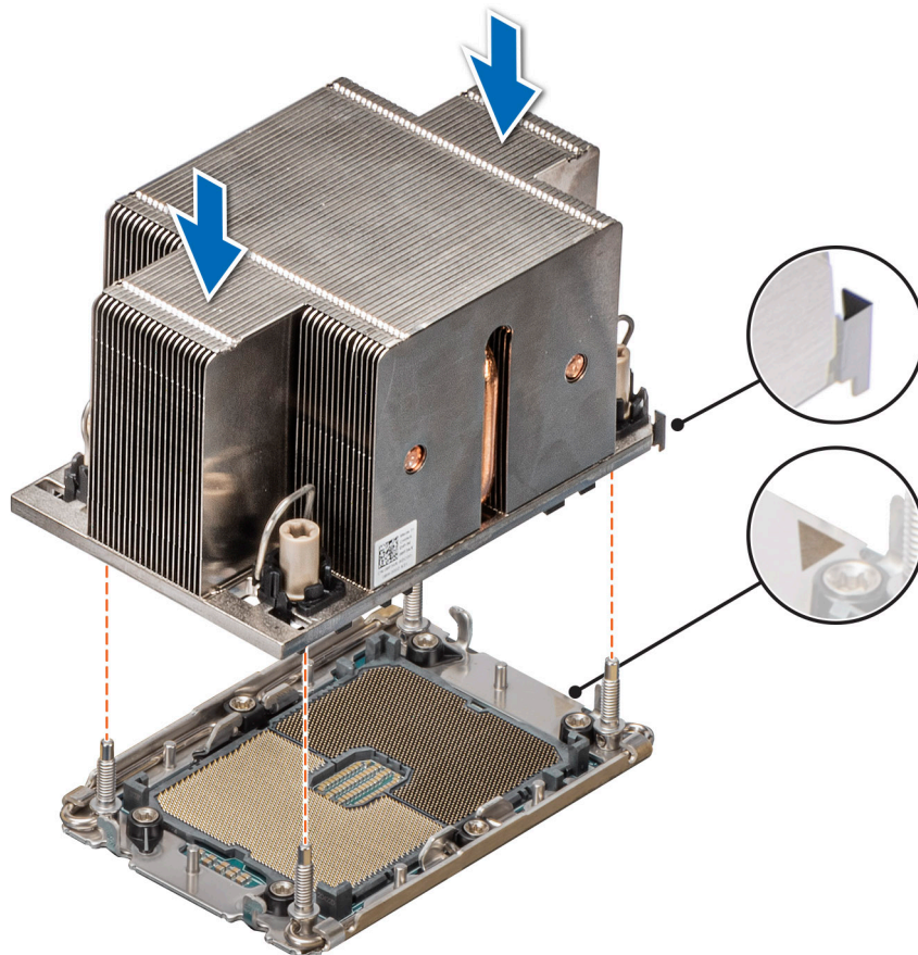
Ilustración 114. Instalación del disipador de calor del procesador
