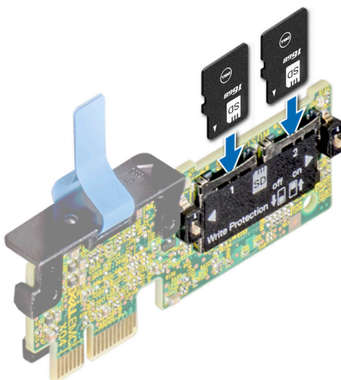
Ilustración 183. Instalación de la tarjeta microSD
