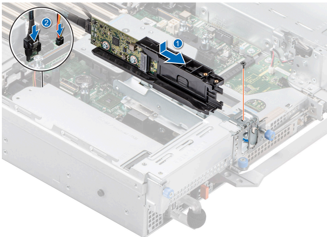
Ilustración 193. Instalación del módulo de Boot Optimized Storage Subsystem S2
