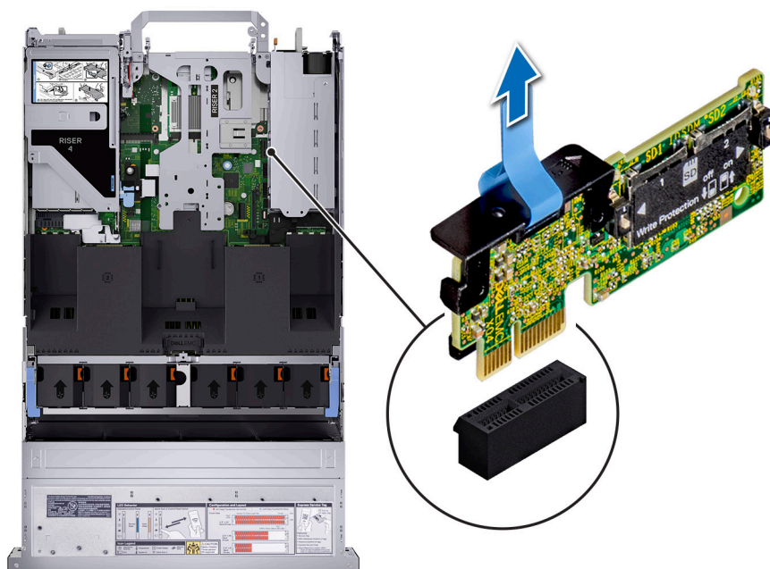
Ilustración 180. Extracción del módulo IDSDM
