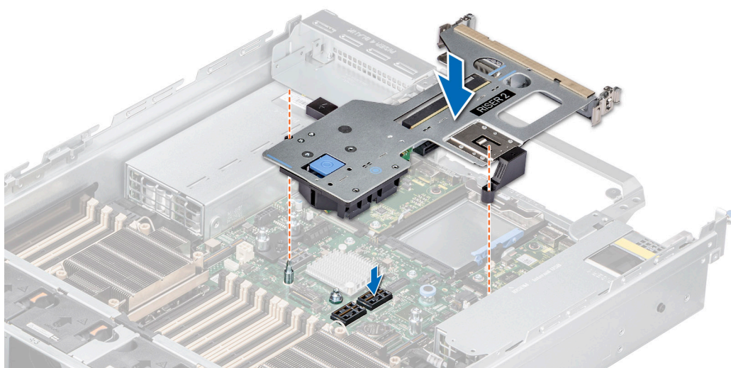
Ilustración 143. Instalación del soporte vertical para tarjetas de expansión (soporte vertical 2)
