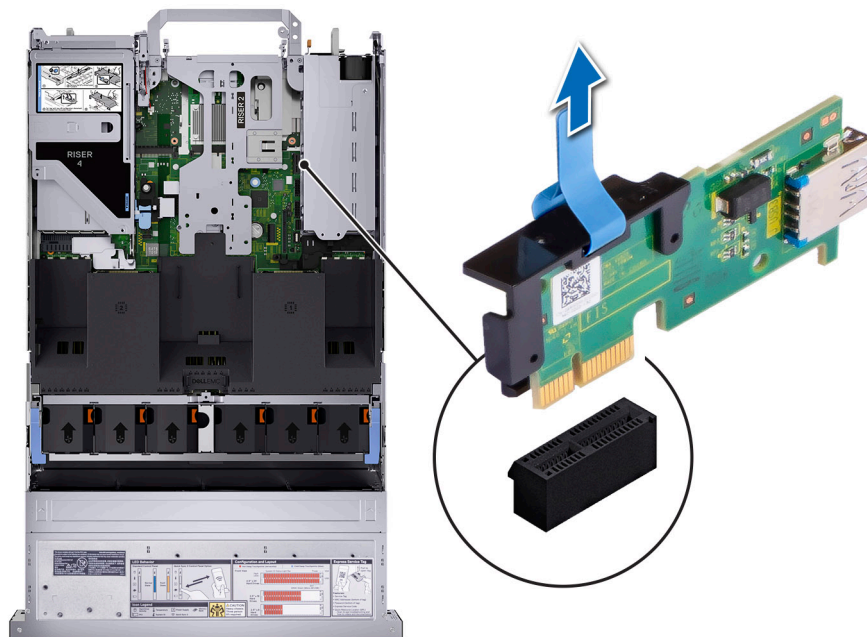
Ilustración 198. Extracción de la tarjeta USB interna
