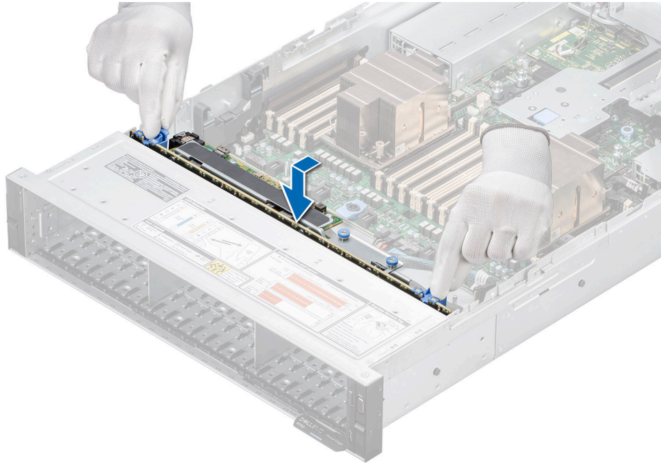
Ilustración 66. Instalación del backplane de la unidad
