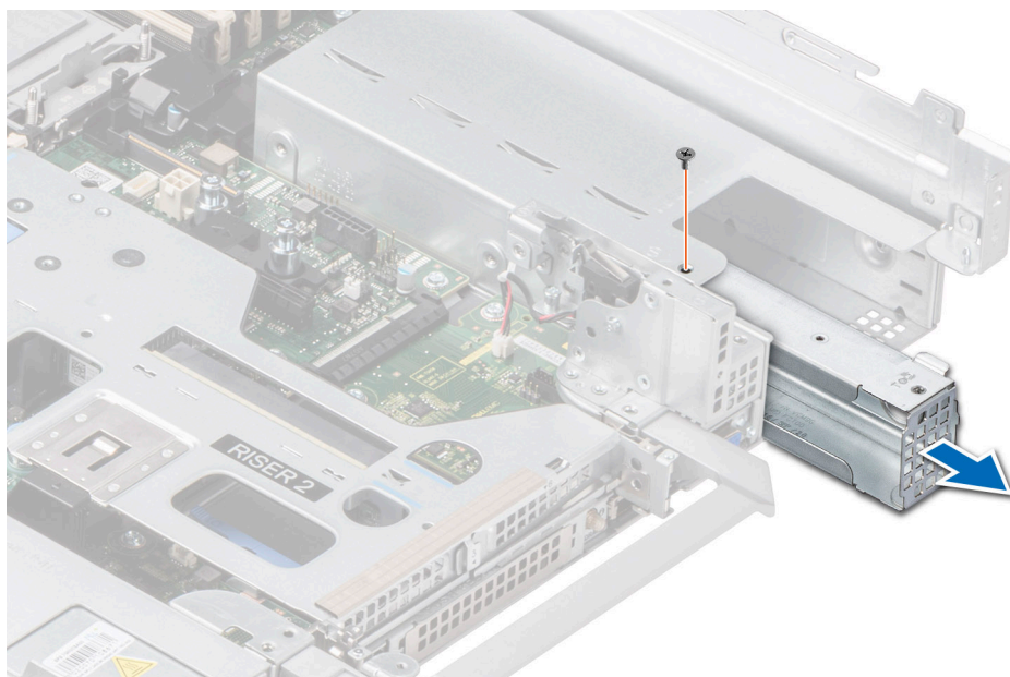
Ilustración 208. Extracción de un adaptador de fuente de alimentación
