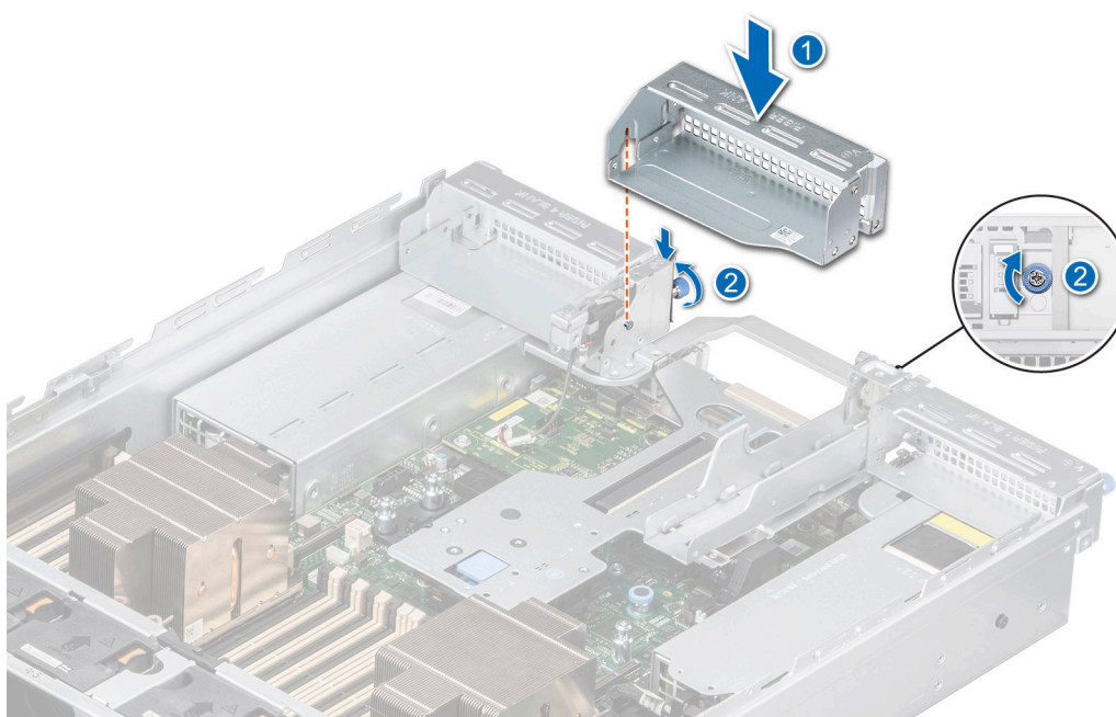
Ilustración 137. Instalación de la tarjeta elevadora de relleno 3
