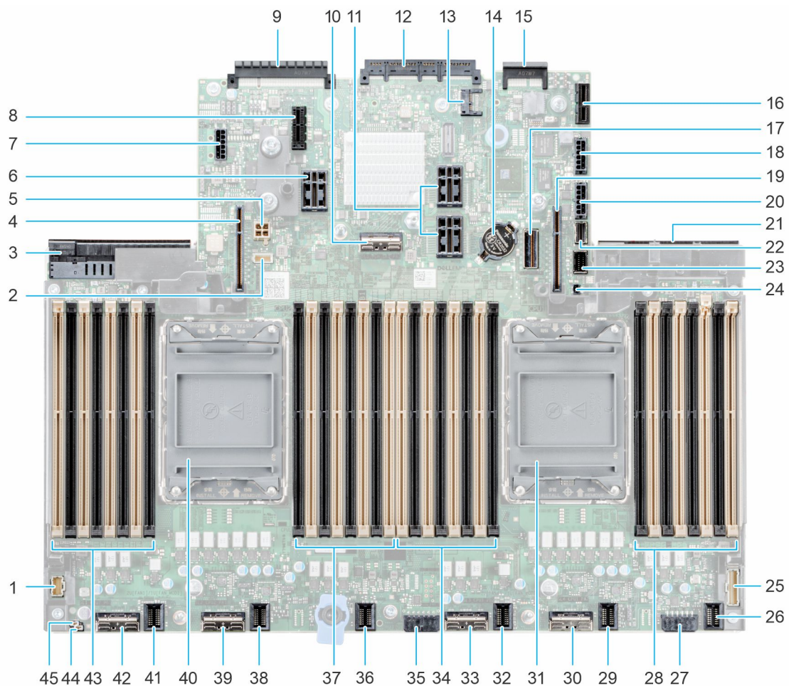
Ilustración 235. Puentes y conectores de la tarjeta madre del sistema
