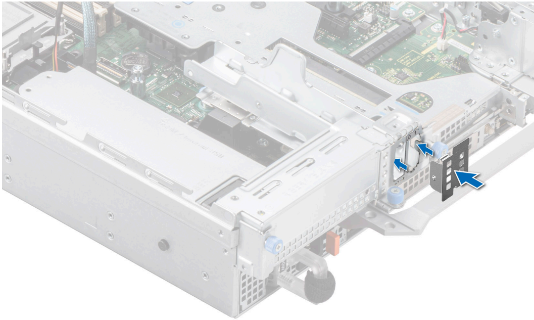
Ilustración 229. Instalación del módulo de Boot Optimized Storage Subsystem S2 de relleno
