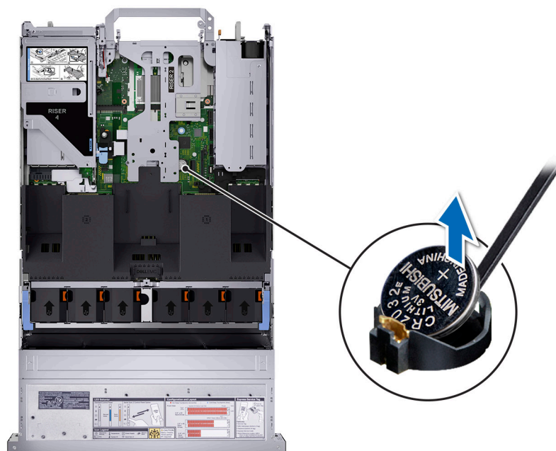
Ilustración 196. Extracción de la batería del sistema
