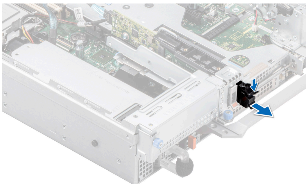
Ilustración 186. Extracción del soporte de tarjeta de Boot Optimized Storage Subsystem S2 de relleno
