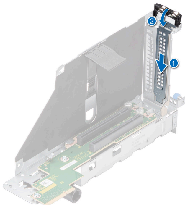
Ilustración 99. Instalación del soporte de relleno
