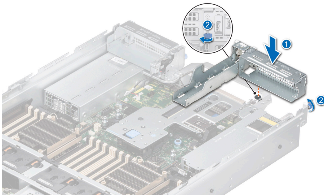
Ilustración 154. Instalación del soporte vertical de relleno 1
