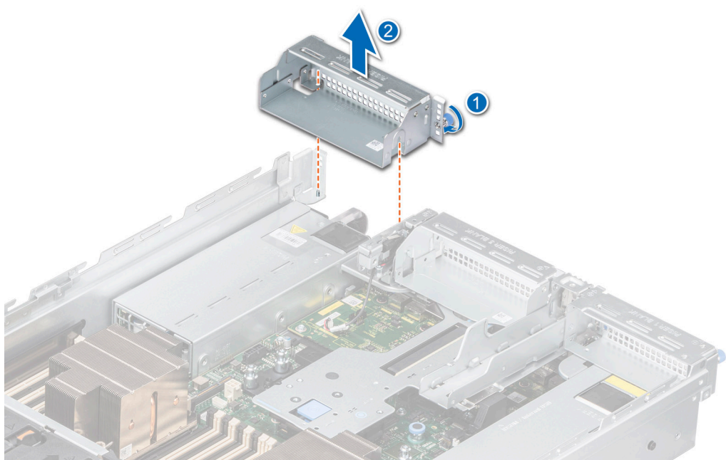
Ilustración 142. Extracción del soporte vertical de relleno 4
