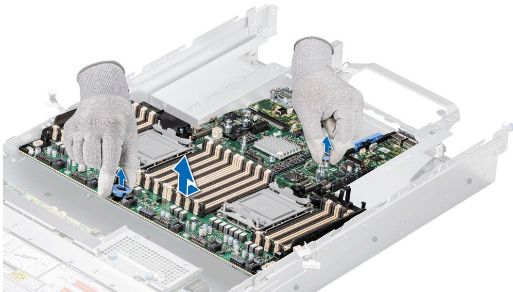
Ilustración 217. Extracción de la tarjeta madre
