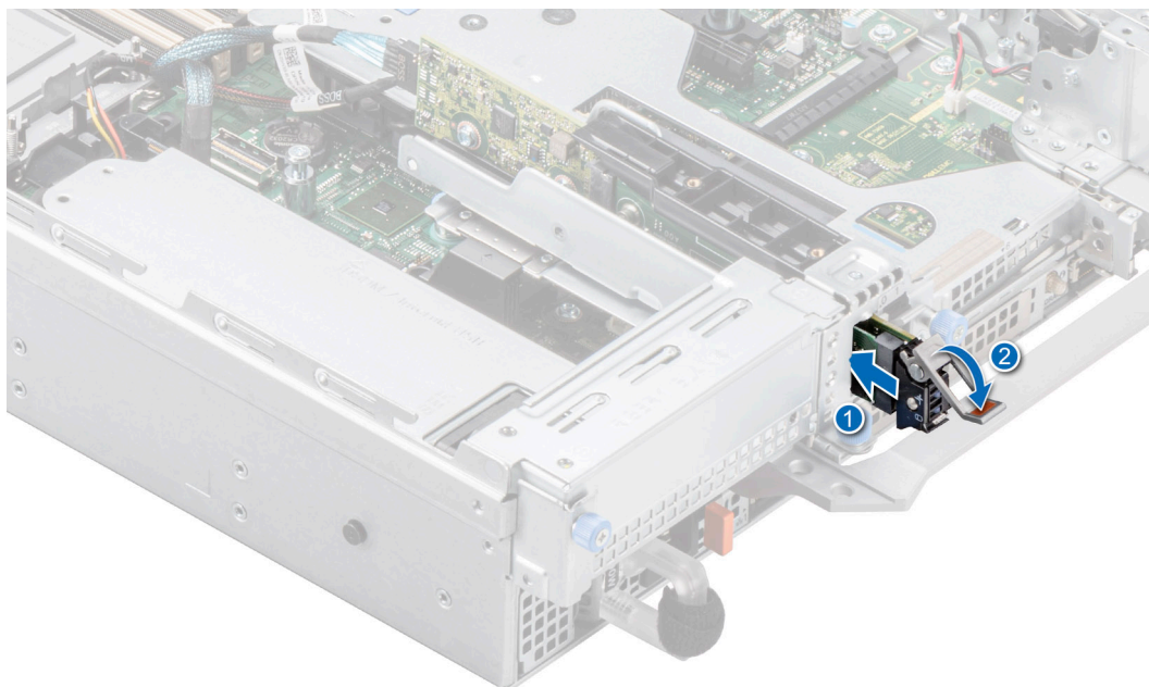
Ilustración 195. Instalación del portaunidades de tarjeta de Boot Optimized Storage Subsystem S2
