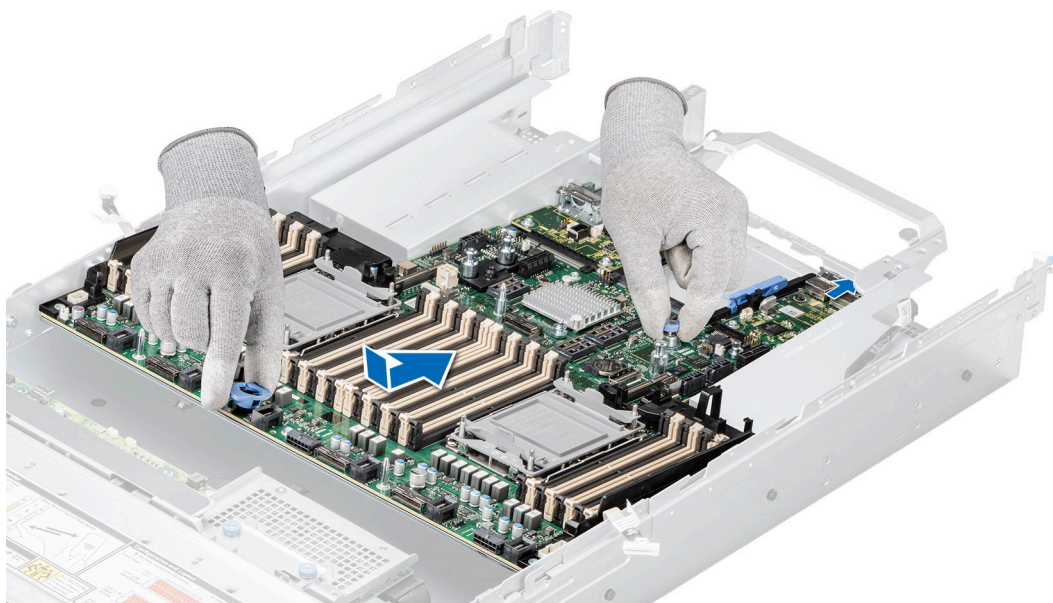
Ilustración 218. Instalación de la tarjeta madre
