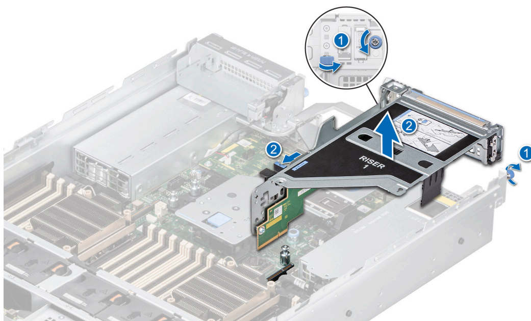
Ilustración 131. Extracción de la tarjeta elevadora para tarjetas de expansión (tarjeta elevadora 1)
