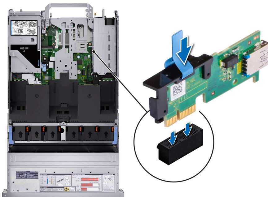
Ilustración 199. Instalación de la tarjeta USB interna
