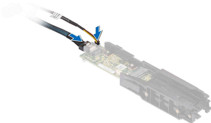
Ilustración 192. Conecte los cables de alimentación y de señal de Boot Optimized Storage Subsystem S2 al módulo de Boot Optimized Storage Subsystem S2.
