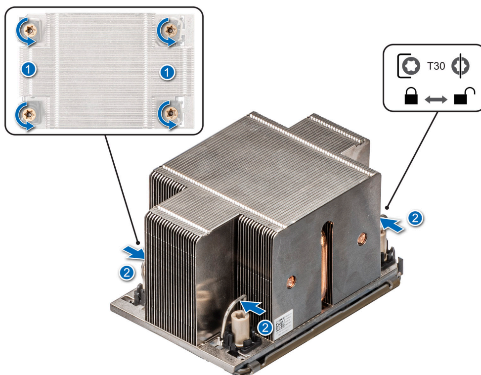
Ilustración 105. Extracción del módulo de disipador de calor del procesador.
