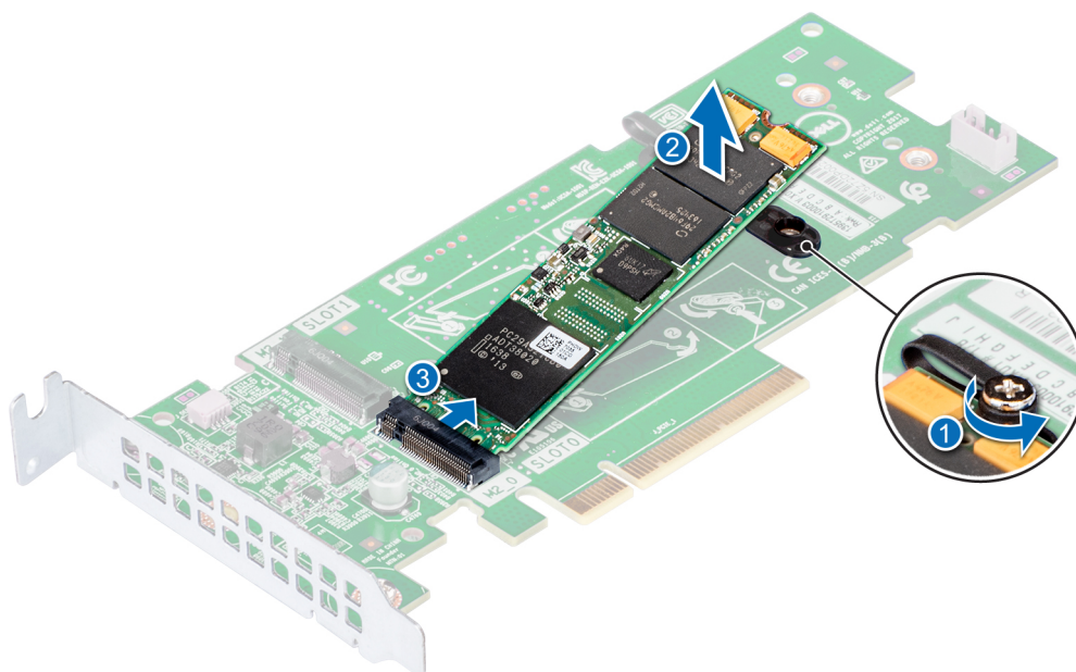
Ilustración 170. Extracción del módulo de SSD M.2
