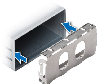
Ilustración 207. Instalación de una fuente de alimentación de relleno
