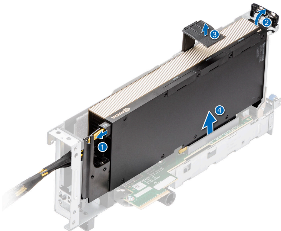
Ilustración 160. Extracción de la GPU del soporte vertical 1
