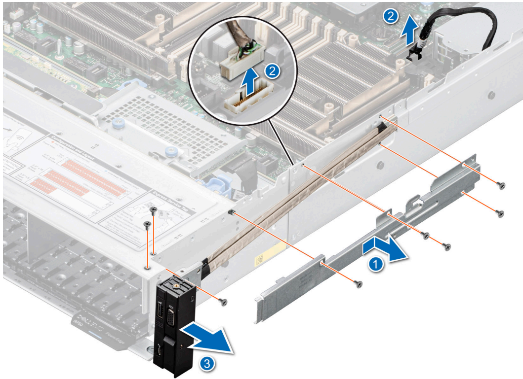
Ilustración 223. Extracción del panel de control derecho
