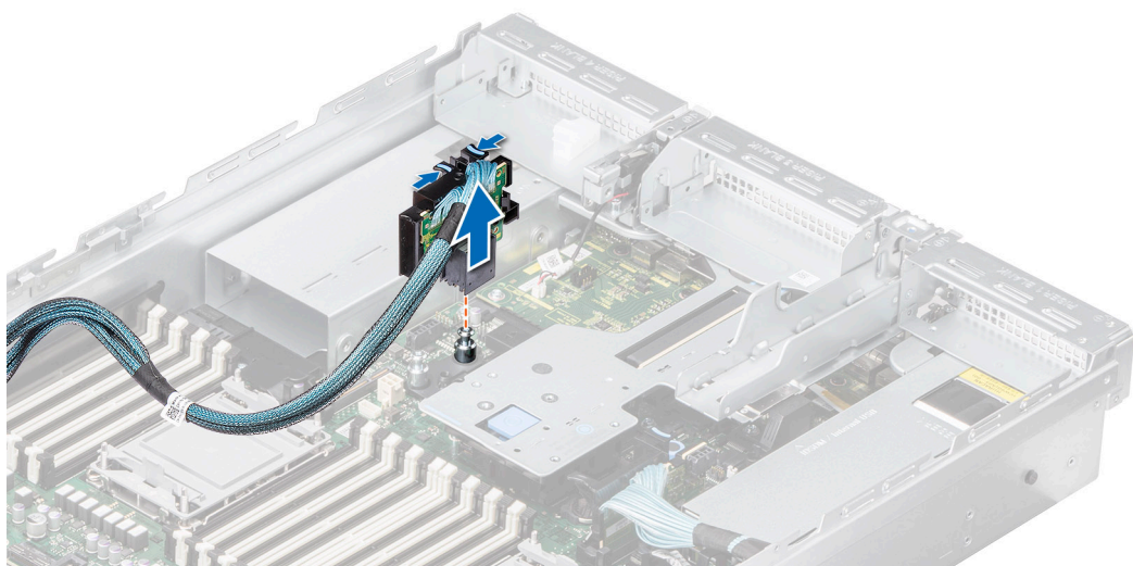
Ilustración 167. Extracción de la tarjeta de paleta R3
