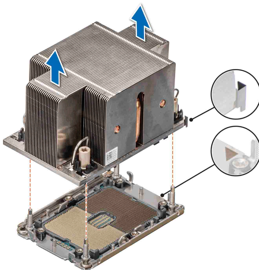
Ilustración 106. Extracción de un disipador de calor
