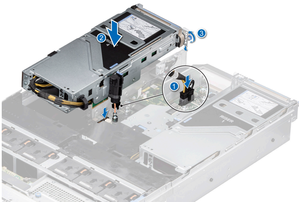
Ilustración 159. Instalación del soporte vertical para tarjetas de expansión (soporte vertical 4)
