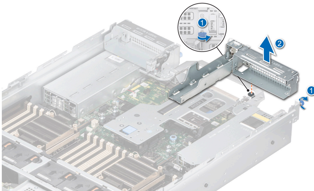
Ilustración 156. Extracción del soporte vertical de relleno 1
