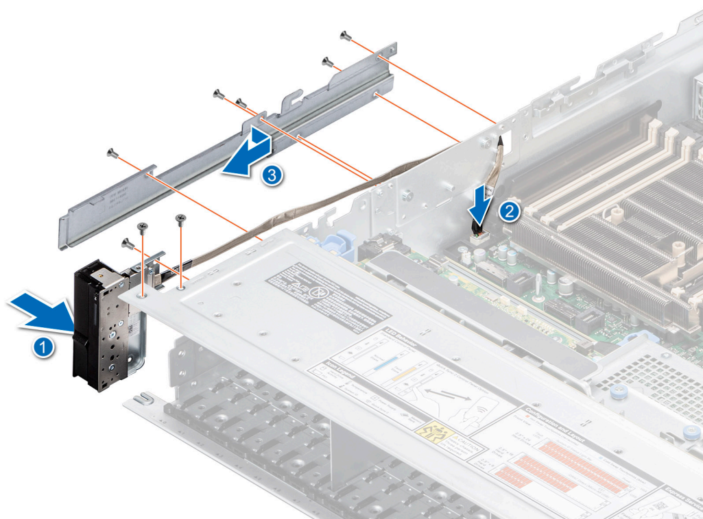
Ilustración 226. Instalación del panel de control izquierdo
