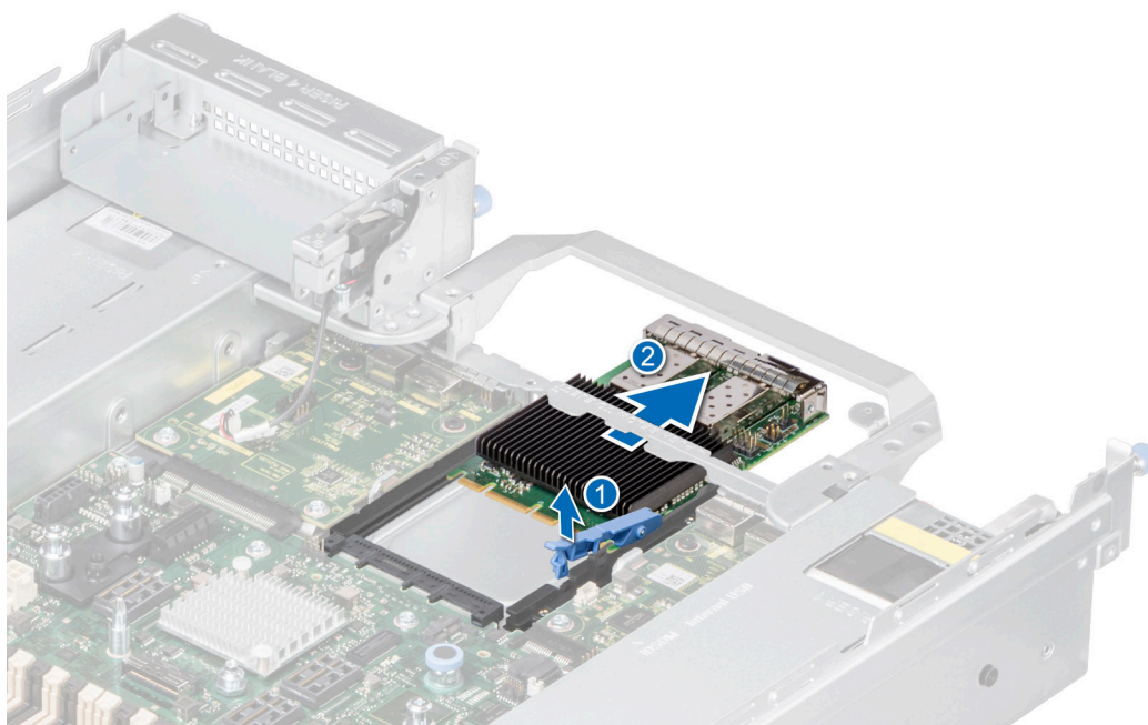
Ilustración 202. Extracción de la tarjeta OCP
