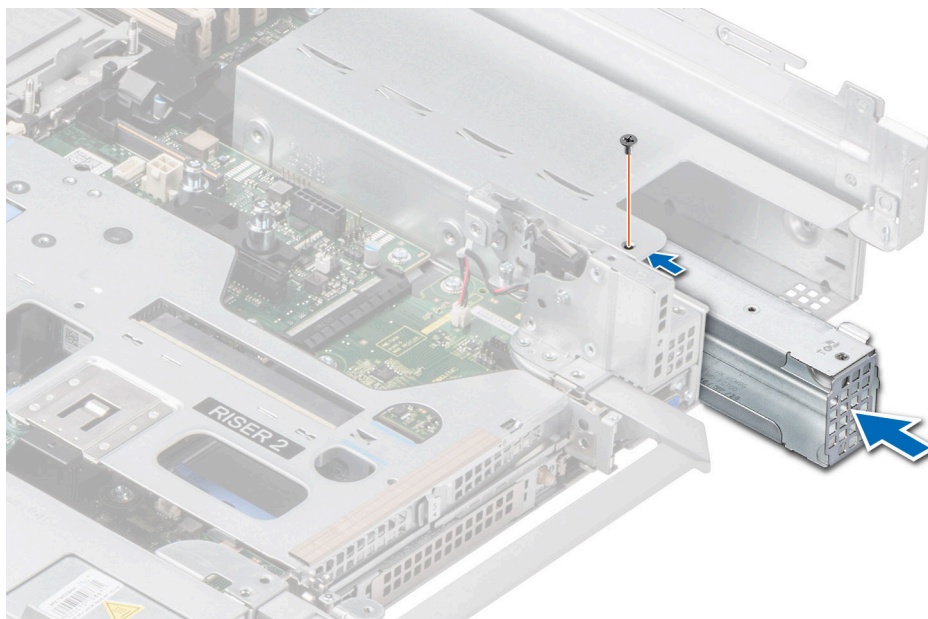
Ilustración 209. Instalación de un adaptador de fuente de alimentación
