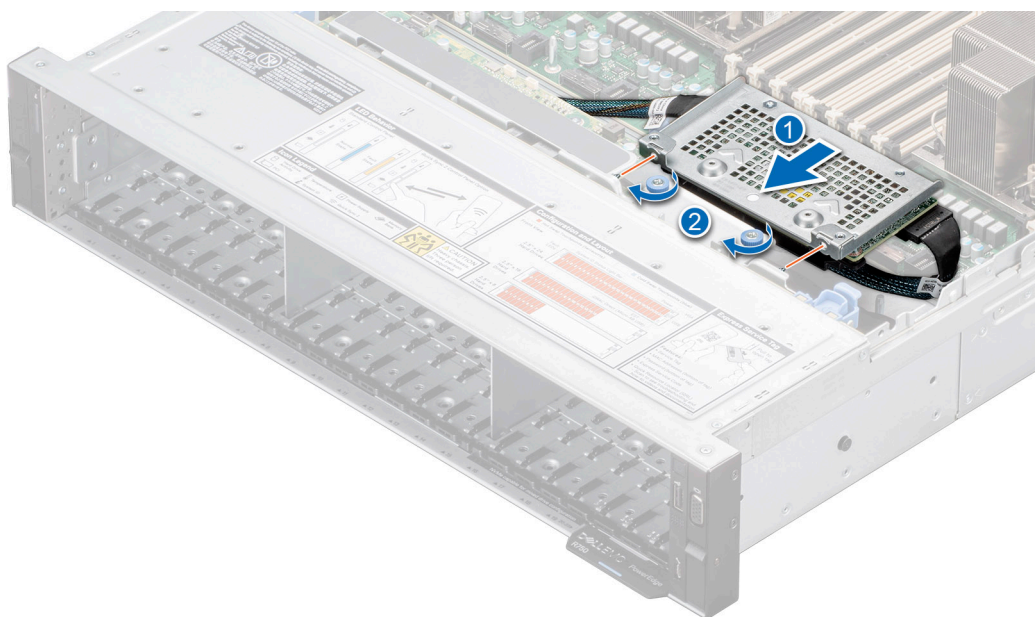
Ilustración 97. Instalación del módulo de PERC frontal de montaje posterior
