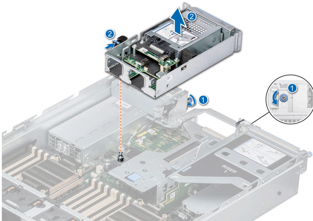
Ilustración 57. Extracción del módulo posterior de 2 unidades de 2,5 pulgadas
