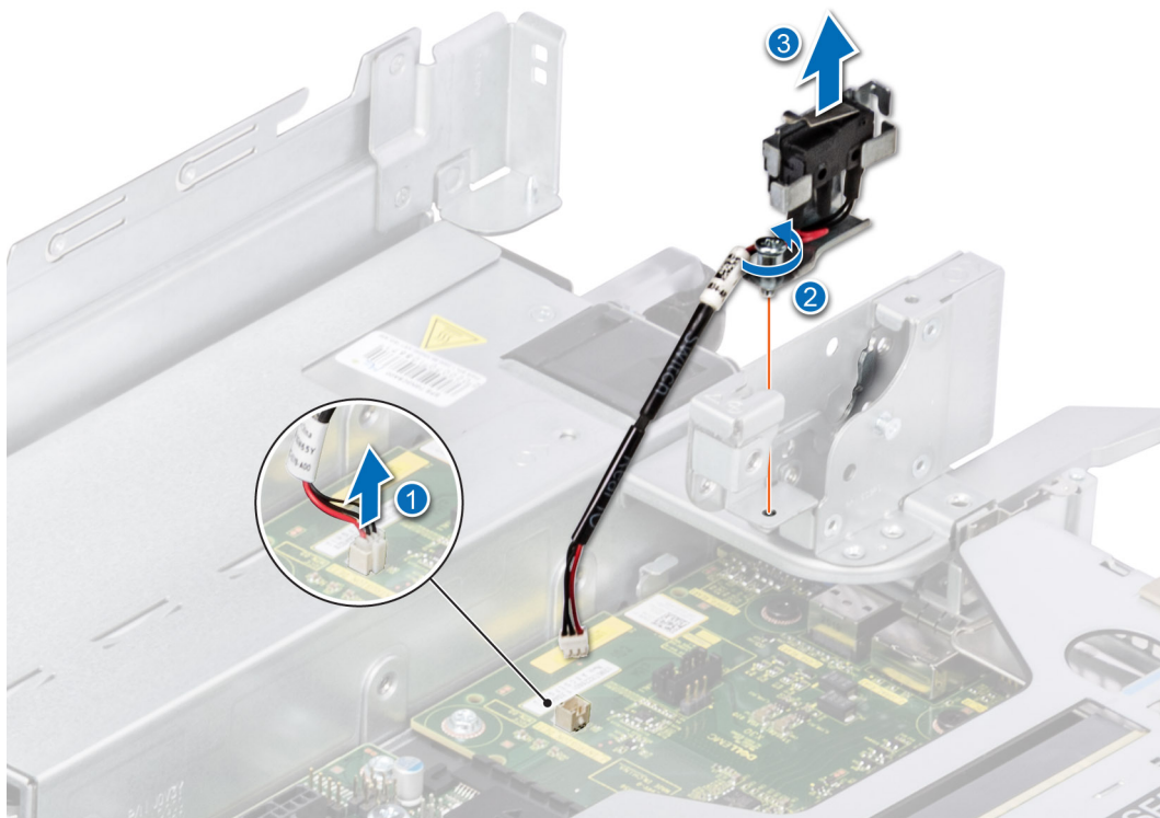
Ilustración 200. Extracción del módulo del interruptor de intrusiones
