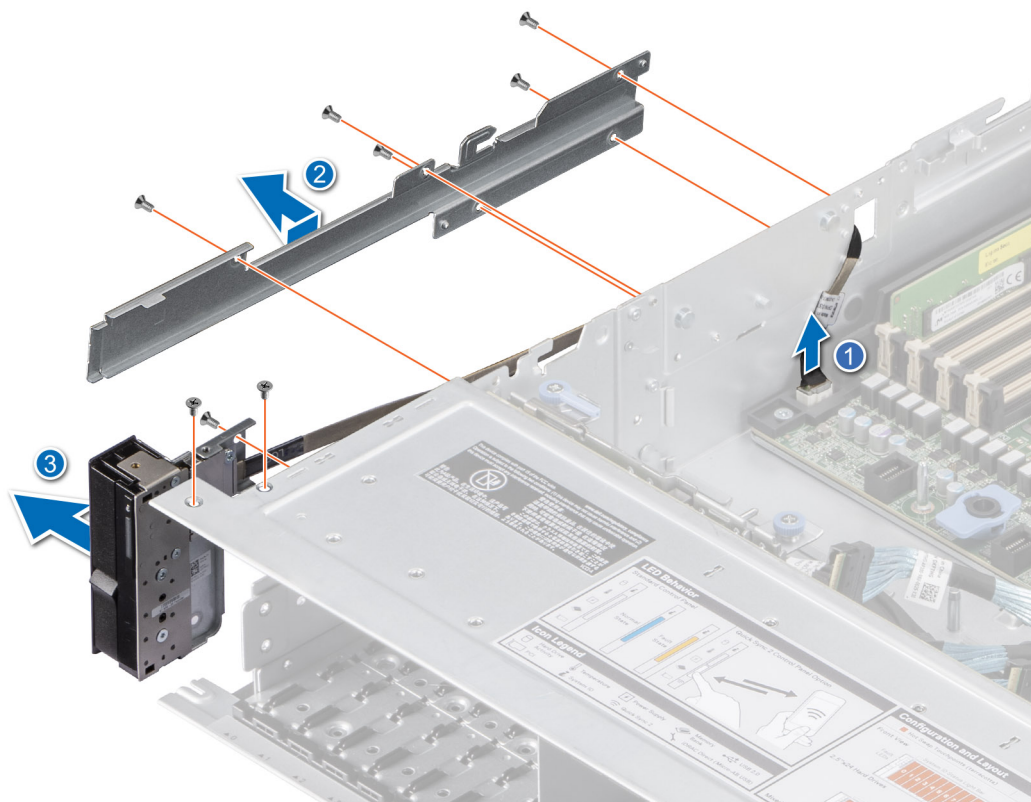
Ilustración 225. Extracción del panel de control izquierdo
