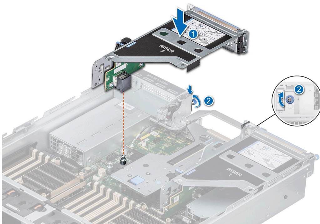
Ilustración 145. Instalación del soporte vertical para tarjetas de expansión (soporte vertical 3)
