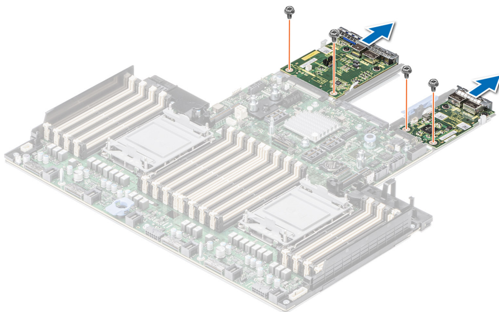
Ilustración 219. Extracción de la tarjeta LOM y la placa de I/O posterior
