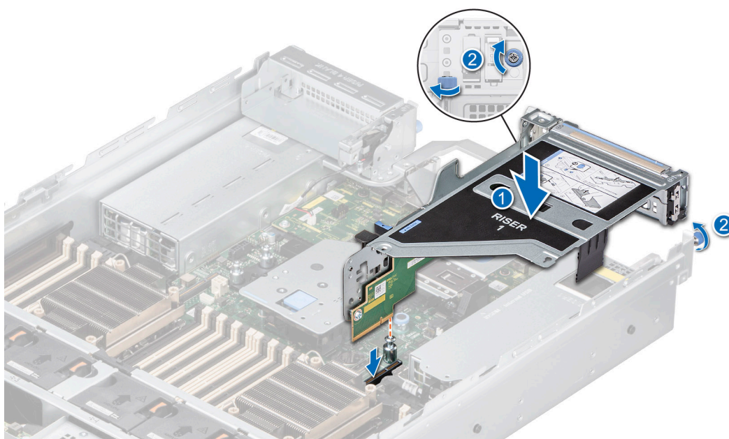
Ilustración 144. Instalación del soporte vertical para tarjetas de expansión (soporte vertical 1)
