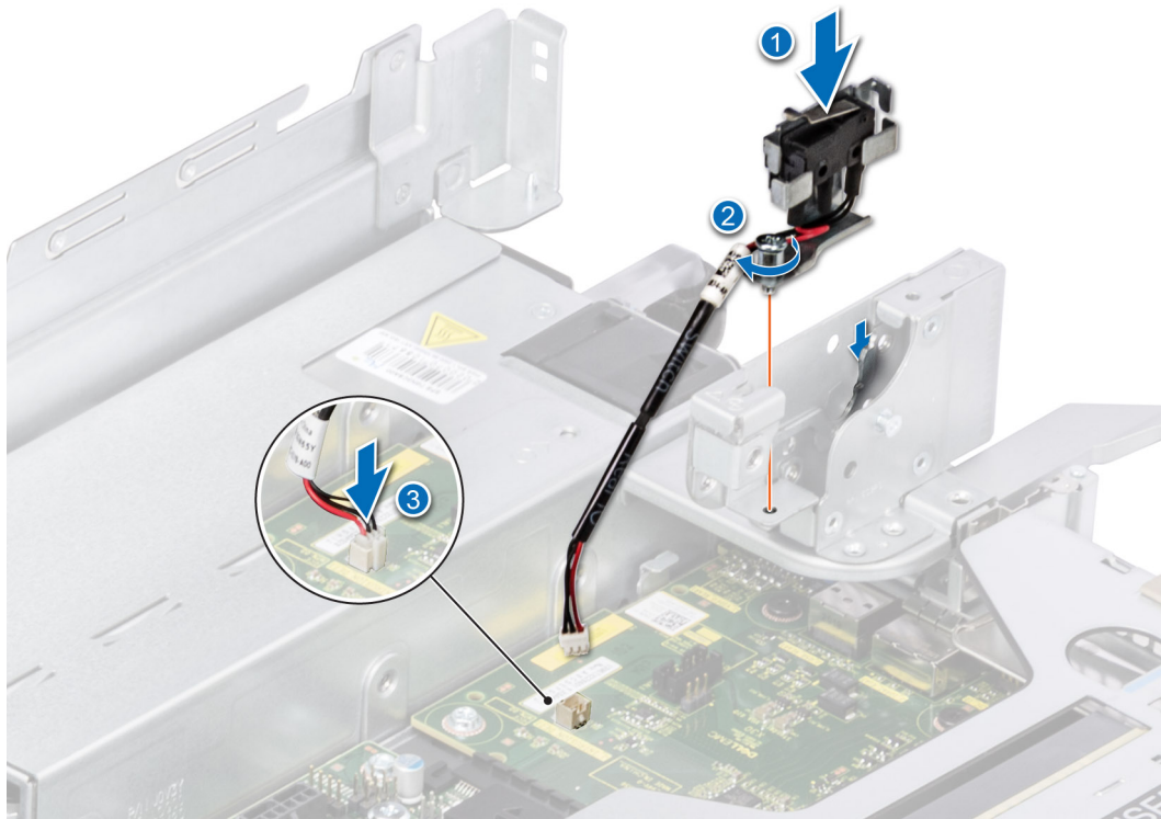
Ilustración 201. Instalación del módulo del interruptor de intrusiones
