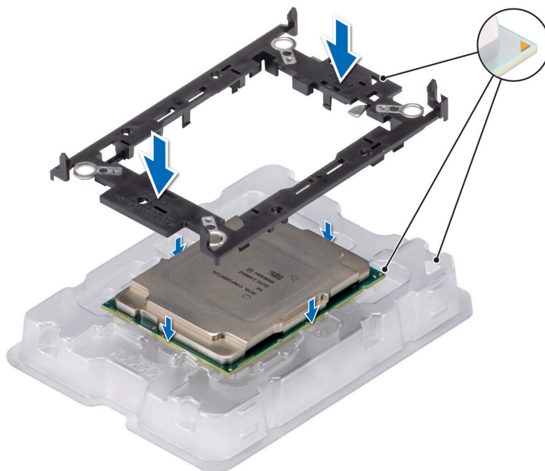
Ilustración 109. Instalación del gancho de retención
