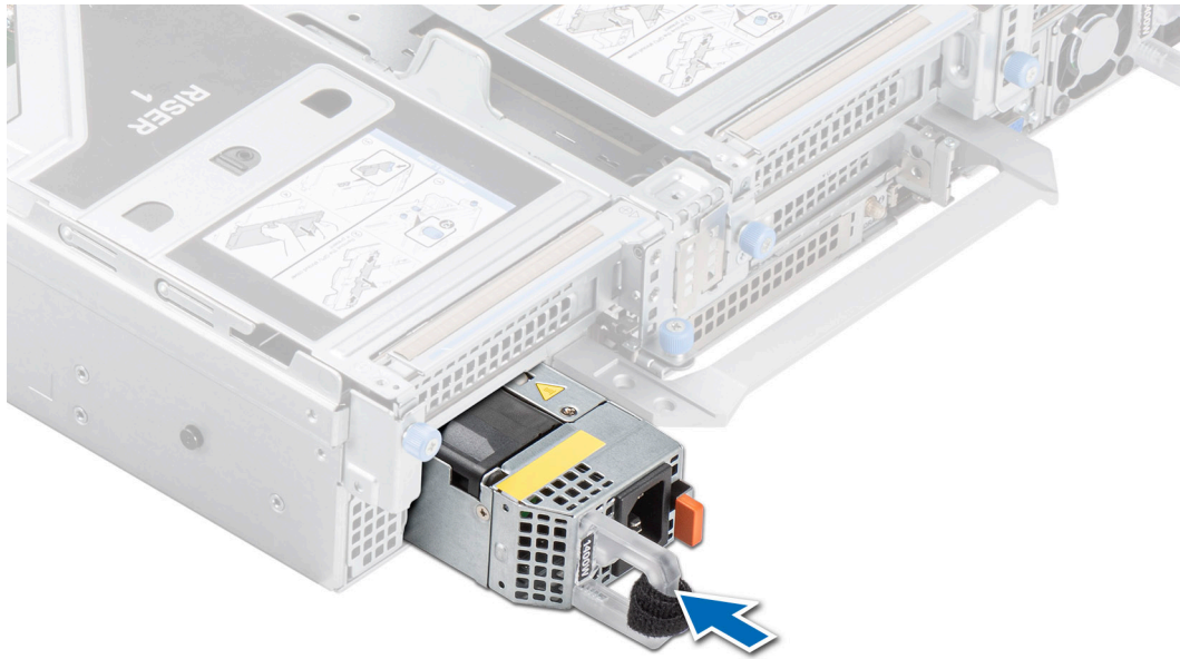
Ilustración 211. Instalación de una fuente de alimentación
