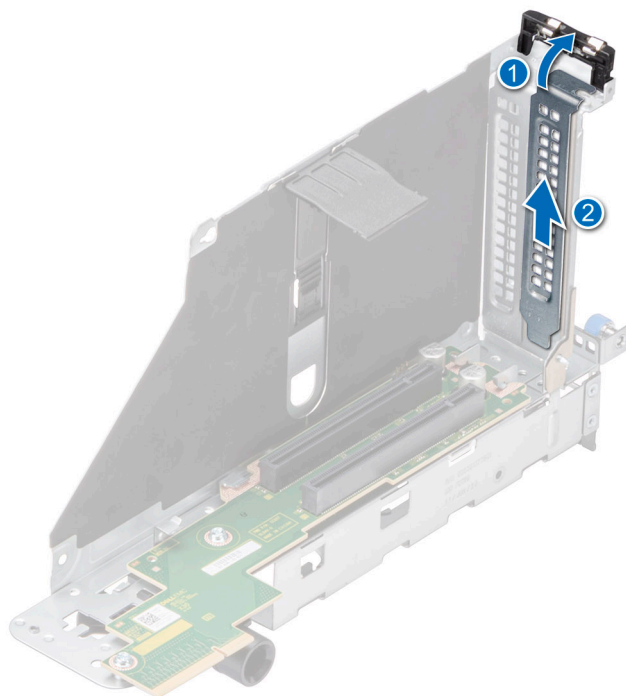
Ilustración 100. Extracción del soporte de relleno
