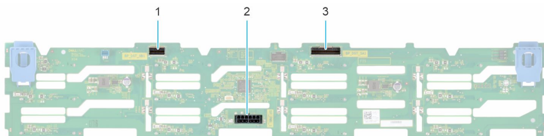
Ilustración 60. Backplane de 12 unidades de 3,5 pulgadas
