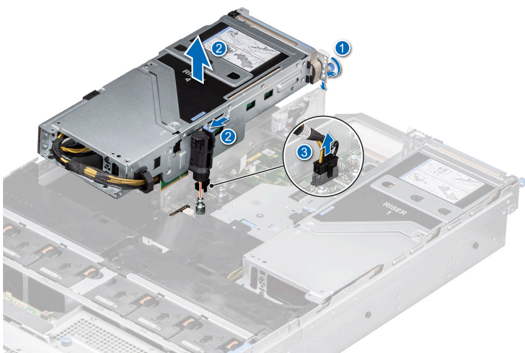
Ilustración 153. Extracción del soporte vertical para tarjetas de expansión (soporte vertical 4)
