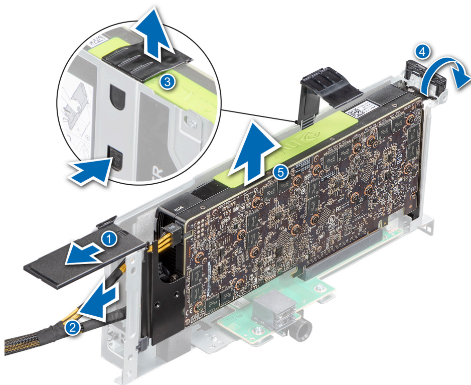
Ilustración 161. Extracción de la GPU del soporte vertical 4
