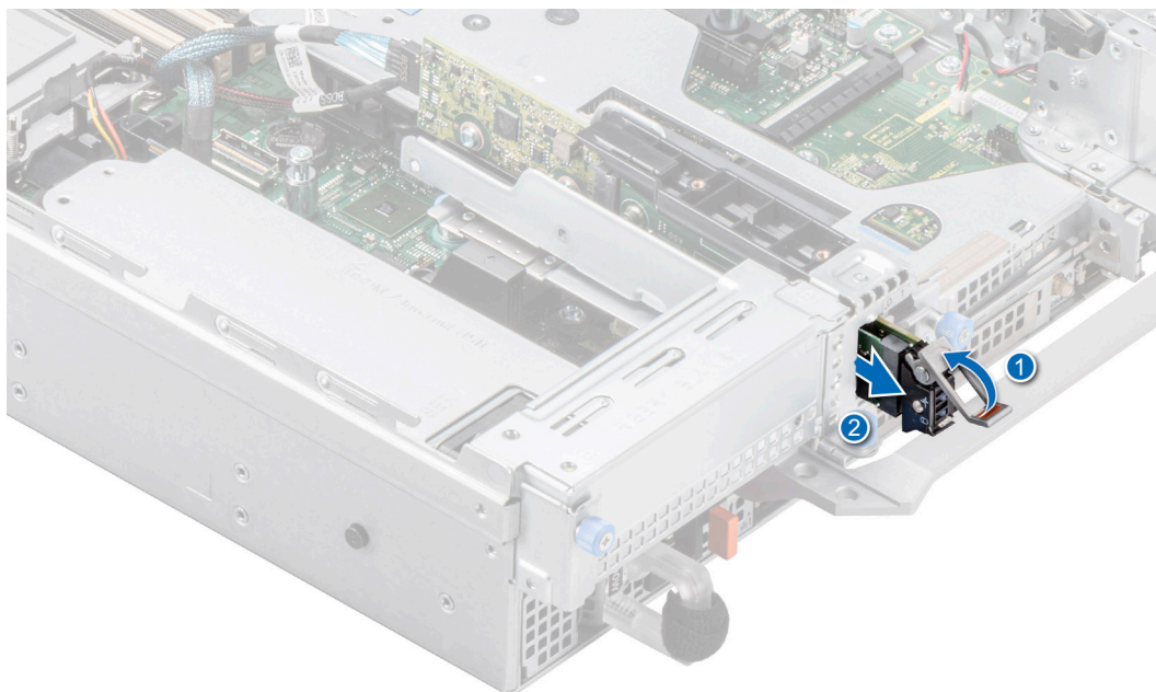
Ilustración 188. Extracción del portaunidades de tarjeta de Boot Optimized Storage Subsystem S2
