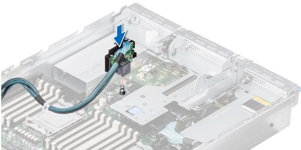
Ilustración 169. Instalación de la tarjeta de paleta R3
