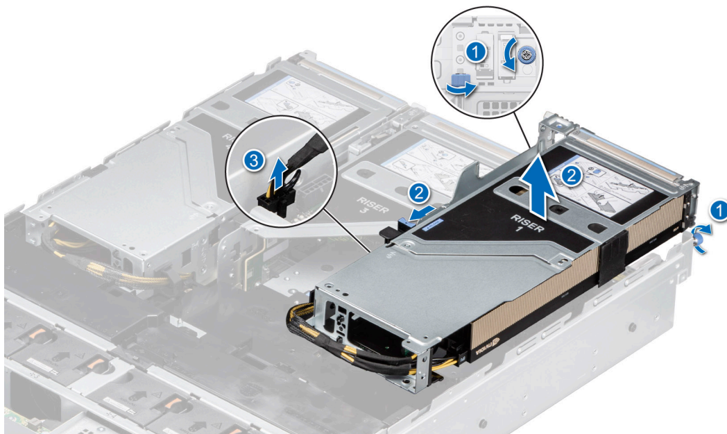
Ilustración 152. Extracción del soporte vertical para tarjetas de expansión (soporte vertical 1)
