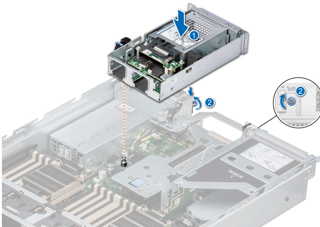
Ilustración 58. Instalación del módulo posterior de 2 unidades de 2,5 pulgadas
