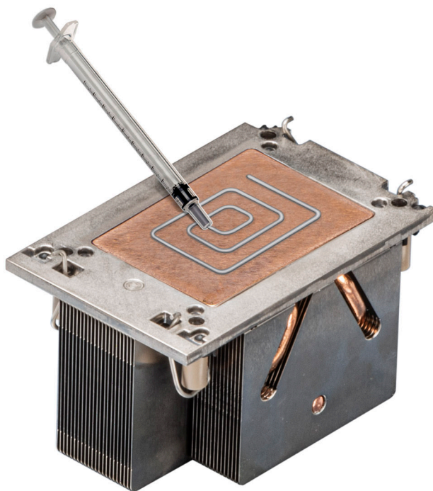
Ilustración 111. Aplicación de la grasa térmica
