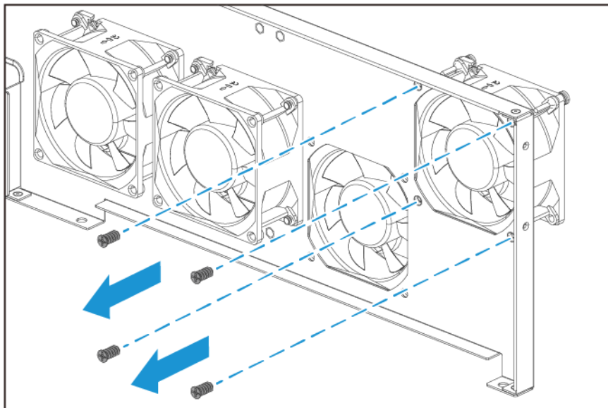
2,5-Zoll Laufwerksschachtlüfter
