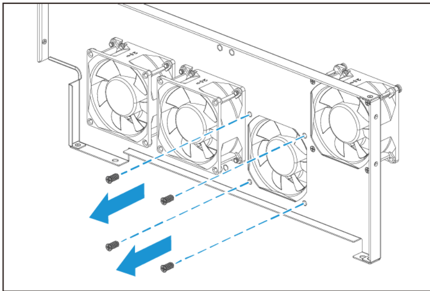
CPU-Lüfter
