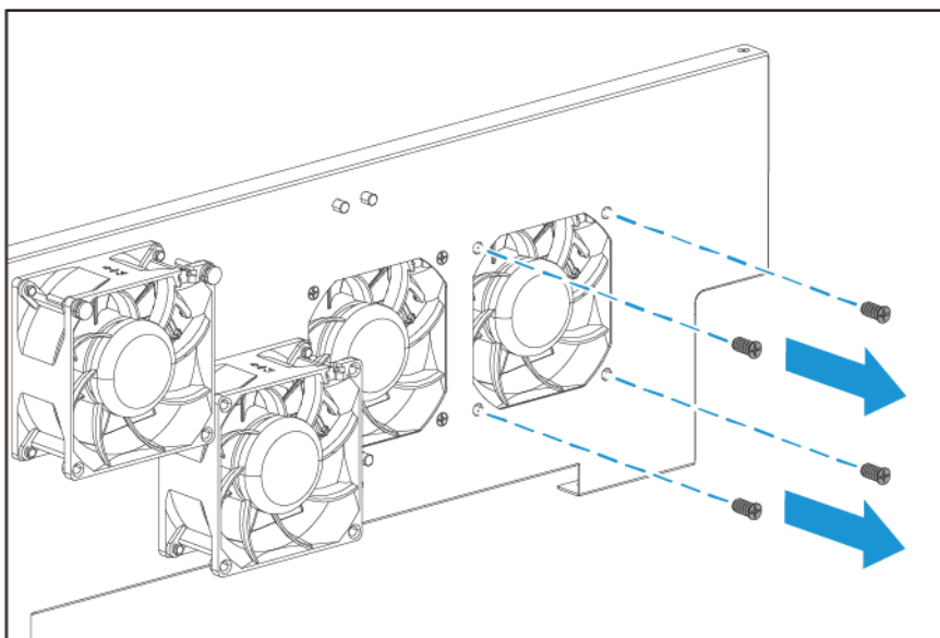
Systemlüfter
