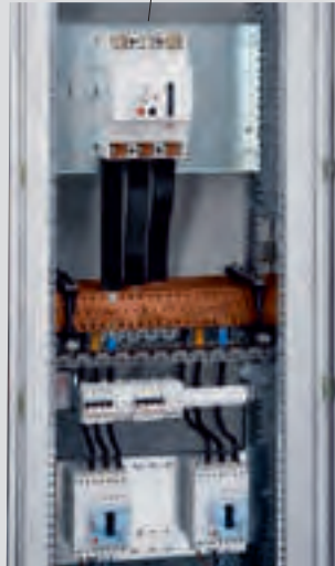
Montage d'un DPX 3 1600 A et d'un DPX 250 A (vue intérieure d'armoire, plastrons ôtés)
