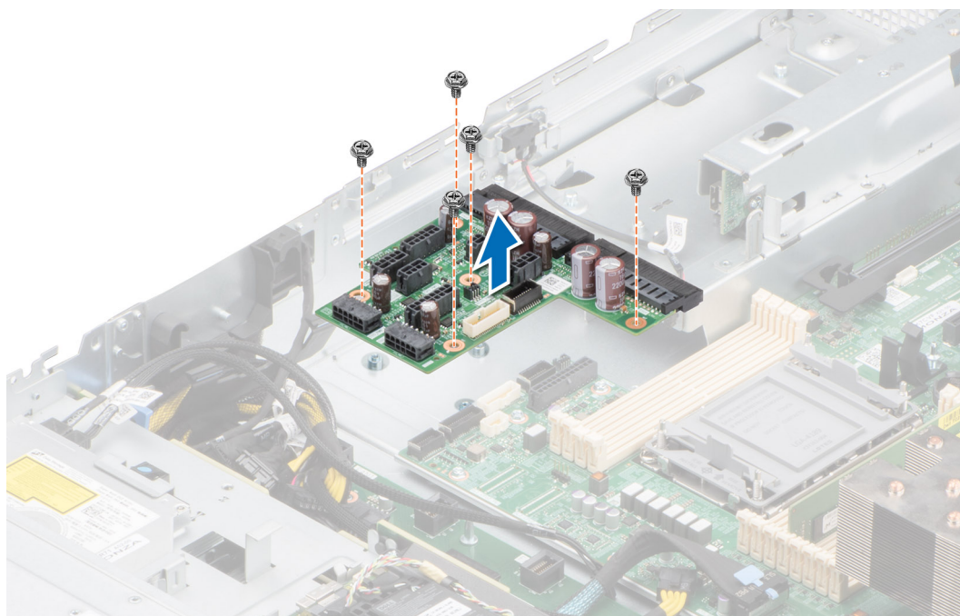
Abbildung 102. Stromzwischenplatine entfernen
