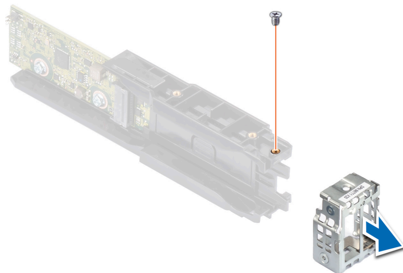
Abbildung 79. Entfernen der BOSS-Abdeckung
