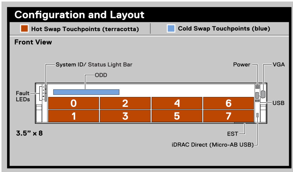
Abbildung 13. Konfiguration und Layout
