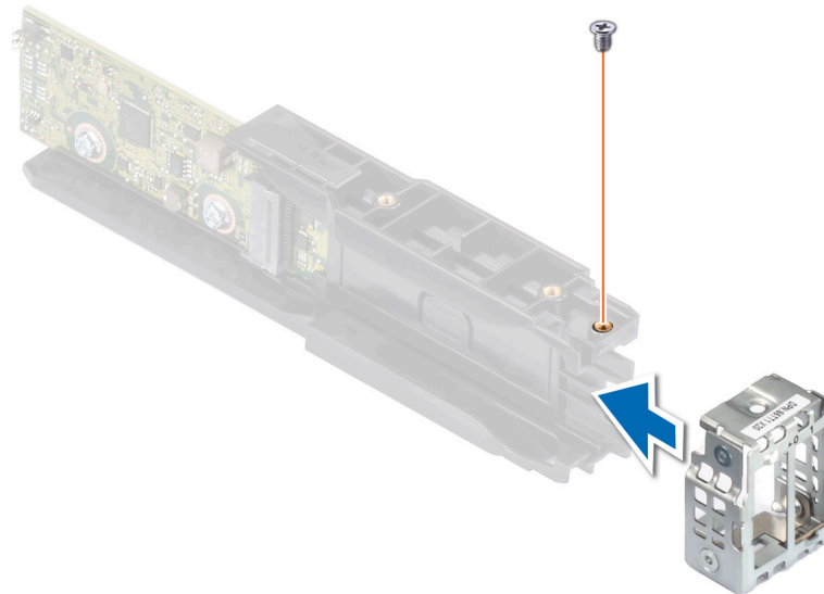
Abbildung 80. Installieren der BOSS-Abdeckung
