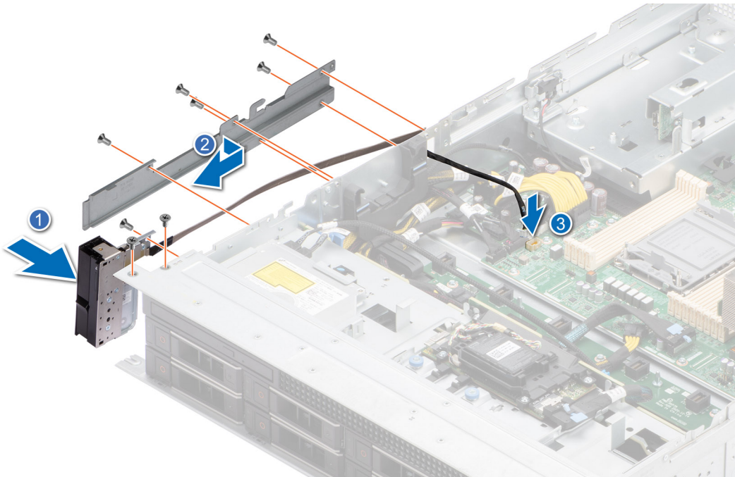
Abbildung 110. Installieren des linken Bedienfelds
