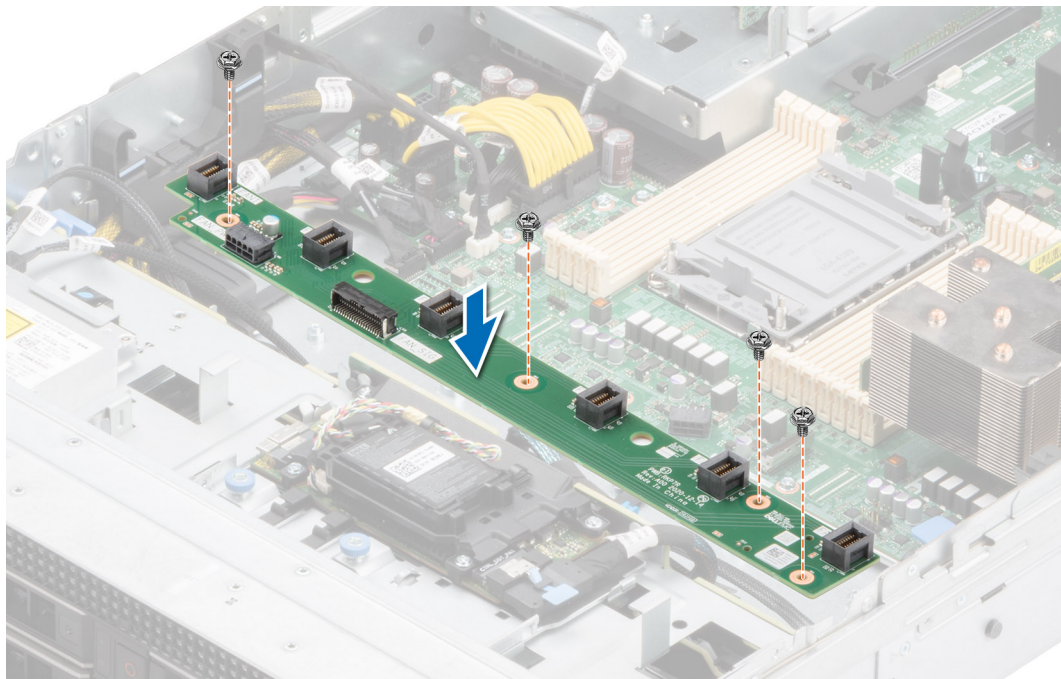
Abbildung 105. Installieren der Lüftergehäuseplatine
