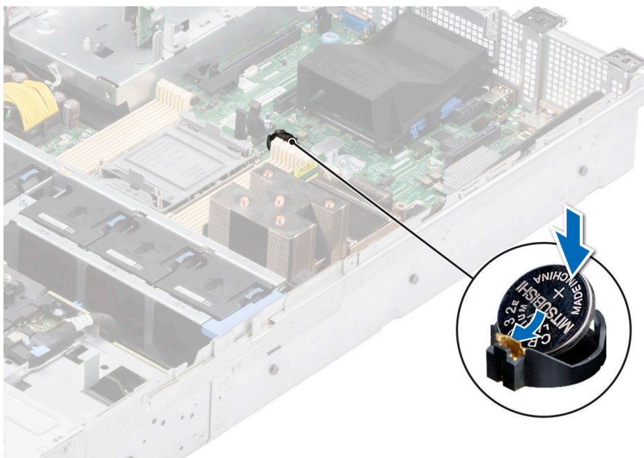
Figure 93. Installation de la pile du système
