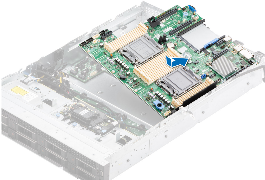
Figure 107. Installation de la carte système
