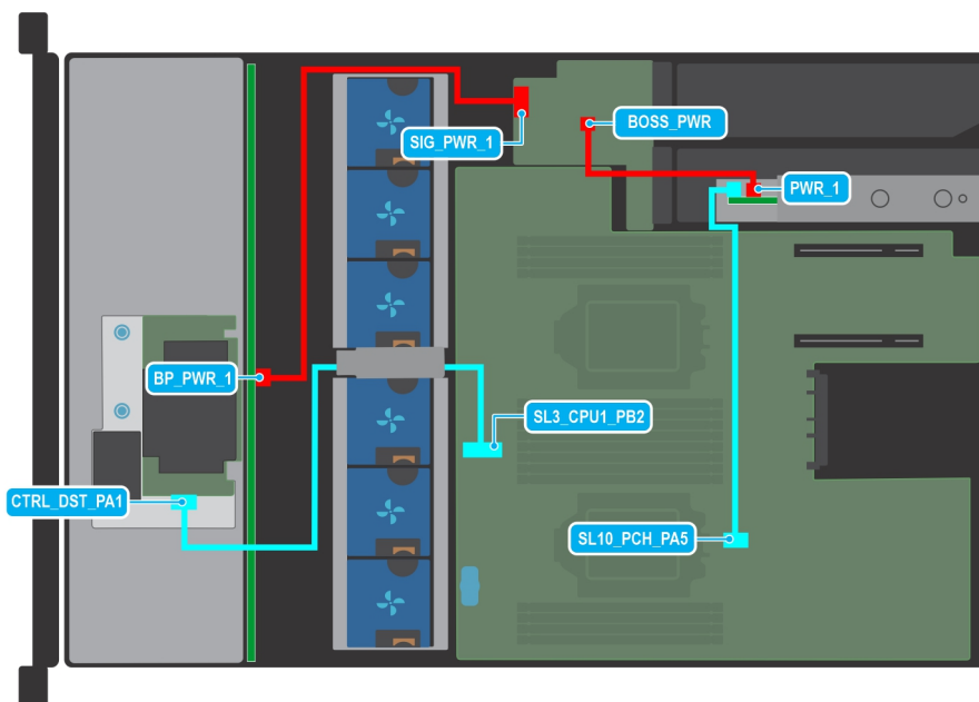
Figure 48. 8 disques SAS/SATA de 3,5 pouces
