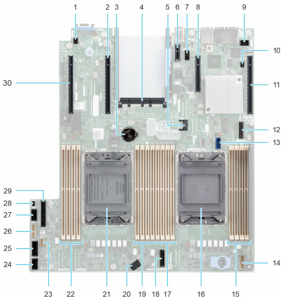
Figure 115. Connecteurs et cavaliers de la carte système
