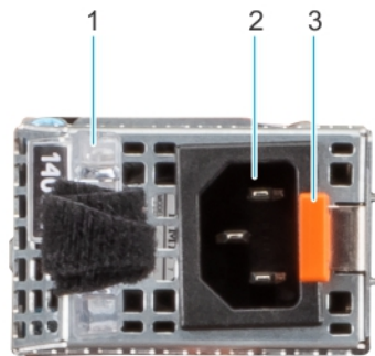
Figure 120. Voyant d'état du bloc d'alimentation secteur
