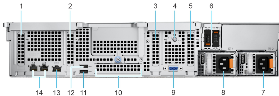
Figure 7. Vue arrière du système
