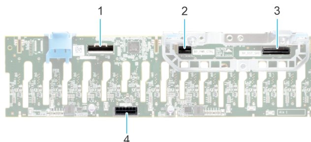
Figure 42. Fond de panier SAS/SATA de 16 disques de 2,5 pouces
