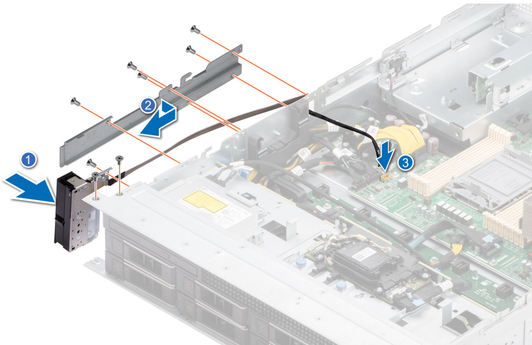
Figure 110. Installation du panneau de configuration gauche
