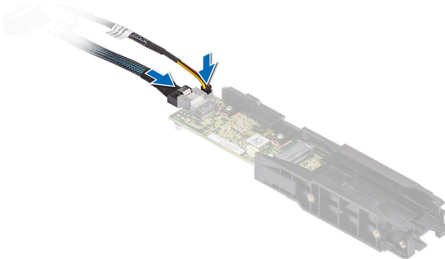
Figure 81. Connexion du câble d'alimentation du Boot Optimized Storage Subsystem et du câble de signal du Boot Optimized Storage Subsystem au module Boot Optimized Storage Subsystem S2
