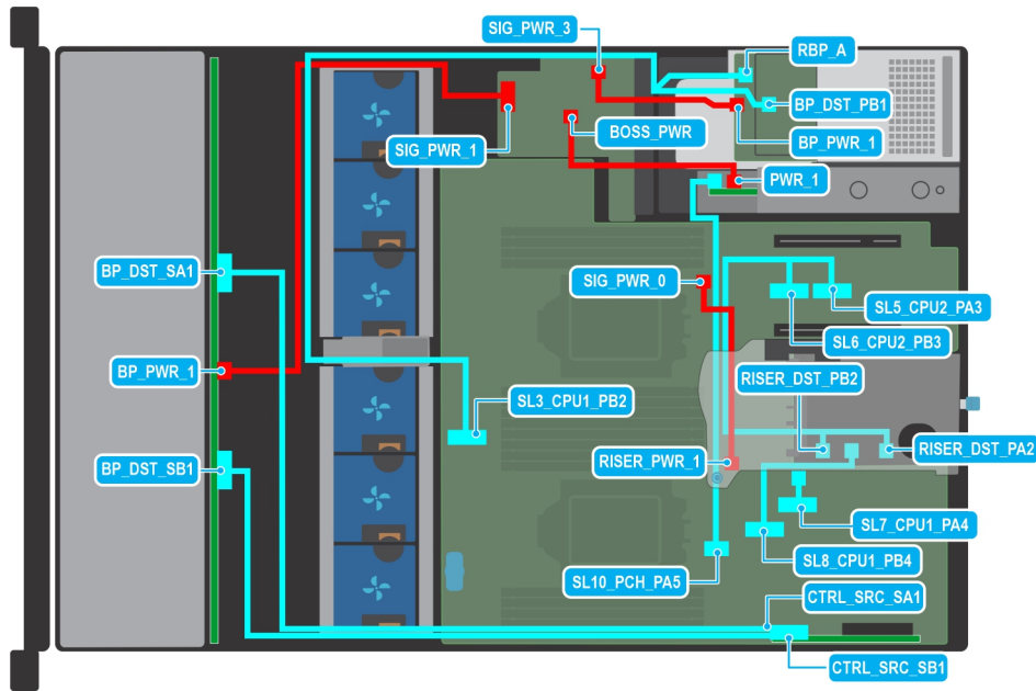
Abbildung 59. Kabelführung: 12 x 3,5-Zoll-SAS/SATA-Laufwerkrückwandplatte + hinterer 2 x 2,5-Zoll-NVMe mit Kabel-Riser 1A und BOSS-S2-Karte
