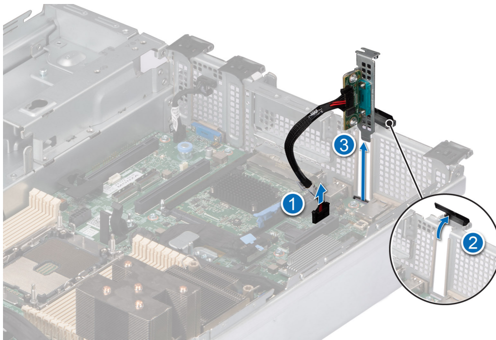
Abbildung 37. Entfernen des seriellen COM-Ports
