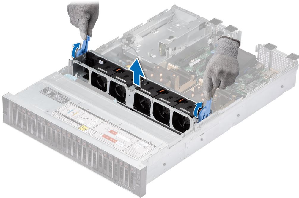
Abbildung 29. Entfernen des Kühlungs-Lüftergehäuses
