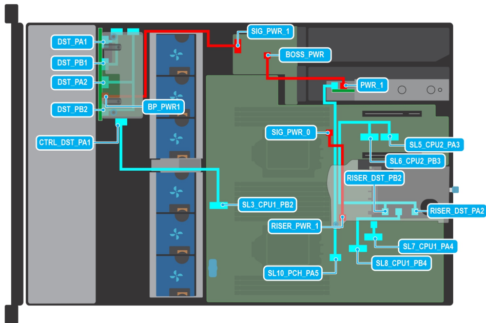
Abbildung 57. Kabelführung: 8 x 2,5-Zoll-NVMe-Laufwerkrückwandplatte zum vorderen PERC mit Kabel-Riser 1A und BOSS-S2-Karte
