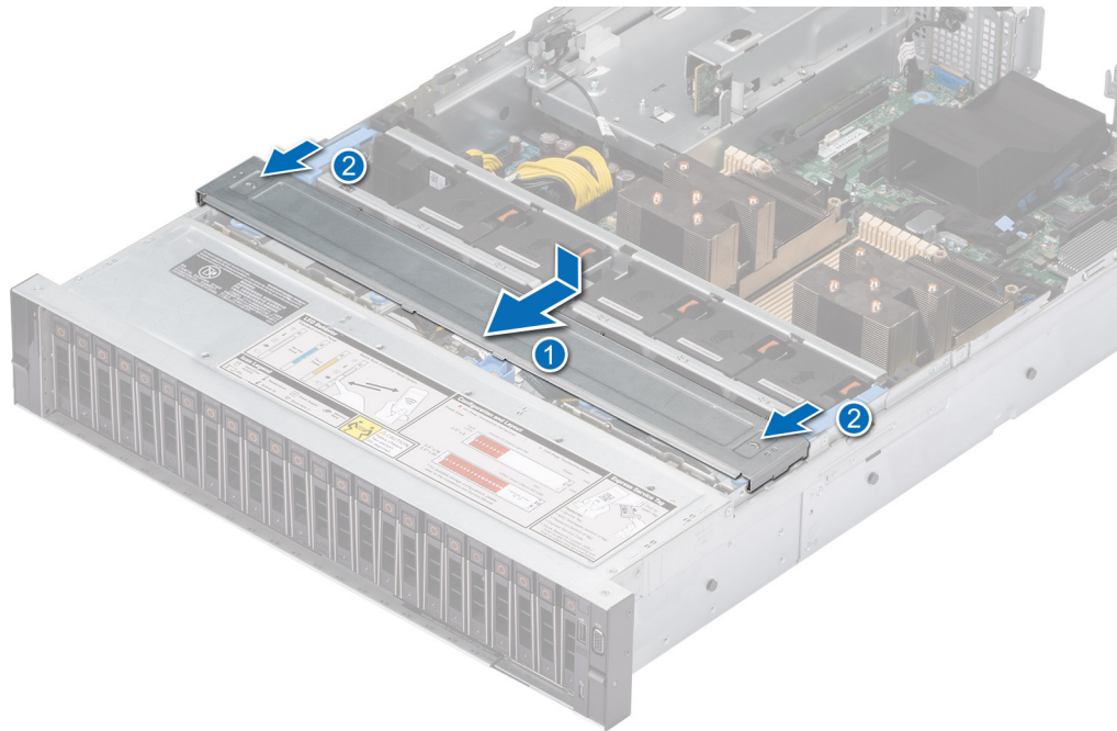
Abbildung 22. Installieren der Rückwandplattenabdeckung
