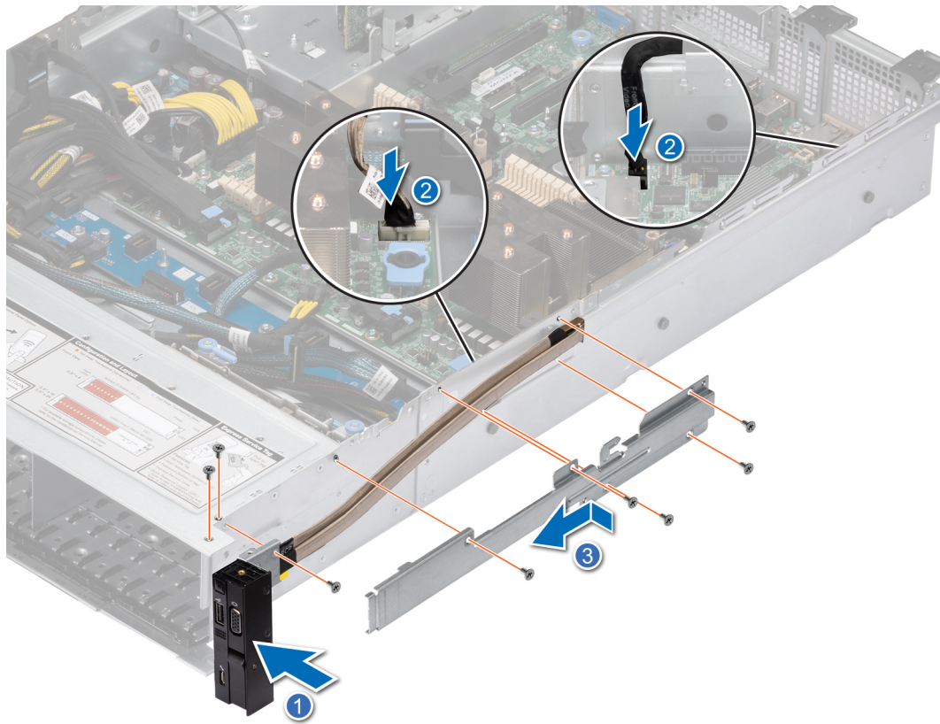
Abbildung 132. Installieren des rechten Bedienfelds
