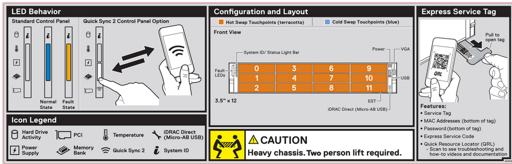
Abbildung 14. LED-Verhalten, Konfiguration und Layout, Express-Service-Tag für 3,5-Zoll-Laufwerksystem
