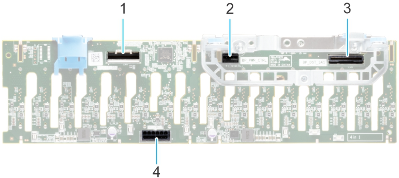
Abbildung 45. 16 x 2,5-Zoll-SAS/SATA-Rückwandplatine
