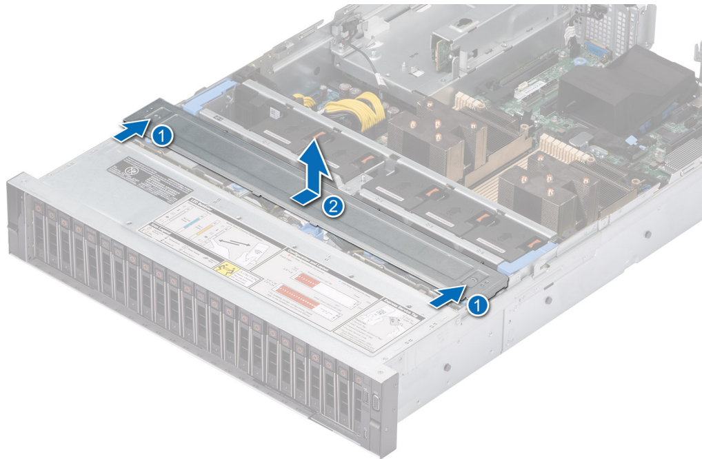
Abbildung 21. Entfernen der Laufwerk-Rückwandplattenabdeckung
