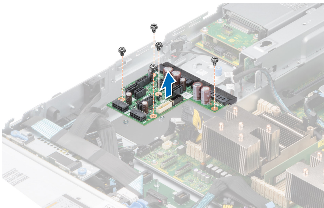
Abbildung 124. Stromzwischenplatine entfernen
