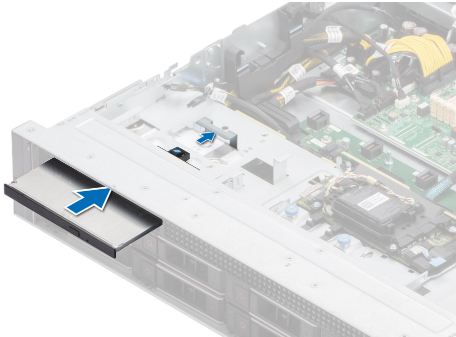
Abbildung 24. Installieren des optischen Festplattenlaufwerks
