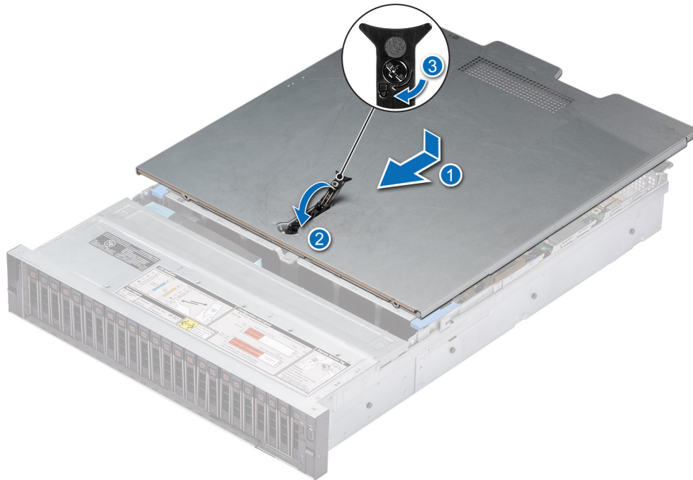
Abbildung 20. Systemabdeckung anbringen
