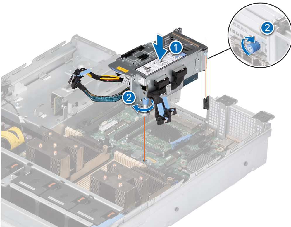
Abbildung 83. Installieren des Risers 1B
