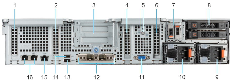
Abbildung 8. Rückansicht des Systems
