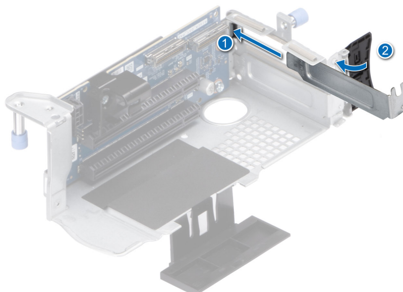
Abbildung 86. Installieren des Abdeckblechs in Riser 1A und Riser 1B
