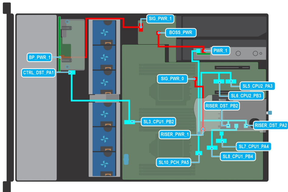
Abbildung 55. Kabelführung: 8 x 2,5-Zoll-SAS/SATA-Laufwerkrückwandplatte zum vorderen PERC mit Kabel-Riser 1A und BOSS-S2-Karte
