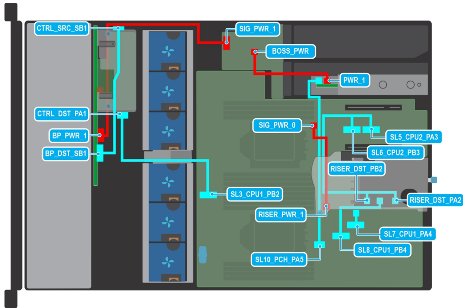
Abbildung 60. Kabelführung: 16 x 2,5-Zoll-Laufwerkrückwandplatte zum vorderen PERC mit-Riser 1A und BOSS-S2-Karte
